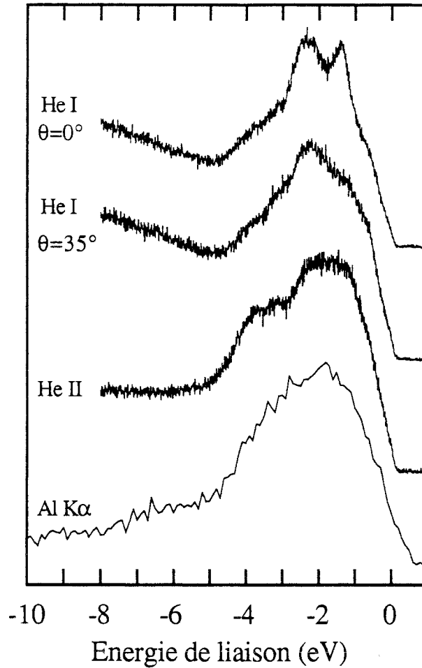
Figure III-38: Spectres de bandes de valence enregistrés en He I, He II et Al K\alpha sur un dépôt de 64 Å recuit à 550°C. Les spectres enregistrés en He I présentent une dispersion angulaire semblable à celle observée sur Pd(111) (Fig. III-9).
