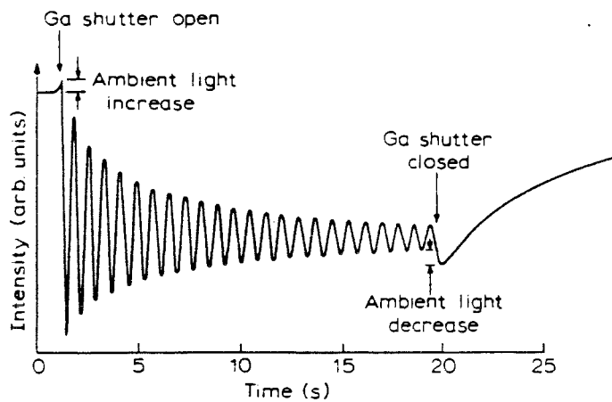
Figure II-19: Oscillations d'intensité de la réflexion directe d'un diagramme RHEED au cours de la croissance de GaAs. La période des oscillations correspond à la formation d'une monocouche de Ga+As. (d'après [23])
