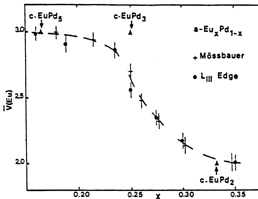
Figure III-5: Evolution de la valence moyenne de l'euprimum dans les alliages amorphes \text{Eu}_x\text{Pd}_{1-x} en fonction de la concentration x en europium. (d'après [14])
