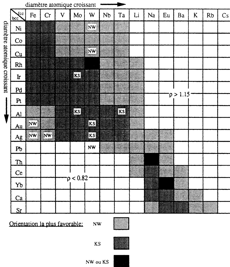
Figure I-4: Prédiction d'orientation pour les épitaxies bcc/fcc (d'après [5])
