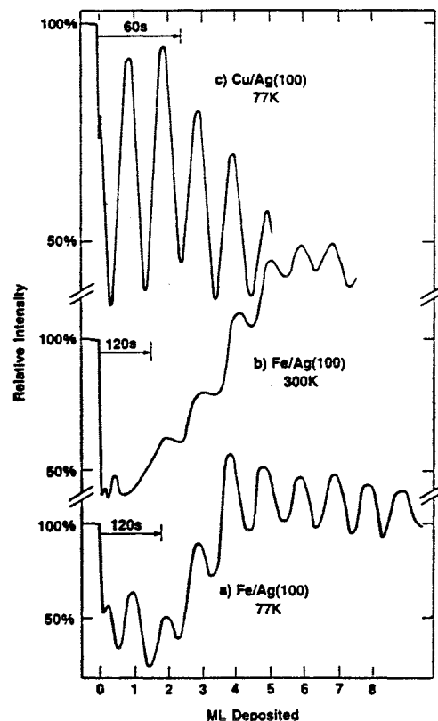
Figure II-20: Oscillations d'intensité RHEED dans le cas de la croissance de fer et de cuivre sur Ag(110) à différentes températures. (d'après [28])
