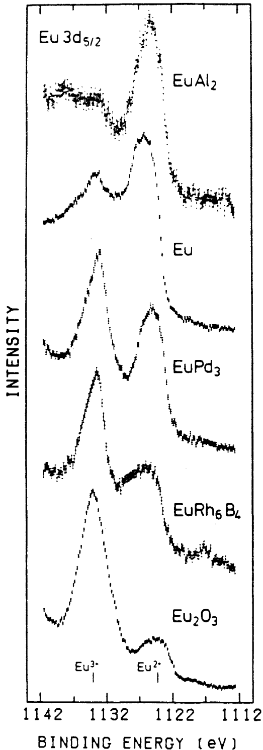
Figure III-3 : Spectres de \text{Eu } 3d_{5/2} dans différents composés. La structure à 1138 eV dans \text{EuAl}_2 est due à une perte par plasmons. (d'après [11])
