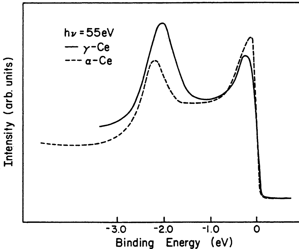
Figure I-23: Spectres de photoémission de Ce- \gamma et Ce- \alpha . Les spectres ont été normalisés à l'intensité de E_B = -1 eV. (d'après [76])
