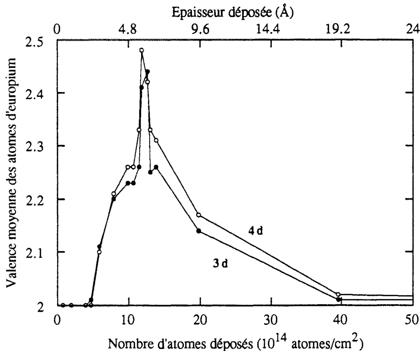
Figure III-27: Evolution de la valence moyenne de l'euporium, déduite des spectres 3d (symboles pleins) et 4d (symboles vides), en fonction de la quantité d'euporium déposé.
