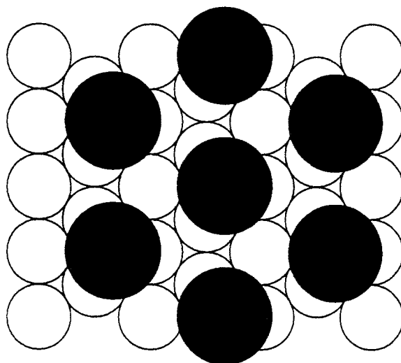
Figure III-26: Structure p(2 \times 2) pour \theta = 1 ; les atomes d'euporium en noir et de palladium en blanc sont représentés à l'échelle.
