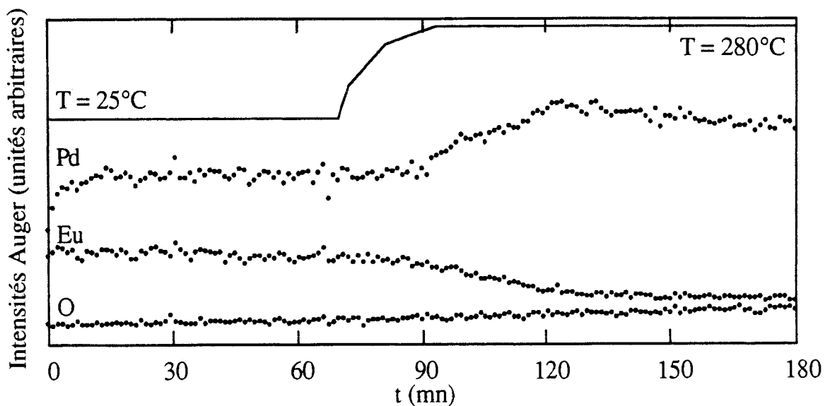
Figure III-7: Evolution des intensités Auger d'euporium et de palladium en fonction du temps et de la température pour un dépôt de 50 Å d'euporium à température ambiante. La contamination progressive en oxygène peut expliquer la diminution du signal de palladium à partir de t \approx 150 mn.
