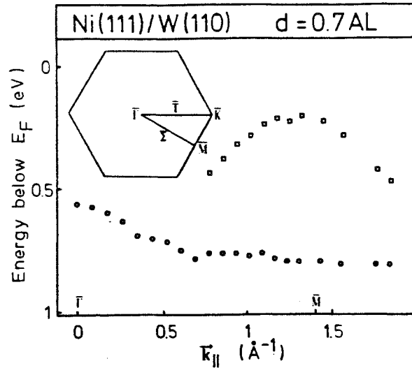
Figure II-17: Courbes de dispersion E(k_{||}) (déduites des spectres de la figure II-16) le long de la direction \bar{\Gamma} - \bar{M} de la zone de Brillouin bidimensionnelle de 0.7 monocouche de Ni(111) sur W(110). (d'après [20])
