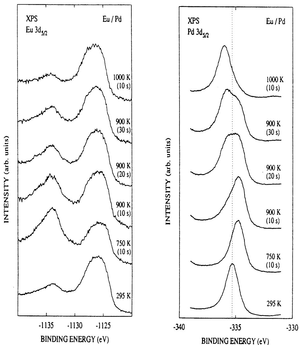
Figure III-6: Spectres de Eu 3d et Pd 3d pour un dépôt de 8.8 Å d'euporium et différents recuits. (d'après [15])
