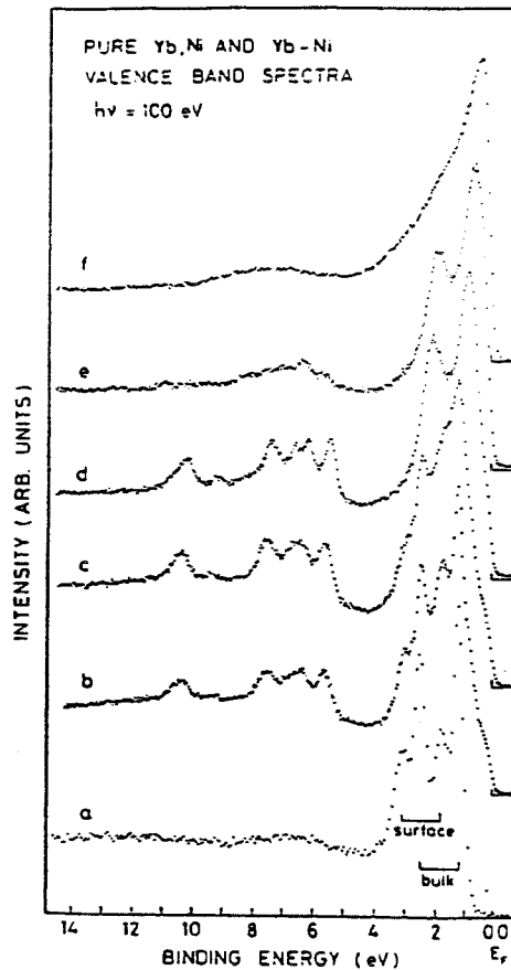
Figure I-14: Evolution des spectres des bandes de valence dans le système Yb-Ni (a: Yb pur - b→e: dilution d'ytterbium croissante - f: Ni pur). Les structures entre 0 et 4 eV sont les états 4f de l'ytterbium 2^+ et les structures 4f des atomes 3^+ sont situées entre 5 et 11 eV. (d'après [50])
