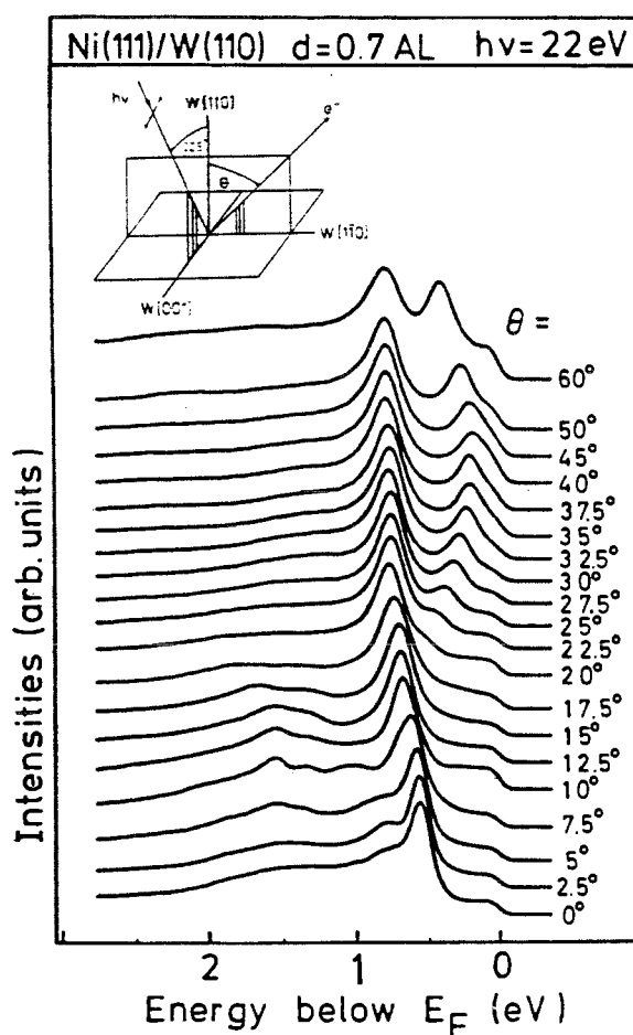
Figure II-16 : Spectres de photoémission de bandes de valence pour 0.7 monocouche de Ni(111) sur W(110) suivant différents angles d'émission et selon la géométrie présentée en insert. (d'après [20])
