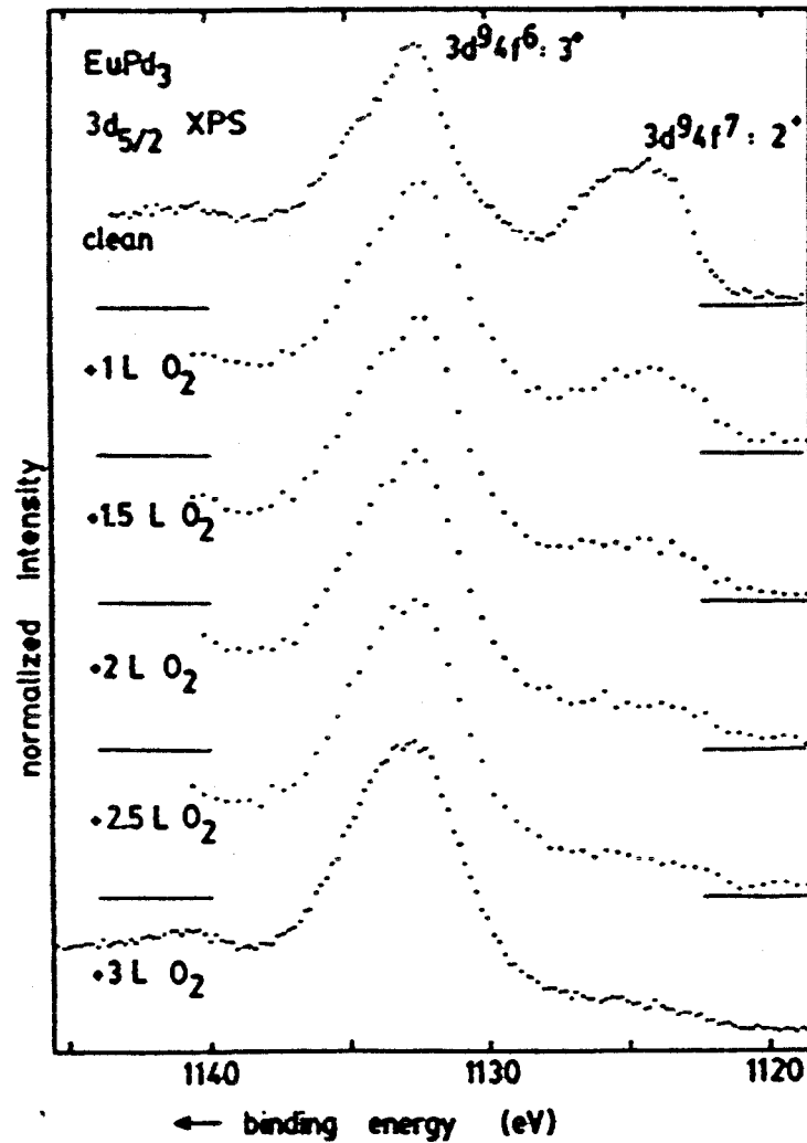
Figure III-4: Spectres de photoémission Eu 3d_{5/2} dans \text{EuPd}_3 en fonction de l'oxydation. (d'après [13])
