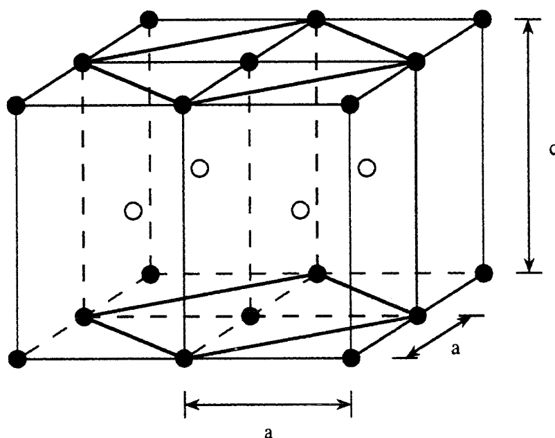
Figure I-11: Relation entre les cellules tétragonales centrées et à faces centrées (bct et fct). Les atomes aux centres des cellules bct sont représentés en blanc pour plus de clarté (d'après [29])
