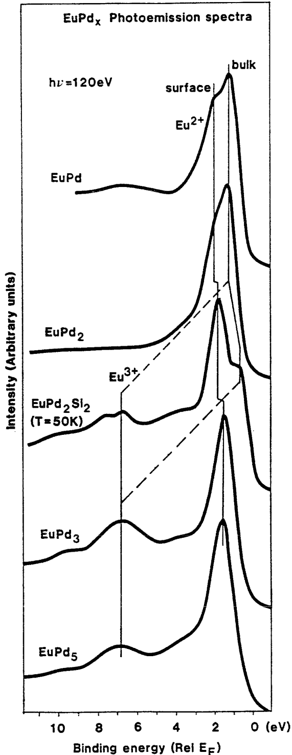
Figure III-2: Spectres de photoémission 4f dans les composés \text{EuPd}_x . Les spectres sont dominés par les états 4f de l'euprimum car, à cette énergie de photons, la bande 4d du palladium présente un minimum de section efficace. (d'après [10])
