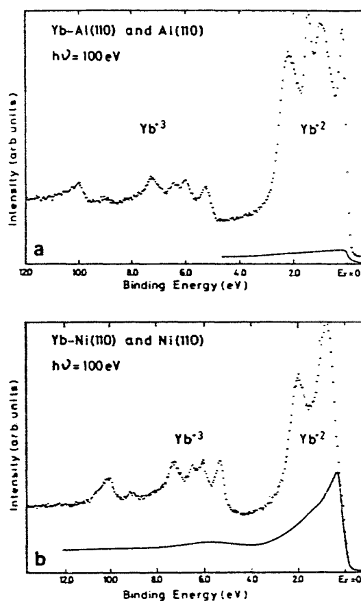
Figure I-13: Spectres des bandes de valence des systèmes Yb/Al(110) et Yb/Ni(110). Les spectres des substrats seuls sont représentés en trait plein. (d'après [49])
