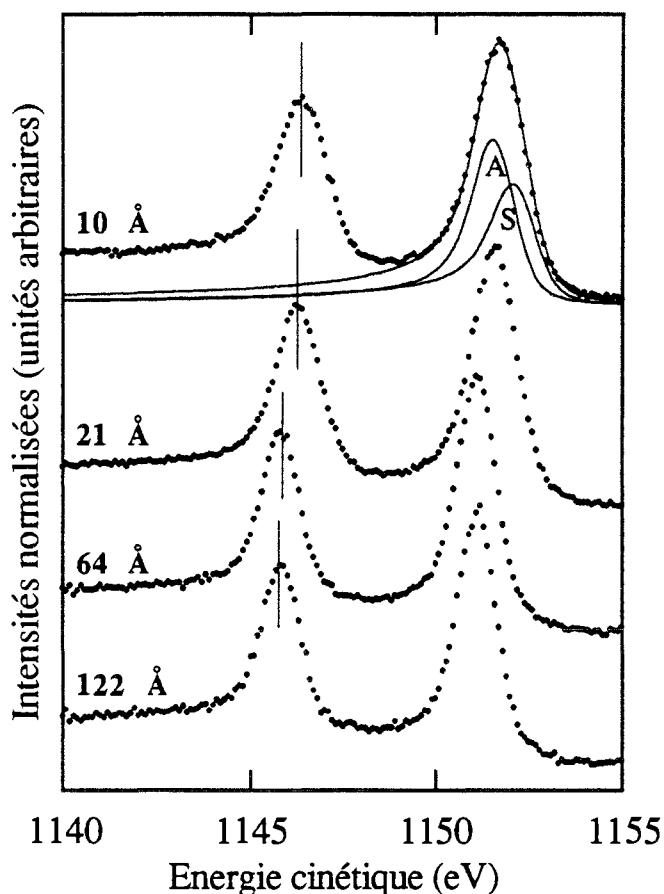
Figure III-28: Spectres de photoémission de palladium 3d pour 10, 21, 64 et 122 Å d'euporium déposés. Pour le spectre à 10 Å, un ajustement de la composante 3d_{5/2} avec une contribution due au substrat (S) et une contribution d'alliage (A) est présenté en traits pleins.
