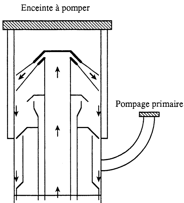
Figure II-2: Schéma de principe d'une pompe à diffusion d'huile
