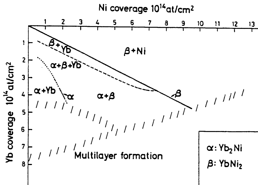
Figure I-17: Diagramme de phase du système Yb-Ni sur Mo(110). Phase \alpha : \text{Yb}_2\text{Ni} de structure (7x2) et phase \beta : \text{YbNi}_2 de structure (3x2). (d'après [54])
