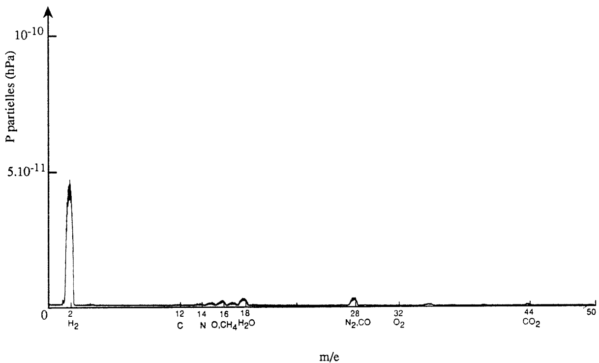
Figure II-3: Spectre de gaz résiduel ( P_{\text{totale}} = 6 \cdot 10^{-11} hPa)
