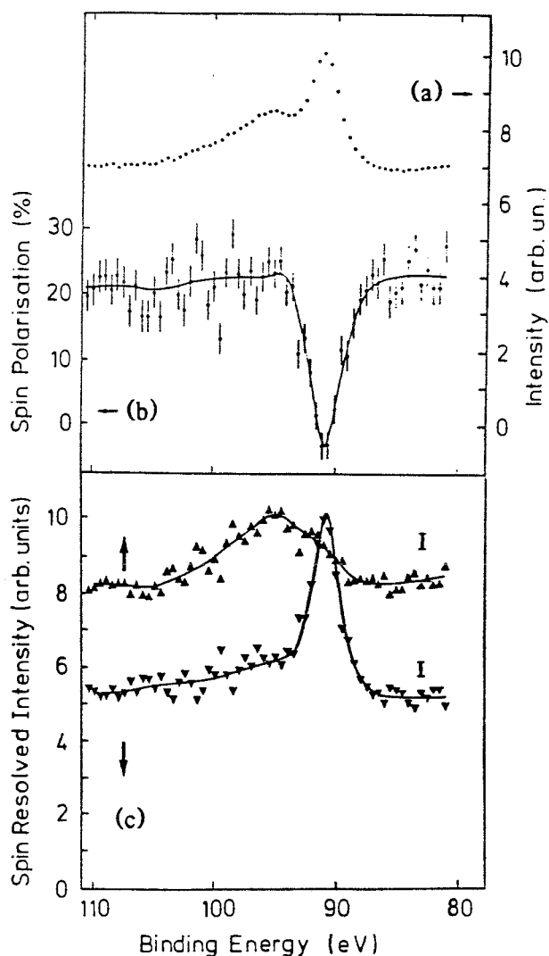
Figure II-13 : (a) spectre de photoémission de Fe 3s non résolu en spin, (b) polarisation en spin du spectre, (c) spectres résolus en spin (spins majoritaires \uparrow ). (d'après [15])
