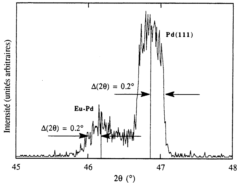
Figure III-34 : Diagramme de diffraction obtenu pour R = -30^\circ en fixant l'angle d'incidence \omega à la valeur du maximum de la rocking curve et en variant l'angle de détection.
