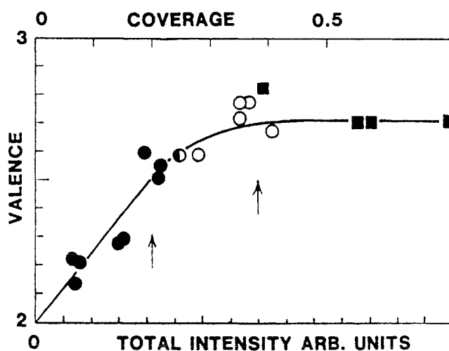
Figure I-18 : Evolution de la valence moyenne du samarium sur Cu(001). (d'après [55])
