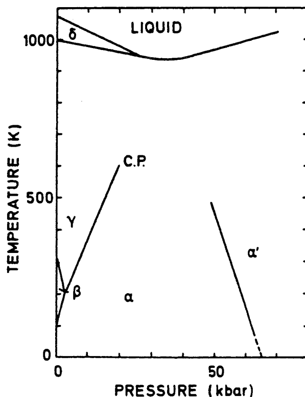
Figure I-22: Diagramme de phase du cérium. (d'après [74])
