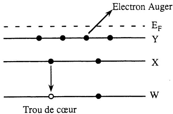
Figure II-8: Représentation d'un processus Auger WXY
