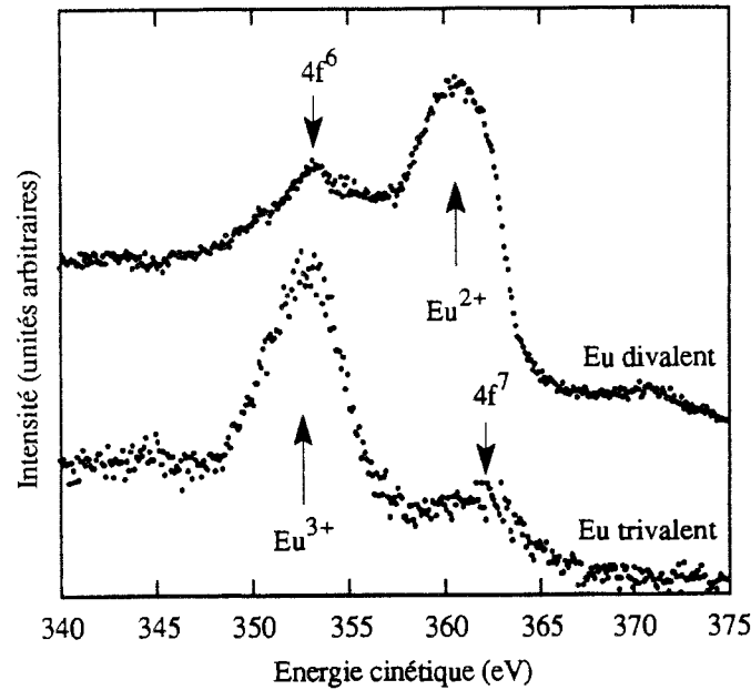
Figure II-15: Spectres de photoémission 3d_{5/2} d'euporium divalent et d'euporium trivalent. Les structures 4f^6 dans Eu divalent et 4f^7 dans Eu trivalent correspondent à des effets d'états finaux.
