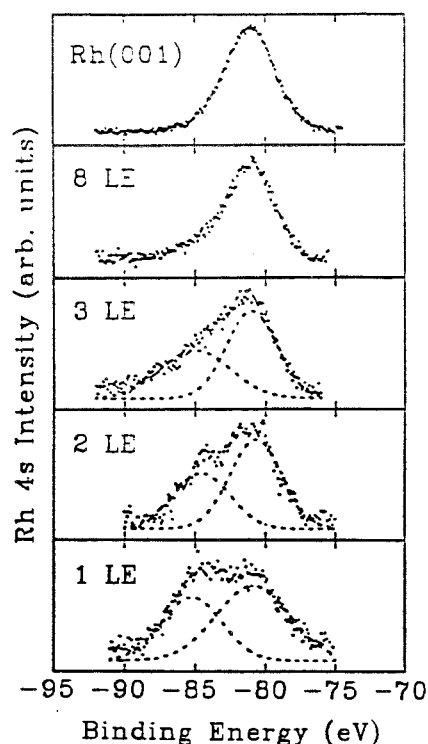
Figure I-8: Spectres de photoémission 4s de films ultra-minces de rhodium sur Ag(001) et comparaison avec Rh(001) (d'après [20])
