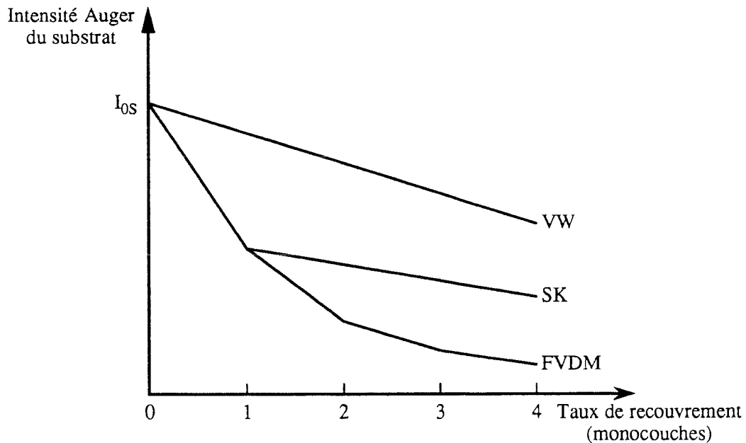
Figure II-10: Variation de l'intensité Auger du substrat en fonction du recouvrement et du mode de croissance. (VW: Volmer-Weber, SK: Stranski-Krastanov, FVDM: Frank van der Merwe)
