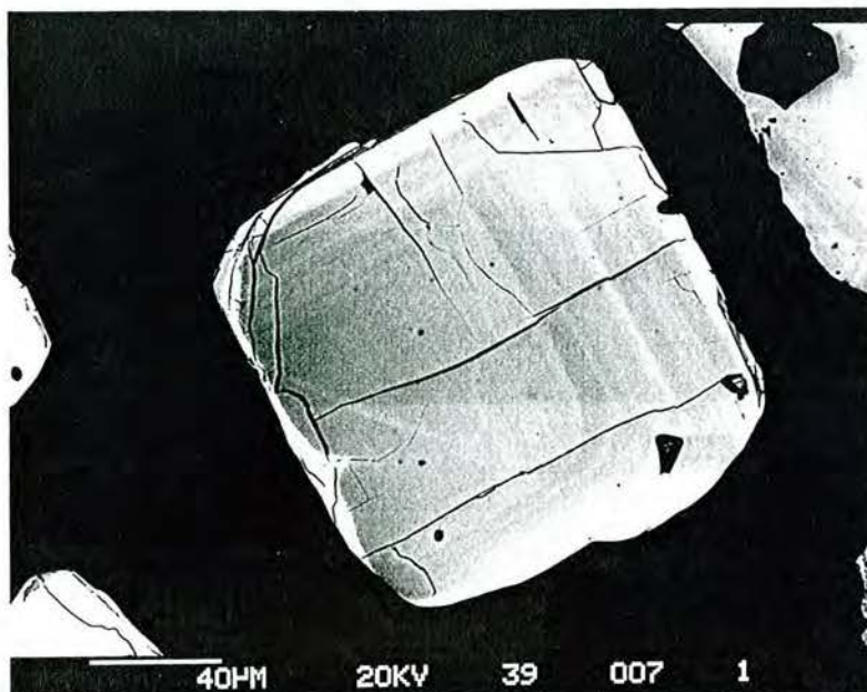
Photo V.3 - Section basale d'un zircon du gneiss oillé montrant de fines zonations de croissance. Il ressort que le contour interne de la couche externe est irrégulier (partie gauche de la photo) indiquant une corrosion du cristal avant cette surcroissance, ou un remplacement progressif à partir de la bordure. Fraction 200-150 \mu , magnétique à 3,6 Amp., 2°.
