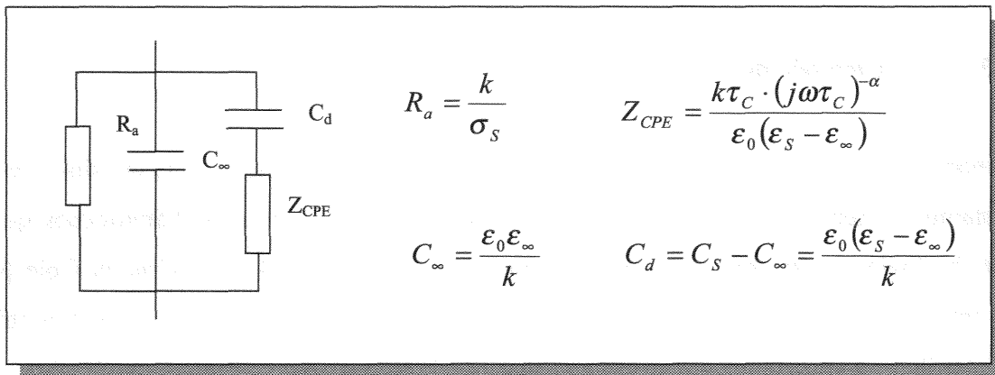
Figure I.15 : Réseau équivalent à l'équation de Cole-Cole Le paramètre k est un facteur géométrique ( cm^{-1} ) (d'après [RIG 96])
