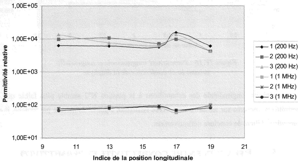
Figure IV.15 : Variation de la permittivité longitudinale le long et autour de la diaphyse. Permittenités à 200 Hz et 1 MHz.
