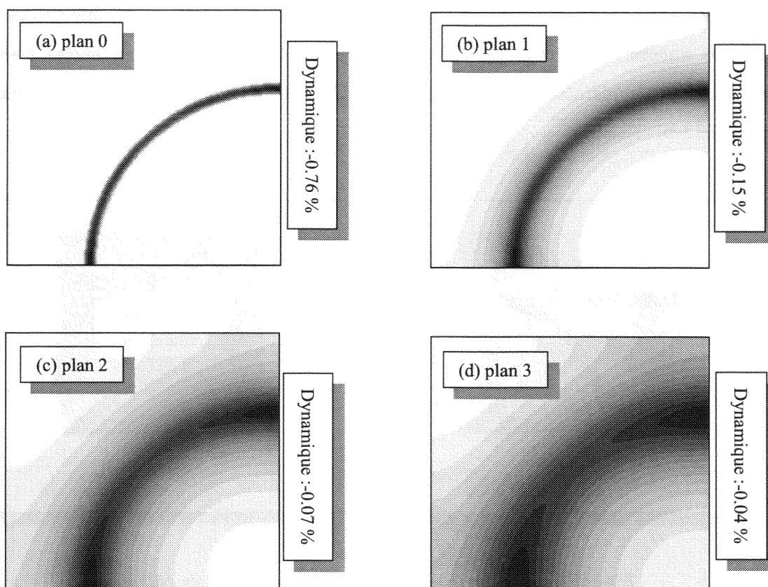
Figure II.34 (a), (b), (c), (d) : Champ de potentiel dans les 4 premières tranches du volume 3D
