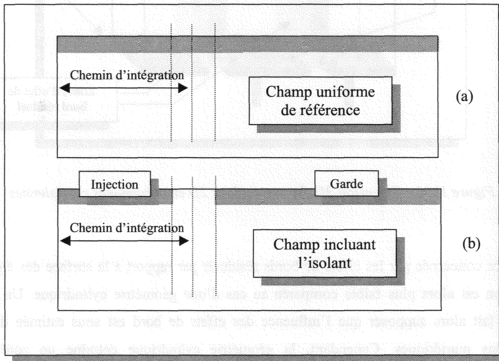
Figure II.31 (a) et (b) : Chemin d'intégration de la densité de courant
