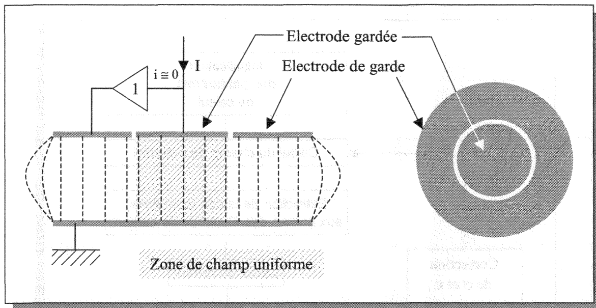
Figure II.5 : Principe de l'électrode de garde
