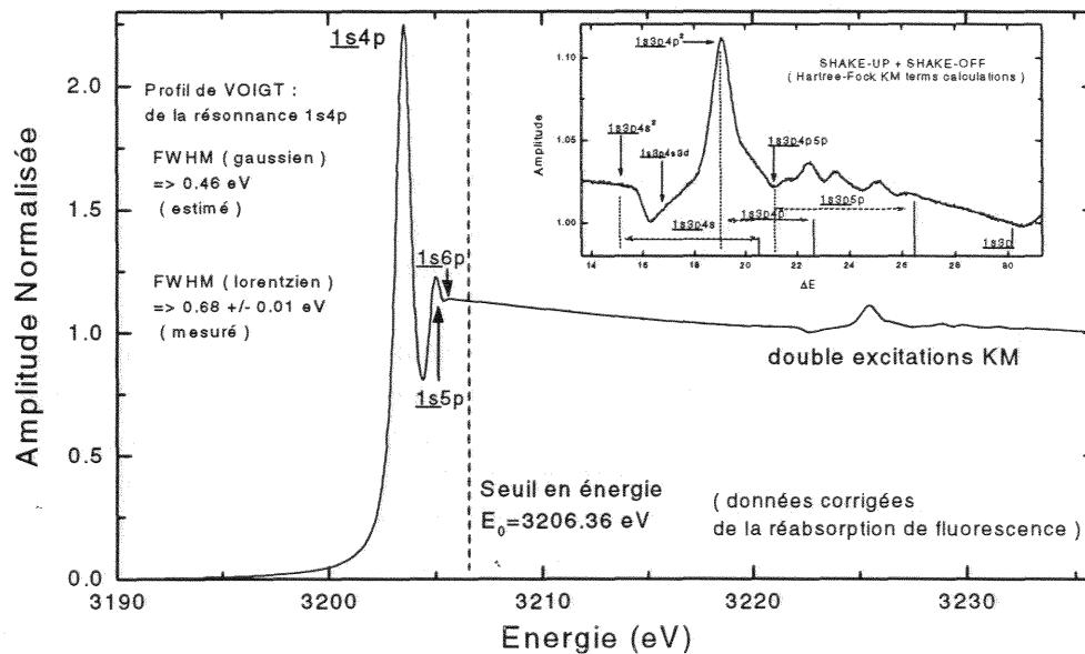
Fig 1 : Spectre XANES de l'argon gaz au seuil K, avec les excitations multiélectroniques KM .
