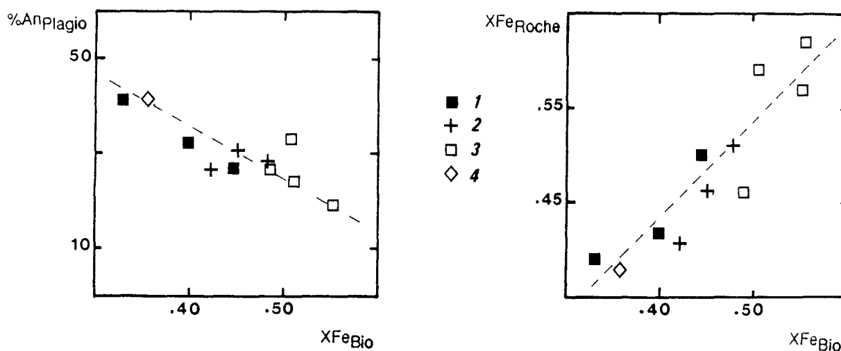
Figure II.32 - Variations du XFe (moyennes) des biotites en fonction du % d'An des plagioclases et du XFe des diorites. 1 : méladiorite ; 2 : diorite commune; 3 : diorite hétérogène ; 4 : diorite microgrenue TAG 130.
