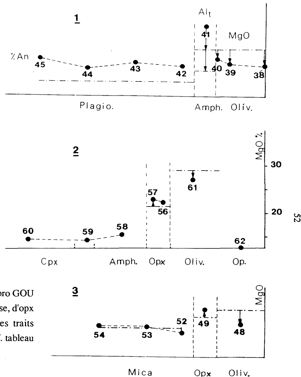
Figure II.9 - Variations de quelques éléments le long des profils étudiés à la microsonde dans les couronnes des olivines du gabbro GOU 43. --- moyenne de l'élément dans les mêmes minéraux hors couronnes
