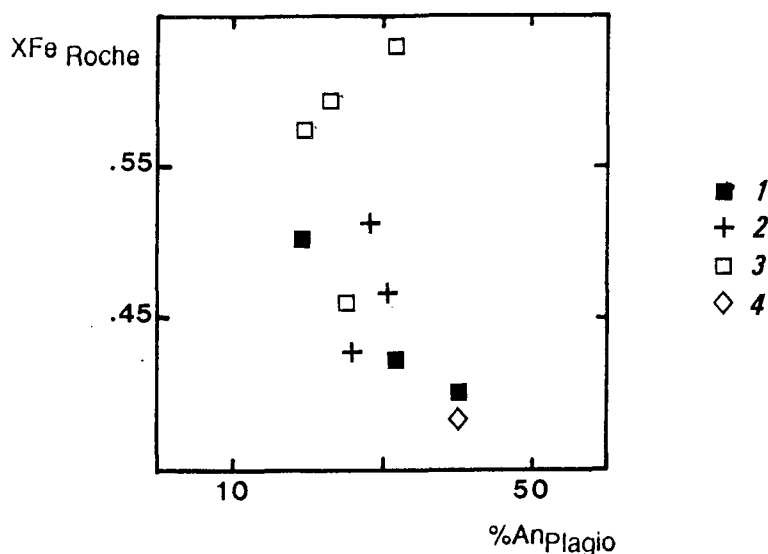
Figure II.34 - Variations du pourcentage en anorthite du plagioclase (moyennes) en fonction du XFe de la roche hôte. 1 : méladiorite ; 2 : diorite commune ; 3 : diorite hétérogène ; 4 : diorite microgrenue.
