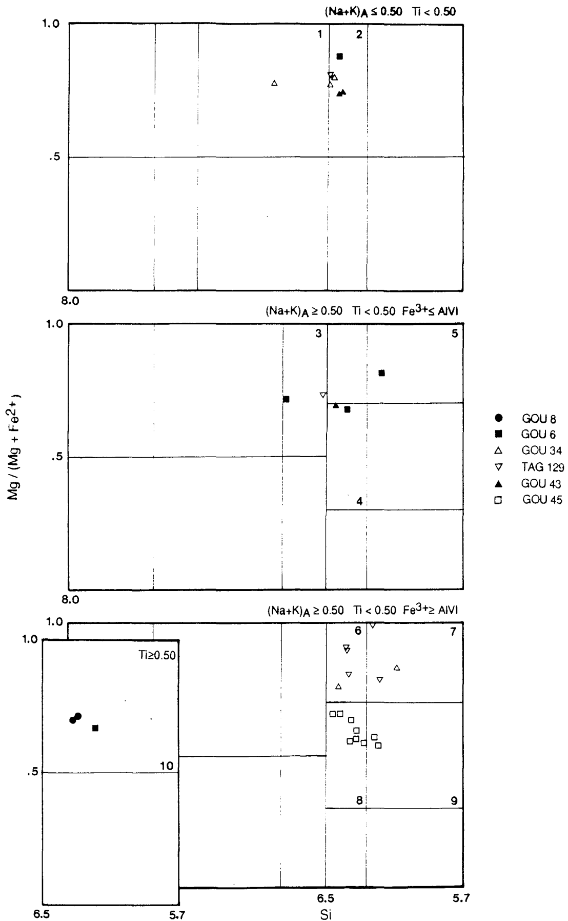
Figure II.19 - Position des amphiboles des gabbros dans la classification de Leake (1978). 1: magnésio - hornblende. 2 : tschermakitic hornblende; 3 : edenitic hornblende; 4 : ferroan pargasitic hornblende; 5 : pargasite; 6 : magnésio - hastingsitic hornblende; 7 : magnésio - hastingsite; 8 : magnésian hastingsitic hornblende; 9 : magnésian hastingsite; 10 : kaersutite.
