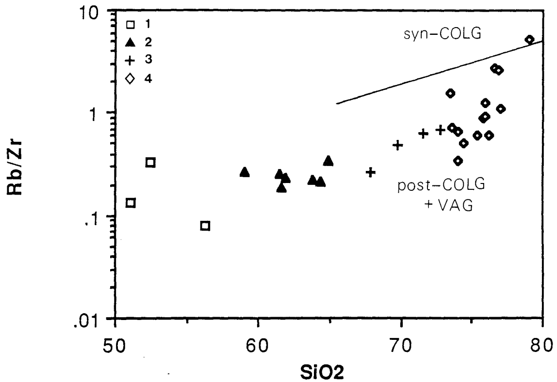
Figure IV.13 - Diagramme Rb / Zr = f(SiO_2) de Harris et al. (1986). 1 : diorites ; 2 : granodiorites-tonalites ; 3 : monzogranites ; 4 : leucogranites. Syn-COLG : granites syn-collision, post-COLG : granites post-collision, VAG : granites des arcs volcaniques.
