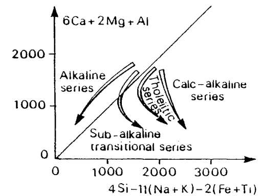
Figure IV.9 - Diagramme R1/R2 (De La Roche et Leterrier, 1973, 1980). Les analyses sont regroupées par unité géographique définie dans le chapitre II . 1 : SW du massif, 2 : centre du massif, 3 : N du massif. (Mêmes figurés que IV.7).
