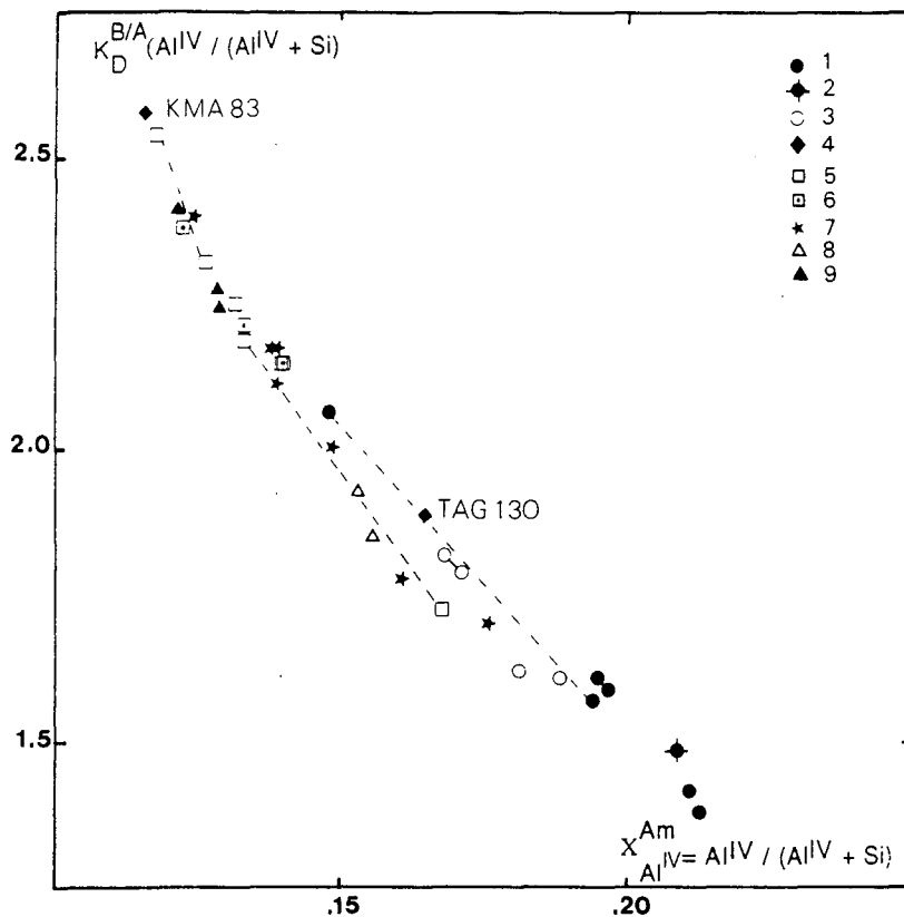
Figure II.53 - Diagramme K_D^{Bio/Amph} (Al^{IV}/(Al^{IV}+Si)) = f (X_{Al^{IV}}^{Am}) . 1 : gabbros ; 2 : leucogabbro GOU 45 ; 3 : méladiorites ; 4 : filon doléritique KMA 83 et "lamprophyrique" NFI 51 ; 5 : diorites hétérogènes ; 6 : diorites communes ; 7 : granodiorites-tonalites ; 8 : granites leucocrates ; 9 : monzogranites.
