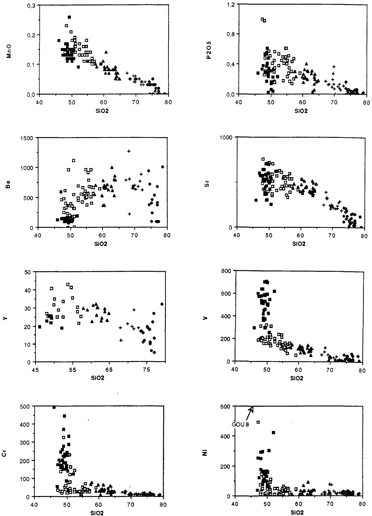
Figure IV.3 - Diagrammes oxydes - silice (suite) et éléments traces (ppm) - silice (%) des cinq groupes de roches composant le Massif du Tichka. Mêmes figurés que précédemment.
