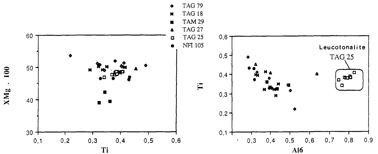
Figure II.39 - Diagrammes XMg / Ti et Ti / AlVI des biotites des GDT.
