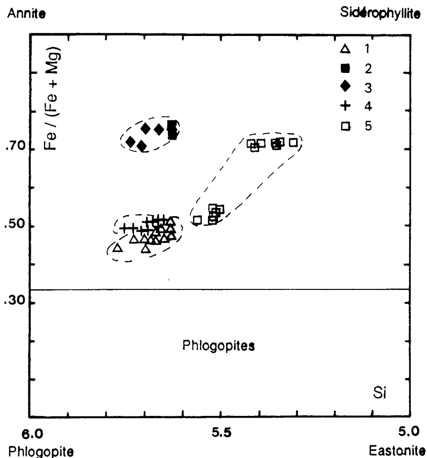
Figure II.45 - Position des biotites des granites dans le diagramme Fe / Fe+Mg -- Si. 1 : monzogranites (TAG 126 + TAG 135 + GOU 69) ; 2 et 3 : leucogranites à biotite et amphibole (2 : TAM 27 ; 3: MED 38) ; 4 : leucogranites à biotite (NFI 72 et NFI 83) ; 5 : leucogranite à deux micas (ASF 39).
