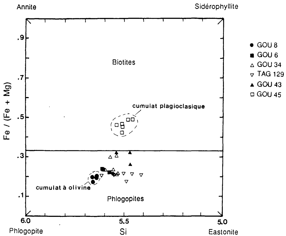
Figure II.22 - Diagramme Si - XFe de classification des micas des gabbros
