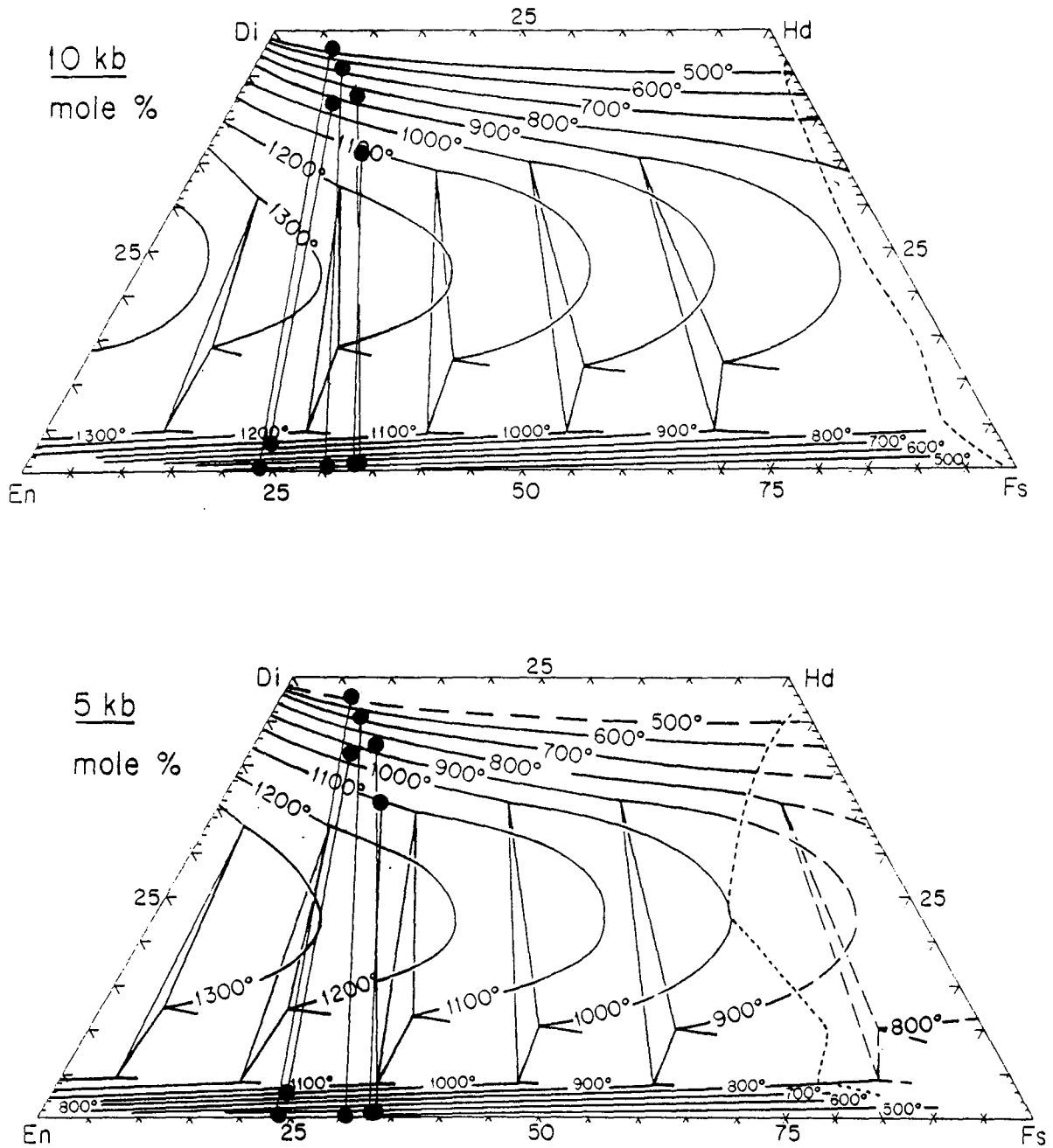
Figure III.1 - Diagramme Wo-En-Fs des couples cpx - opx des gabbros. Les isothermes sont extraits de Lindsley (1983). A droite de la courbe en pointillés, les relations des pyroxènes sont métastables.
