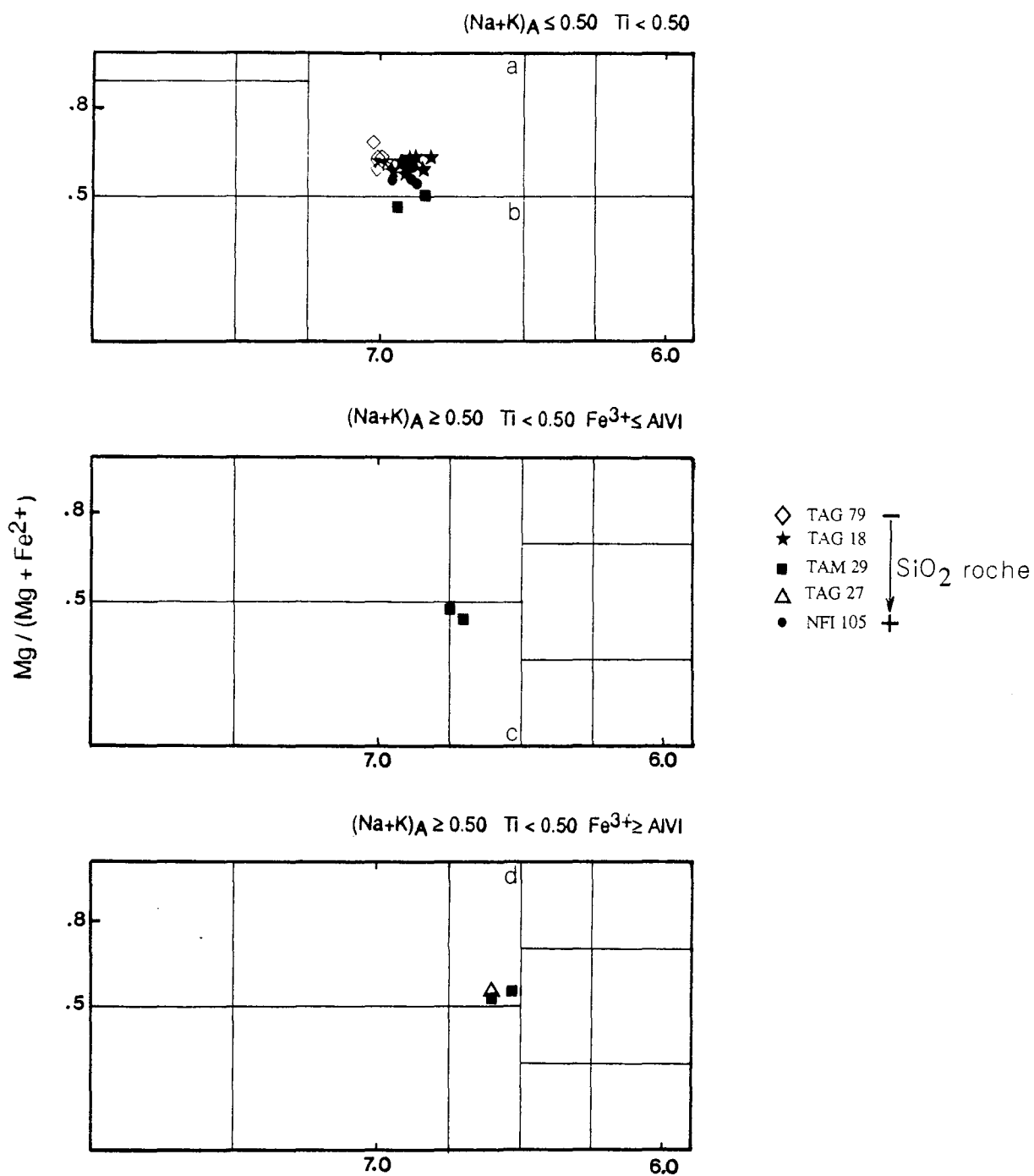
Figure II.36 - Position des amphiboles des granodiorites-tonalites dans la classification de Leake (1978).
