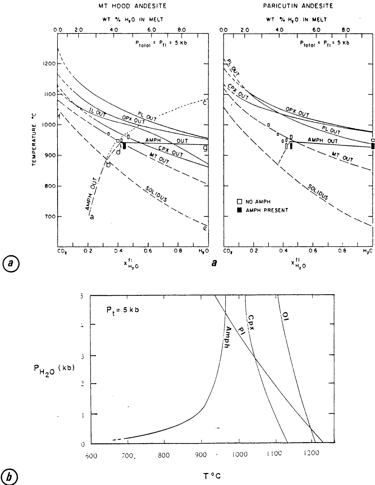
Figure III.11 - a. Sections T - X pour l'andésite de Mount Hood et l'andésite de Paracutin (Eggler, 1972). b. Courbes schématiques de fusion des silicates dans un liquide basaltique d'après Yoder et Tilley (1962) et Eggler (1972).
