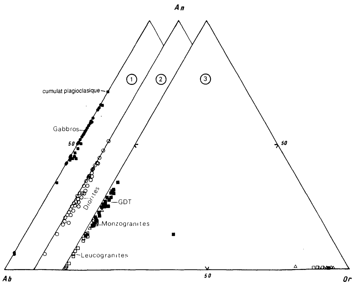
Figure II.56- Position des feldspaths dans le diagramme An / Ab / Or.
