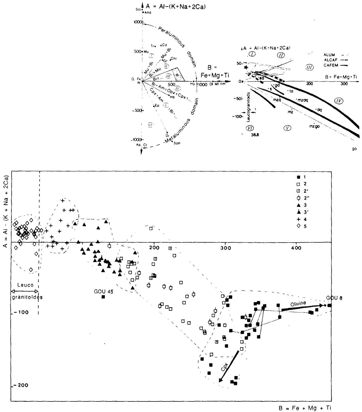
Figure IV.8 - Diagramme A / B de Debon et Lefort (1983, 1988). 1 : gabbro ; 2 : diorite 2' : diorite en enclave ; 2'' diorite proche d'une interface diorite / GDT; 3 : GDT ; 3' : GDT proche d'une interface ou en enclave dans monzogranite ; 4 : monzogranite ; 5 : leucogranite.
