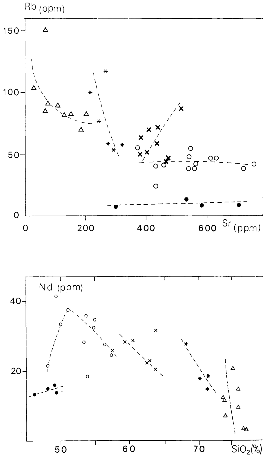
Figure IV.5 - Diagrammes Rb / Sr et Nd / SiO 2 de l'ensemble des roches du Massif du Tichka. 1 : gabbros ; 2 : diorites ; 3 : granodiorites-tonalites ; 4 : monzogranites ; 5 : leucogranites. Seules les analyses de Sr et de Nd faites pour l'étude isotopique, ont été retenues dans ces diagrammes.
