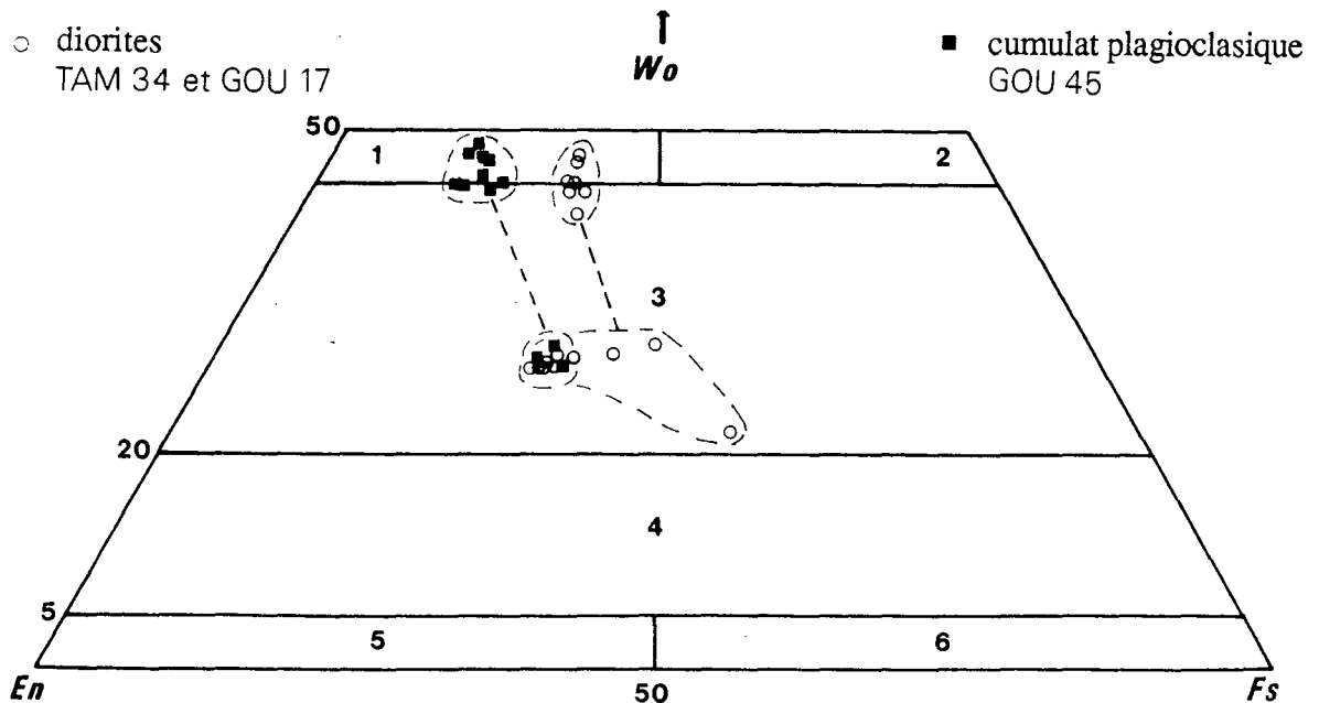
Figure II.13 - Diagramme de classification des pyroxènes des diorites et du leucogabbro en enclave GOU 45, d'après Morimoto (1988). Wo : wollastonite, En : enstatite, Fs : ferrosilite, 1 : diopside, 2 : hédenbergite, 3 : augite, 4 : pigeonite, 5 : clinoenstatite, 6 : clinoferrosilite.
