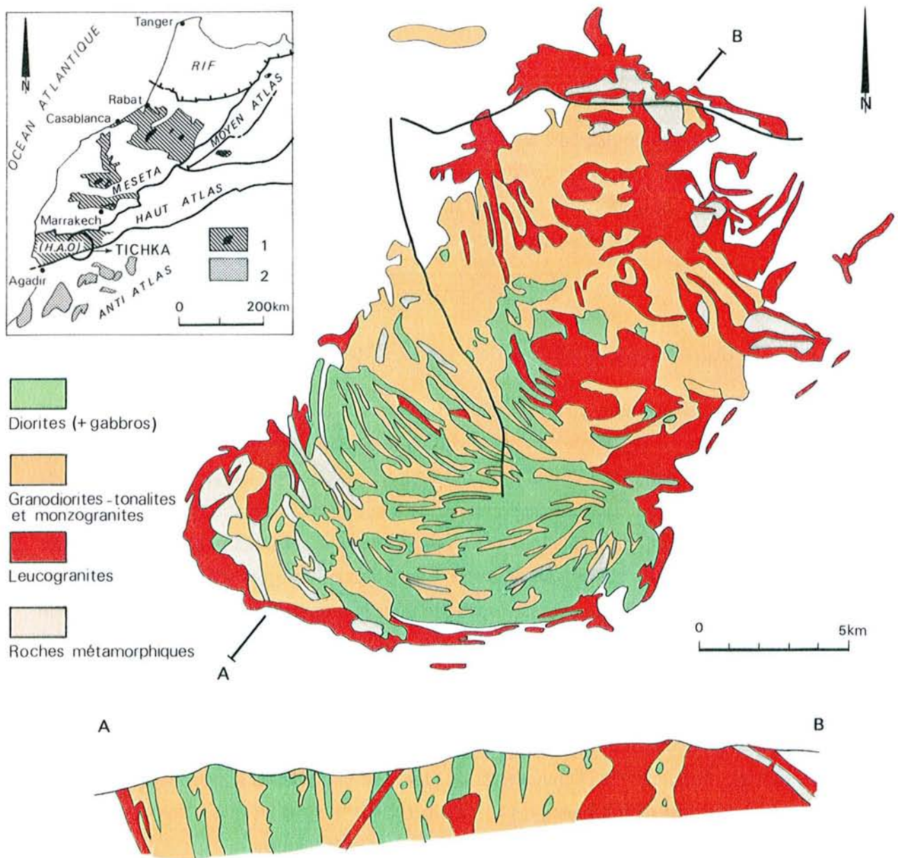
Figure II.1 - Carte géologique schématique du Massif du Tichka et coupe synthétique montrant les relations entre les différents faciès. (cf. carte 1/50 000° en annexe pour une plus grande précision)
