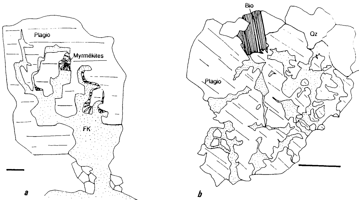
Figure II.41 - Association plagioclase - FK dans les granodiorites-tonalites. La barre d'échelle équivaut à 0.5 mm. Pointillés : FK, traits fins : plagioclase. a : TAG 105 - microcline envahissant un plagioclase à partir de la mésostase. b : NFI 105-remplacement du plagioclase par le FK avec développement de myrmékites entre les 2 types de minéraux.
