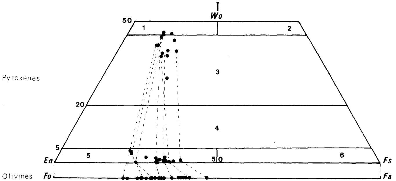
Figure II.12 - Diagramme de classification des pyroxènes des gabbros, d'après Morimoto et al. (1988). Wo : wollastonite, En : enstatite, Fs : ferrosilite, 1 : diopside, 2 : hédenbergite, 3 : augite, 4 : pigeonite, 5 : clinoenstatite, 6 : clinoferrosilite.
