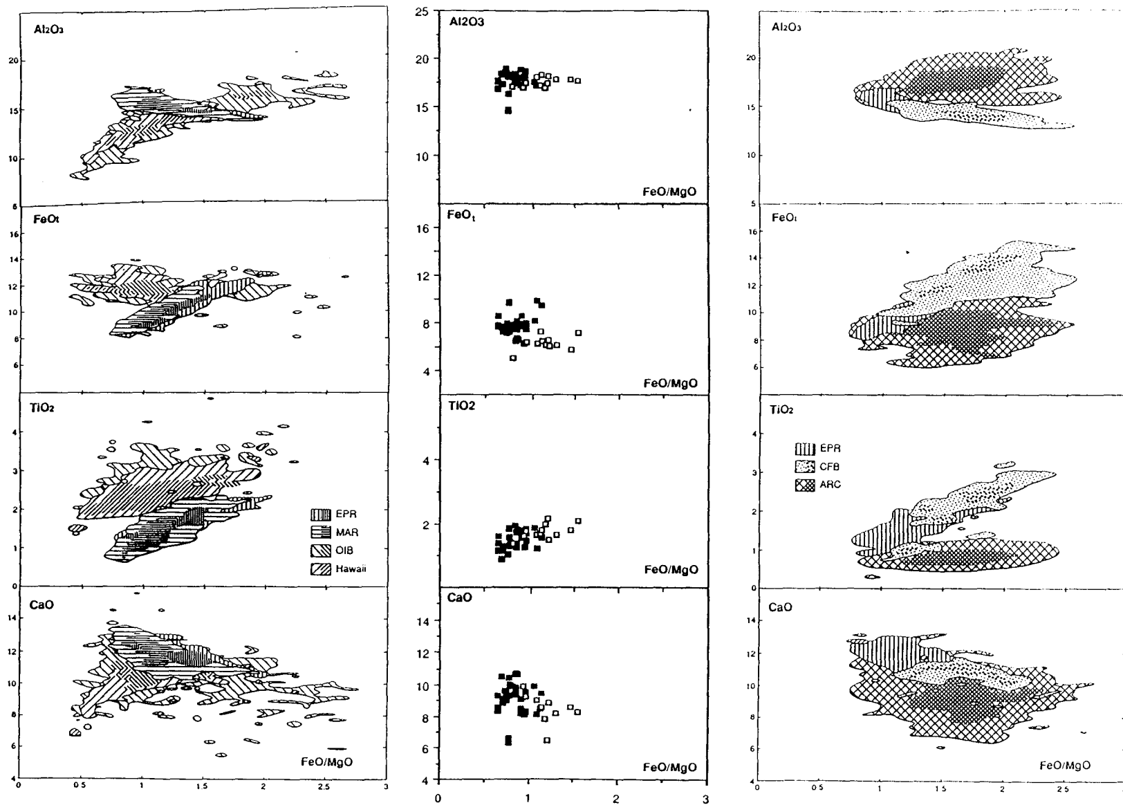
Figure IV. 11 - Diagrammes de variations des éléments majeurs ( \text{Al}_2\text{O}_3 , \text{FeO}_t , \text{TiO}_2 , \text{CaO} ) en fonction de \text{FeO} / \text{MgO} . Mêmes figurés que précédemment. Les diagrammes de référence sont issus de Albarède (1991) : ARC = Orogenic Basalts, CFB = Continental Flood Basalts, EPR = East Pacific Rise, MAR = Mid - Atlantic Ridge, OIB = Ocean Island Basalt.
