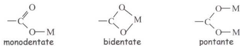
Figure V-J : Représentation schématique des différents types de coordination entre une fonction carboxylate et un cation métallique M (dans le cas présent M = Al).
