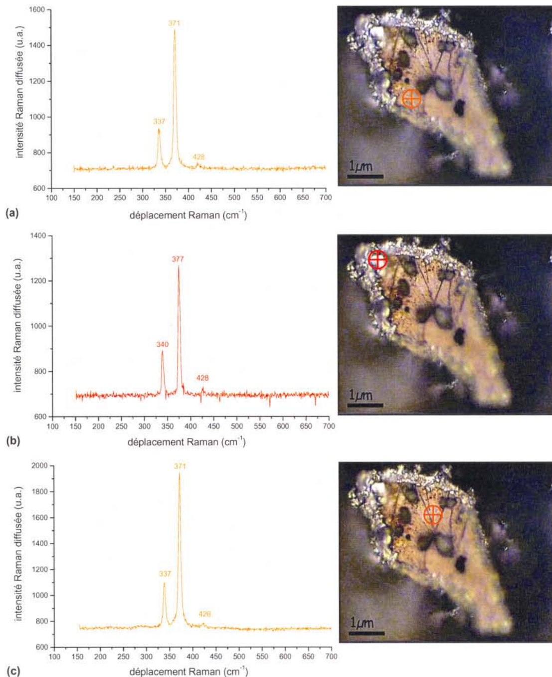
Figure IV-T : Spectres Raman collectés sur une particule de pyrite après 20 heures d'oxydation par du chrome (VI) à pH = 5,0 (Figure IV-N) ; expérience menée sous barbotage d'argon ( [Cr(VI)]_0 = 1,97 \times 10^{-4} M, [Cr(tot)]_{20h} = 1,48 \times 10^{-4} M) : zones (a) et (c) « orangées », (b) « argentée ».
