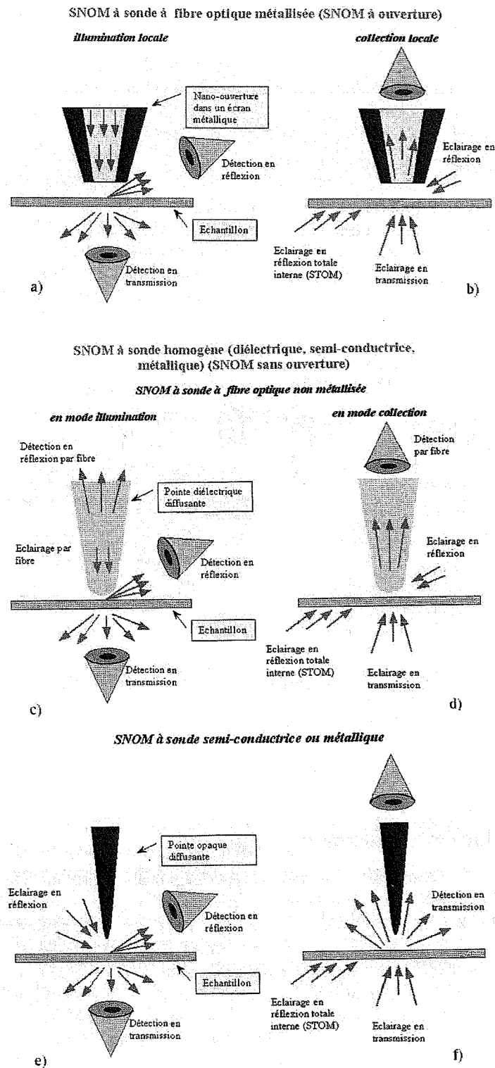
Figure III-U : Principales configurations de microscopes optiques en champ proche (Courjon et Bainier, 2001) (SNOM : Scanning Near Field Optical Microscopy) :
