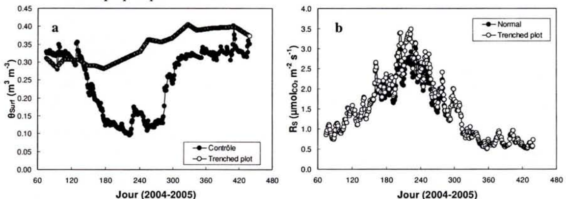
Figure 9. (a) Evolution saisonnière du contenu volumique en eau du sol ( \theta_{\text{Surf}} ) dans une parcelle contrôle et dans un trenched plot et (b) évolution de la respiration du sol (R S ) simulée avec l'équation (5) avec les contenus en eau de sol contrôles (Normal) ou des trenched plots. Données de la placette H1A (CPH1).
