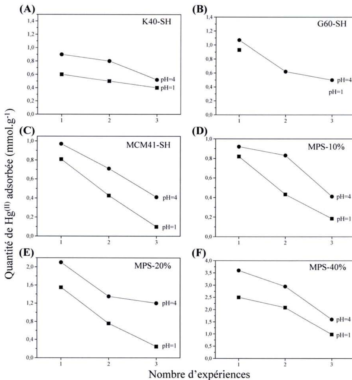
Figure 36 : Evolution de la capacité de fixation de Hg^{(II)} au cours de trois cycles accumulation - désorption successifs pour les matériaux : (A) K40-SH, (B) G60-SH, (C) MCM41-SH, (D) MPS-10%, (E) MPS-20%, (F) MPS-40%. Les accumulations sont réalisées en large excès de Hg^{(II)} ( 2 à 4 \cdot 10^{-3} M ) pour des suspensions d'adsorbant de 1g.L^{-1} à pH=1 (■) ou à pH=4 (●). La désorption a lieu en milieu [HCl]=12M avec toujours des suspensions de 1g.L^{-1} .
