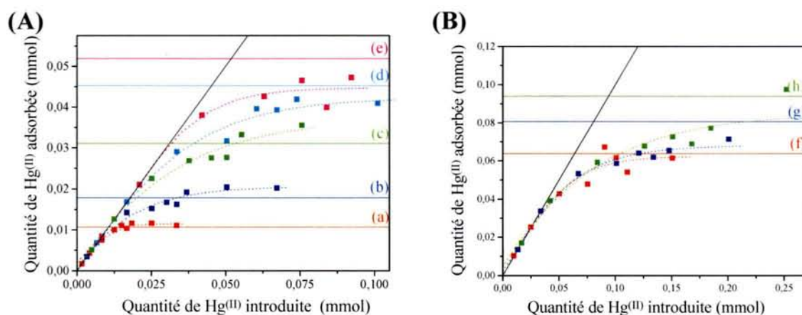
Figures 33 : Suivi de l'adsorption de Hg^{(II)} sur différents matériaux type MPS pour différentes quantités initiales de Hg^{(II)} . Expériences réalisées à pH=1 ( [HNO_3]=0,1M ), avec des suspensions à 1g.L^{-1} (20 mL). — capacité maximale théorique ■ quantité de Hg^{II} fixée ... interpolation des valeurs expérimentales
