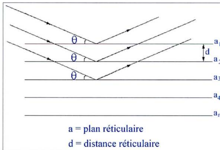
Figure 15 : Illustration de la diffraction des rayons X selon la loi de Wulff-Bragg.
