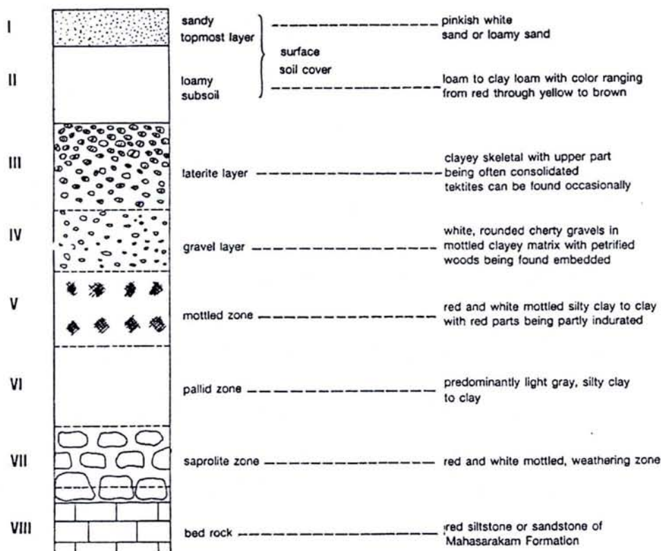
Figure 4 : Stratigraphie Tertiaire et Quaternaire du Nord-Est Thaïlandais
