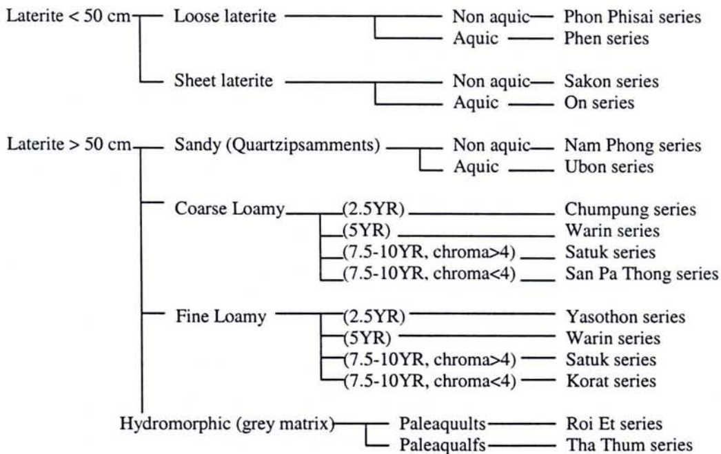
Figure 5 : Organisation et classification des sols dans le Nord-Est Thaïlandais
