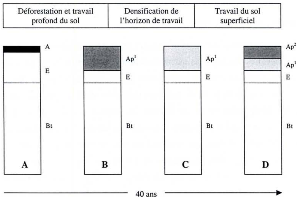
Figure 7 : Evolution du profil de sol aux cours des travaux agricoles avec (a) profil sous forêt ; (b) travail profond ; (c) effondrement de la structure de l'horizon travaillé ; et (c) travail superficiel.
