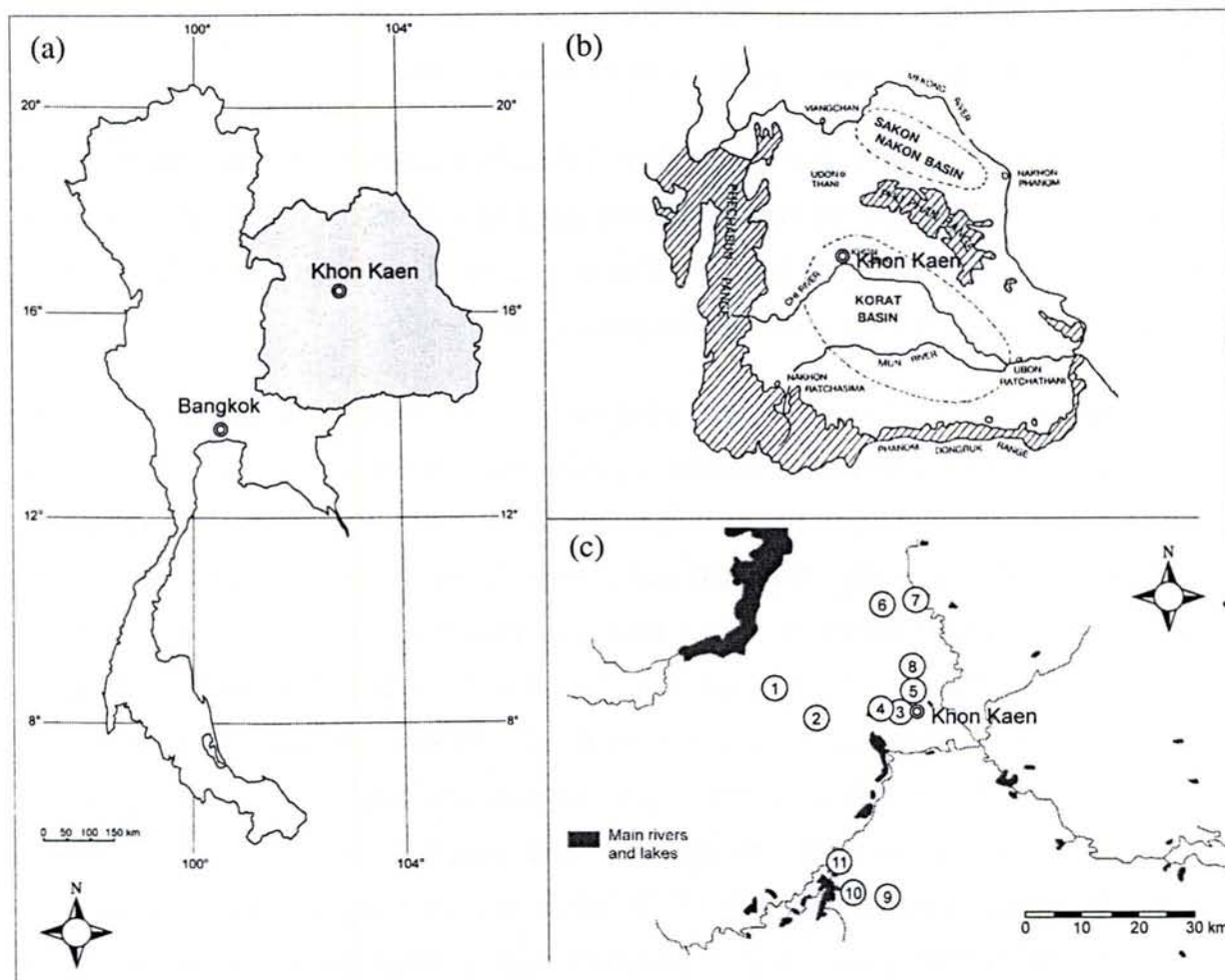
Figure 2 : Situation géographique (a) et physiographique (b) du Nord-Est Thaïlandais et position des sites d'étude (c)
