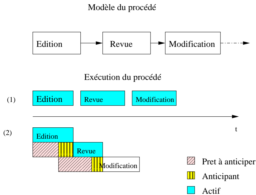
FIG. 4.8 – Les états des activités dans l'exécution d'un procédé sans (1) et avec (2) anticipation
