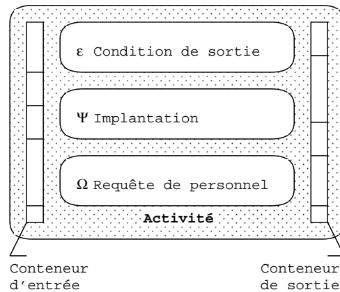
FIG. 4.1 – Structure d'une activité
