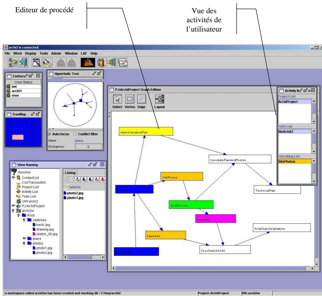
FIG. 5.2 – Interface incluant les outils de workflow
