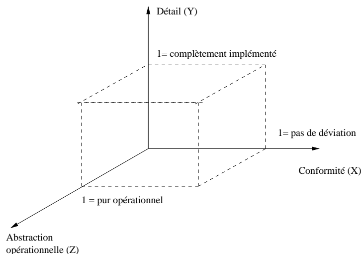
FIG. 3.4 – L'espace domaine du modèle
