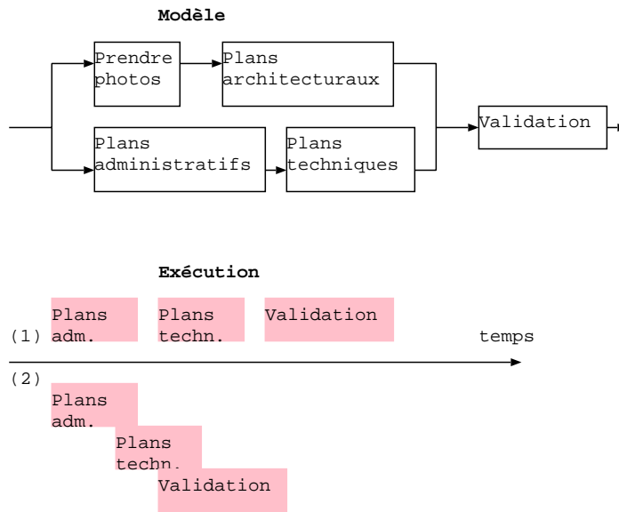
FIG. 2.1 – Exécution rigide (1) ou flexible (2)
