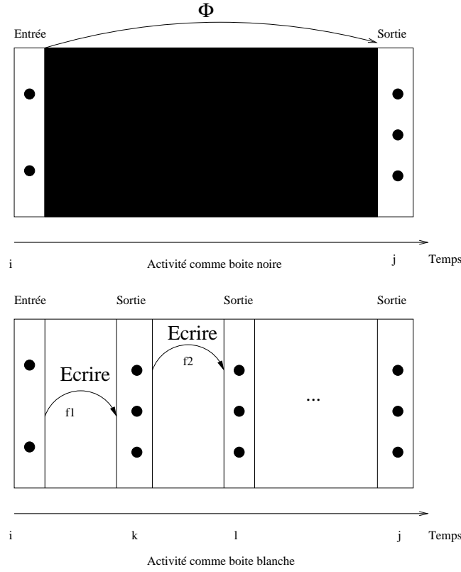
FIG. 4.6 – Activité boîte noire et boîte blanche
