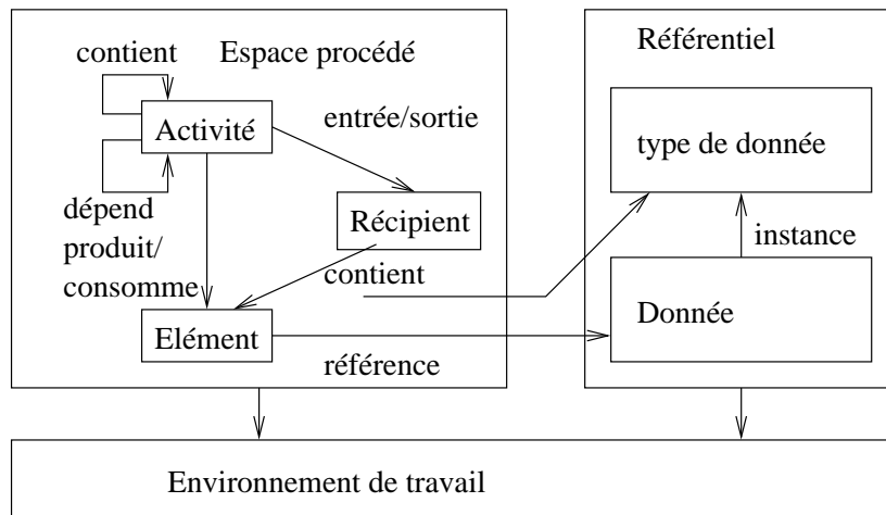
FIG. 3.2 – Approches orientées flot de données
