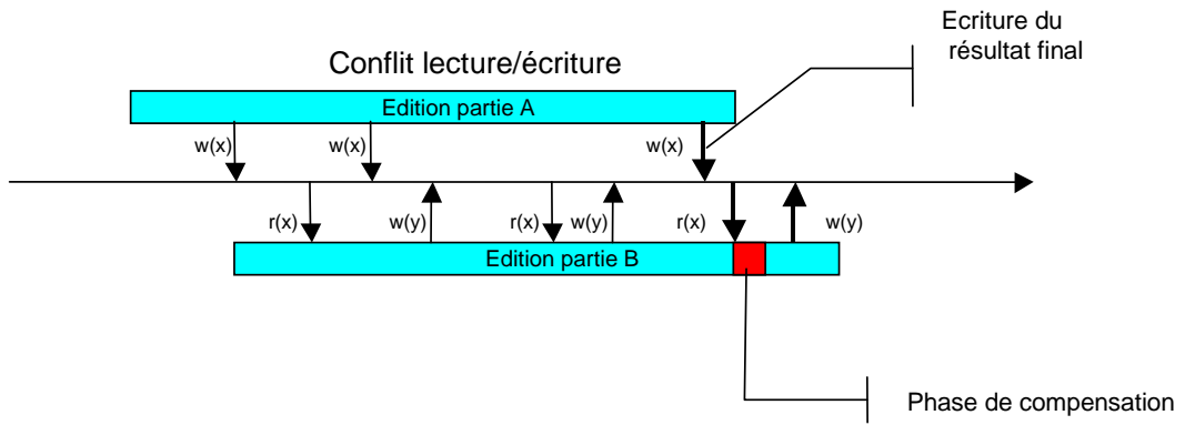
FIG. 4.10 – Échanges de résultats intermédiaires
