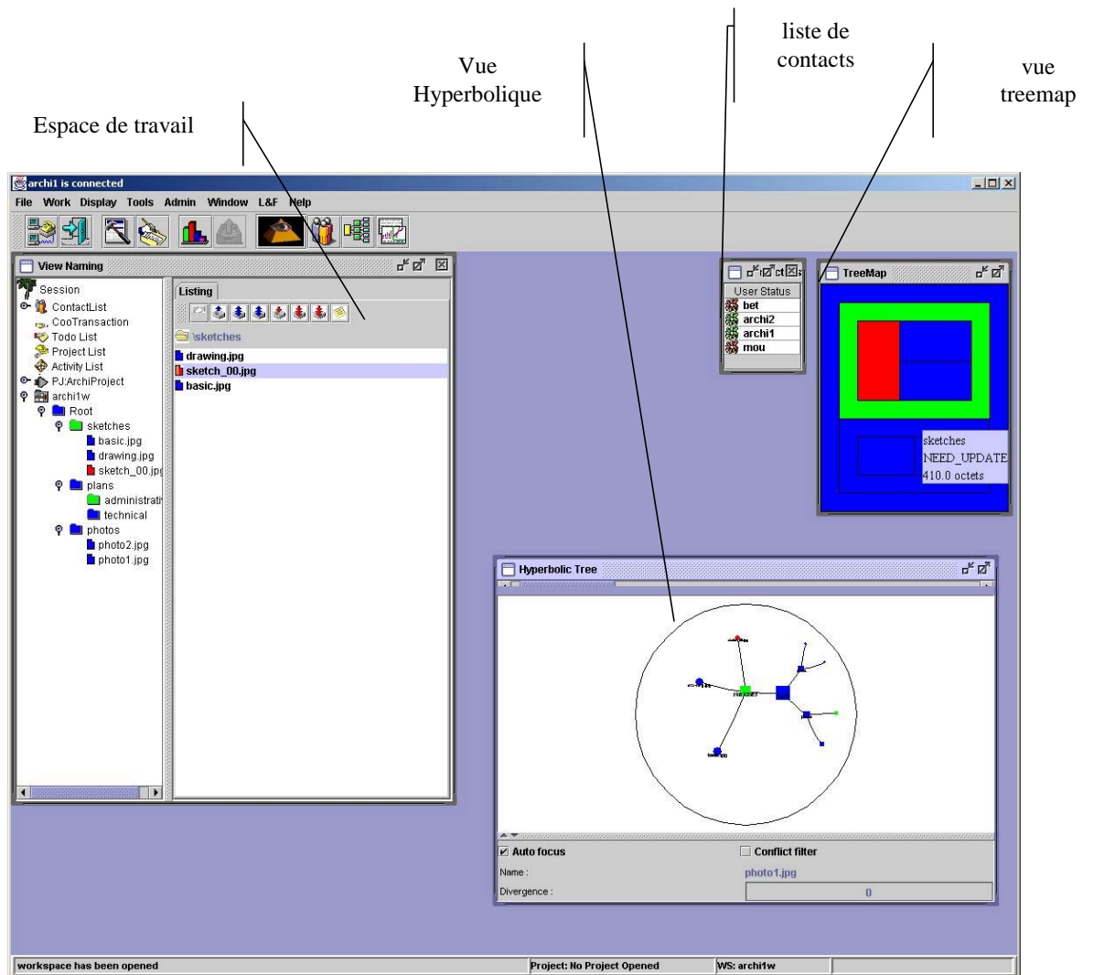
FIG. 5.1 – Interface utilisateur de MOTU
