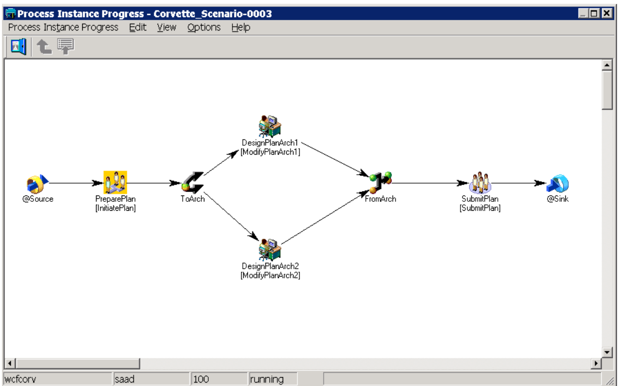
FIG. 5.4 – Définition d'un procédé WorkCoordinator
