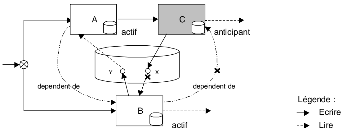
FIG. 4.17 – Interdiction des cycles de dépendances
