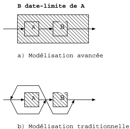
FIG. 3.6 – Modélisation d'une dépendance de type date-limite
