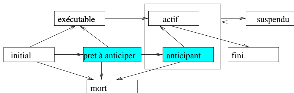
FIG. 4.4 – Diagramme d'états d'activité
