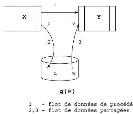
FIG. 4.15 – Flot de données
