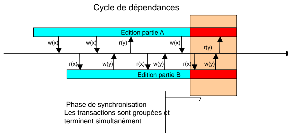
FIG. 4.11 – Cycle de dépendances
