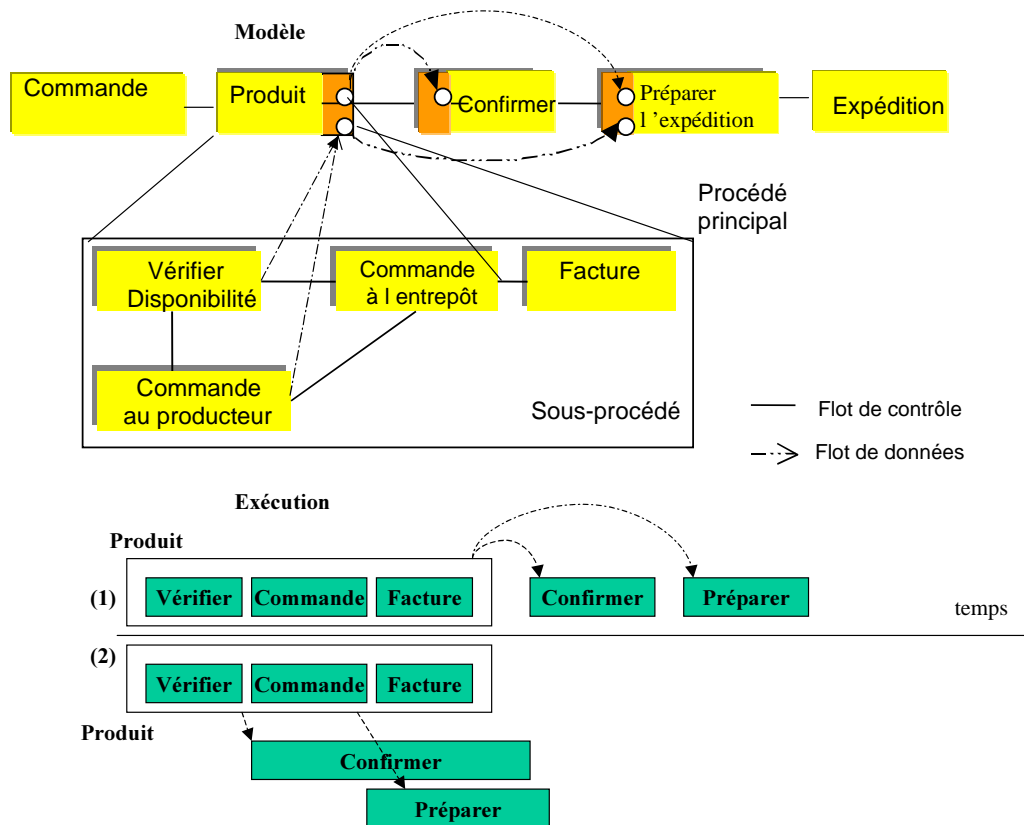
FIG. 4.7 – Echange de données entre procédés
