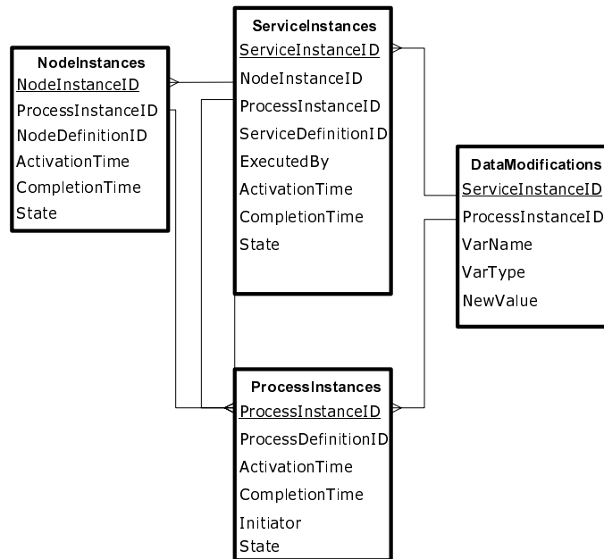
FIG. 6.1 – Schéma de la base de données de l'historique
