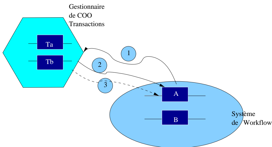
FIG. 4.14 – Terminaison d'une activité et de la transaction attachée
