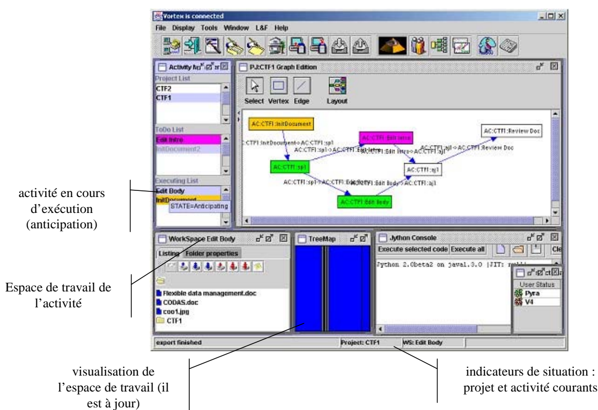
FIG. 5.3 – Intégration des services
