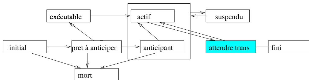
FIG. 4.13 – Diagramme d'états d'activité
