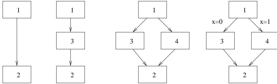
FIG. 3.10 – Insertion d'une activité
