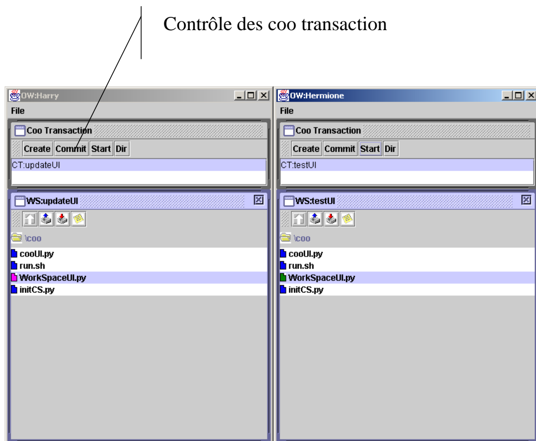
FIG. 5.7 – Vue des coo transactions
