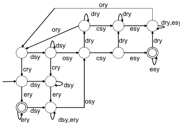
Figure 111 : Exemple d'instance de superviseur du module de contrôle de l'EPO "vérin Y"
