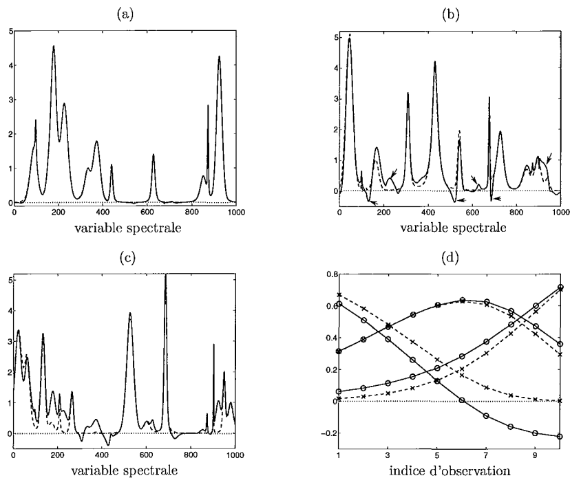
FIG. 5.5 – Résultat de la séparation en utilisant NNICA : (a,b,c) sources originales (discontinu) et sources estimées (continu). (d) coefficients de mélange originaux (croix) et coefficients identifiés (cercles).
