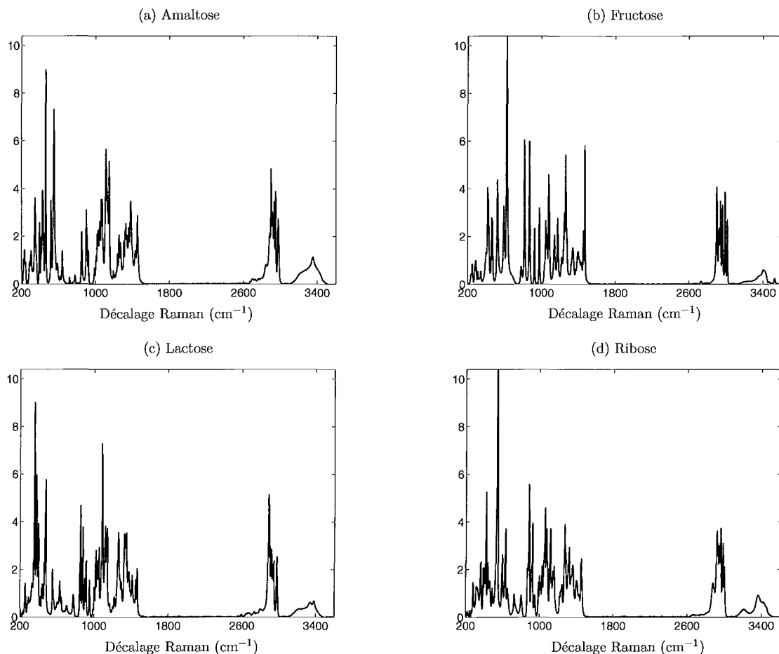
FIG. 6.2 – Spectres Raman des quatre composés organiques ( p=4 et n = 3400 ).
