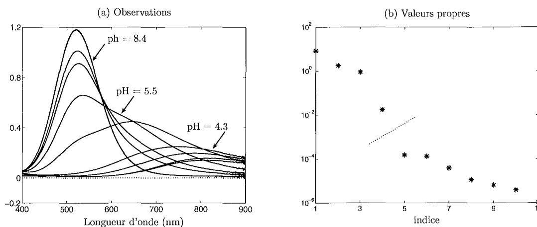
FIG. 6.14 – (a) Observations enregistrées pour plusieurs valeurs du pH et (b) valeurs propres de la matrice de covariance empirique des observations.
