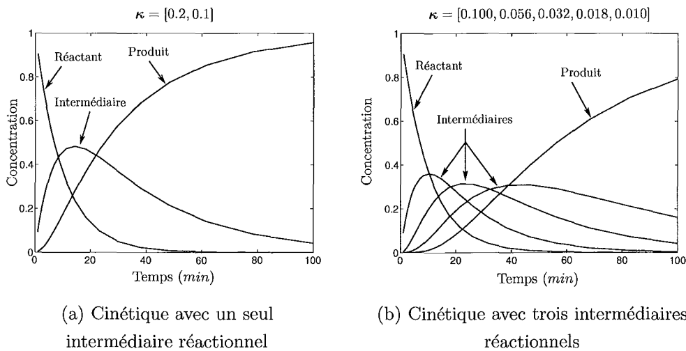
FIG. 5.2 – Coefficients de mélange simulés à partir d'une cinétique chimique.
