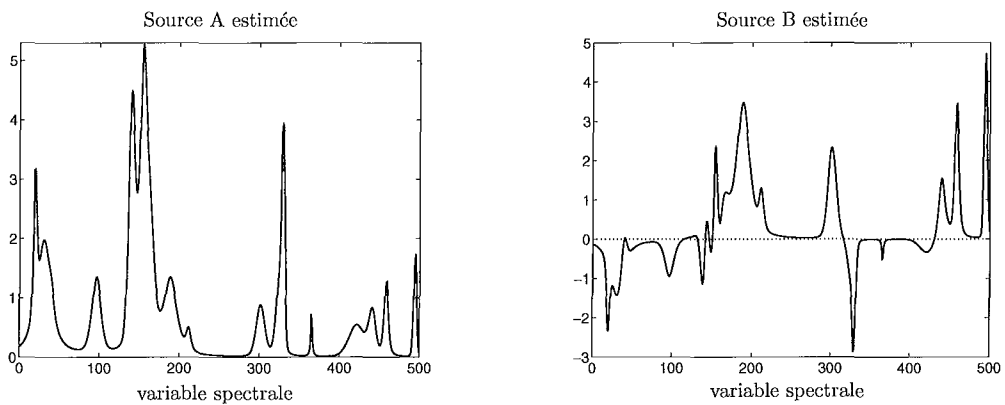
(b) Composantes indépendantes estimées à partir des mélanges bruts
