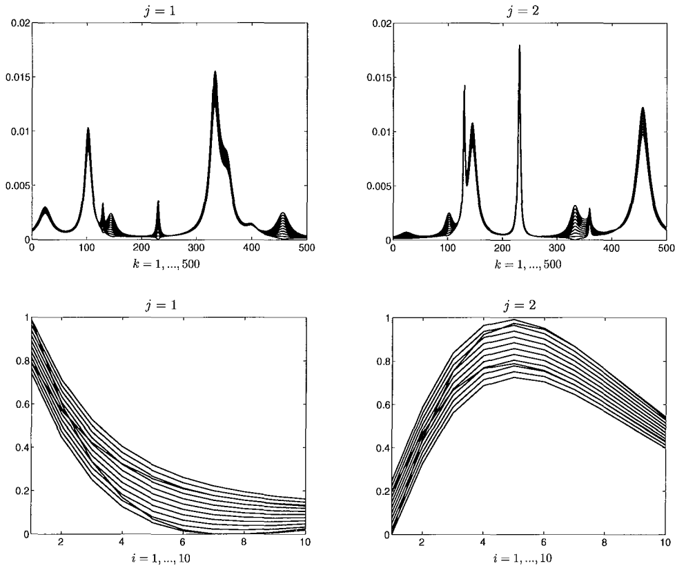
FIG. 2.2 – Quelques solutions admissibles des sources et des coefficients de mélange
