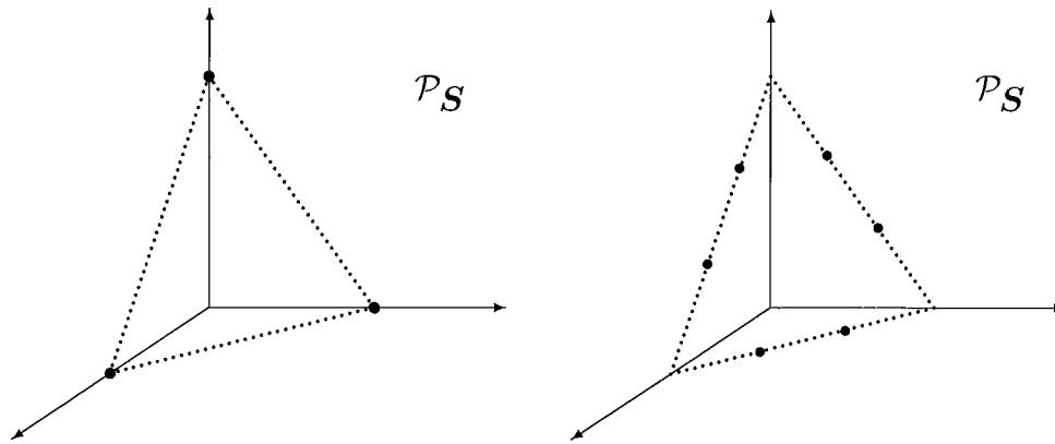
Cas 1 : Conditions de la proposition 3 Cas 2 : Conditions de Donoho-Stodden
