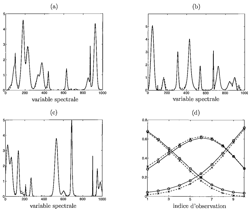
FIG. 5.7 – Résultat de la séparation en utilisant NNSC : (a,b,c) sources originales (discontinu) et sources estimées (continu). (d) coefficients de mélange originaux (croix) et coefficients identifiés (cercles).
