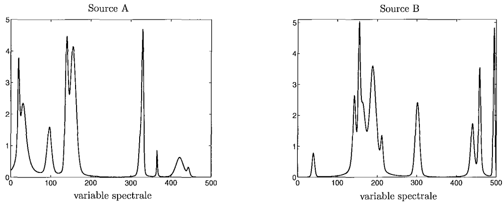
(a) Signaux sources avec un coefficient de corrélation \rho=+0.28 .
