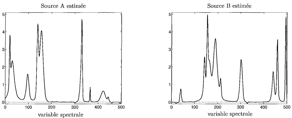
(c) Sources estimées en utilisant une analyse en composantes indépendantes sur les dérivées secondes
