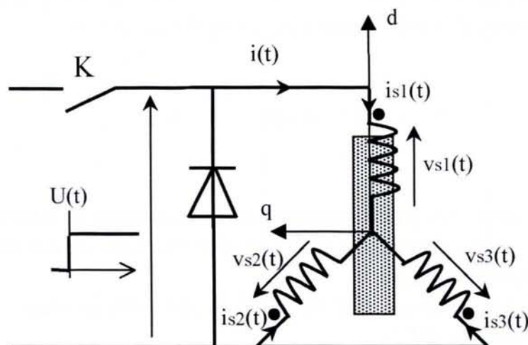
Figure III.2. Schéma du montage pour la méthode de l'échelon
