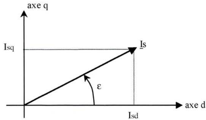
Figure V.1. Définition de l'angle de commande \varepsilon
