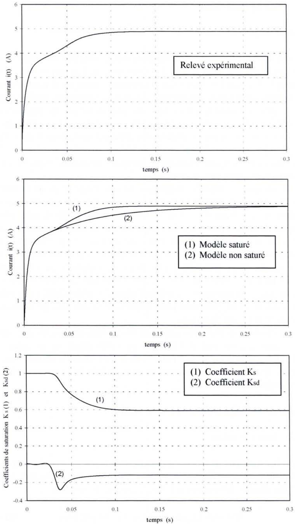
Figure III.13. Réponse en courant face à un échelon de tension en régime saturé; Essai suivant l'axe q
