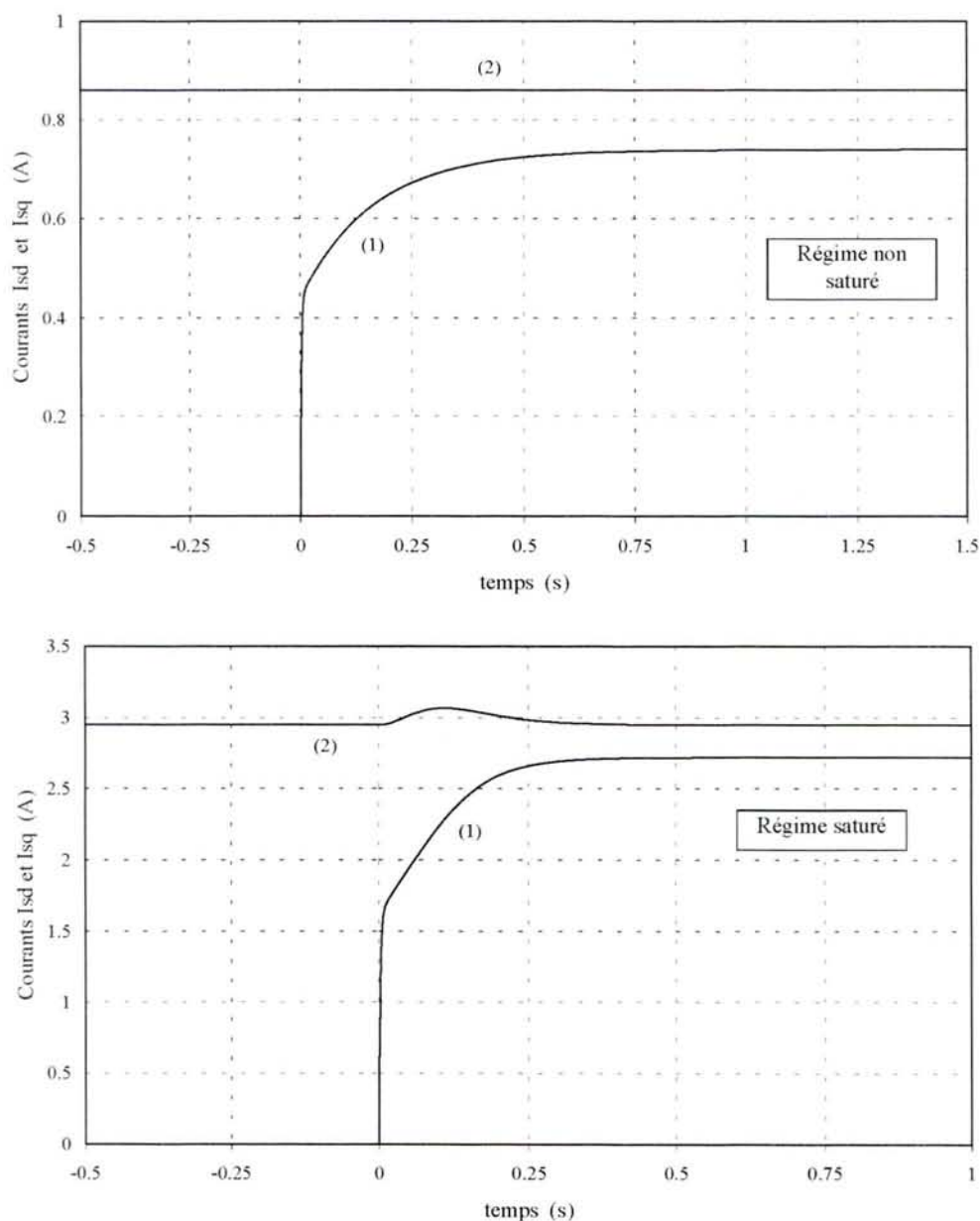
Figure III.21. Mise en évidence de l'effet croisé sur un transitoire; Résultats de simulation
