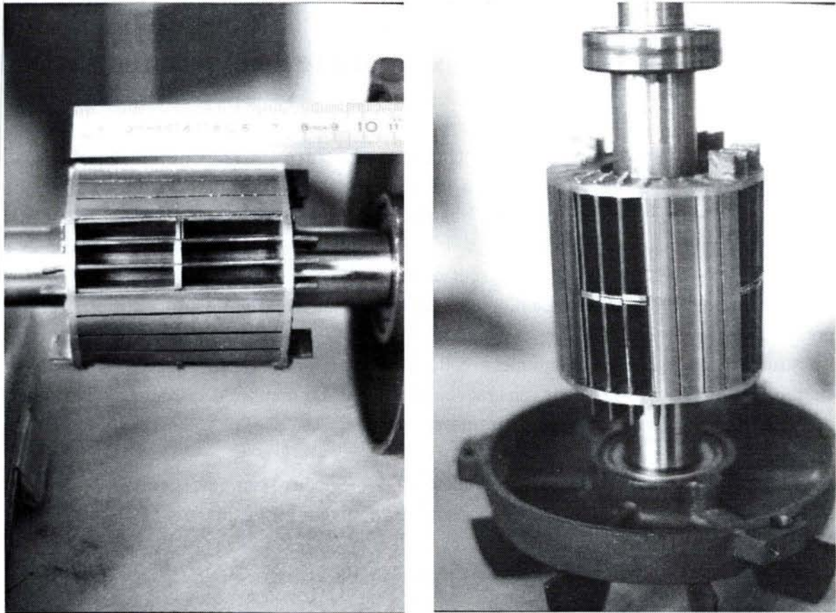
Figure AI.2. Vues détaillées du rotor
