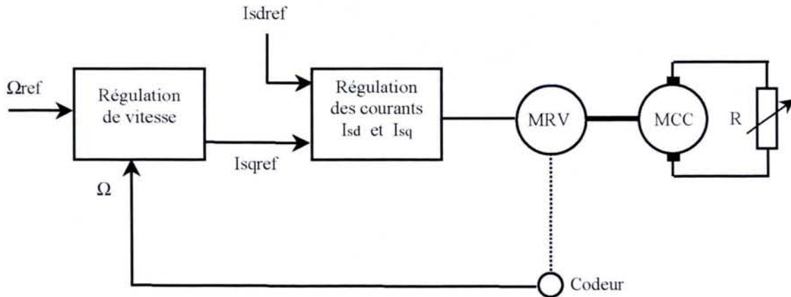
Figure V.5. Schéma du montage permettant de vérifier la loi de commande à couple maximal
