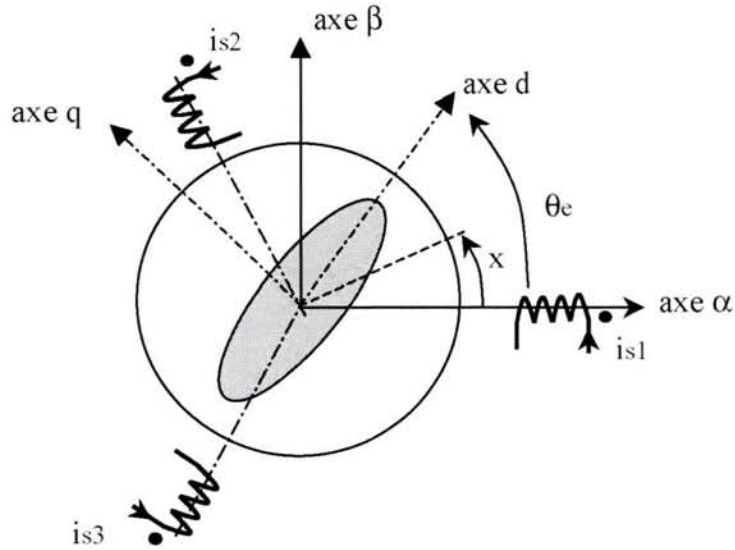
Figure I.8. Représentation symbolique de la machine
