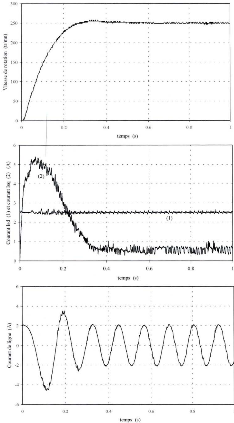
Figure IV 14. Echelon de vitesse de 250 tr/mm ; I_{sd} = 2,5A Résultats expérimentaux
