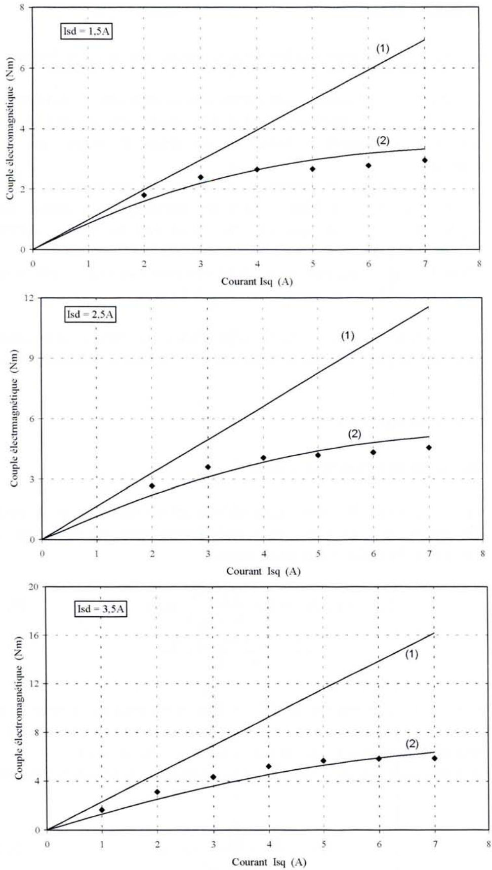
Figure IV.9. Couple électromagnétique en fonction de I_{sq} pour différentes valeurs de I_{sd} (1) Modèle non saturé (2) Modèle saturé ♦ expérience
