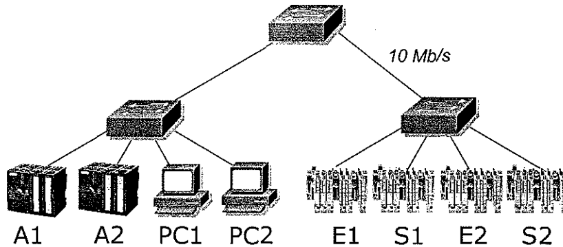
FIG. 4.17 – Exemple de réseau Ethernet Industriel
