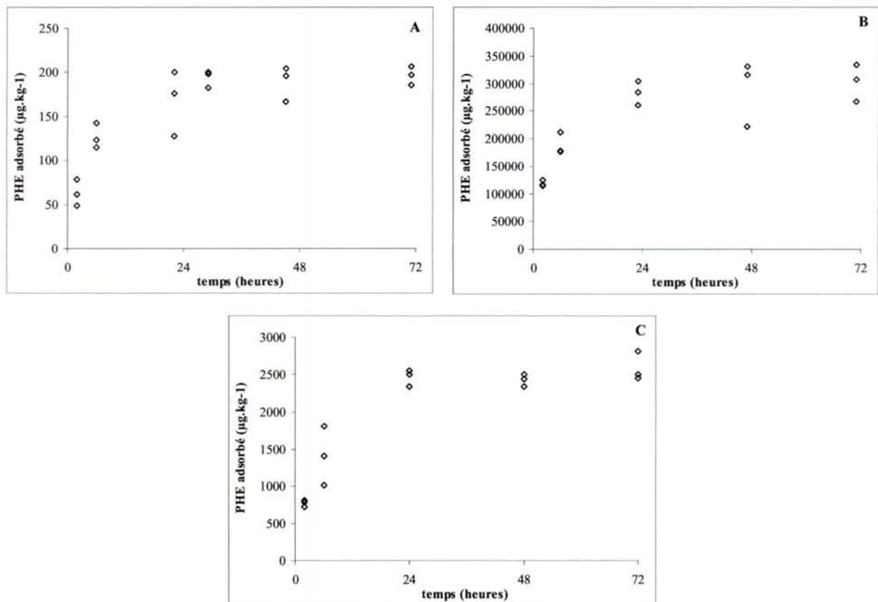
Figure 12. Cinétique d'adsorption du phénanthrène sur la pouzzolane (A), le charbon actif (B) et la pouzzolane recouverte de fioul (C).
