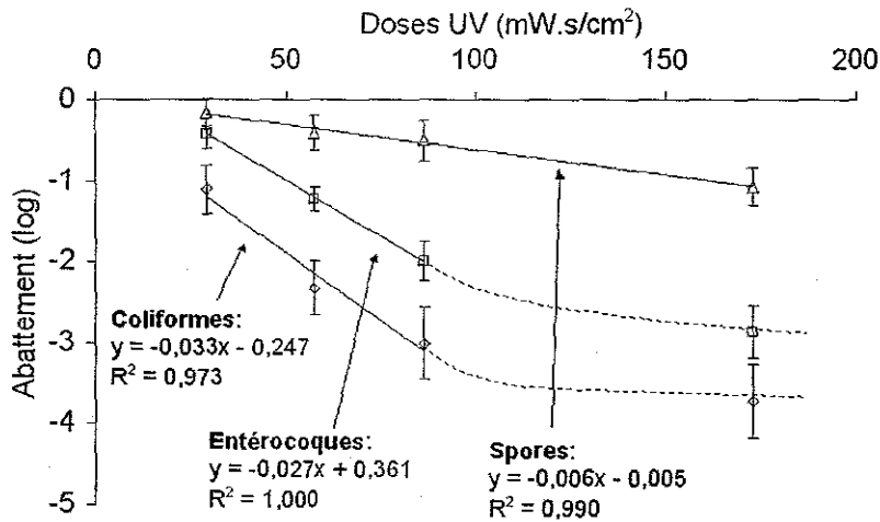
Figure 40 : Abattements calculés en fonction des doses UV pour les différents indicateurs bactériens
