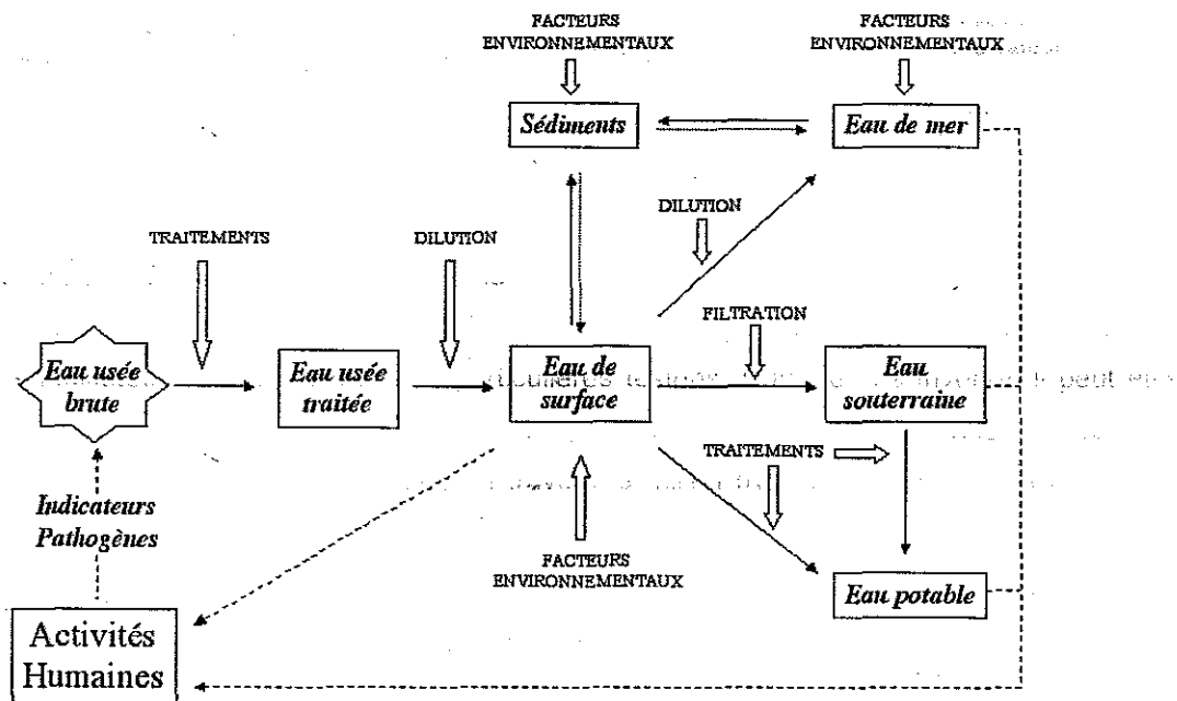
Figure 22: Parcours des indicateurs et des pathogènes dans le milieu hydrique
