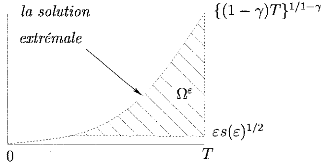
FIG. 1.3 – Le domaine \Omega^\varepsilon
