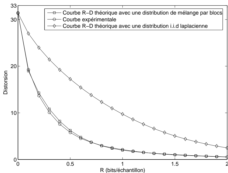
FIG. 4.11: Fonctions débit-distorsion pour la QVAZM - sous-bande V2 de l'image de Lena : données réelles, modèle de mélange proposé, modèle i.i.d laplacien - vecteurs de taille (4 \times 2) .
