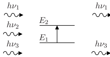
FIG. 1.6 – Absorption infrarouge.
