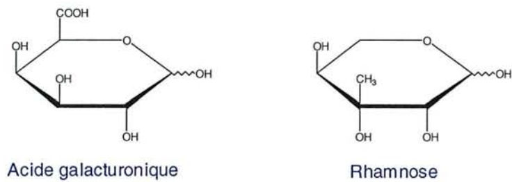
Figure 5 : Monomères constitutifs des substances pectiques.
