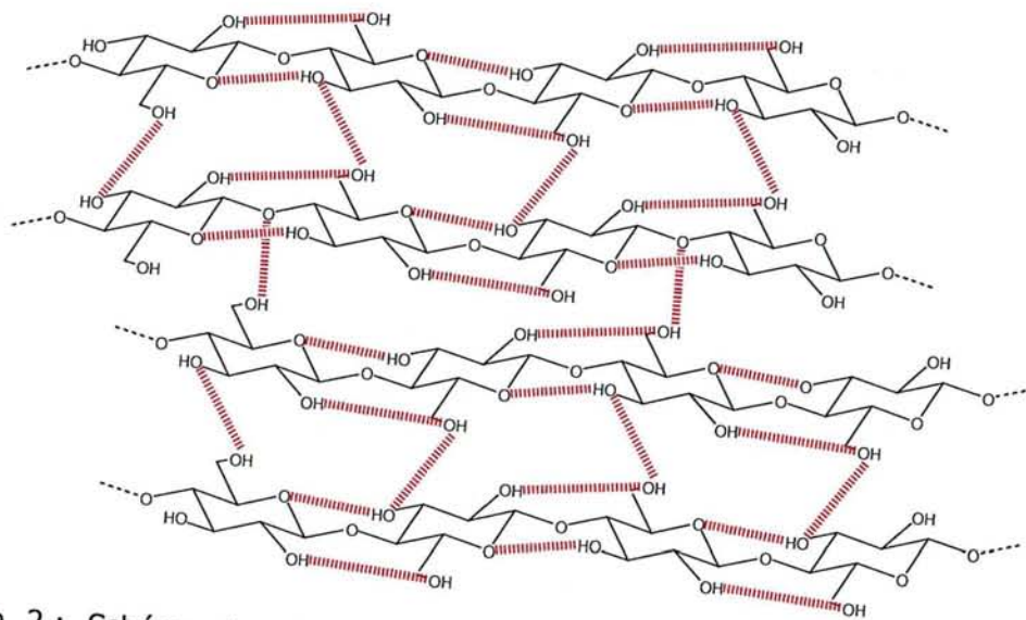
Figure 1 : Schéma de la structure primaire de la cellulose (Adapté de Béguin et Aubert, 1994).
