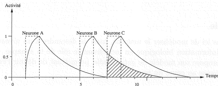
FIG. 1.4 – Neurones à fuite. L'activité des neurones est prolongée dans le temps, ce qui permet de corrélérer des événements impossibles à détecter avec des décharges classiques (ici en pointillés). D'après [Frezza-Buet et al., 2000]
