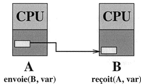
FIG. 3.2 – L'obtention de la donnée var par le processeur B nécessite deux opérations explicites. 1) Le processeur A demande explicitement l'envoi d'un message contenant var au processeur B . 2) Le processeur B demande explicitement la réception d'un message contenant var du processeur A .
