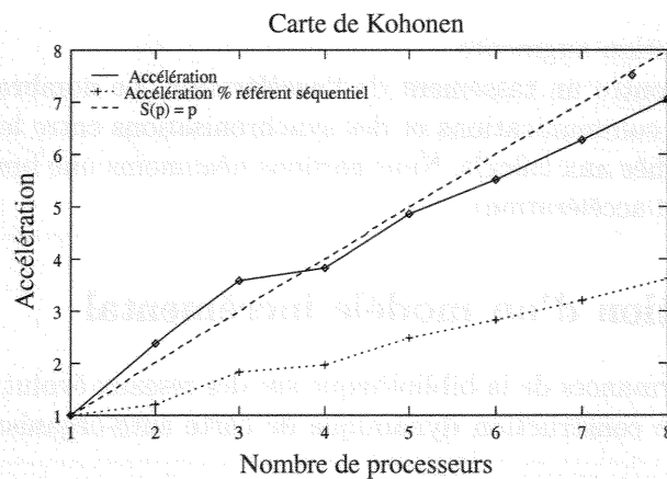
FIG. 9.4 – Accélération d'une carte de Kohonen. Nous avons placé l'accélération idéale (Accélération = Nombre de processeurs utilisés) et l'accélération par rapport au temps d'exécution du programme séquentiel.
