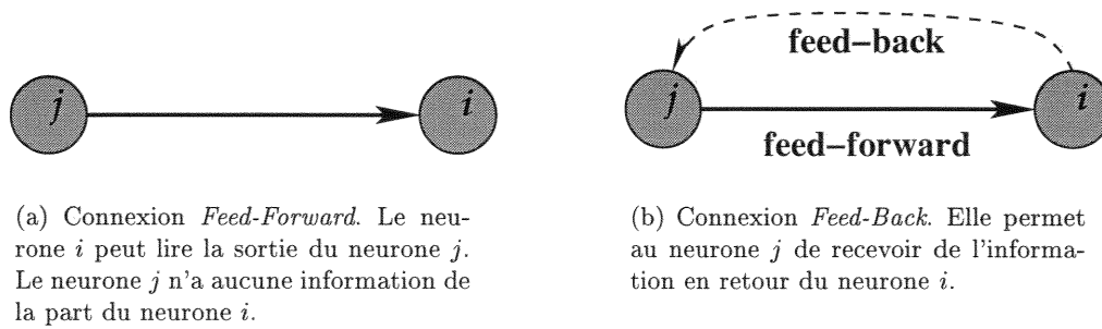
FIG. 2.2 – Les deux types de connexions du neurone i au neurone j .
