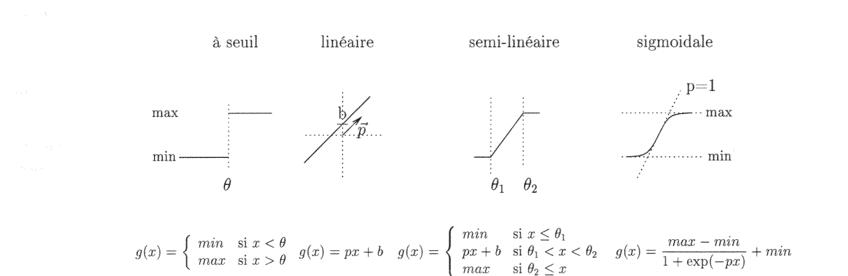
FIG. 1.3 – Les quatre fonctions de transfert les plus fréquemment utilisées dans les neurones artificiels
