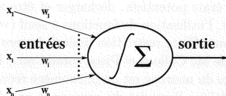
FIG. 1.2 – Un neurone formel
