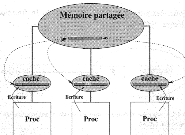
FIG. 8.3 – Faux partage de cache. Des données différentes et chacune modifiée par un processeur différent de la machine partagent une même ligne de cache.
