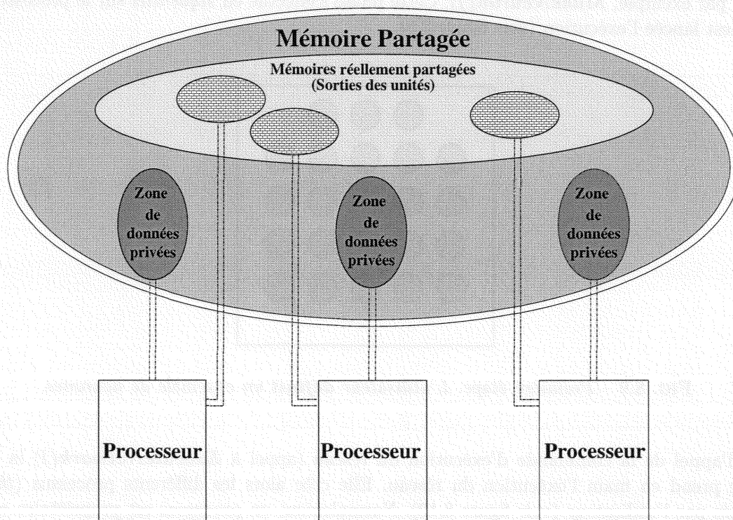
FIG. 8.8 – Notre gestion de la mémoire. La mémoire partagée est scindée en deux parties. Une première contenant les variables non partagées par les différents processeurs. Une seconde contenant les variables partagées, accessibles en lecture à tous les processeurs. Cette dernière est séparée en zones de données modifiables par un unique processeur.
