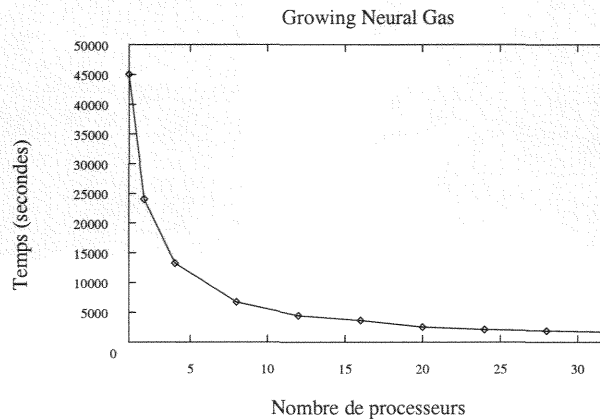
FIG. 9.8 – Temps d'exécution d'un réseau de type Growing neural gas en fonction du nombre de processeurs utilisés.
