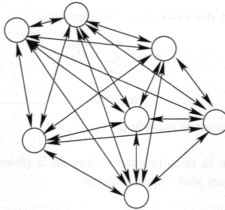
FIG. 2.9 – Réseau de Hopfield. Un neurone est lié à tous les autres, les liaisons sont symétriques, un neurone n'est pas lié à lui-même et un seul neurone est actualisé par itération. Chaque neurone est à la fois neurone d'entrée et de sortie du réseau.
