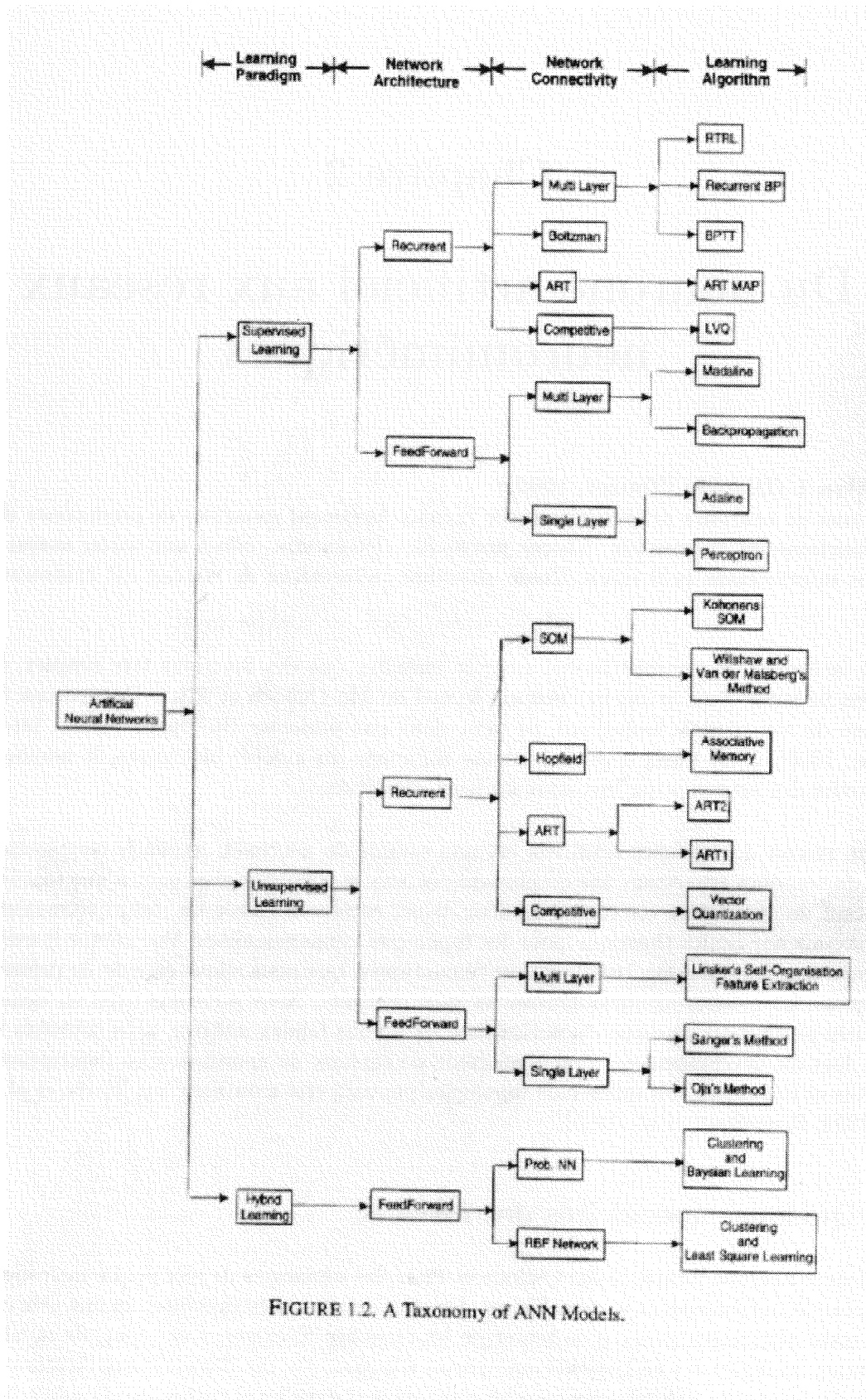
FIG. 2.1 – Un exemple de taxonomie des réseaux de neurones. D'après [Sundararajan et Saratchandran, 1998]
