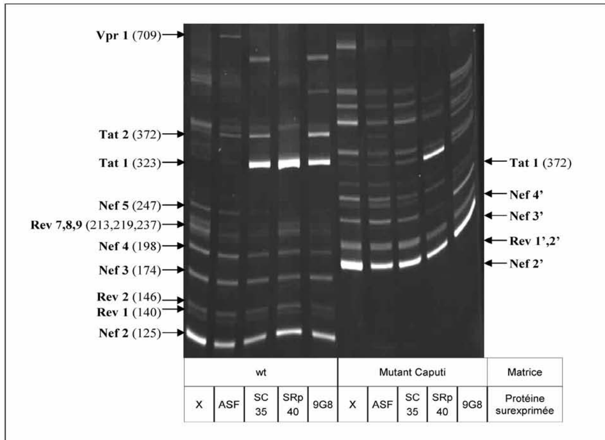
Fig. 80 : Effet de la mutation mutESS2 sur l'épissage du transcrite du plasmide p\Delta PSP dans des cellules HeLa
