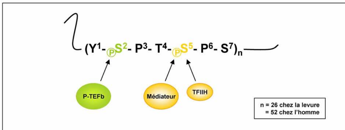
Fig. 14 : Site de phosphorylation du CTD (D'après Hirose and Ohkuma, 2007)
