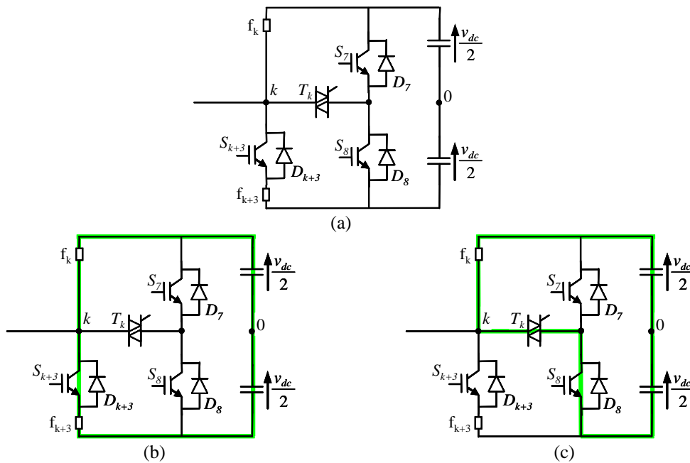
Figure 3-5. (a) Circuit équivalent de la phase k du CCM pour la topologie avec bras redondant lors d'un défaut de type court-circuit.
