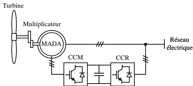
Figure 1-1 : Système éolien à vitesse variable basé sur une MADA.
