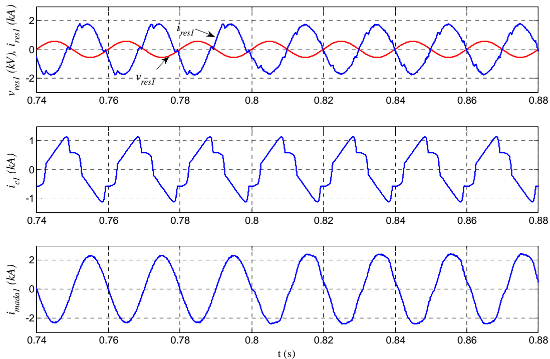
Figure 2-20 : Grandeurs électriques au PRR avant et après la compensation de la puissance réactive et des courants harmoniques prépondérants du réseau de rangs 5 et 7 à t = 0,8 s.
