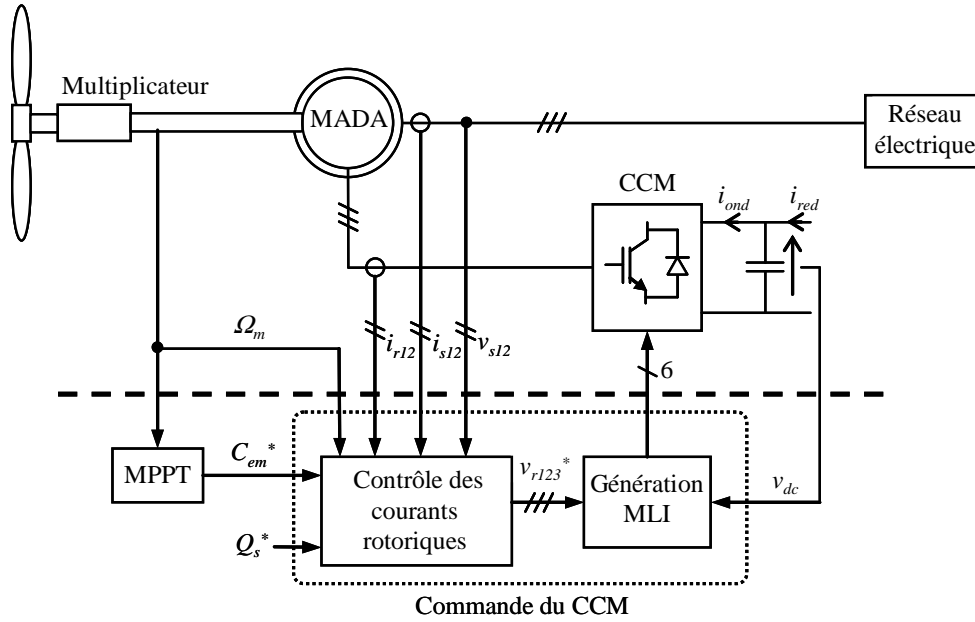
Figure 1-12 : Principe de la commande du CCM.
