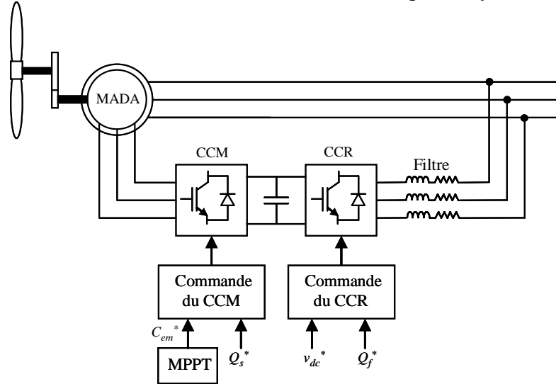
Figure 1-7 : Architecture de commande du système éolien.
