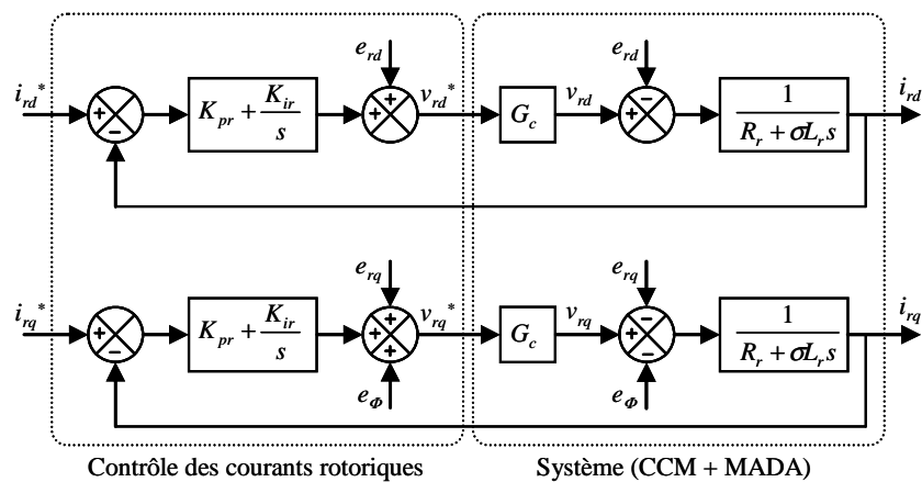
Figure 1-15 : Principe du contrôle des courants rotoriques de la MADA.
