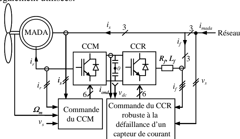
Figure 4-2. Système éolien robuste à la défaillance d’un capteur de courant.
