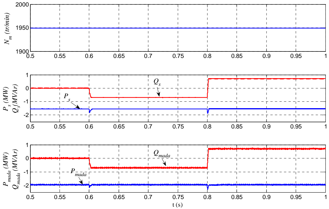
Figure 2-12 : Mode hypersynchrone : vitesse mécanique de la MADA, puissances active et réactive statoriques et puissances active et réactive fournies par la MADA au réseau.
