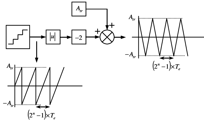
Figure 5-10. Génération numérique de la porteuse triangulaire.
