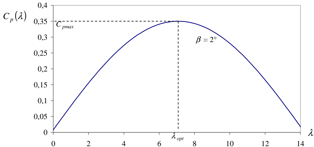
Figure 1-10 : Coefficient de puissance C_p en fonction de \lambda pour \beta = 2^\circ .
