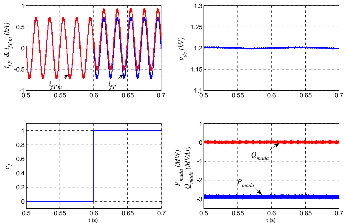
Figure 4-16. Performance du système éolien intégrant la commande du CCR proposée : défaut de type offset du capteur de la phase 1.
