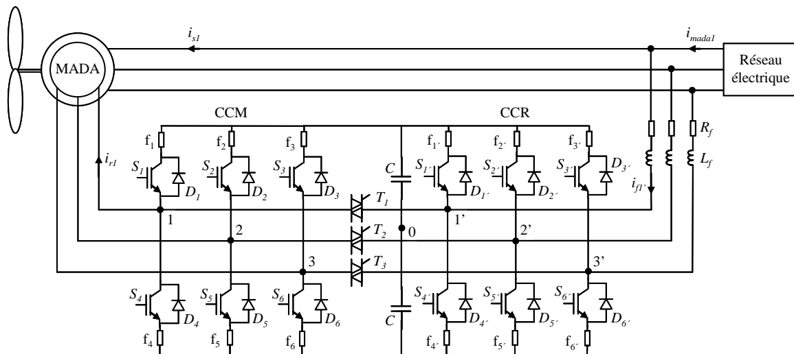
Figure 3-2. Système éolien basé sur une MADA intégrant une topologie “fault tolerant” sans bras redondant.
