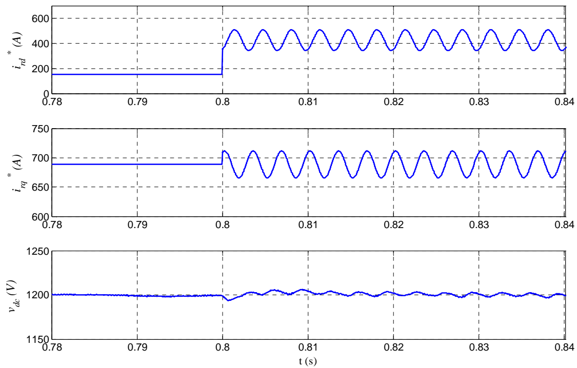
Figure 2-19 : Courants rotoriques totaux de référence et tension du bus continu avant et après la compensation de la puissance réactive et des courants harmoniques prépondérants de rangs 5 et 7 à l'instant t = 0,8 s.
