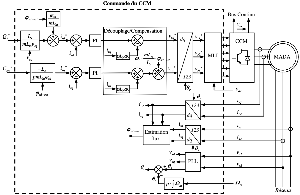
Figure 1-16 : Commande du CCM.
