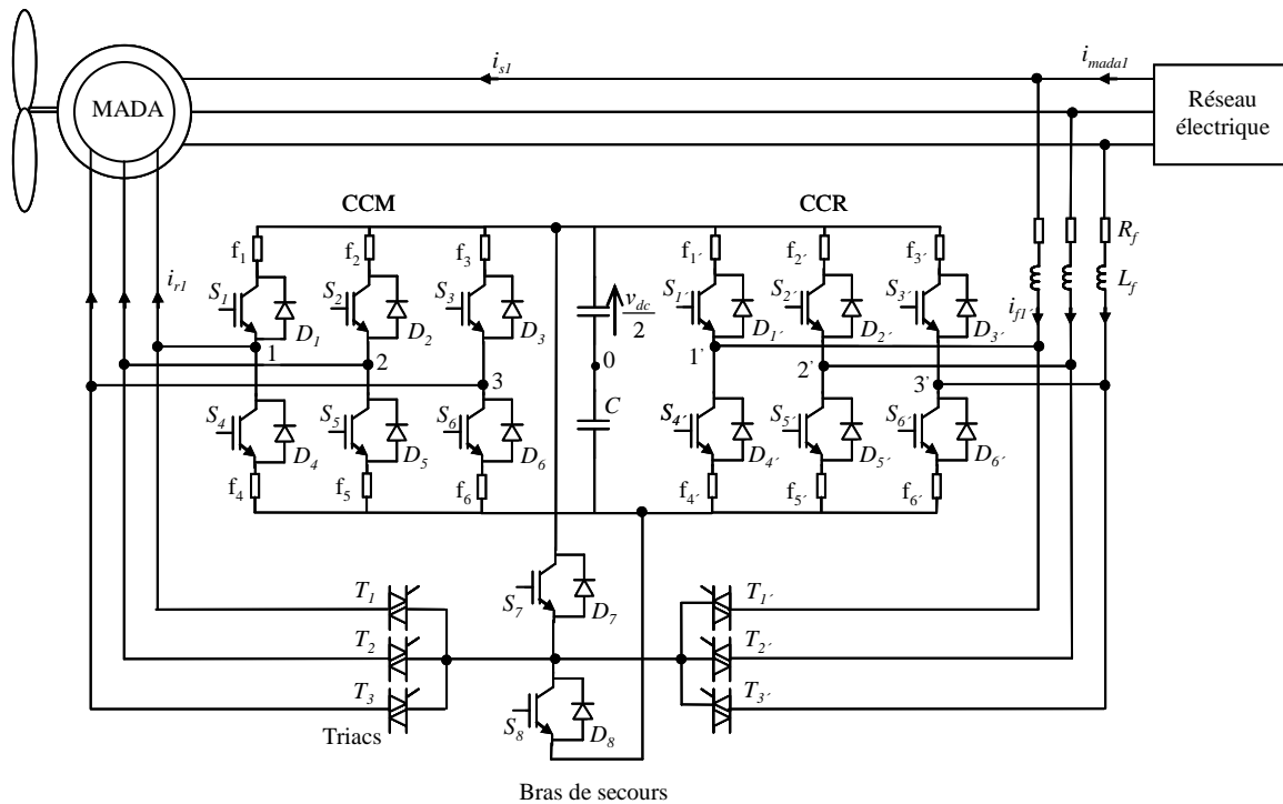
Figure 3-1. Système éolien basé sur une MADA intégrant une topologie “fault tolerant” avec un bras redondant.
