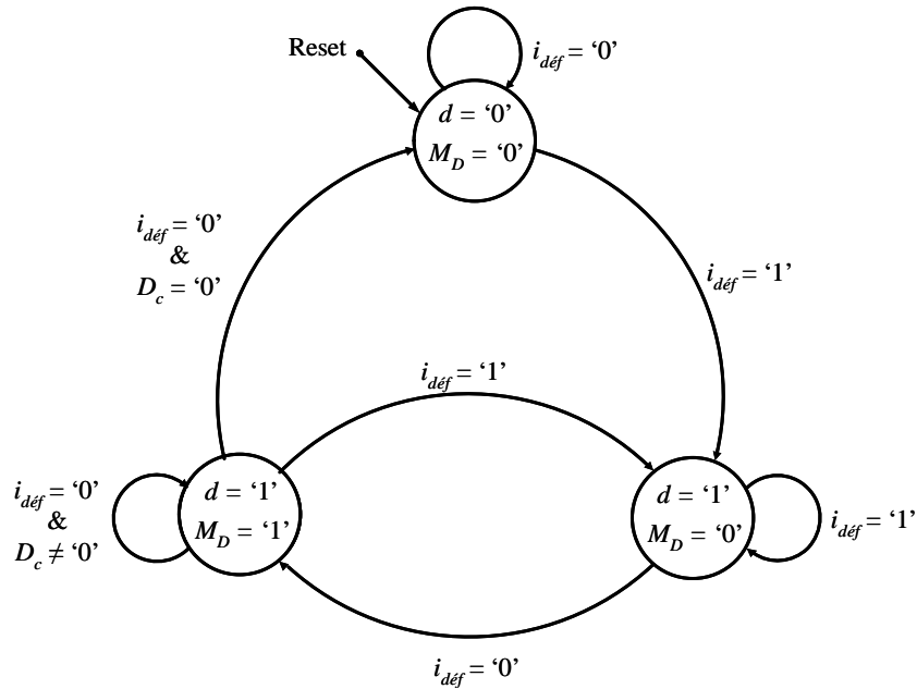
Figure 5-22. Graphe d'états de la mémorisation du défaut.
