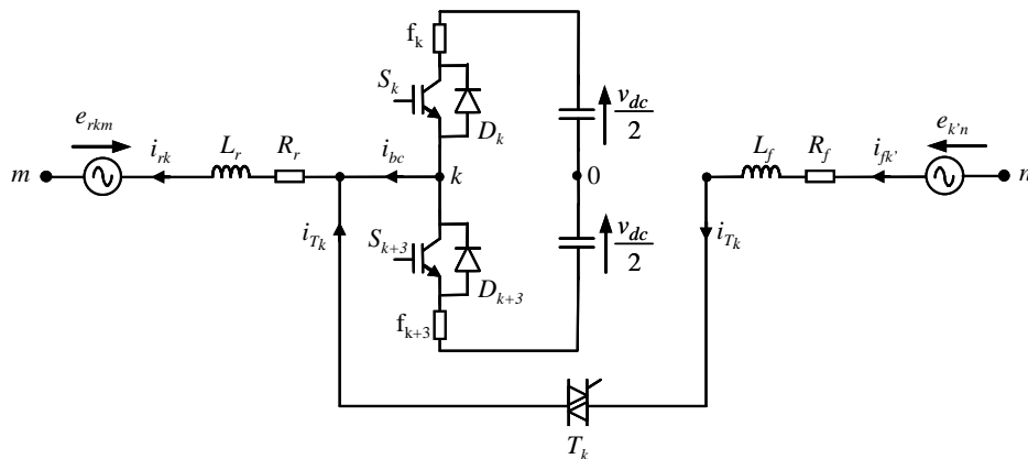
Figure 3-19. Connexion du bras commun pour la topologie sans bras redondant lors d'un défaut de type court-circuit au niveau du bras k' du CCR.
