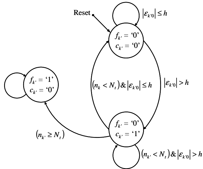
Figure 5-11. Graphe d'états de la détection de défaut.
