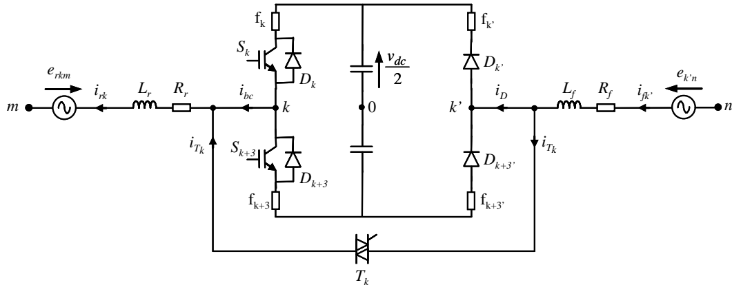
Figure 3-18. Connexion du bras commun pour la topologie sans bras redondant lors d'un défaut de type circuit-ouvert au niveau du bras k' du CCR.
