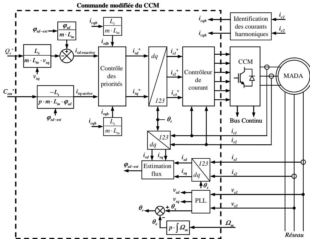
Figure 2-8 : Commande modifiée du CCM intégrant un contrôle des priorités pour les courants rotoriques.
