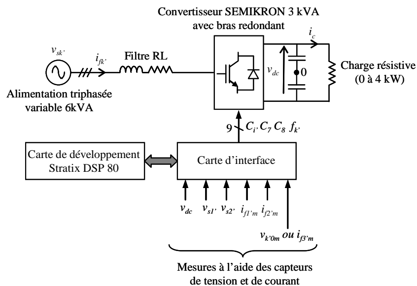
Figure 5-28. Principe du banc d’essai expérimental.
