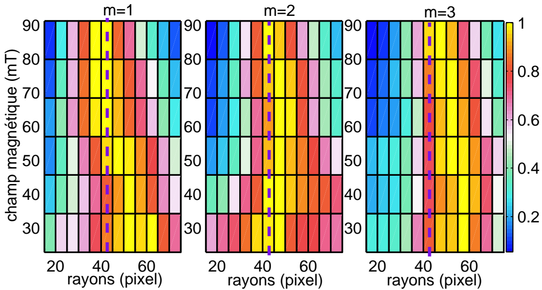
FIG. 3.22 – Localisation des maxima des modes m = 1 (gauche), m = 2 (milieu) et m = 3 (droite) en fonction du champ magnétique. La position radiale de la triple sonde est indiquée par un trait vertical à 43 pixels.
