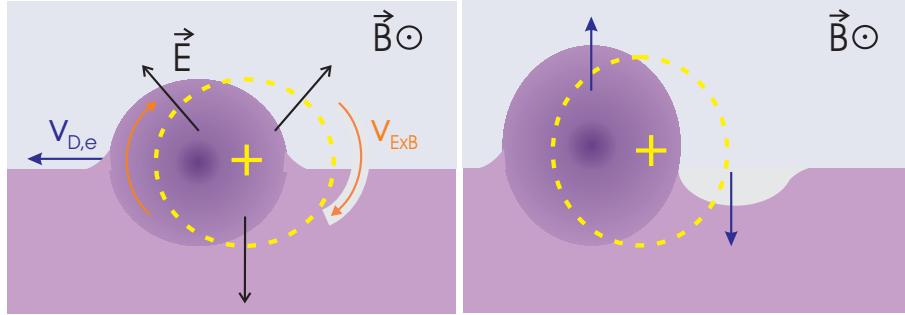
FIG. 1.4 – Une perturbation de densité dans un plasma non-uniforme. Le potentiel, en jaune est en retard sur la densité. Les dérives v_{E \times B} ne contribuent plus seulement à la propagation de la perturbation, mais aussi à sa croissance.
