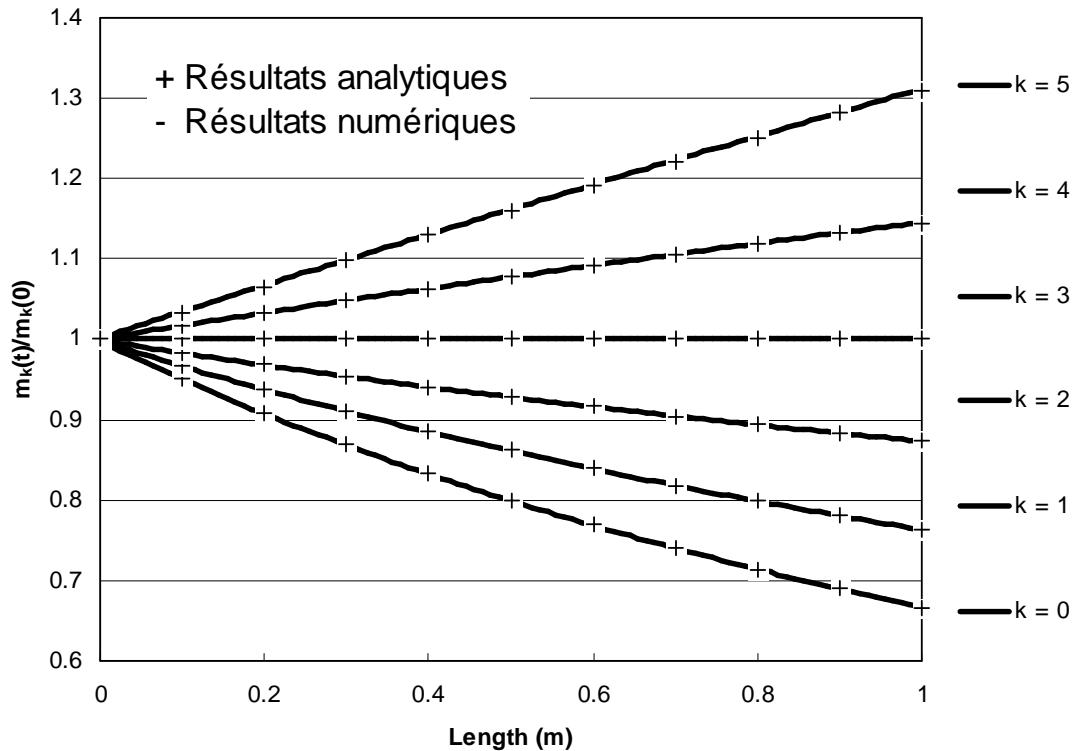
Figure 4.10 : Résultats adimensionnés de la validation du couplage Fluent®/Multi-QMOM pour un écoulement uniforme v_x = 1\text{m/s} en conduite avec une vitesse d’agrégation constante \beta_0 = 1\text{m}^3/\text{s} , un pas de temps de \Delta t = 0.05\text{s} sur une distance d’1 mètre découpée par 100 cellules identiques.
