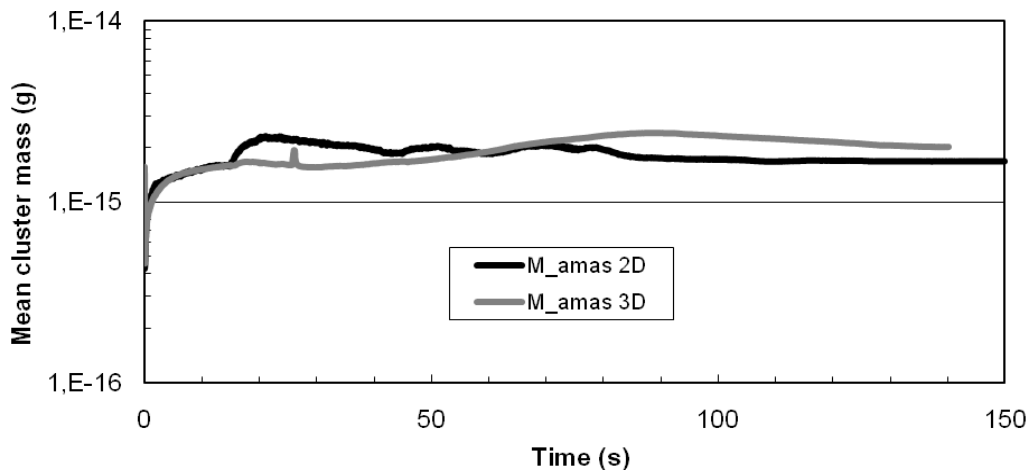
Figure 5.45 : Évolution temporelle de la masse moyenne d'un l'amas lorsque l'injection du titane est réalisée 15 secondes après celle de l'aluminium pour les maillages 2D et 3D.
