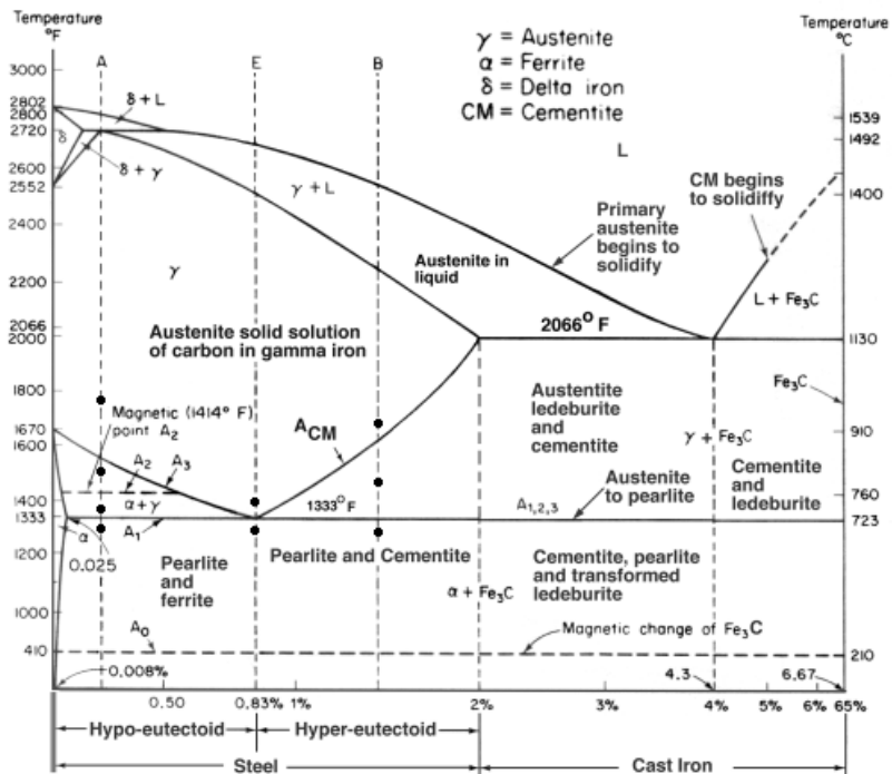
Figure 3 : Diagramme de phase Fer-Carbone.
