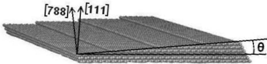
Figure A-6 : Illustration de la notion de face vicinale avec la face (788) vicinale de la face (111) d'un réseau métallique cubique à faces centrées (d'après « Nanoobjets sous contrôle », CNRS publications, 2009)
