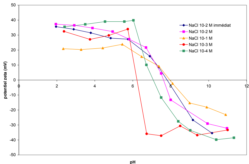
Figure C-9 : Mesures du potentiel électrocinétique des particules de quartz Roth-goëthite ; la courbe notée « NaCl 10-2 M immédiat » a été tracée sans délai d'équilibrage après l'immersion du solide dans la suspension.
