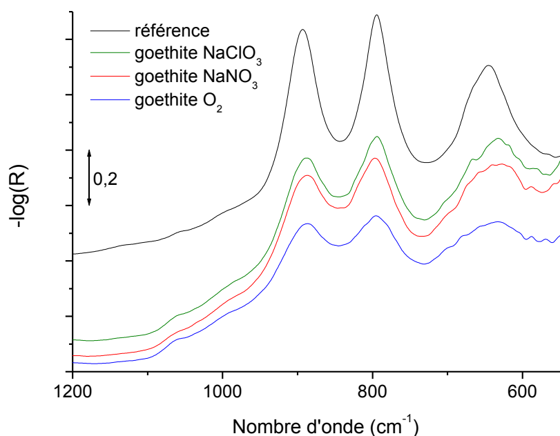
Figure B-3 : Spectres infrarouges collectés en mode réflexion diffuse des trois variétés de goëthite préparées avec différents oxydants, ainsi qu'une goëthite de référence bien cristallisée (Gaboriaud et Ehrhardt, 2001). L'ordonnée est une pseudo-absorbance, R représente le rapport des intensités diffusées par l'échantillon et par KBr, non absorbant dans ce domaine, pris comme référence.
