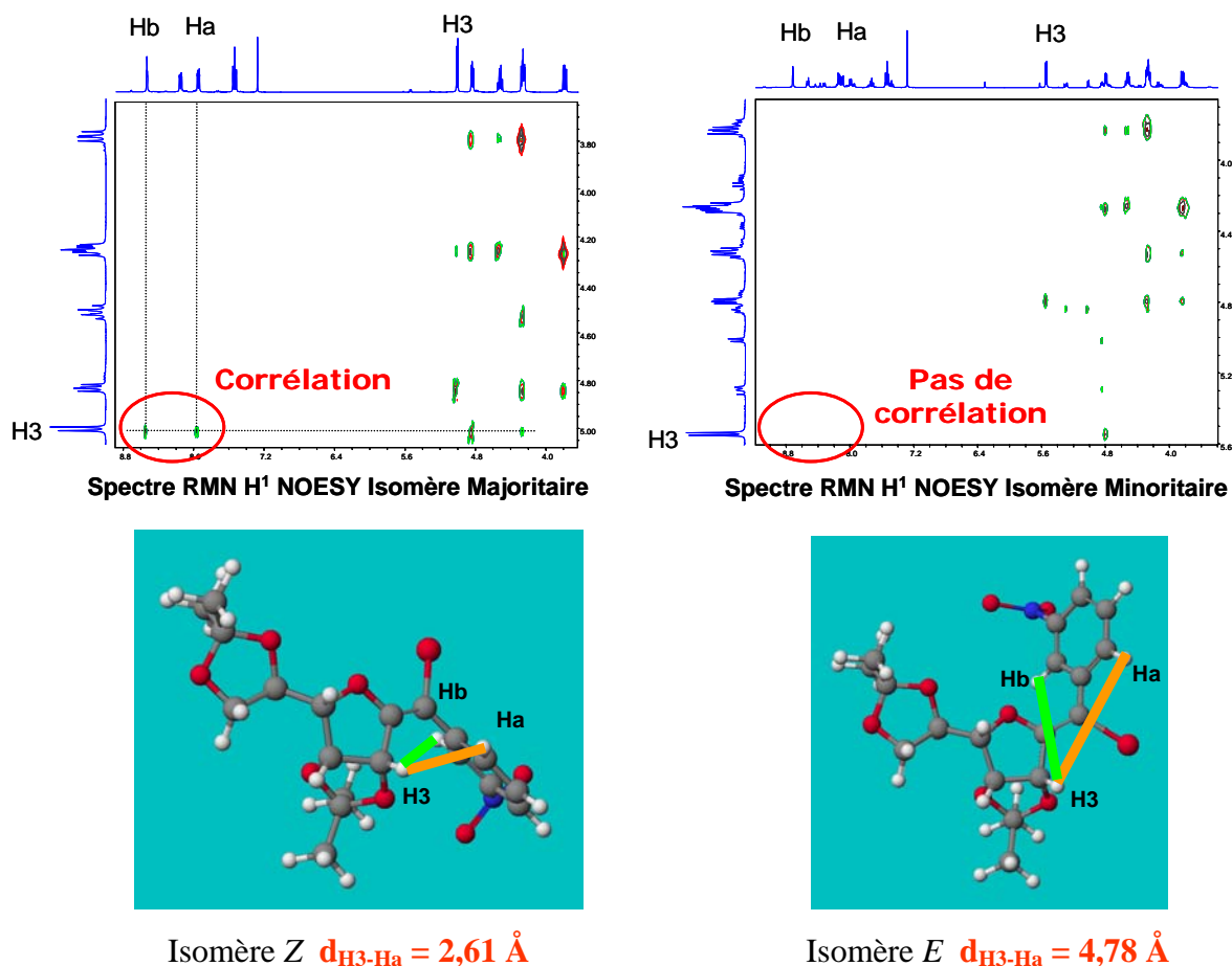
Figure 8. Carte NOESY et calcul des distances des protons Ha et Hb avec H-3 sur les deux isomères E et Z issus de la monosubstitution de l' exo -glycol dibromé avec l'acide 3-nitrophénylboronique
