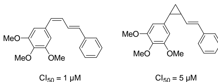
Figure 20. Dérivés de la combretastatine après élongation du pont éthylénique
