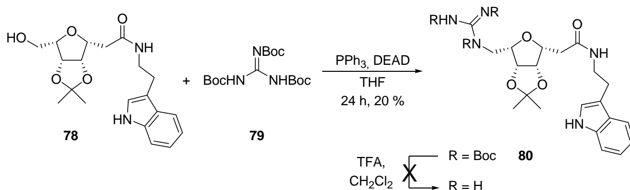
Schéma 95. Réaction de Mitsunobu entre l'alcool 78 et la guanidine triBoc 79
