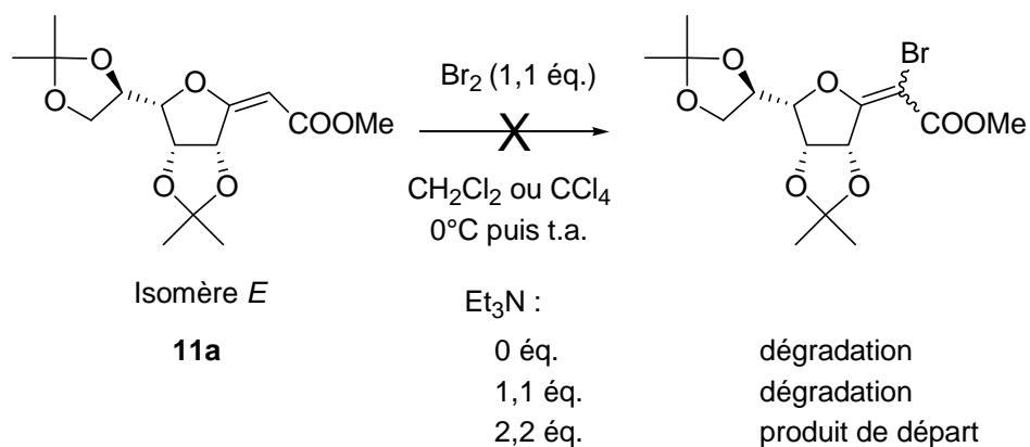
Schéma 53. Essai de bromation du composé 11a
