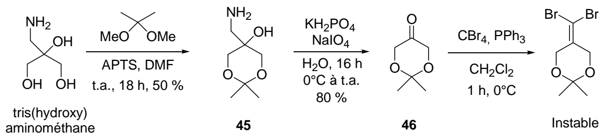
Schéma 79. Synthèse du dérivé dibromoéthylène
