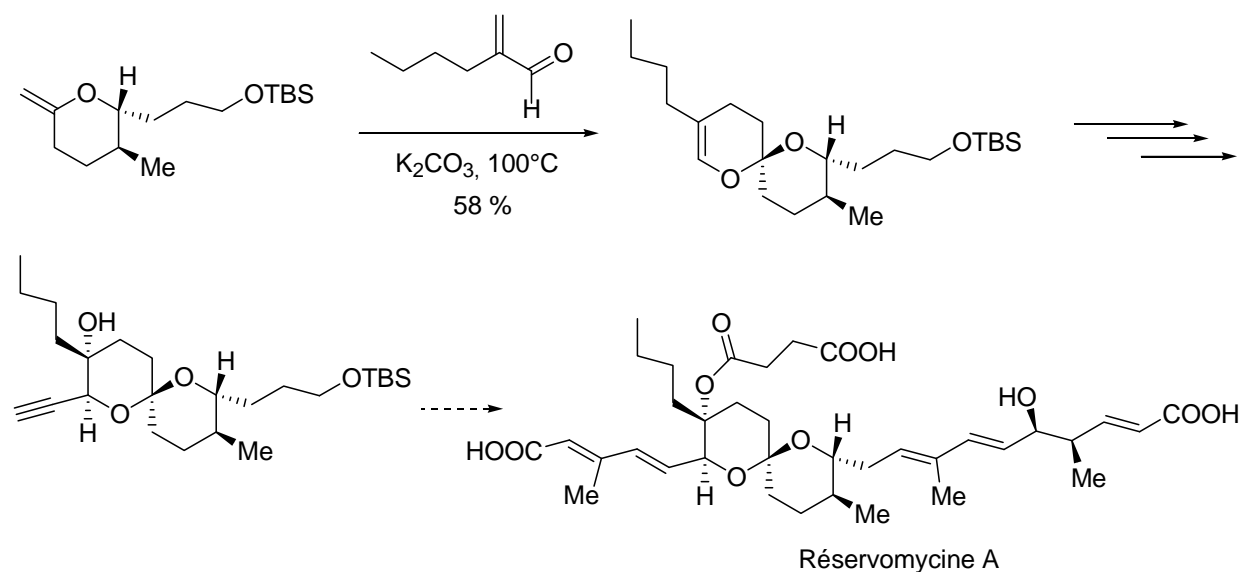
Schéma 22. Synthèse partielle de la réservomicine A
