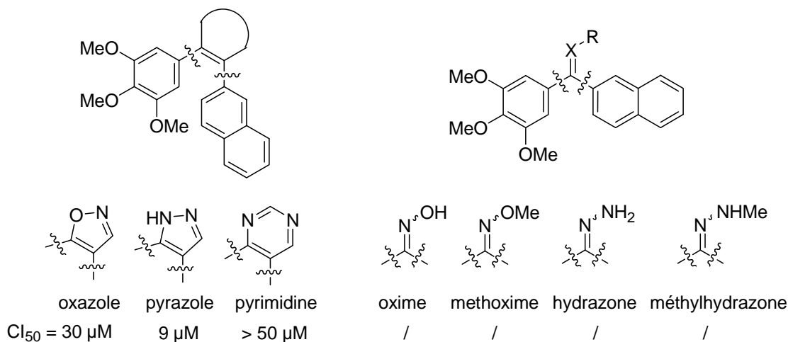
Figure 18. Influence du remplacement de la fonction centrale des naphtylcombrétastatines et phenstatines
