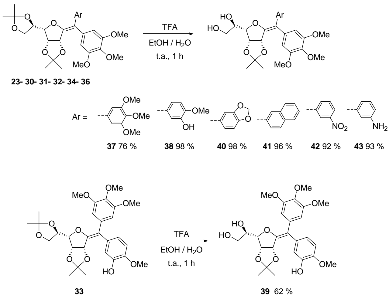
Schéma 77. Réaction de déprotection sélective de l'isopropylidène 6,7
