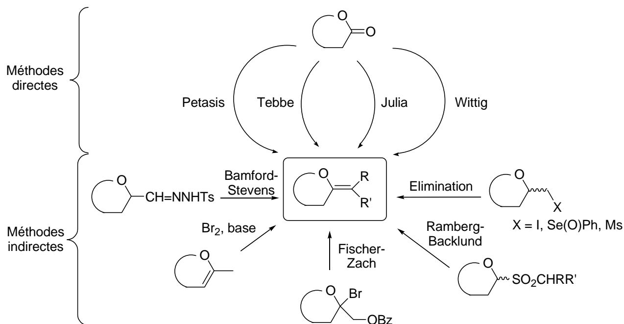
Figure 2. Différentes voies d'accès aux exo -glycols
