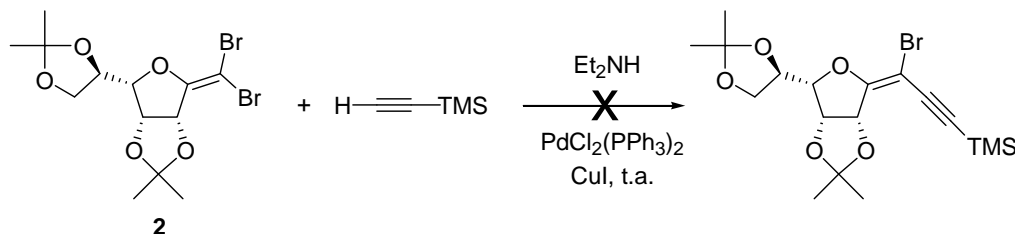
Schéma 43. Essai en couplage de Sonogashira sur l' exo -glycol dibromé
