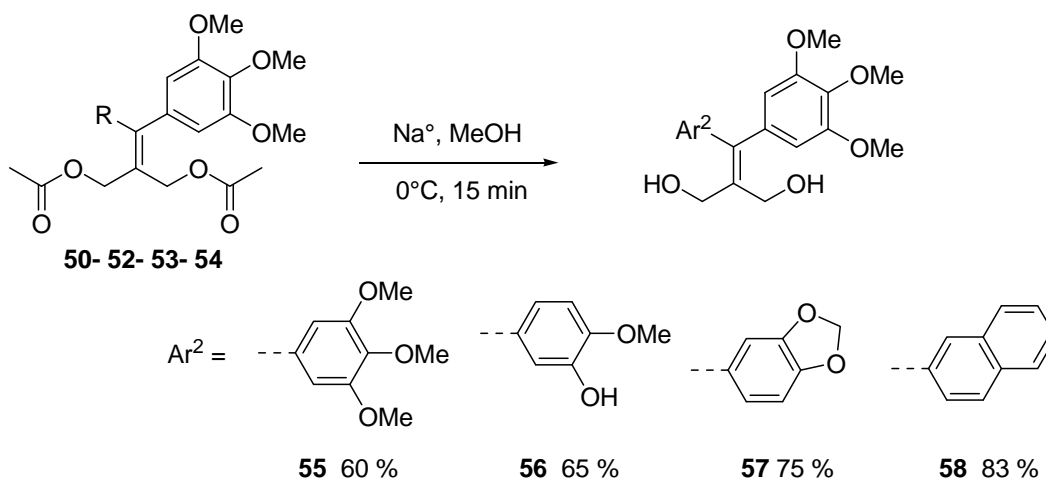
Schéma 82. Déprotection des acétates par réaction de Zemplen
