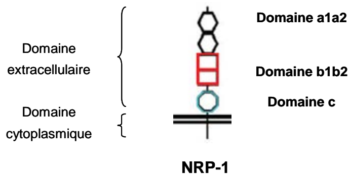
Figure 34. Les différents domaines du récepteur NRP-1
