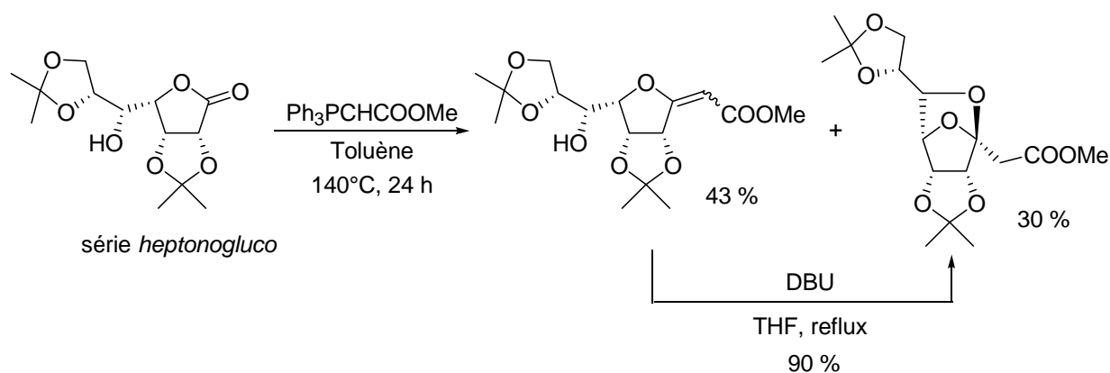
Schéma 4. Formation de bicyclic osidique
