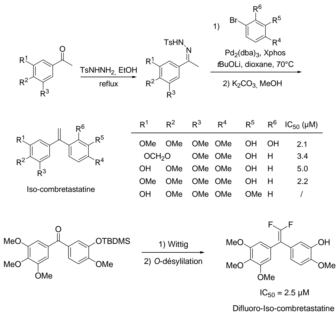
Schéma 73. Synthèse et activité biologique des dérivés de l'iso-combretastatine
