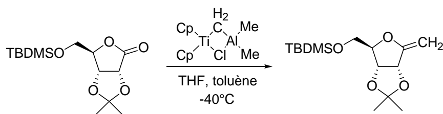
Schéma 7. Oléfination par le réactif de Tebbe
