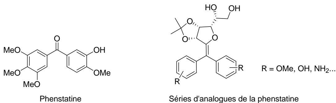
Figure 5. Figure générale des analogues visés de la phenstatine
