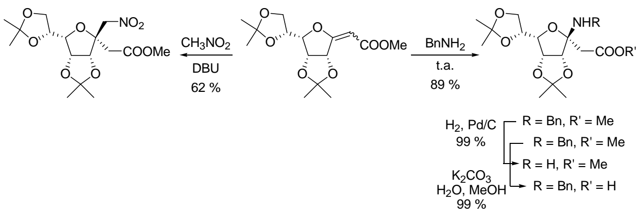
Schéma 5. Synthèse d'acides \beta et \gamma -aminés
