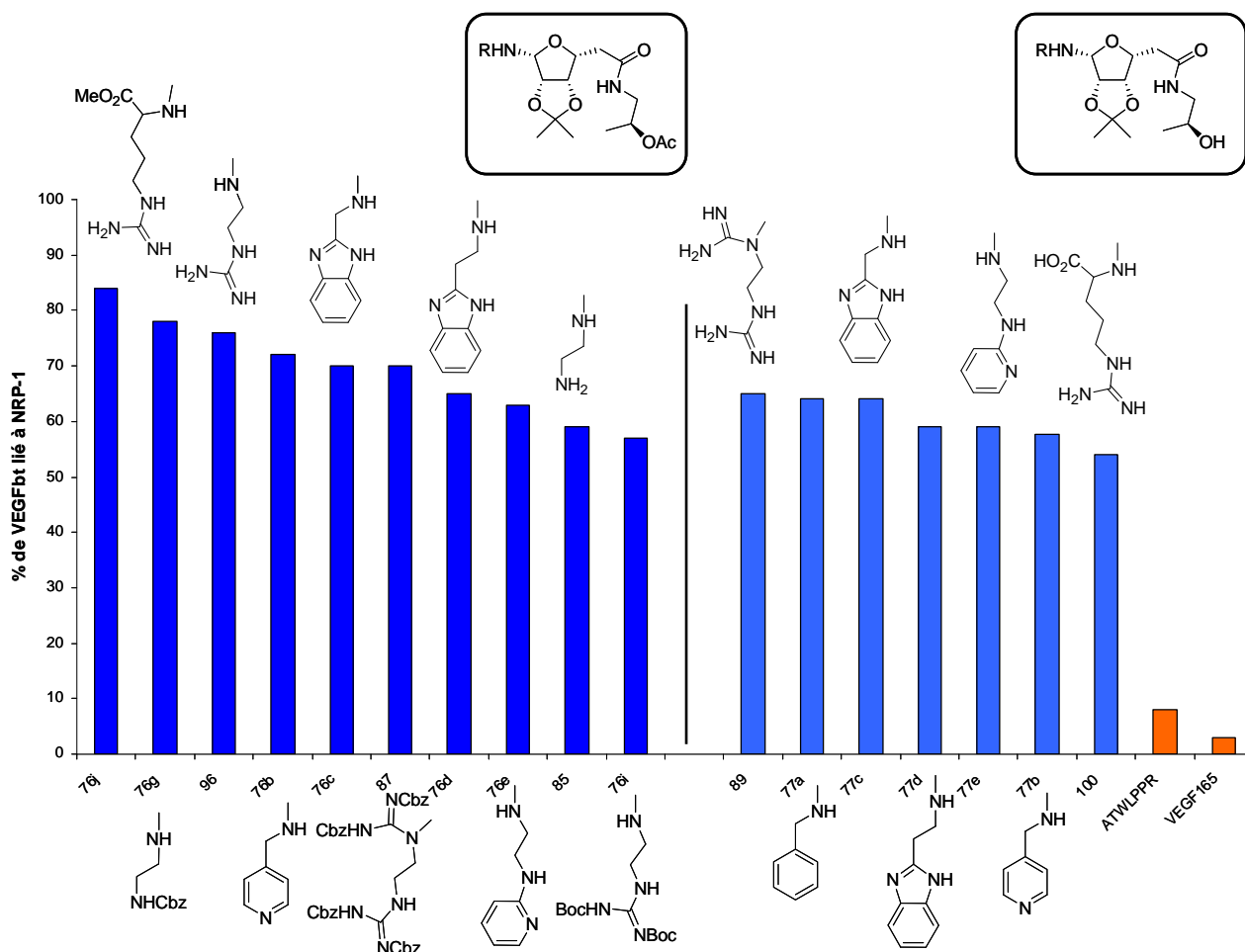
Figure 49. Classement de l'affinité des fonctions mimant l'arginine pour la série 2-acétoxy/2-hydro-propyl (selon le % de VEGFbt restant lié à NRP-1 pour 100 \mu M de composé)
