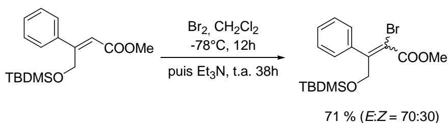
Schéma 47. Réaction de bromation au dibrome
