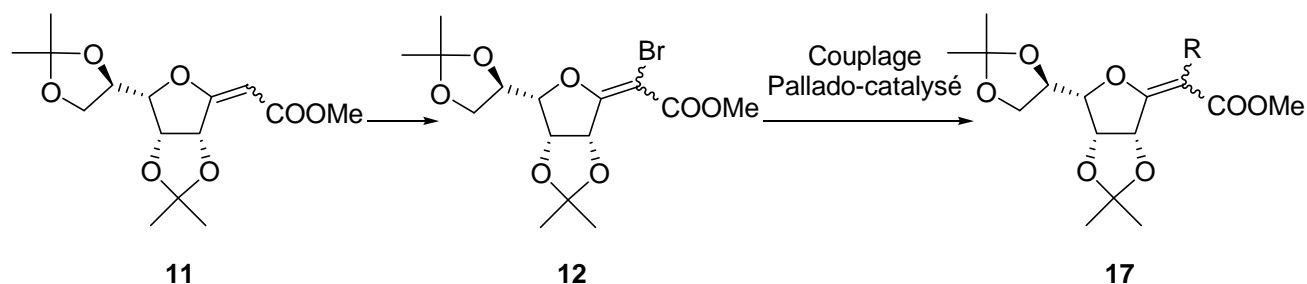
Schéma 46. Schéma général de synthèse
