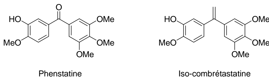
Figure 12. La phenstatine et l' iso -combretastatine
