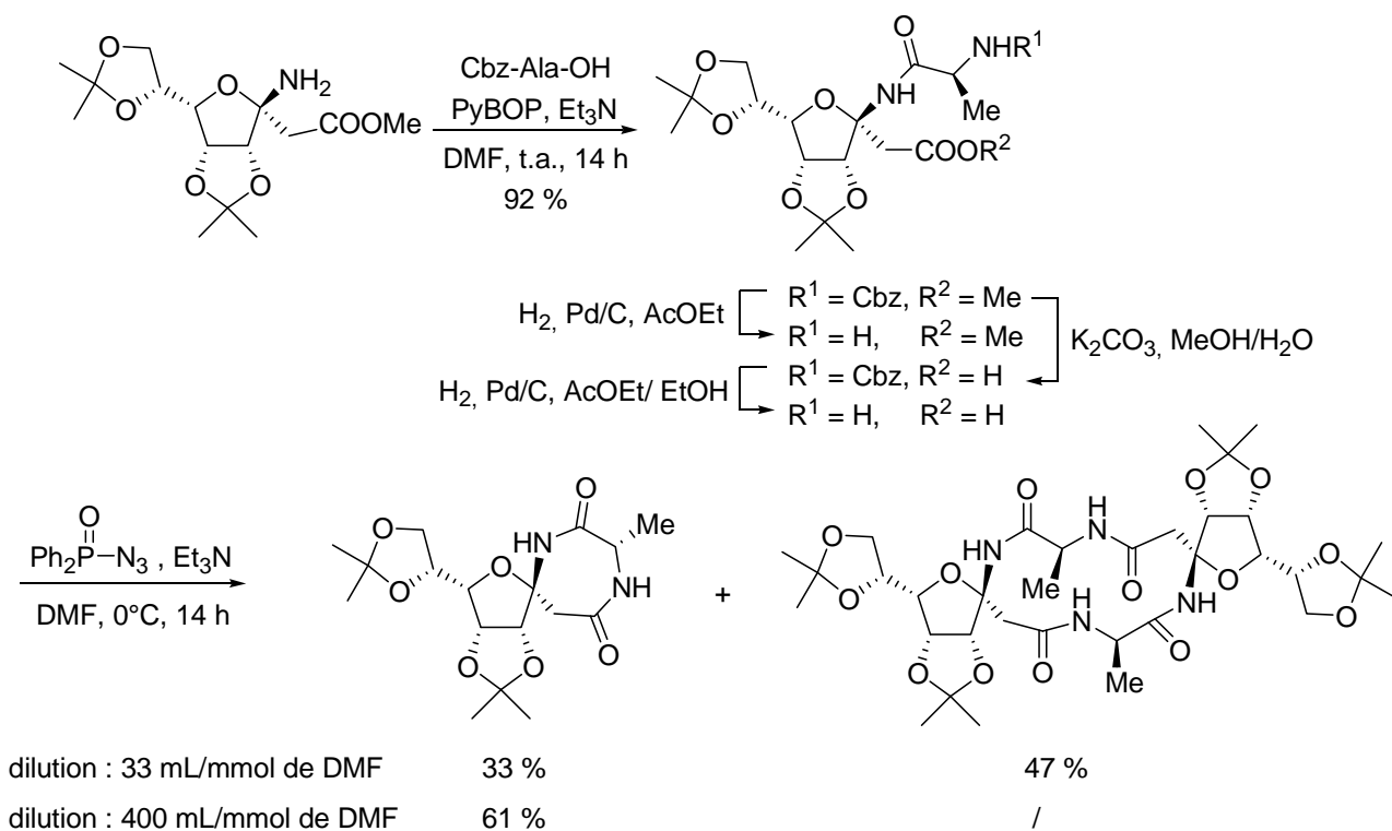
Schéma 26. Synthèse d'analogues de spironucléoside
