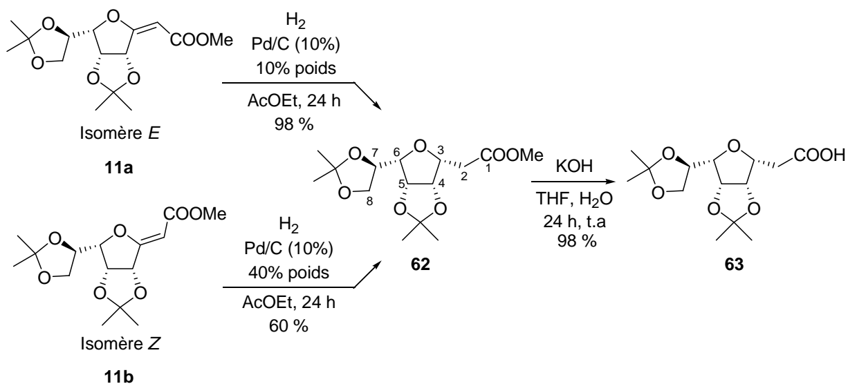
Schéma 88. Préparation de l'acide carboxylique 63
