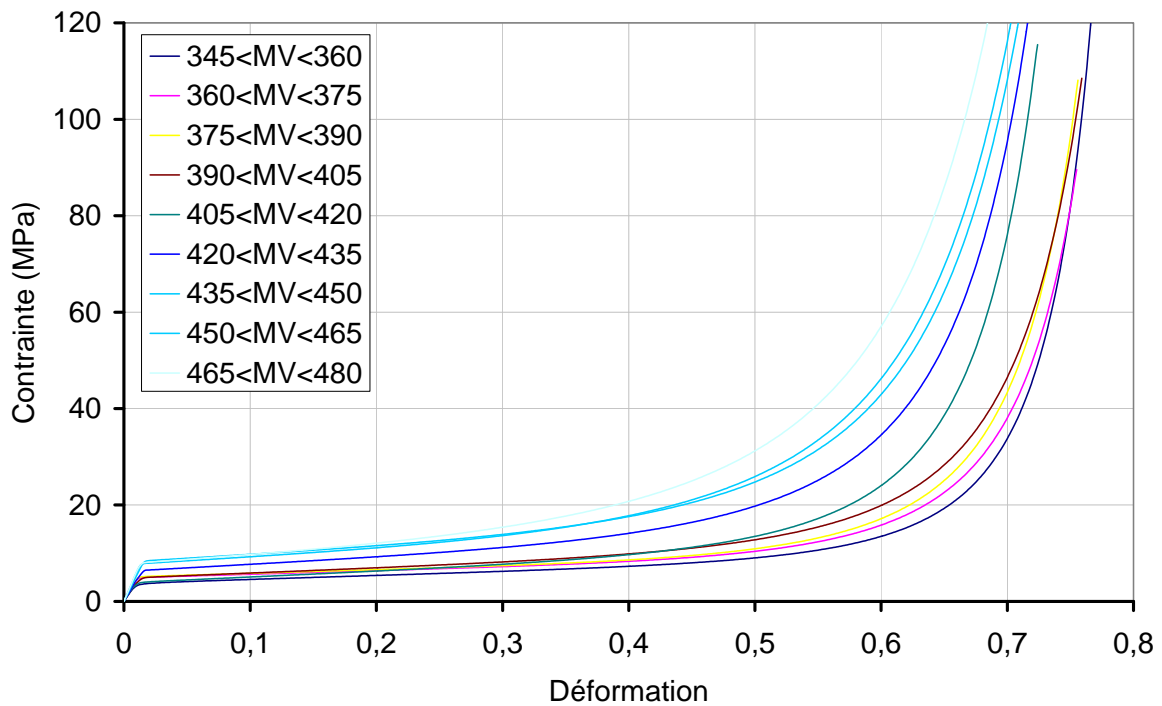
(b) Loi de comportement du bois d'Epicéa en compression radiale
