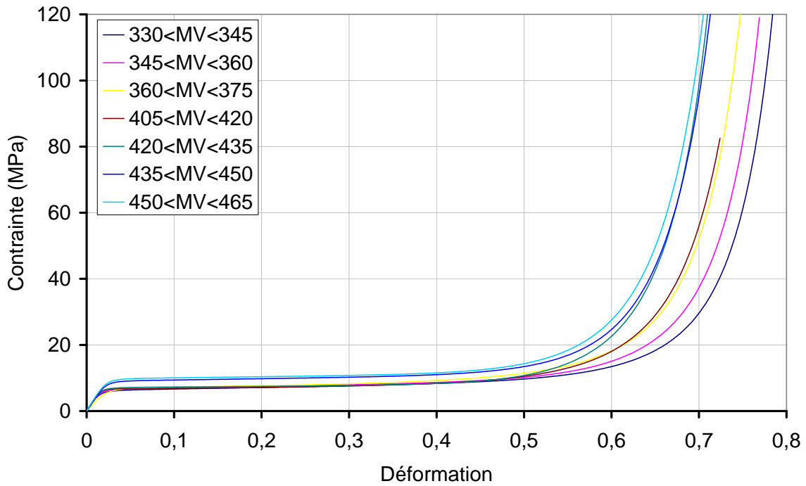
(a) Loi de comportement du bois d'Epicéa en compression tangentielle
