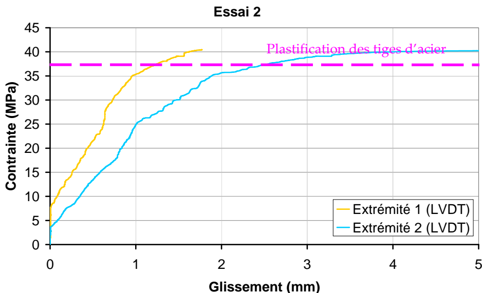
Figure 72 : Comparaison du comportement de l'éprouvette n°1 avant et après précontrainte avec un écart de temps de 14 mois
