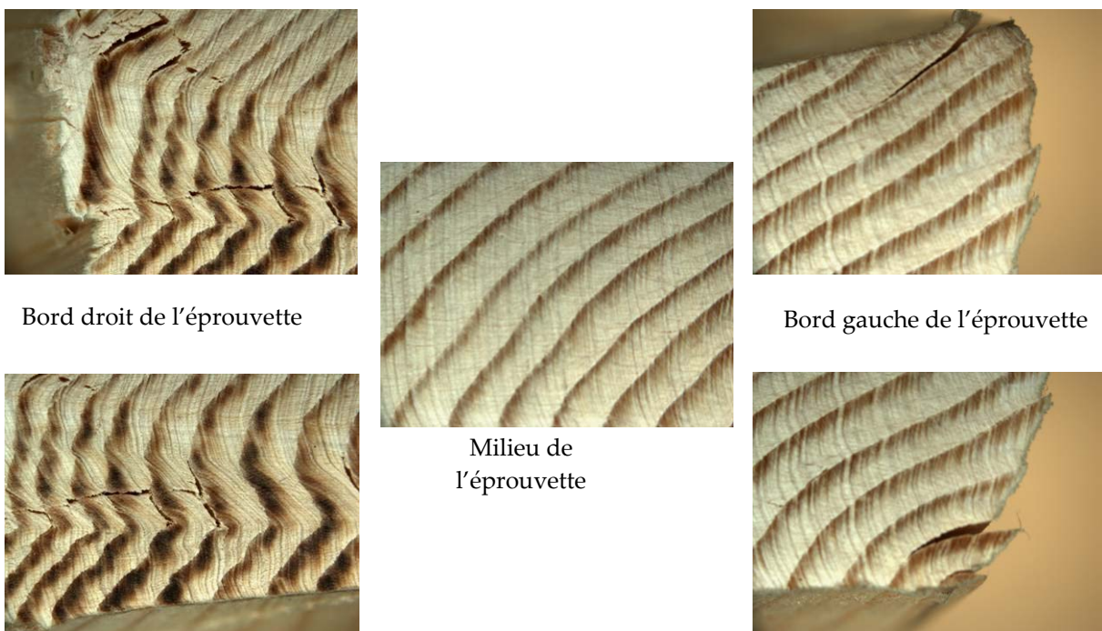
Figure 127 : Observations au stéréomicroscope Olympus SZW12 (zoom=×11,2) d'une éprouvette densifiée tangentiellement
