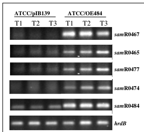
Figure 3 Analyses transcriptionnelles par RT-PCR de la souche mutant ATCC/OE484 et du control ATCC/pIB139, en culture MP5. L'expression de gènes de PKS samR0467 , 0465, 0477, 0474 a été testé. Le gène hrdB code pour le sigma facteur majeur en Streptomyces et il est utilisé comme control interne.
