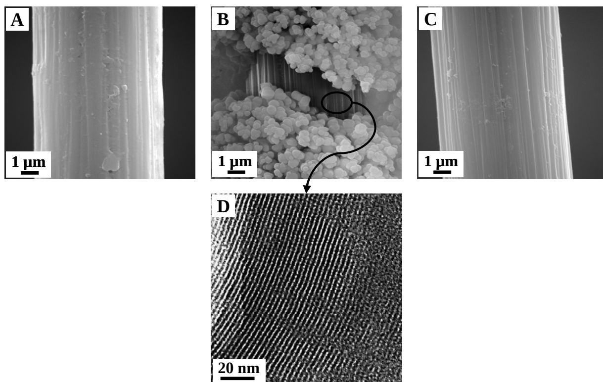
Figure 3.40 : (A-C) Photographies MEB obtenues sur une fibre de carbone nue (A), et sur des fibres de carbone modifiées par (B) un film de silice ordonnée électro-déposé à -2,2 V pendant 5 s à partir d'un sol n_{CTAB}/n_{TEOS} = 0,32 et (C) un film déposé par dip-coating avec un sol adapté. (D) Photographie MET correspondant à l'image (B) (film électro-déposé sur carbone à -2,2 V pendant 5 s).
