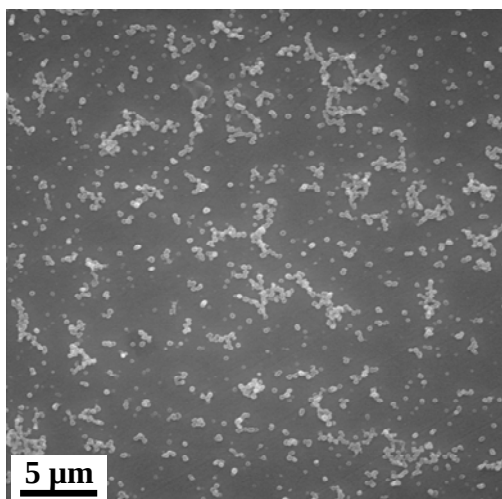
Figure 3.22 : Photographie MEB d'un film à base de silice ordonné électro-déposé sur cuivre à -1,3 V pendant 5 s à partir d'un sol n_{\text{CTAB}}/n_{\text{TEOS}} = 0,32 .
