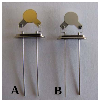
Figure A.12 : Photographies de cristaux de quartz (résonateurs pour microbalance) recouverts (A) d'or et (B) de platine.
