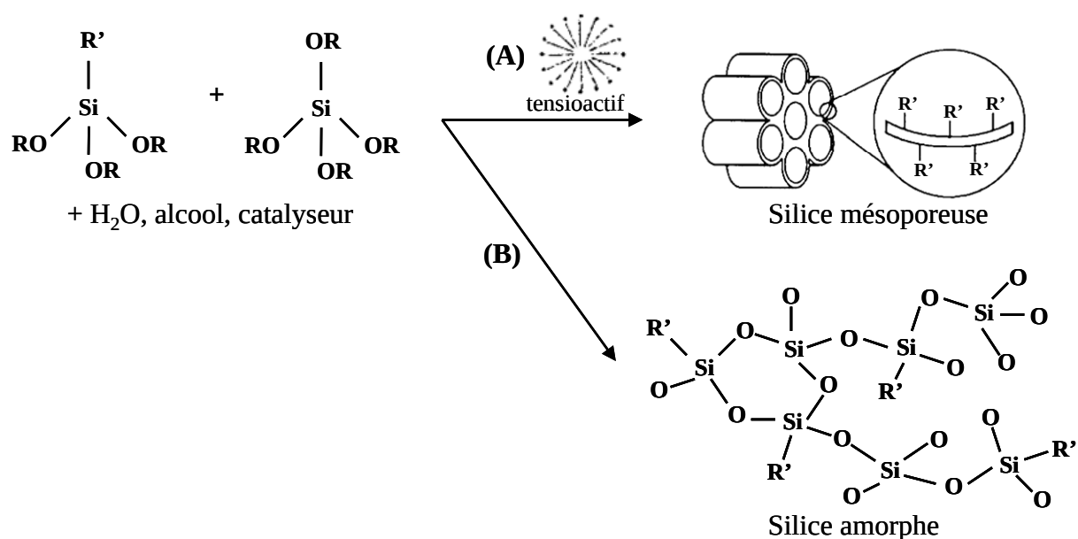
Figure 1.4 : Schématisation de la synthèse par (co)condensation (A) en présence de tensioactif et (B) en absence de tensioactif (d'après 58 ).
