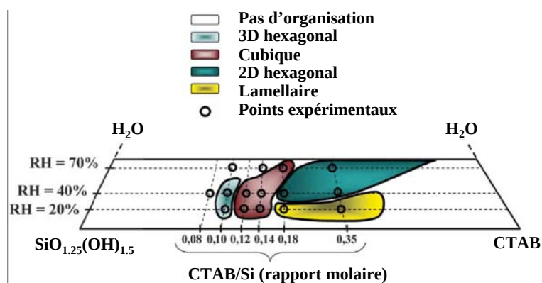
Figure 1.6 : Diagramme adapté pour l'EISA des textures de la phase MSS établit pour le système \text{CTAB/SiO}_{1,25}(\text{OH})_{1,5}/\text{EtOH}/\text{H}_2\text{O} (en %) (d'après 74 ).
