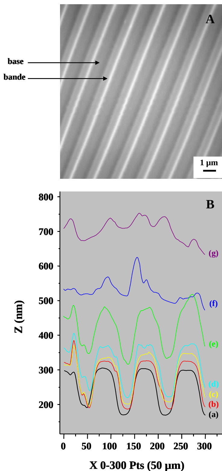
Figure 2.19 : (A) Photographie MEB d'une Au-CDtrode. B) Profils enregistrés par AFM in situ au cours du processus d'électro-dépôt d'un film fonctionnalisé par des groupements thiol (à partir d'un sol TEOS/MPTMS 90:10). Les différentes courbes correspondent au support d'or nu (a) et aux lignes AFM mesurées après 10 s (b), 40 s (c), 100 s (d), 125 s (e), 170 s (f) et 210 s (g).
