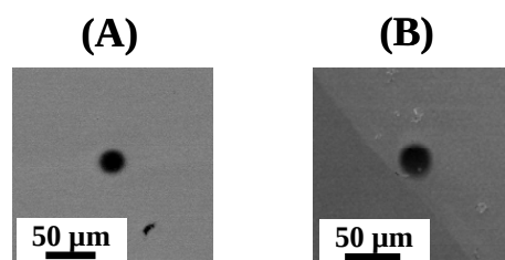
Figure 4.7 : Photographies FESEM de micro-dépôts obtenus avec une UME de platine (25 \mu\text{m} de diamètre) placée à (A) 5 \mu\text{m} et (B) 10 \mu\text{m} du substrat d'or à laquelle on a appliqué (A) -1,1 V pendant 3 s et (B) -0,9 V pendant 20 s dans un sol n_{\text{CTAB}}/n_{\text{TEOS}} = 0,32 .
