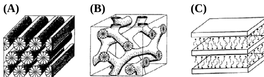
Figure 1.2 : Schématisation des différentes structures de silice mésoporeuses organisées : (A) hexagonale, (B) cubique et (C) lamellaire (d'après 42 ).
