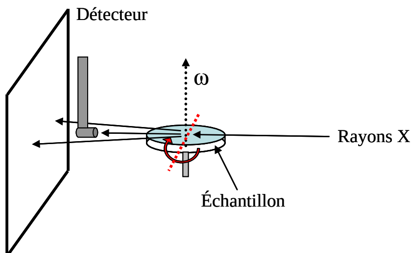
Figure A.16 : Illustration du montage de diffraction des rayons X en angle rasant.
