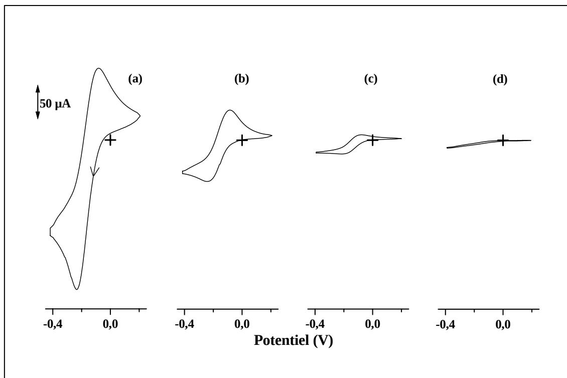
Figure 2.31 : Voltampérogrammes cycliques enregistrés dans \text{Ru}(\text{NH}_3)_6^{3+} 5mM (+ \text{NaNO}_3 0,1 M) au moyen (a) d'une électrode d'or nue et (b-d) d'électrodes d'or recouvertes de films de silice aminée électro-déposés à -1,2 V pendant 2 min à partir d'un sol contenant des quantités variables d'APTES : 10 % (b), 30 % (c) et 50 % (d). Vitesse de balayage : 5 \text{ mV s}^{-1} .
