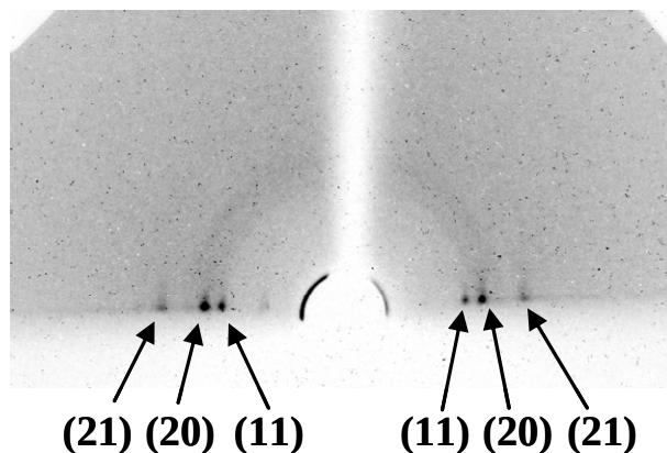
Figure 3.15 : Cliché de diffraction des rayons X obtenu sur un film électro-déposé à -1,3 V pendant 20 s sur ITO (les billes de silice ont été décollées à l'aide d'un adhésif) à partir d'un sol n_{\text{CTAB}}/n_{\text{TEOS}} = 0,32 .
