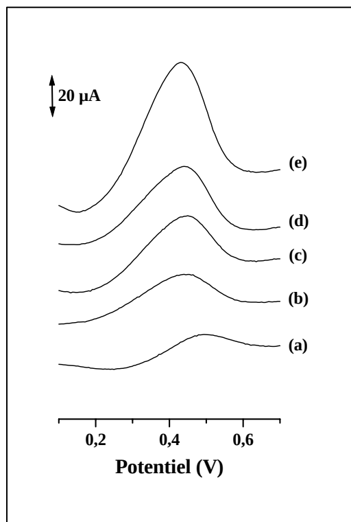
Figure 2.36 : Signaux de détection de \text{Cu}^{2+} obtenus pour différentes concentrations en cuivre dans le milieu d'accumulation. Le temps d'accumulation est de 6 minutes dans chaque cas et la déprotonation électrochimique de 3 minutes à -1,3 V. L'électrode d'or est modifiée par un film aminé électrogénéré à -1,2 V pendant 30 s dans un sol TEOS/APTES 90:10.
