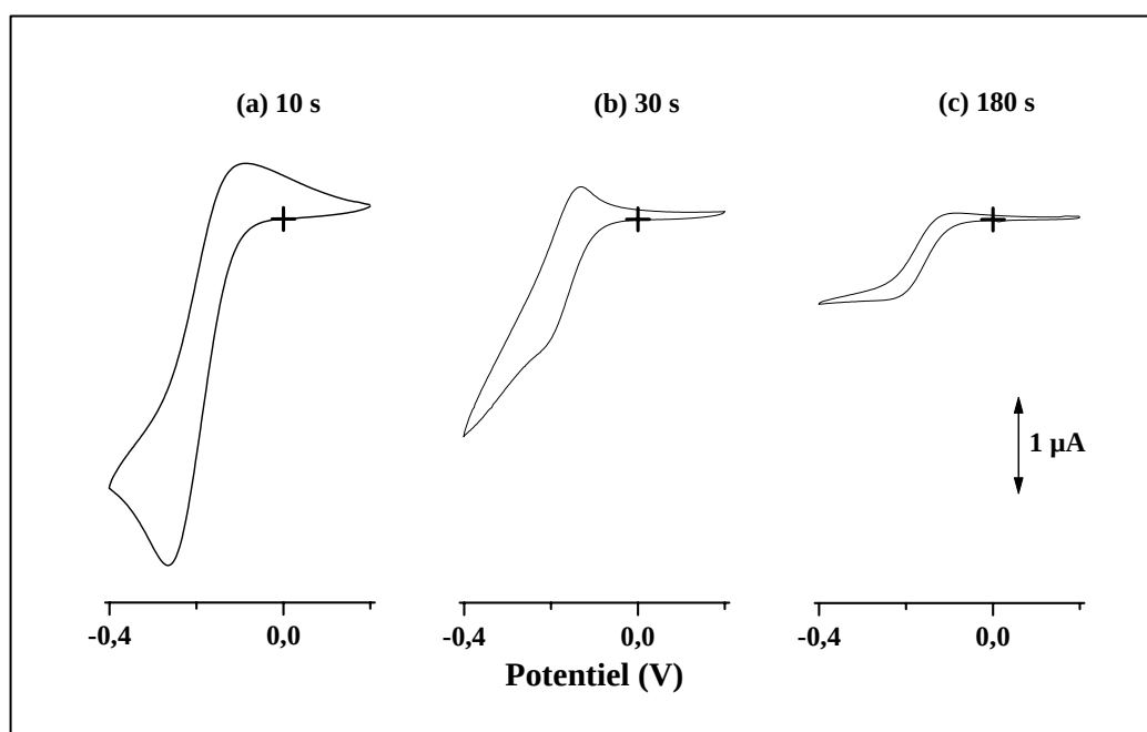
Figure 2.28 : Voltampérogrammes cycliques enregistrés dans \text{Ru}(\text{NH}_3)_6^{3+} 5 \times 10^{-3} \text{ M} (+ \text{NaNO}_3 0,1 \text{ M} ) au moyen d'électrodes d'or recouvertes de films de silice thiolée électro-déposés à -1,2 \text{ V} pendant des temps variables : (a) 10 s, (b) 30 s et (c) 180 s, en rotation, dans un sol TEOS/MPTMS 90:10. Vitesse de balayage : 20 \text{ mV s}^{-1} .
