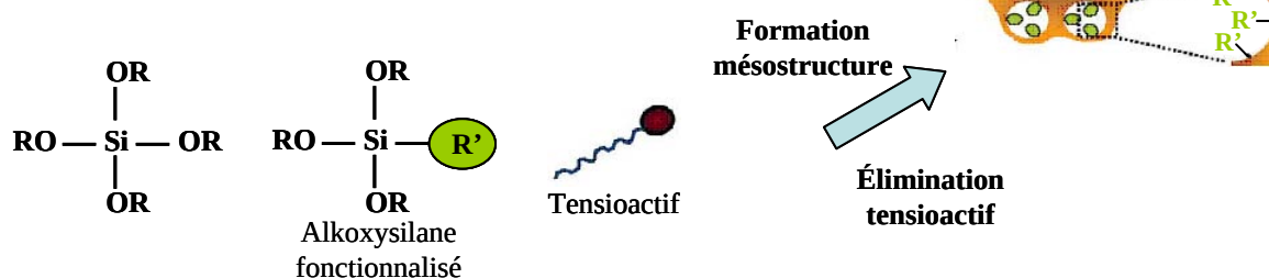
Figure 1.7 : Méthodes de (A) post-fonctionnalisation et (B) pré-fonctionnalisation pour la synthèse de matériaux hybrides mésoporeux.
