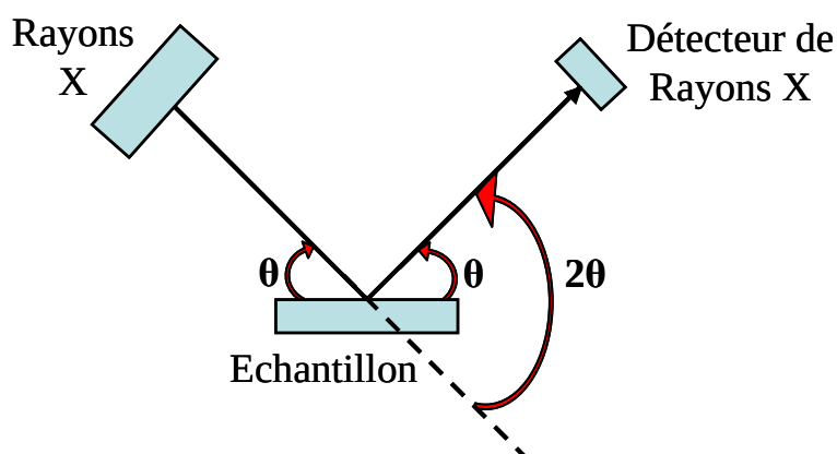
Figure A.15 : Illustrations du montage de Bragg de diffraction des rayons X et de la définition des angles.
