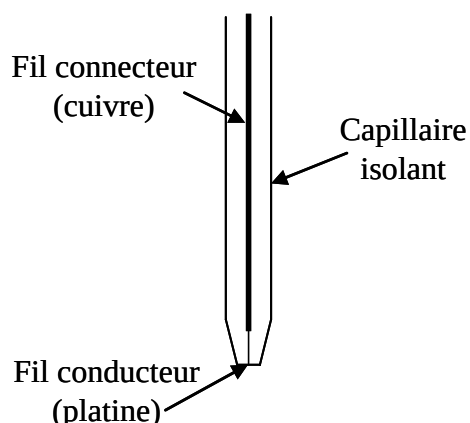
Figure A.6 : Schéma d'une ultramicroélectrode de platine disque-plan insérée dans un capillaire de verre.
