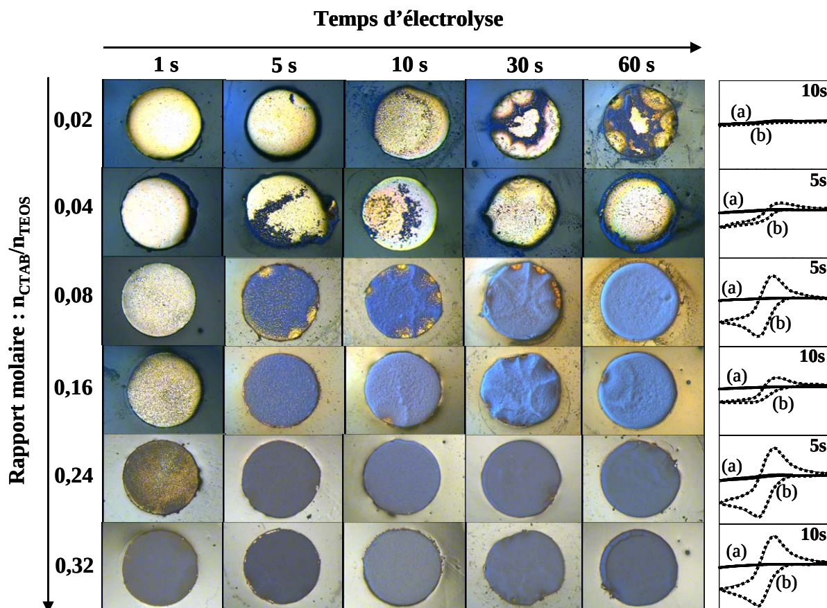
Figure 3.3 : Photographies de microscopie optique obtenues après électro-dépôt de films à base de silice en présence de CTAB en concentrations variables pendant un temps allant de 1 s à 60 s à -1,3 V ; y sont associés certains voltampérogrammes cycliques (correspondant à 5 s ou 10 s de dépôt) enregistrés dans Ru(NH_3)_6^{3+} 5 \times 10^{-3} M , avant (a, en traits pleins) et après (b, en pointillés) le traitement EtOH/HCl. Vitesse de balayage : 20 mV s^{-1} .
