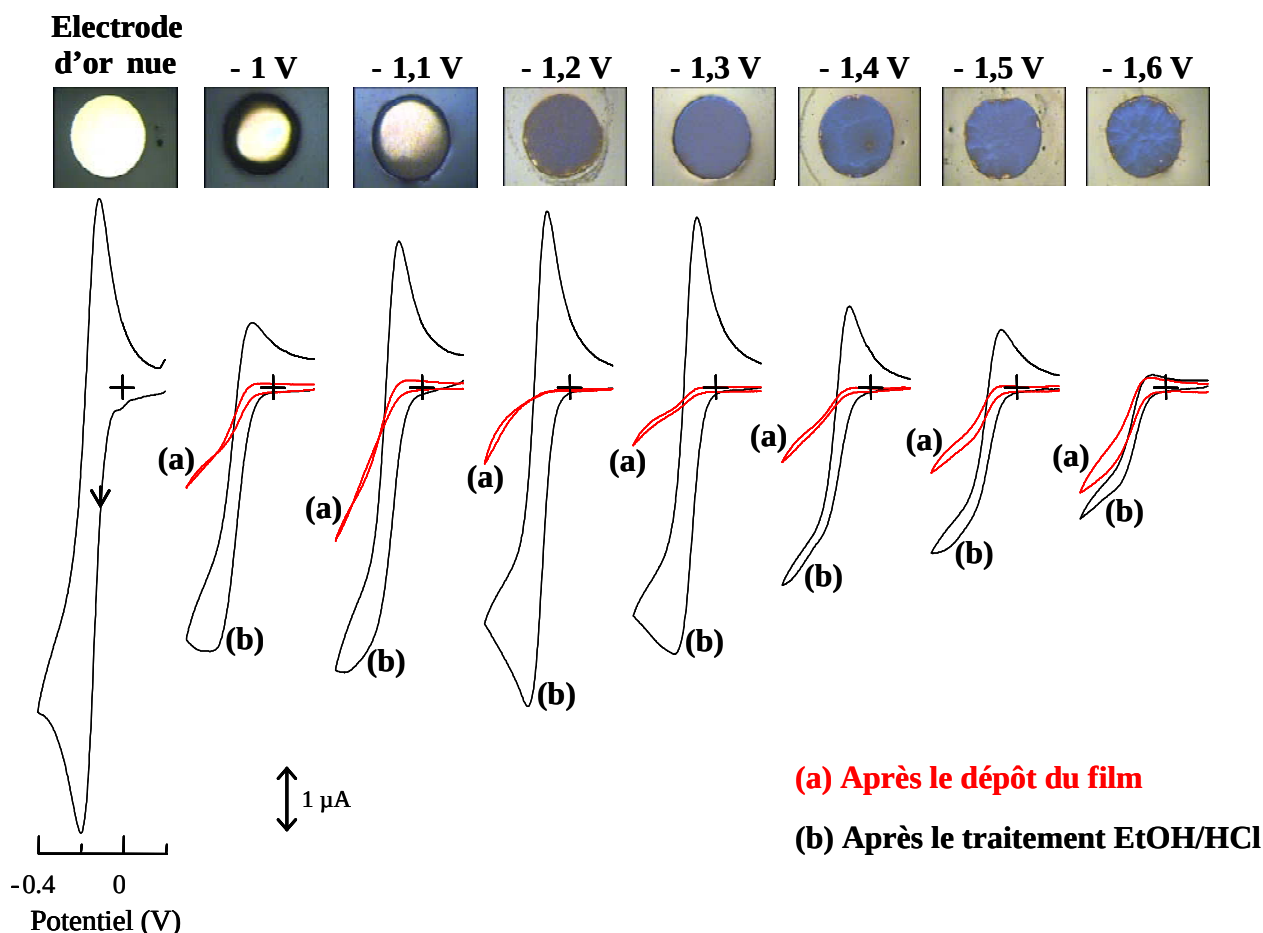
Figure 3.5 : Voltampérogrammes cycliques enregistrés dans \text{Ru}(\text{NH}_3)_6^{3+} 5 \times 10^{-3} \text{ M} au moyen d'une électrode d'or nue et d'électrodes recouvertes de films électro-déposés (à partir d'un sol n_{\text{CTAB}}/n_{\text{TEOS}} = 0,16 ) à différents potentiels pendant 5 s, avant (a) et après le traitement EtOH/HCl (b). Vitesse de balayage : 20 \text{ mV s}^{-1} .
