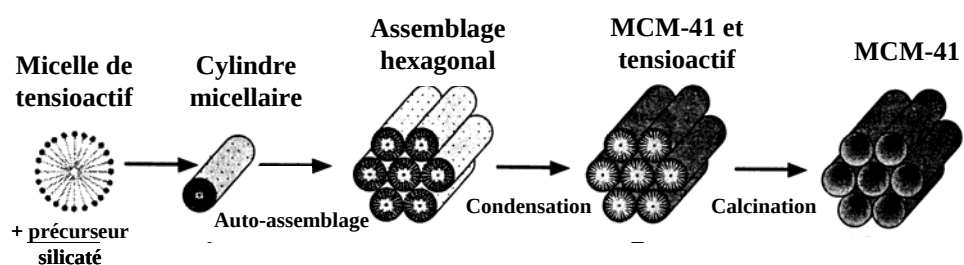
Figure 1.1 : Mécanisme simplifié de la synthèse de MCM-41 proposé par Kresge (d'après 42 ).
