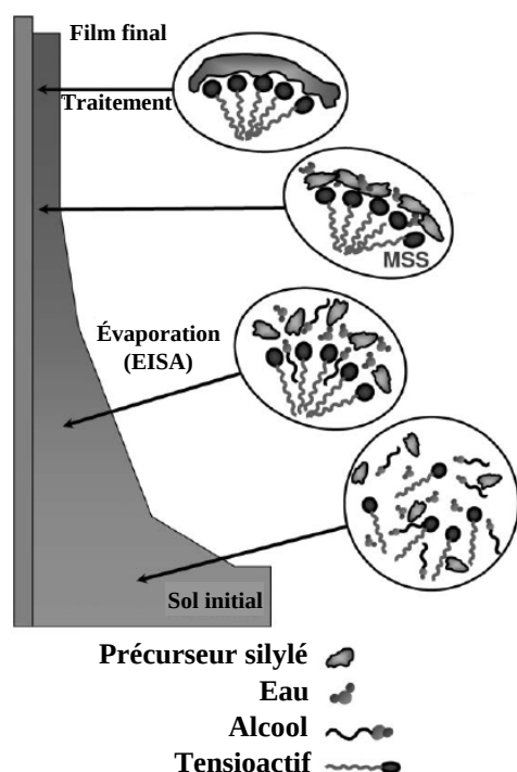
Figure 1.5 : Illustration des différentes étapes (EISA) menant à la formation d'un film de silice mésostructurée par dip-coating (d'après 69 ).
