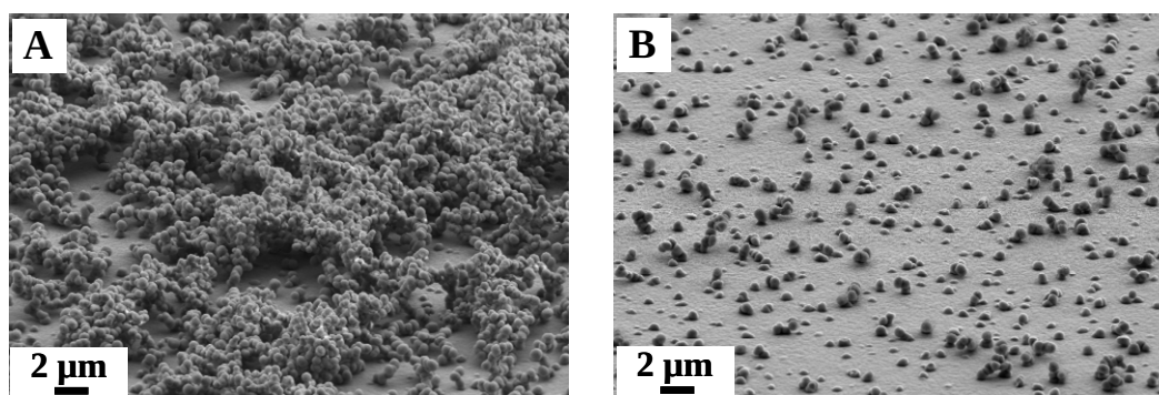
Figure 3.14 : Photographies de FESEM obtenues sur un film à base de silice ordonnée électro-déposé sur ITO à -1,3 V pendant 20 s à partir d'un sol n_{\text{CTAB}}/n_{\text{TEOS}} = 0,32 avant (A) et après (B) avoir retiré les billes de silice à l'aide d'un adhésif.
