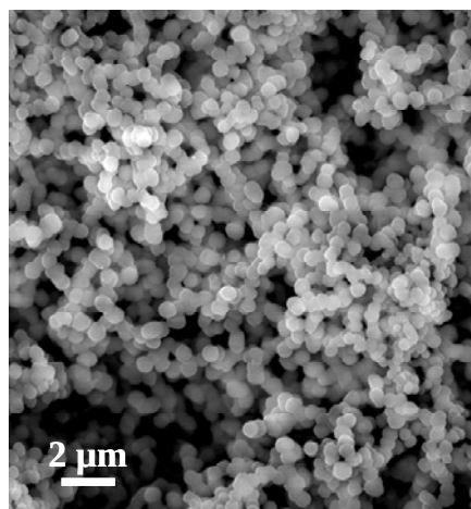
Figure 3.7 : Photographie MEB d'un film électrogénéré sur or à -1,3 V pendant 5 s à partir d'un sol n_{\text{CTAB}}/n_{\text{TEOS}} = 0,32 .
