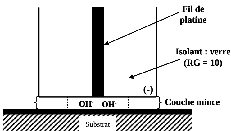
Figure 4.8 : Schématisation de l'ultramicroélectrode et du substrat séparés par une couche mince.
