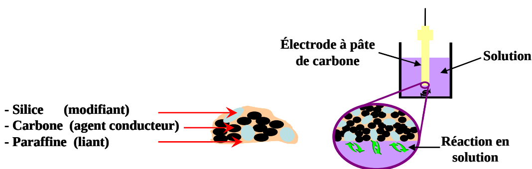
Figure 1.8 : Représentation d'une électrode à pâte de carbone.
