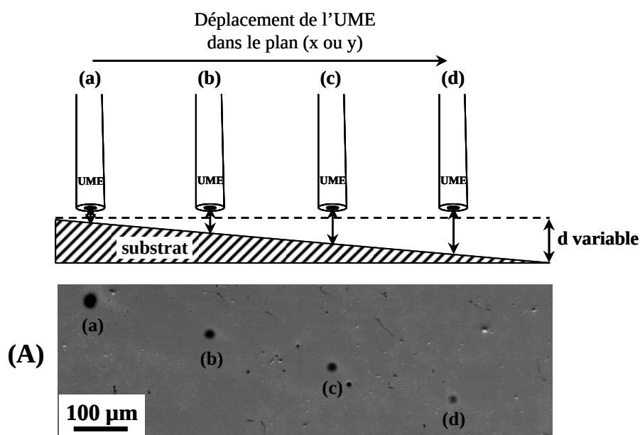
Figure 4.12 : Photographie FESEM d'une série de dépôts localisés (a-d) obtenus en appliquant, à une UME de platine (de 25 \mu\text{m} de diamètre) placée à 5 \mu\text{m} (pour le point a) du substrat d'or, un potentiel réducteur de (A) -0,9 V pendant 3 s dans un sol n_{\text{CTAB}}/n_{\text{TEOS}} = 0,32 .
