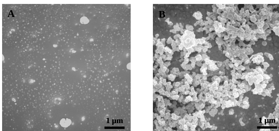
Figure 2.10 : Images obtenues en microscopie à balayage d'électrodes d'or recouvertes de films de silice fonctionnalisée par des groupements amine (A et B) préparés par électrogénération à -1,4 V pendant 10 s (A) et 120 s (B), en rotation, à partir d'un sol TEOS/APTES 90:10.
