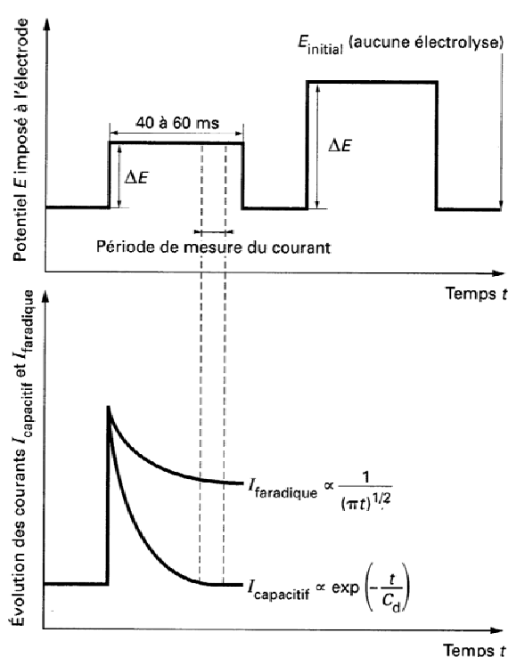
Figure A.8 : Schéma de principe de la voltampérométrie impulsionnelle : profil de potentiel appliqué à l'électrode et évolution des courant faradique et capacitif.
