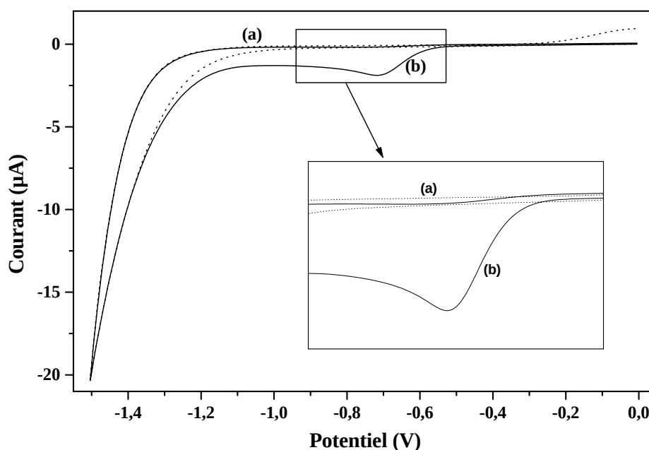
Figure 2.4 : Voltampérogrammes cycliques enregistrés dans (a) le « milieu neutre » composé de EtOH et \text{NaNO}_3 0,1 M (courbe pointillée) et (b) le même milieu après ajout de \text{HCl} 10^{-3} M (trait plein). Vitesse de balayage : 20 \text{ mV s}^{-1} .
