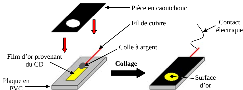
Figure A.1 : Schéma décrivant la préparation d'une Au-CDtrode.
