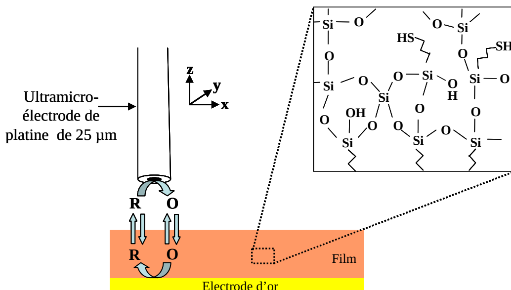
Figure 2.26 : Principe de caractérisation par SECM des films de silice thiolée électrogénérés.
