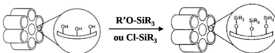
Figure 1.3 : Exemple de greffage post synthèse d'une MCM-41 (d'après 58 ).
