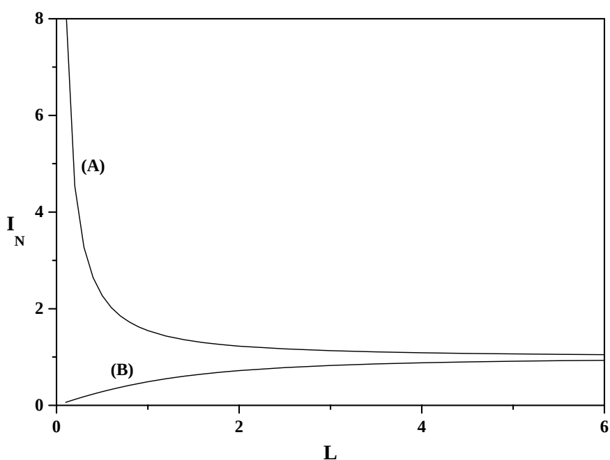
Figure 2.25 : Courbes d'approche théoriques des modes feedback (A) positif et (B) négatif pour RG = 10 .
