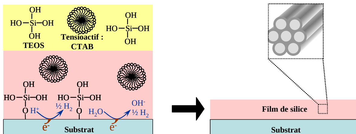
Figure 3.1 : Electrogénération d'un film à base de silice ordonnée.
