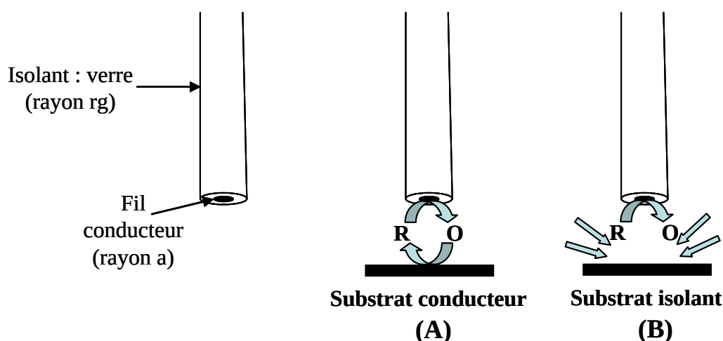
Figure 2.24 : Principe du mode feedback en microscopie électrochimique à balayage : (A) feedback positif et (B) feedback négatif.
