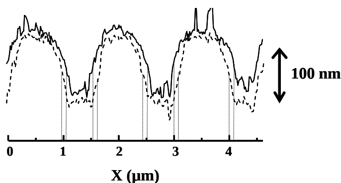
Figure 3.34 : Profils d’AFM mesurés perpendiculairement à l’électrode d’or avant (en pointillés) et après (en traits pleins) l’électro-dépôt d’un film mésoporeux à -1,3 V pendant 5 s à partir d’un sol où n_{\text{CTAB}}/n_{\text{TEOS}} = 0,32 .
