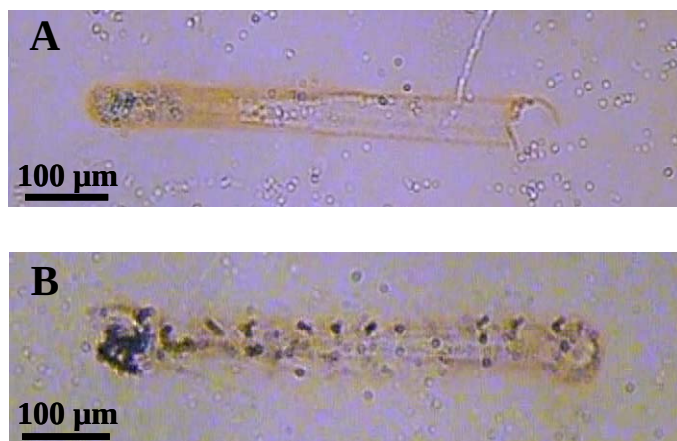
Figure 4.14 : Photographies de microscopie optique de lignes de silice obtenues en déplaçant une UME de platine (25 µm de diamètre) placée à 10 µm d'un substrat d'or et déplacée sur 500 µm à (A) 1 \mu\text{m s}^{-1} et (B) 20 \mu\text{m s}^{-1} tout en lui appliquant -1,1 V.
