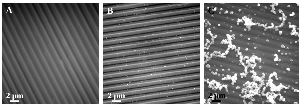
Figure 3.33 : Photographies MEB d'Au-CDtrodes nue (A) et recouvertes de films de silice mésoporeuse électro-déposés à -1,3 V pendant 5 s (B) et 10 s (C) à partir d'un sol n_{\text{CTAB}}/n_{\text{TEOS}} = 0,32 .
