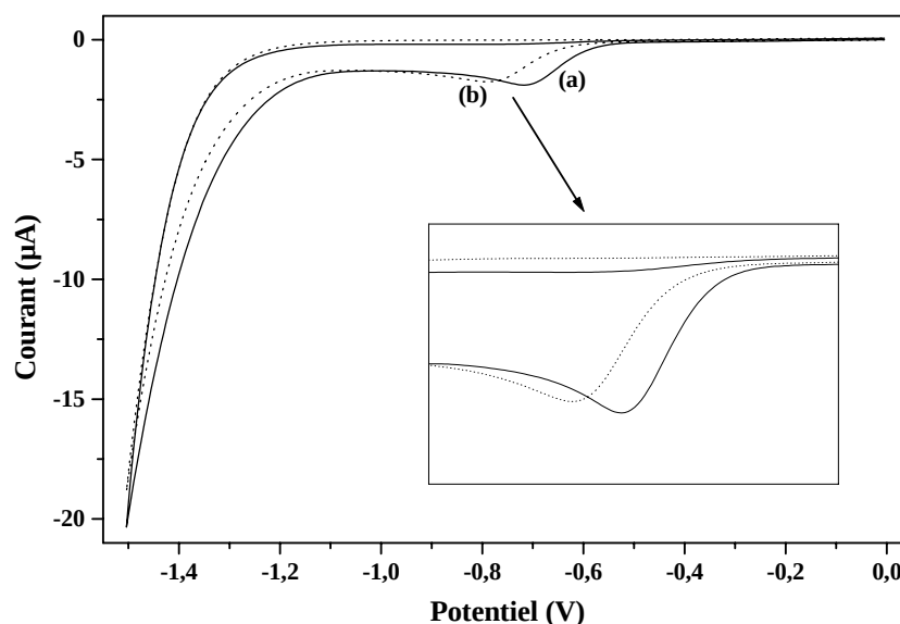
Figure 2.18 : Voltampérogrammes cycliques enregistrés sur une électrode d'or nue dans une solution contenant \text{HCl } 10^{-3} \text{ M} (dans \text{NaNO}_3 \text{ } 0,1 \text{ M} ) en absence (a) et en présence (b) de butylamine 1,5 \times 10^{-3} \text{ M} . Vitesse de balayage : 50 \text{ mV s}^{-1} .
