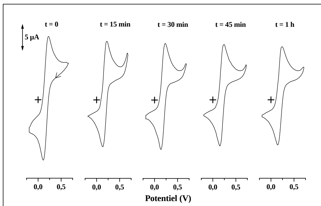
Figure 2.5 : Voltampérogrammes cycliques enregistrés après différentes périodes de séjour d'une électrode d'or dans un milieu contenant \text{Fe}(\text{CN})_6^{3-} 10^{-3} M et TEOS/MPTMS 90:10 à pH 3. Vitesse de balayage : 5 \text{ mV s}^{-1} .
