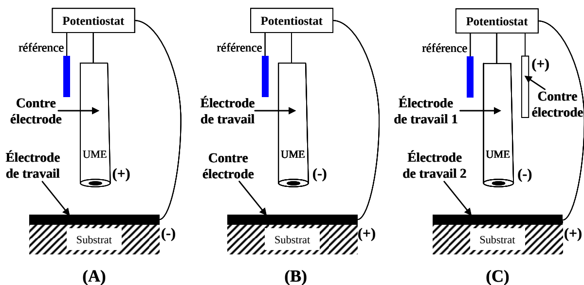
Figure 4.3 : Montages expérimentaux envisagés pour réaliser des électro-dépôts localisés de silice : (A) l'UME est utilisée en contre-électrode et le substrat en électrode de travail ; (B) l'UME est utilisée en électrode de travail et le substrat en contre-électrode ; (C) l'UME est utilisée en électrode de travail 1, le substrat en électrode de travail 2 et la contre-électrode est dans le milieu. Une quasi-référence est placée dans le milieu.
