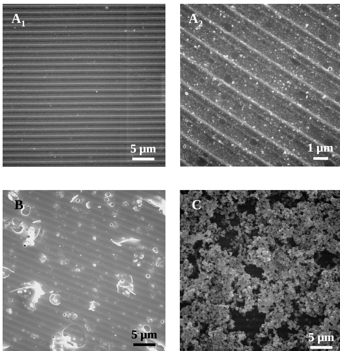
Figure 2.32 : Photographies MEB des surfaces d'or Au-CDtrodes recouvertes de films de silice aminée électro-déposés à -1,2 V pendant des temps variables : 10 s (A), 30 s (B) et 2 min (C) à partir d'un sol TEOS/APTES 90:10 (A 2 est un zoom de A 1 ).
