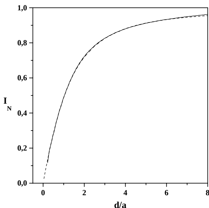
Figure 4.2 : Courbe d'approche SECM (en traits pleins) enregistrée à 0,1 \mu\text{m s}^{-1} et obtenue grâce à une ultramicroélectrode de platine de 25 \mu\text{m} de diamètre sur le substrat d'or dans un sol n_{\text{CTAB}}/n_{\text{TEOS}} = 0,32 . Le potentiel appliqué à l'UME est de -0,5 V. La courbe théorique du mode feedback négatif, pour \text{RG} = 10 , y est superposée (en pointillés).
