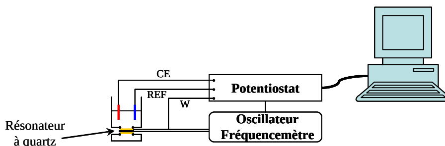
Figure A.11 : Schéma d'un montage de microbalance à cristal de quartz électrochimique.
