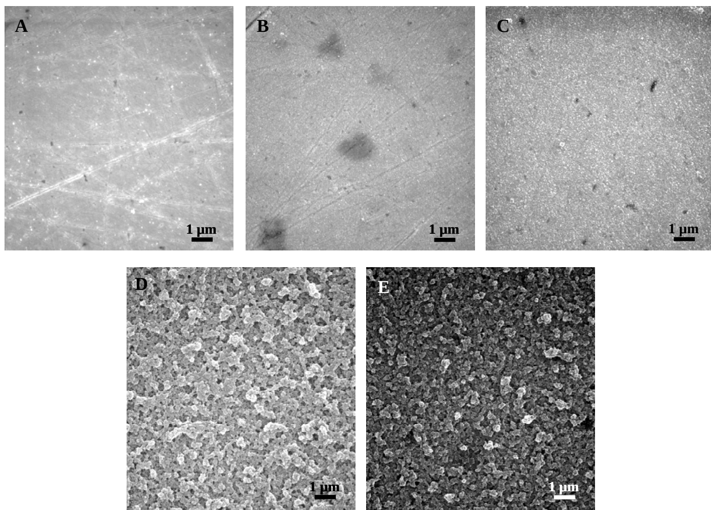
Figure 2.9 : Images obtenues en microscopie à balayage d'une électrode d'or nue (A) ou d'électrodes d'or recouvertes de films de silice fonctionnalisée par des groupements thiol (B-E) préparés par électrogénération à -1,2 V pendant 10 s (B), 20 s (C), 30 s (D) et 60 s (E), en rotation, à partir d'un sol TEOS/MPTMS 90:10.
