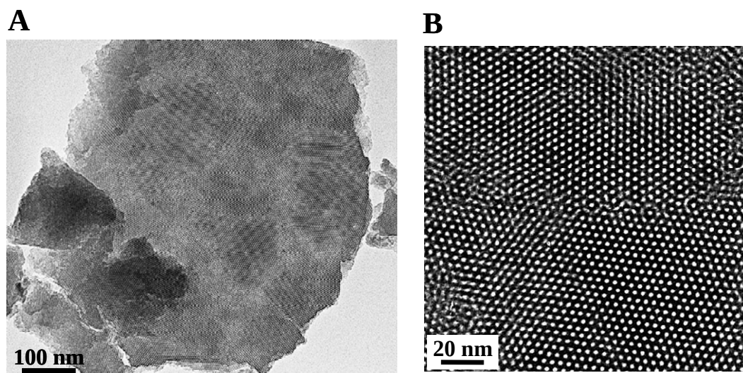
Figure 3.13 : Photographies MET d'un film électro-déposé sur ITO à -1,3 V pendant 10 s à partir d'un sol n_{\text{CTAB}}/n_{\text{TEOS}} = 0,32 . La photographie A est vue large et B est un grossissement du même film.
