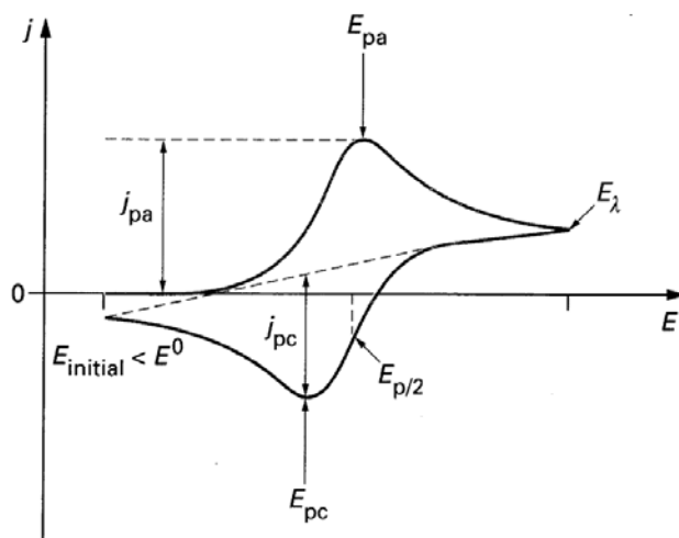
Figure A.7 : Voltampérogramme cyclique entre E_i et E_\lambda d'un système rapide.
