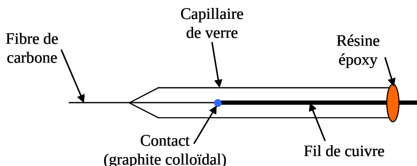
Figure A.5 : Schéma d'une ultramicroélectrode cylindrique constituée d'une fibre de carbone.
