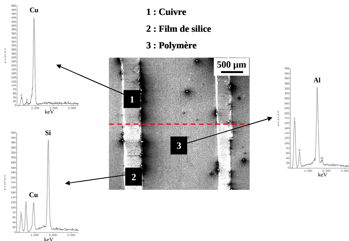
Figure 3.38 : Photographie MEB d'un circuit imprimé sur lequel on a réalisé un électro-dépôt à -1,3 V pendant 5 s dans un sol n_{\text{CTAB}}/n_{\text{TEOS}} = 0,32 . Le trait en pointillé représente la limite de la solution. Les spectres EDX obtenus sur les trois zones différentes sont associés à la photographie.
