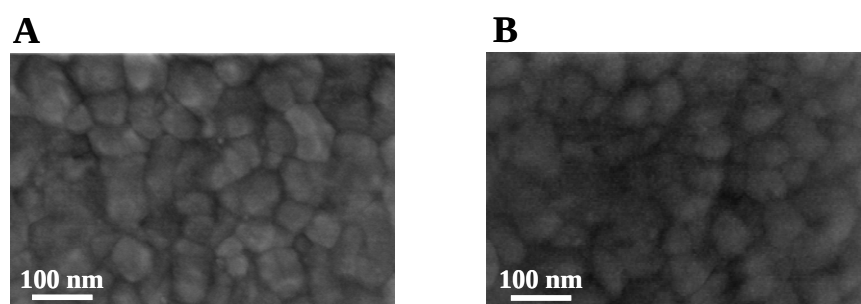
Figure 4.11 : Photographie FESEM de la texture (A) du substrat d'or et (B) du micro-dépôt obtenu avec une UME de platine (25 \mu\text{m} de diamètre) placée à 10 \mu\text{m} du substrat d'or, à laquelle on a appliqué -1,1 V pendant 10 s dans un sol n_{\text{CTAB}}/n_{\text{TEOS}} = 0,32 .
