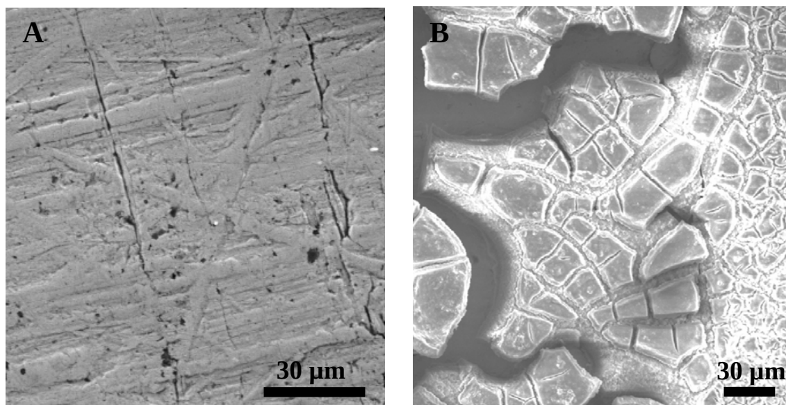
Figure 2.2 : Photographies MEB de la surface d'or modifiée par un film à base de silice électro-déposé avec (A) et sans (B) formation préalable d'une monocouche auto-assemblée de MPTMS (photographies MEB obtenues par Stéphanie Sayen 7 ).
