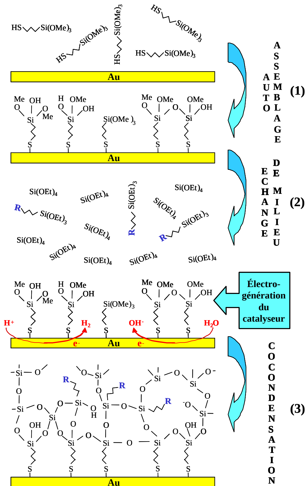
Figure 2.1 : Schéma de principe de la génération électro-assistée d'un film de silice fonctionnalisée par un groupement organique R (R = -\text{NH}_2 ou -\text{SH} ).
