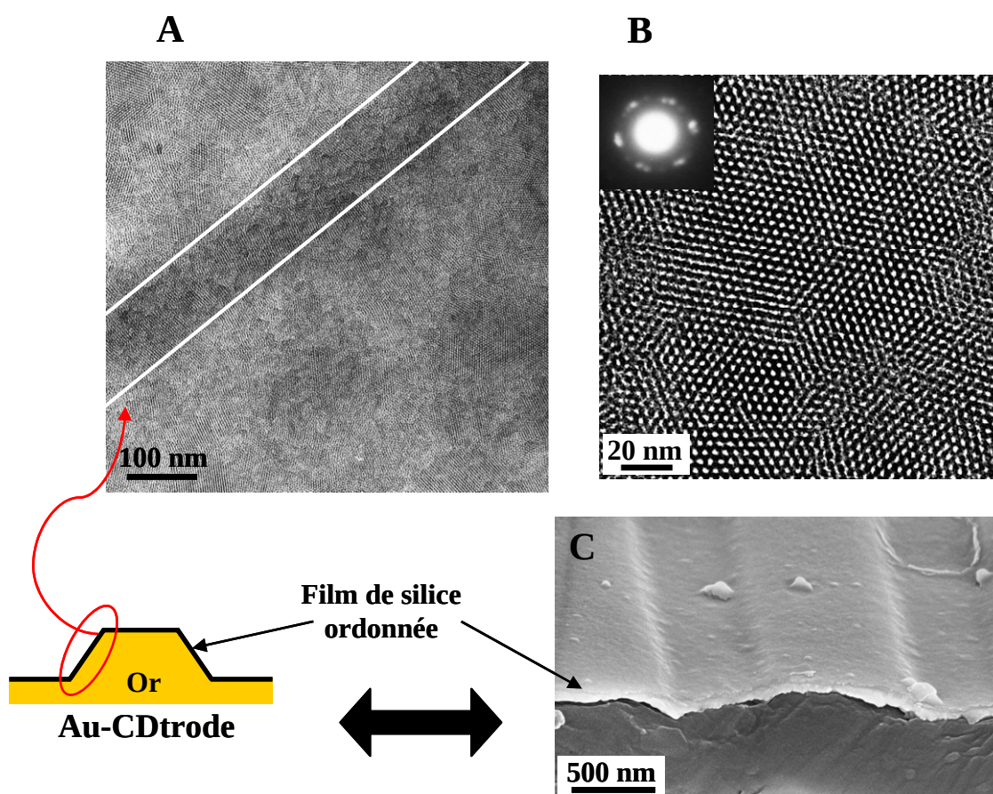
Figure 3.36 : (A-B) Photographies MET d'un film de silice ordonnée électro-déposé sur une Au-CDtrode à -1,3 V pendant 10 s à partir d'un sol n_{CTAB}/n_{TEOS} = 0,32 . L'image A représente une vue large et l'image B une vue zoomée avec en insertion le cliché de diffraction des électrons correspondant. L'image C est une vue transversale de FESEM de l'Au-CDtrode recouverte du film ordonné.
