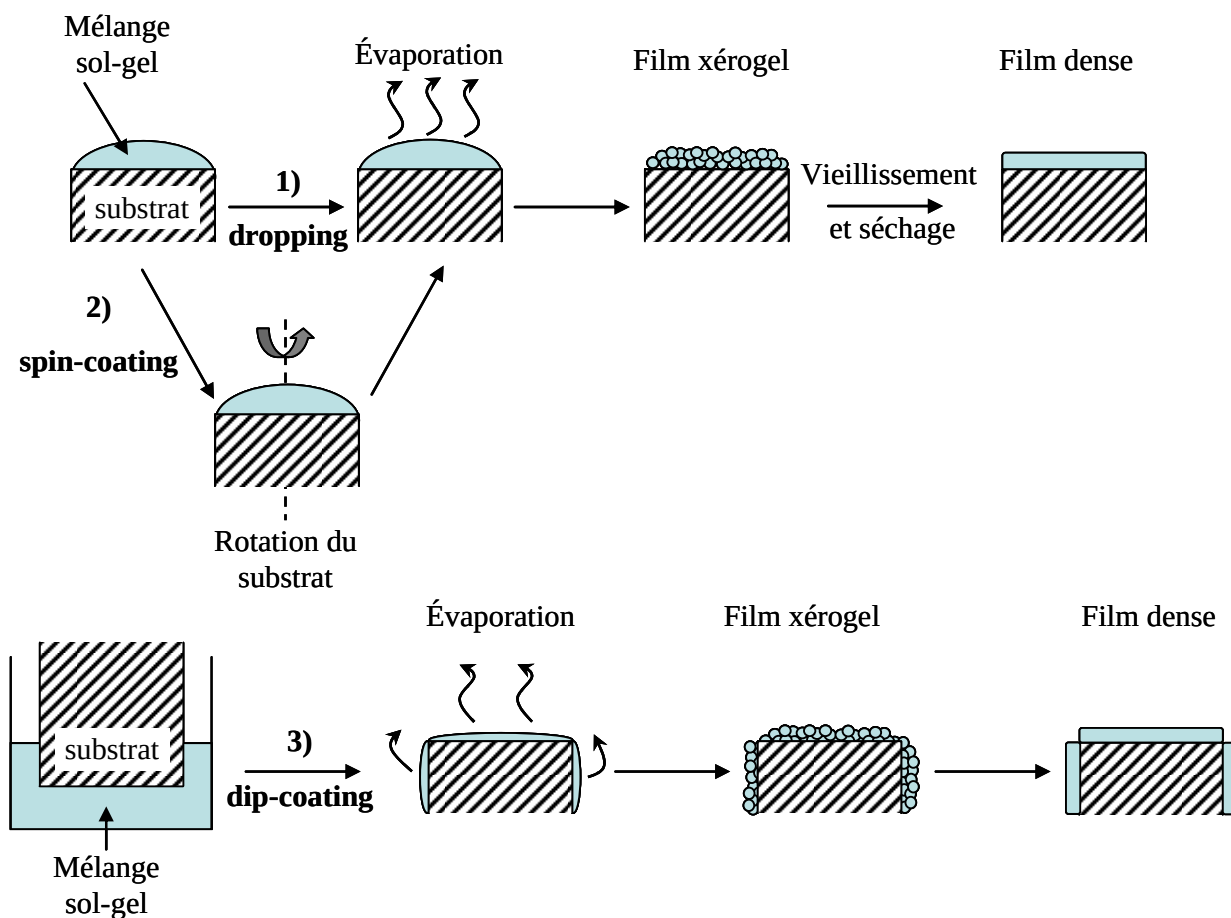
Figure 1.9 : Représentation des différents mode de dépôt de films sol-gel : 1) dropping, 2) spin-coating et 3) dip-coating.
