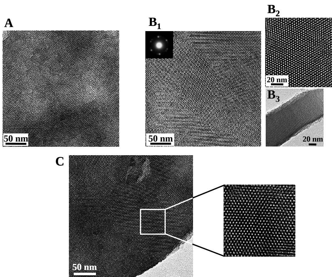
Figure 3 17 : Photographies MET (A) d'un film à base de silice ordonnée électro-déposés sur or préalablement modifié par une monocouche auto-assemblée de MPTMS, et de films à base de silice ordonnée fonctionnalisée par (B 1-3 ) 10 % d'APTES sur carbone et (C) 5 % de MPTMS sur or. Les films sont formés à (A) à -1,3 V pendant 10 s à partir d'un sol n_{\text{CTAB}}/n_{\text{TEOS}} = 0,32 , (B 1-3 ) à -2,2 V pendant 10 s à partir d'un sol n_{\text{CTAB}}/n_{\text{silice}} = 0,32 et TEOS/APTES 90:10, et (C) à -1,3 V pendant 5 s à partir d'un sol n_{\text{CTAB}}/n_{\text{silice}} = 0,32 et TEOS/MPTMS 95:5. Les images A, B 1 , B 2 et C représentent des vues du dessus et l'image B 3 une vue transversale.
