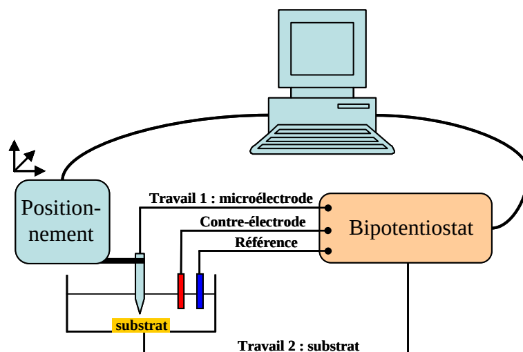
Figure A.14 : Schéma de principe du microscope électrochimique à balayage.
