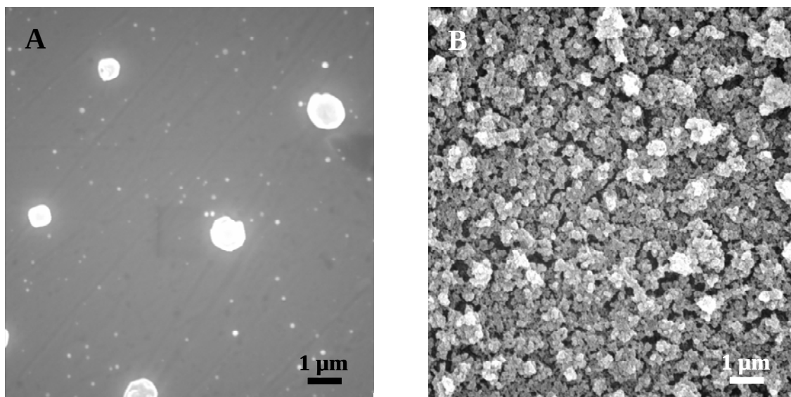
Figure 2.17 : Photographies MEB d'électrodes d'or recouvertes de films de silice fonctionnalisée par des groupements amine (A) et par des groupements thiol (B) électro-déposés dans les mêmes conditions (à -1,2 V pendant 2 minutes), en rotation, à partir de solutions 90:10 TEOS/APTES et TEOS/MPTMS respectivement.
