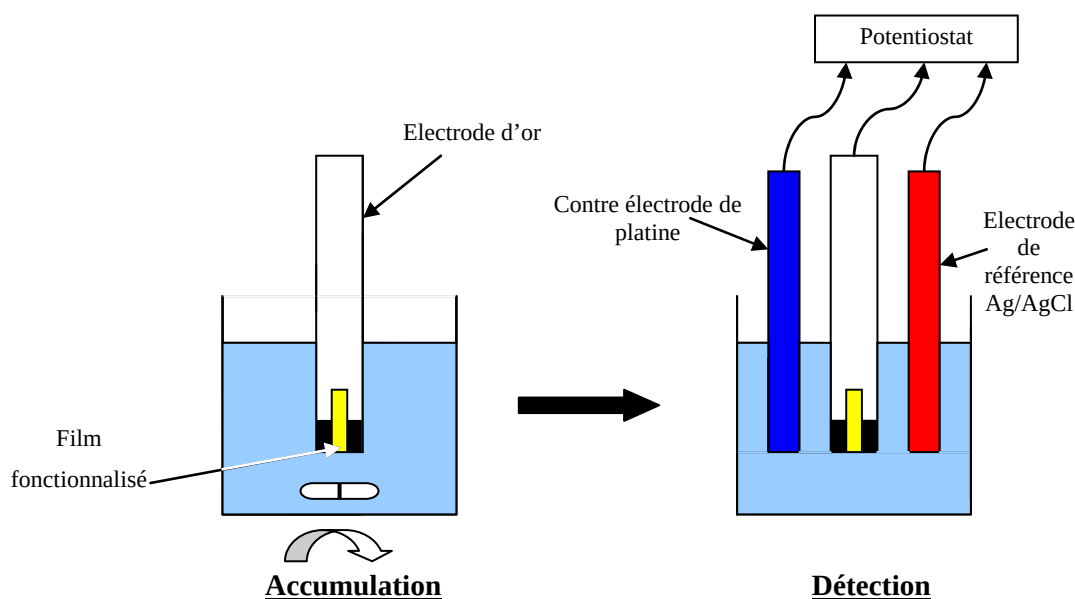
Figure 2.33 : Schéma de principe de la méthode d'accumulation - détection pour l'électrode d'or modifiée par les groupements amine. Le milieu d'accumulation est composé de \text{Cu}^{2+} en concentration précise dans EtOH. Le milieu de détection est composé de \text{HNO}_3 0,1 M, \text{NaNO}_3 0,1 M dans EtOH.
