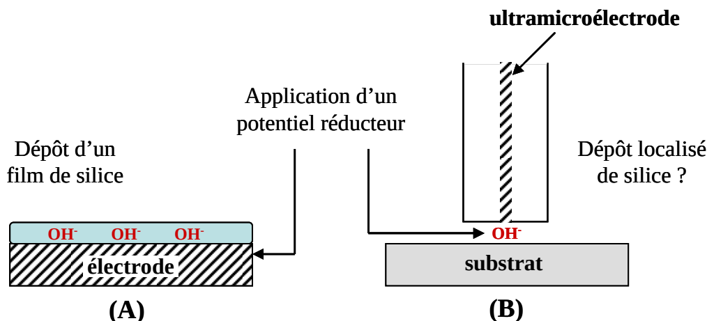
Figure 4.1 : Schéma décrivant le principe d'électro-dépôt d'un film de silice sur une électrode de taille conventionnelle (A) et à partir d'une ultramicroélectrode sur un substrat (B).
