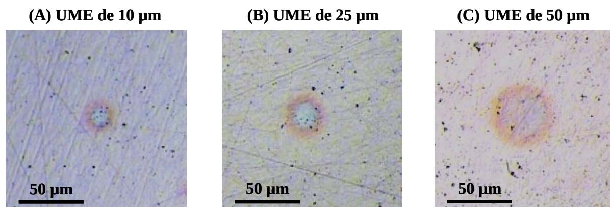
Figure 4.13 : Photographies de microscopie optique de dépôts localisés obtenus en appliquant un potentiel réducteur de -1,2 V pendant 60 s dans un sol n_{\text{CTAB}}/n_{\text{TEOS}} = 0,32 , à des UMEs de platine de diamètres différents : (A) 10 µm, (B) 25 µm et (C) 50 µm, placées, respectivement, à (A) 10 µm, (B) 30 µm et (C) 40 µm du substrat d'or.
