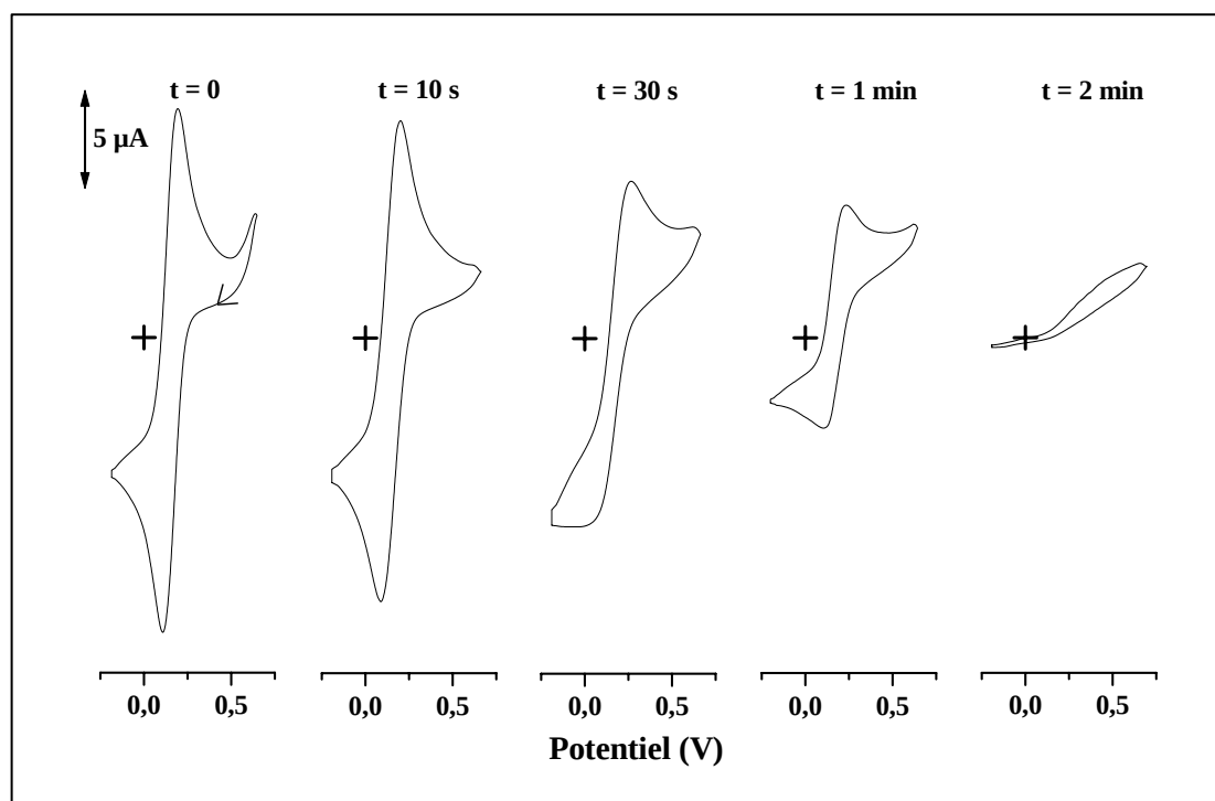
Figure 2.6 : Voltampérogrammes cycliques, enregistrés après différents temps (10 s, 30 s, 1 min et 2 min) d'électrolyse à -1,2 V appliqués à l'électrode d'or dans un milieu contenant \text{Fe}(\text{CN})_6^{3-} 10^{-3} M et TEOS/MPTMS 90:10 à pH 3. Vitesse de balayage : 5 \text{ mV s}^{-1} .
