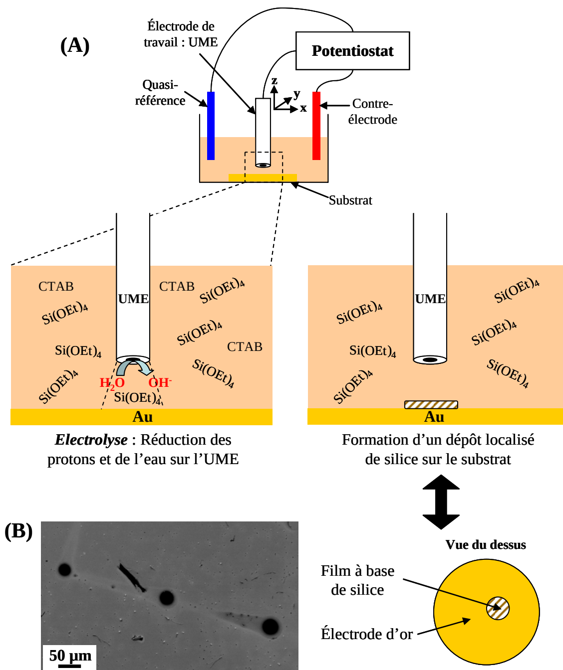
Figure 4.5 : (A) Schéma de principe de l'électro-dépôt localisé de films à base de silice par le mode feedback de la SECM. (B) Photographie FESEM d'une série de dépôts localisés obtenus en appliquant à une UME de platine (de 25 \mu\text{m} de diamètre), placée à 5 \mu\text{m} d'un substrat d'or, un potentiel réducteur de -0,9 V pendant 3 s dans un sol n_{\text{CTAB}}/n_{\text{TEOS}} = 0,32 .
