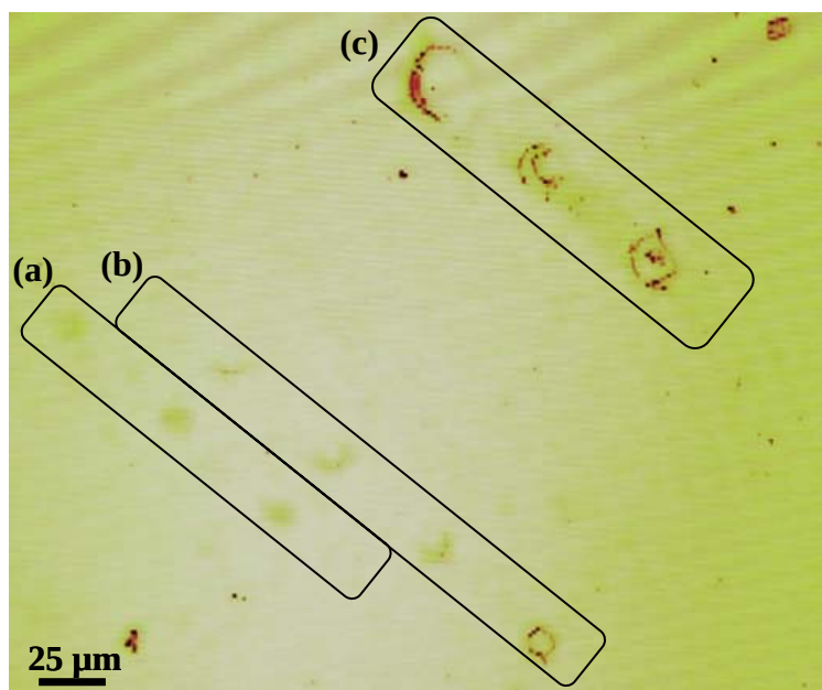
Figure 4.6 : Photographies de microscopie optique de série de dépôts localisés pour une distance entre l'ultramicroélectrode de platine (25 \mu\text{m} de diamètre) et le substrat d'or variable : (a) 25 \mu\text{m} , (b) 20 \mu\text{m} et (c) 10 \mu\text{m} . On applique -1,3 V pendant 30 s à l'UME dans un sol n_{\text{CTAB}}/n_{\text{TEOS}} = 0,32 .
