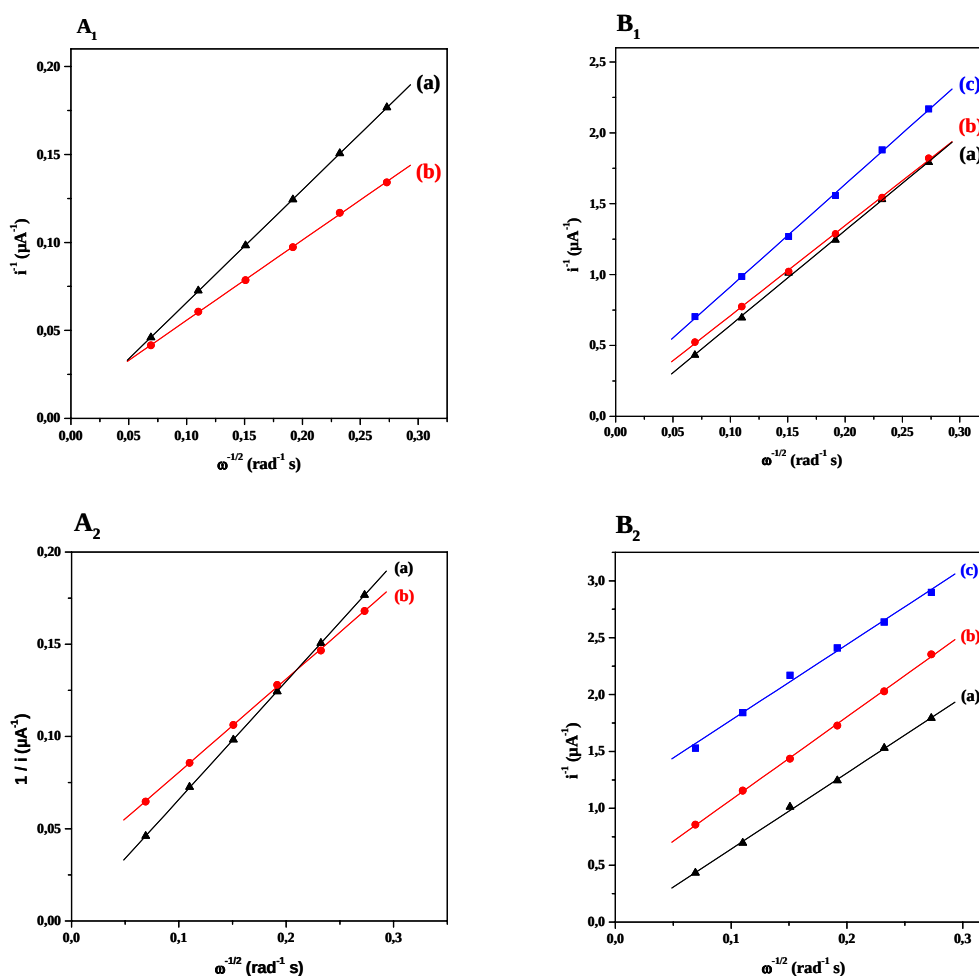
Figure 3.29 : Courbes i^{-1} en fonction de \omega^{-1/2} dans \text{Ru}(\text{NH}_3)_6^{3+} 5 mM ( A_1 et A_2 ) et dans \text{FcEtOH} 0,5 mM ( B_1 et B_2 ), obtenues à partir des voltampérogrammes en électrode tournante réalisés sur une électrode d'or nue (courbes a) et sur des électrodes d'or modifiées par des films à base de silice ordonnée électro-déposés à -1,3 V pendant 1 s à partir d'un sol n_{\text{CTAB}}/n_{\text{TEOS}} = 0,32 ( A_1 et B_1 ) et à partir d'un sol n_{\text{CTAB}}/n_{\text{TEOS+APTES}} = 0,32 et TEOS:APTES 90:10 ( A_2 et B_2 ) avant (courbes c) et après (courbes b) extraction du tensioactif.
