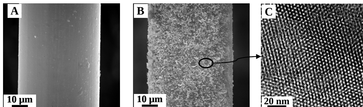
Figure 3.39 : (A-B) Photographies MEB obtenues sur un fil de platine nu (A) et sur un fil de platine modifié par (B) un film de silice ordonnée électro-déposé à -0,9 V pendant 1 s à partir d'un sol n_{\text{CTAB}}/n_{\text{TEOS}} = 0,32 . (C) Photographie MET correspondant au film de l'image (B).
