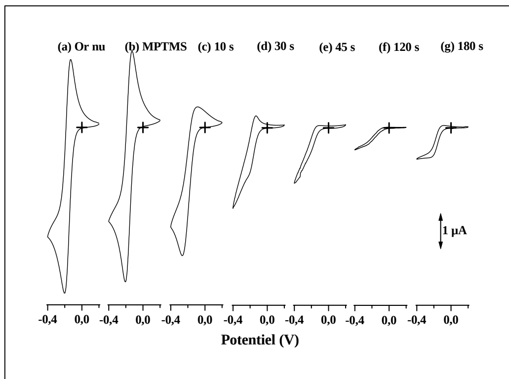
Figure 2.23 : Voltampérogrammes cycliques enregistrés dans \text{Ru}(\text{NH}_3)_6^{3+} 5 \times 10^{-3} \text{ M} (+ \text{NaNO}_3 0,1 M) au moyen d'une électrode d'or nue (a) ou d'électrodes d'or modifiées par une monocouche auto-assemblée de MPTMS (b) ou par des films de silice thiolée électro-déposés à -1,2 V pendant des temps variables : 10 s (c), 30 s (d), 45 s (e), 120 s (f) et 180 s (g), en rotation, dans un sol TEOS/MPTMS 90:10. Vitesse de balayage : 20 \text{ mV s}^{-1} .
