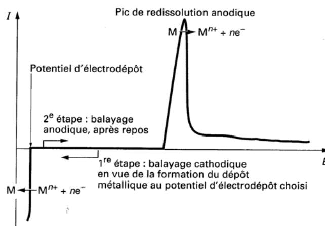
Figure A.10 : Allure d'un voltampérogramme de redissolution anodique après électrolyse pour un cation M^{n+} en solution 11 .
