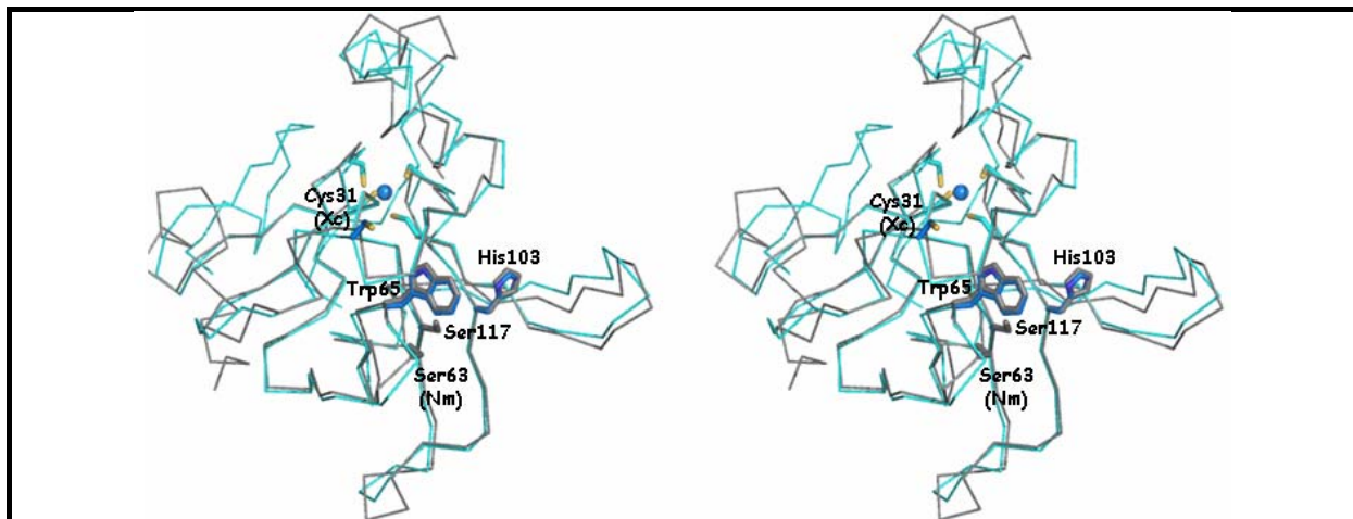
Figure 10 Superposition entre la MsrB de X. campestris (gris) sous sa forme complexée avec le substrat (monomère A) et la MsrB de N. meningitidis également complexée au substrat (monomère A, cyan).
