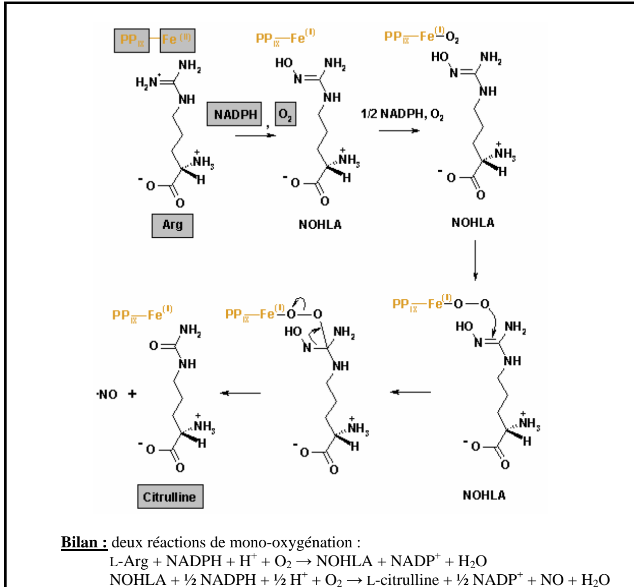
Figure 4 Mécanisme de l'activité oxyde nitrique synthase (pour revue, voir (Marletta 1993)). NOHLA : N-Hydroxyl-L-Arg ; PP IX : protoporphyrine IX ; (tiré de http://en.wikipedia.org/wiki/Nitric_oxide_synthase ).
