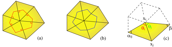
Figure 24. Approximation d'une surface continue autour d'un sommet d'un maillage par une aire de Voronoï (a) et une aire barycentrique (b)
