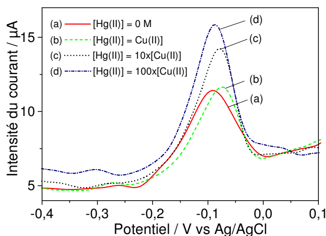
Figure 85 : Voltampérogrammes enregistrés en présence de Hg(II) à différentes concentrations dans le milieu d'accumulation. Conditions: électrode modifiée par K60-bi, Accumulation : 5 min, solution de \text{Cu}(\text{NO}_3)_2 à 5 \cdot 10^{-7} M avec [\text{Hg}(\text{II})] = (a) 0 M, (b) 5 \cdot 10^{-7} M ( 1x[\text{Cu}(\text{II})] ), (c) 5 \cdot 10^{-6} M ( 10x[\text{Cu}(\text{II})] ), (d) 5 \cdot 10^{-5} M ( 100x[\text{Cu}(\text{II})] ), milieu acétate 0,1 M, pH = 5,5 ; Détection : redissolution anodique par voltampérométrie à ondes carrées après 60 s à E = -0,5 V dans \text{HNO}_3 3 M.
