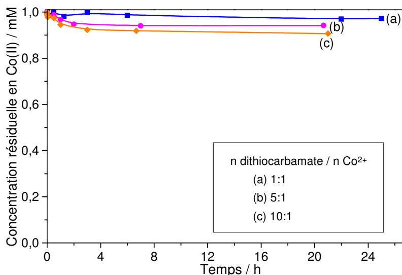
Figure 51 : Evolution de la concentration résiduelle de Co(II) en solution en fonction du temps après ajout de la résine commerciale Q10R. Conditions expérimentales : Solution initiale : [\text{Co(II)}] = 10^{-3} \text{ M} , tampon acétique 0,1 \text{ M} , \text{pH} = 6,5 , V = 200 \text{ mL} ; masses de solide ajoutées (1,25 mmol de groupes dithiocarbamate/g de matériau fonctionnalisé) : (a) m = 160 \text{ mg} soit n_{\text{dithiocarbamate}} = n_{\text{Co(II)}} = 2,10^{-4} \text{ moles} , \text{pH} final de la solution = 6,10 ; (b) m = 800 \text{ mg} soit n_{\text{dithiocarbamate}} = 5 n_{\text{Co(II)}} , \text{pH} final de la solution = 5,98 ; (c) m = 1,6 \text{ g} soit n_{\text{dithiocarbamate}} = 10 n_{\text{Co(II)}} , \text{pH} final de la solution = 5,94. La concentration résiduelle de Co(II) en solution après filtration a été déterminée par analyse ICP-AES.
