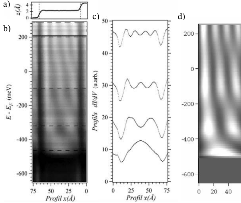
FIGURE 2.14 – Haut droite : (a) Profil topographique de la cavité résonante asymétrique formée par les deux bords de marche séparés de 56 \text{ Å} mesuré avec V_{\text{bias}} = +1.0V et I_t = 0.5nA . (b) Cartographie de conductivité différentielle ( T = 5K , boucle ouverte, \nu = 700Hz , \Delta V = 10mV ). (c) Différentes coupes à énergie constante de (b) réalisées aux différents niveaux d'énergie. (d) Simulation avec r_d = 0.6 , r_a = 0.25 , \phi_a = \phi_d = 2\pi/3 et une largeur de terrasse de 58\text{Å} .
