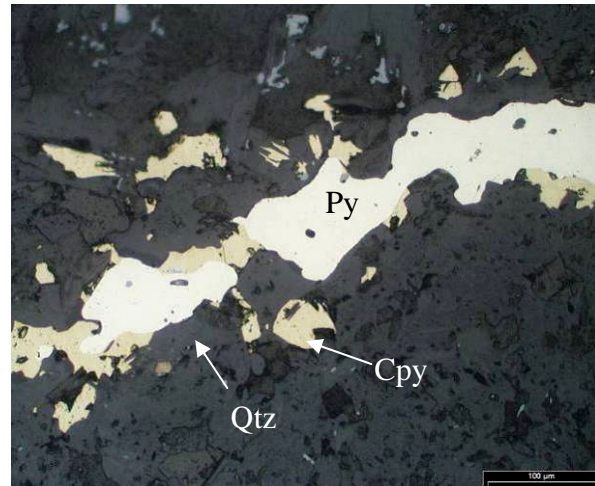
Photo 17. Vue en lumière réfléchie au microscope de cette même veine (F16/592m, photo 12). Abréviations : (Py, Pyrite ; Cpy, Chalcopryrite ; Qtz, Quartz).
