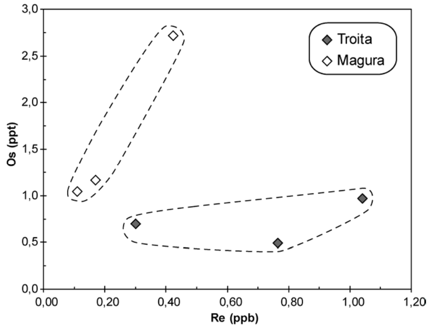
Figure 47. Diagramme des teneurs en rhénium et osmium des échantillons des gisements épithermaux de Troita et Magura.
