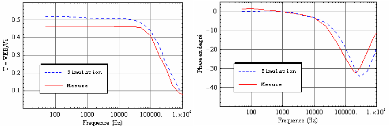
Figure V.14b : Fonction de transfert du stimulateur PM2.
