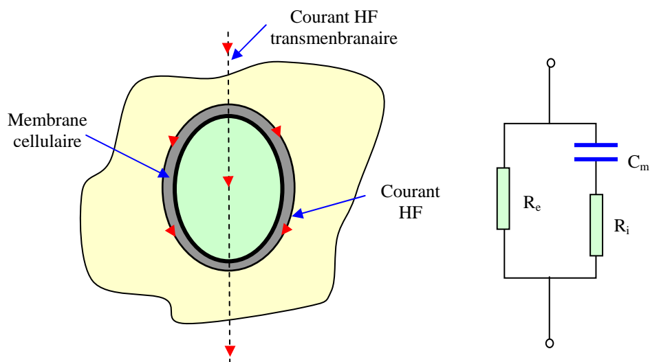
Figure I.15 : Modèle de Fricke.
