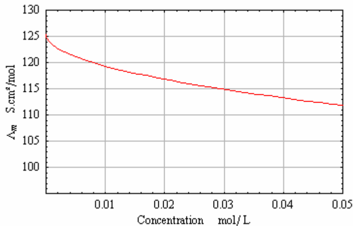
Figure III.22 : Conductivité molaire du chlorure de sodium en fonction de la concentration.
