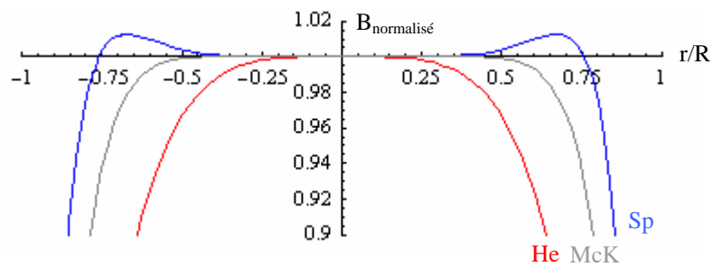
Figure III.10 : Profil radial du champ normalisé.
