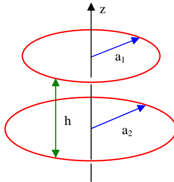
Figure III.12 : Spires coaxiales contenues dans des plans parallèles.
