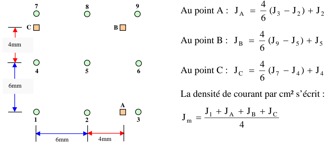
Figure IV.10 : Nouvelle grille de section 1cm 2 .
