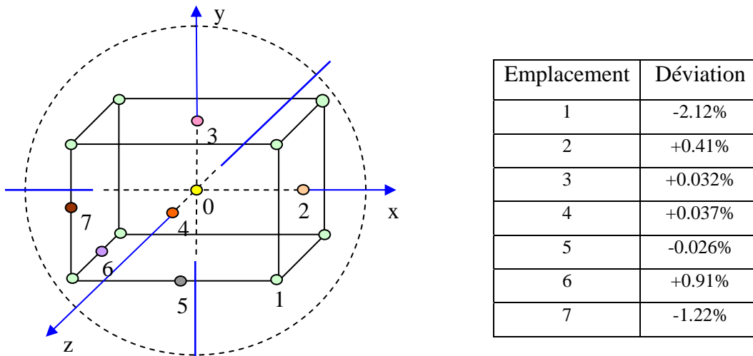
Figure III.17 : Déviation maximale du champ selon la position considérée.
