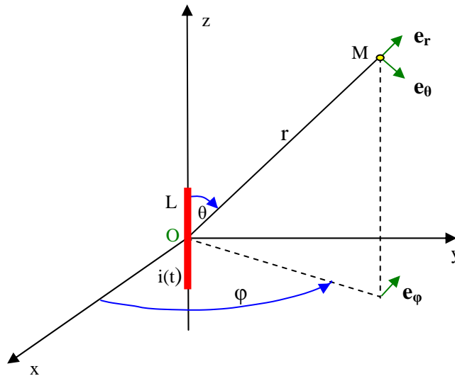
Figure II.15 : Dipôle électrique.
