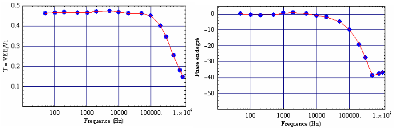
Figure V.10c : Fonction de transfert du stimulateur PM3.
