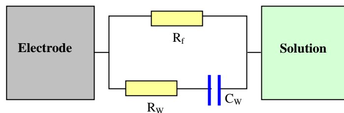
Figure III.32 : Modèle équivalent de Warburg avec résistance faradique.
