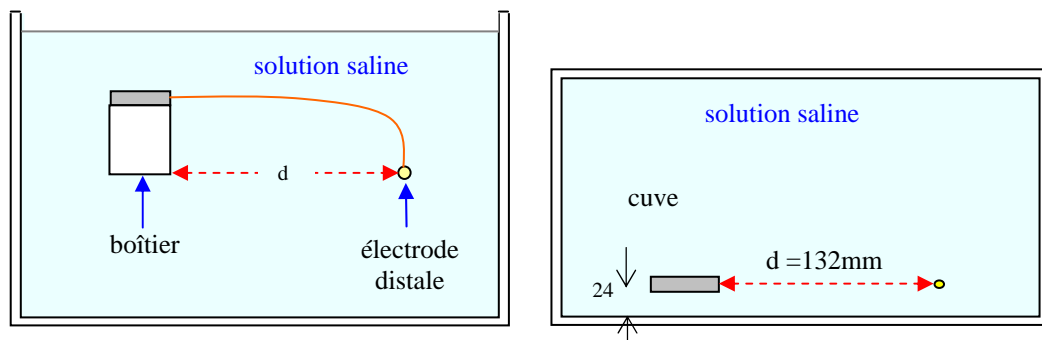
Figure V.7 : Dispositif sous test.
