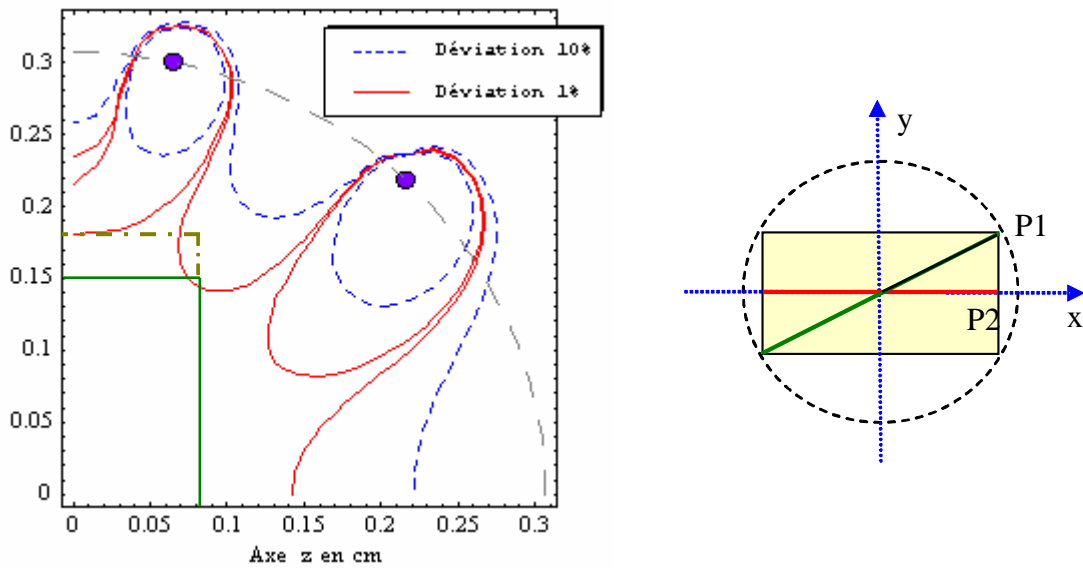
Figure III.16: Courbe d'iso-champ et positionnement du D.S.T. dans le plan (x,0,z) .
