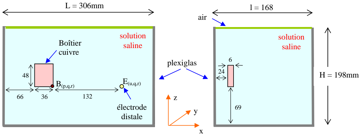
Figure V.31 : Modèle physique du D.S.T. in vitro en perturbations rayonnées.
