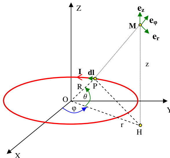
Figure III.4 : Champ magnétique produit par une spire circulaire.
