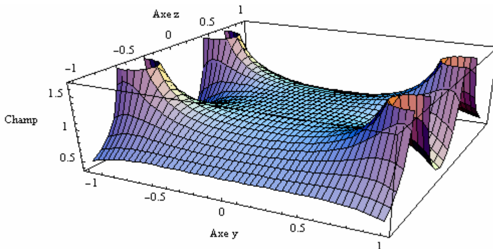
Figure III.6 : Représentation du champ magnétique dans le plan (y,0,z) .
