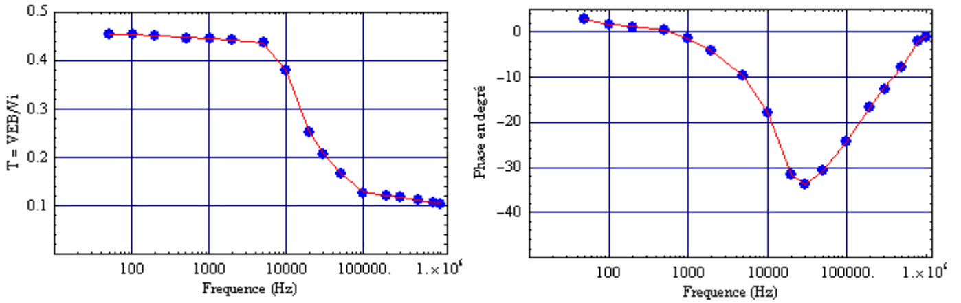
Figure V.10a : Fonction de transfert du stimulateur PM1.
