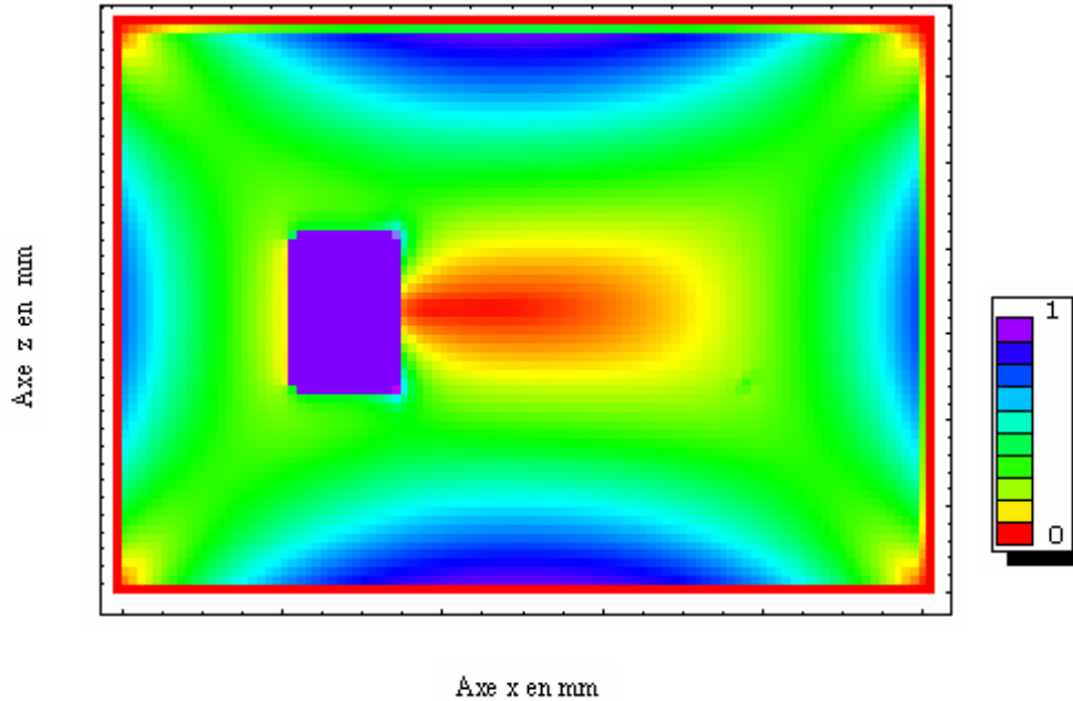
Figure V.32 : Densité de courant relative dans le plan (x0z) contenant le boîtier.
