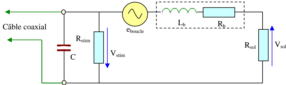
Figure V.26 : Modèle électrique de la boucle formée par l'ensemble boîtier+sonde.
