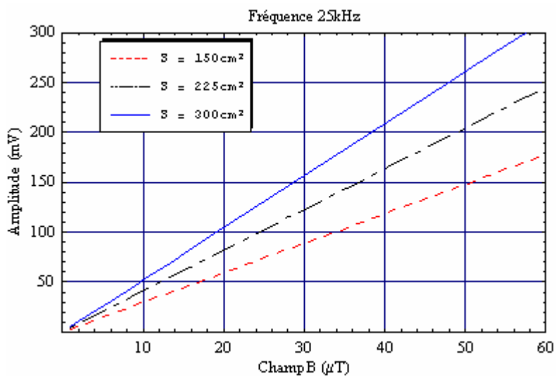
Figure V.36 : Variation de la tension V_{stim} en fonction du champ magnétique pour f = 25 kHz.
