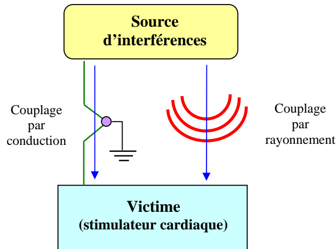
Figure II.13 : Chemins de couplage entre source et victime.
