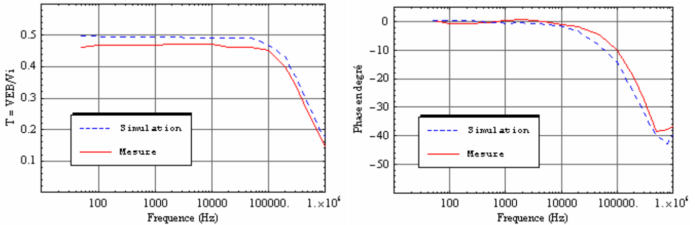
Figure V.16 : Fonction de transfert du stimulateur PM3 avec prise en compte de Z_{pol} .
