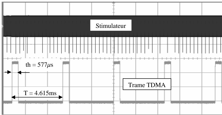
Figure V.23 : Signal de perturbation : trame TDMA.
