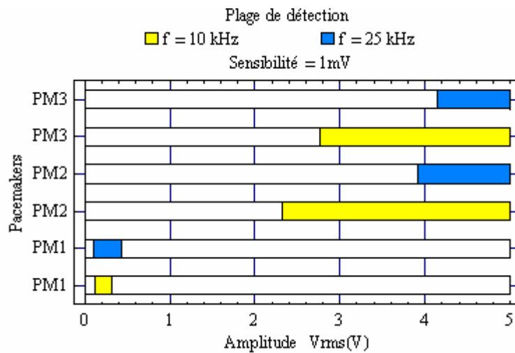
Figure V.3 : Plages de détection des stimulateurs cardiaques simple chambre étudiés.
