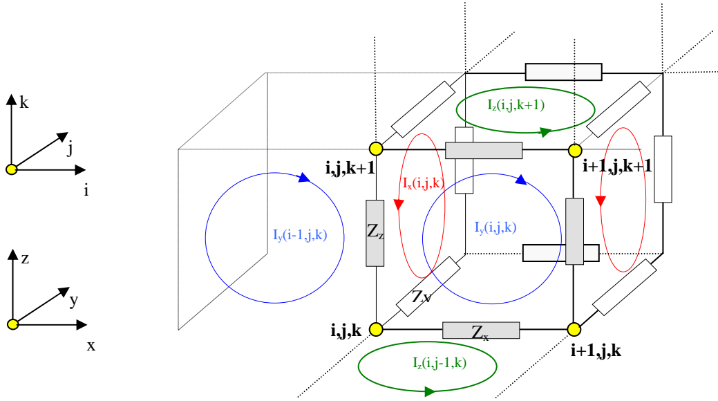
Figure IV.8 : Courants de boucle dans le plan (x,0,z).
