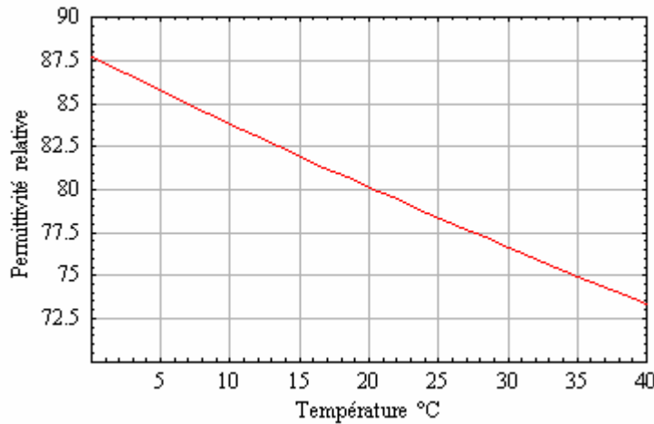
Figure III.25 : Variation de la permittivité relative en fonction de la température.
