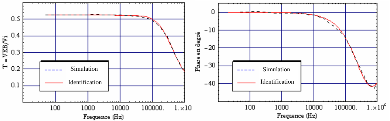
Figure V.18c : Modélisation de la fonction de transfert pour PM3.
