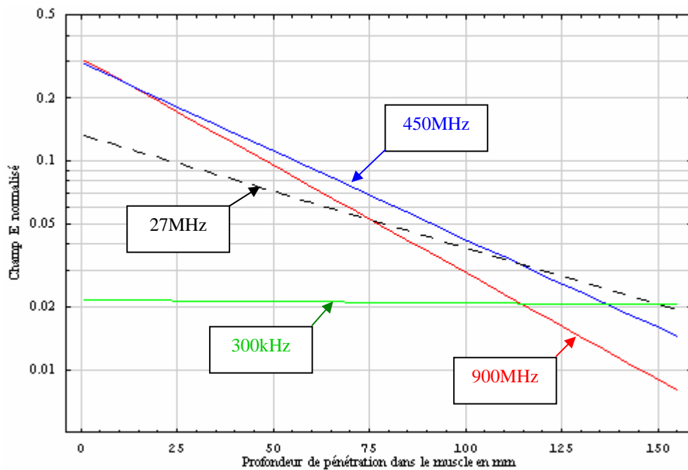
Figure I.10 : Evolution de E_{N(z)} dans le muscle en fonction de la profondeur de pénétration.
