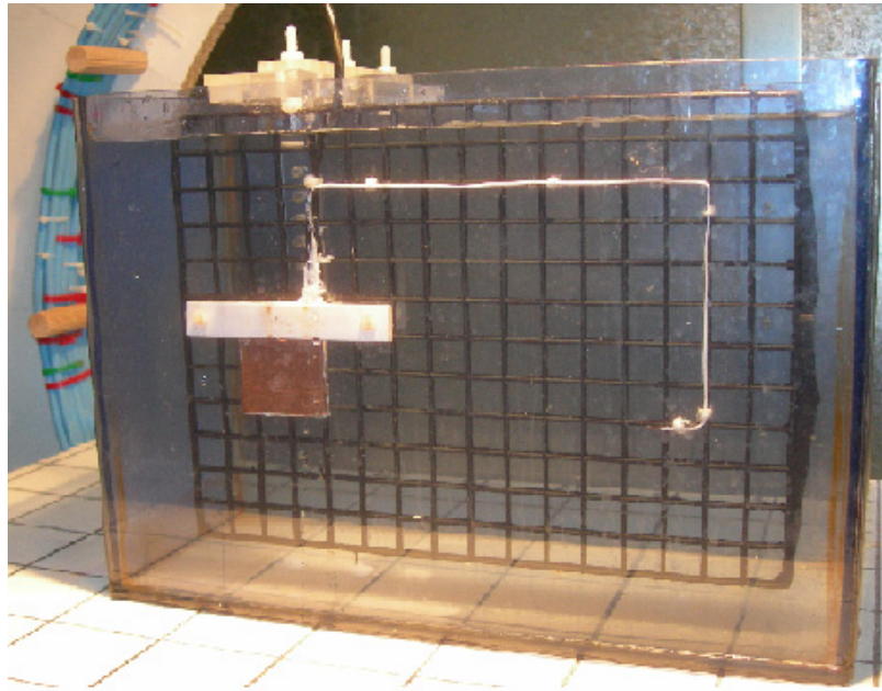
Figure V.29 : Photographie du D.S.T. dans le cas des essais in vitro.
