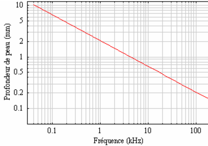
Figure III.13 : Variation de la profondeur de peau dans le cuivre en fonction de la fréquence.
