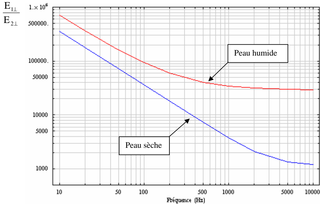
Figure I.4 : Variations du rapport \frac{E_{1\perp}}{E_{2\perp}} en fonction de la fréquence.
