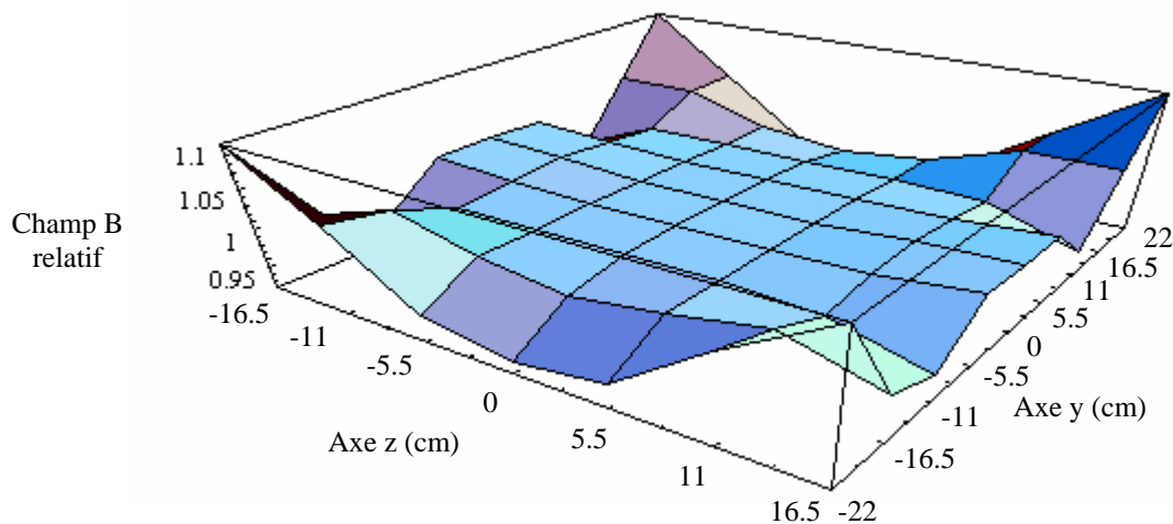
Figure III.20 : Cartographie normalisée du champ magnétique dans le plan (y,0,z).
