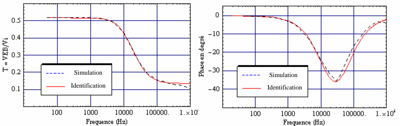
Figure V.18a : Modélisation de la fonction de transfert pour PM1.
