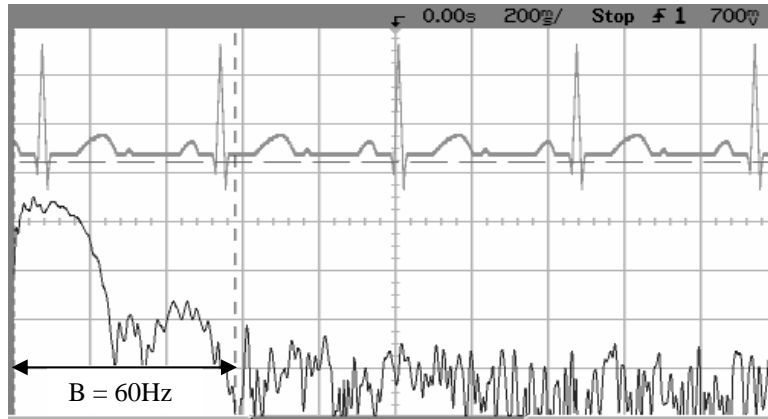
Figure II.6 : Spectre de fréquence d'un signal ECG.
