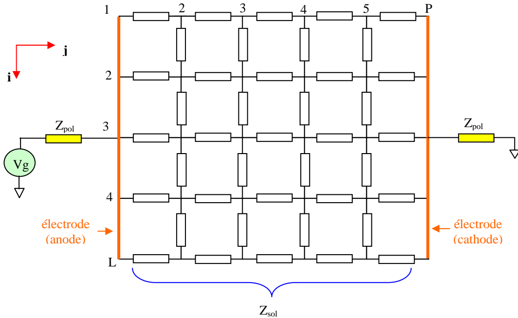
Figure V.15 : Modèle intégrant l'impédance de polarisation.
