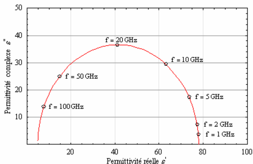
Figure III.29 : Diagramme d'Argand de la solution saline.
