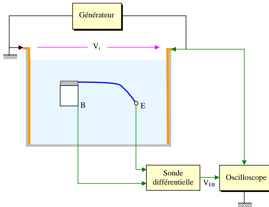
Figure V.9 : Principe de la mesure de la fonction de transfert.
