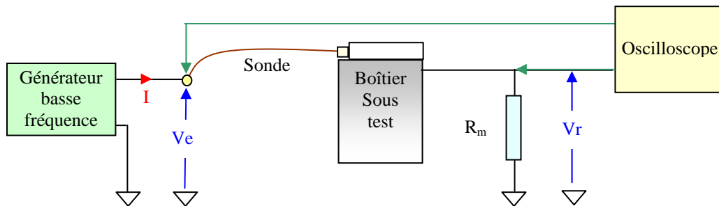
Figure V.5 : Mesure de l'impédance interne des stimulateurs.
