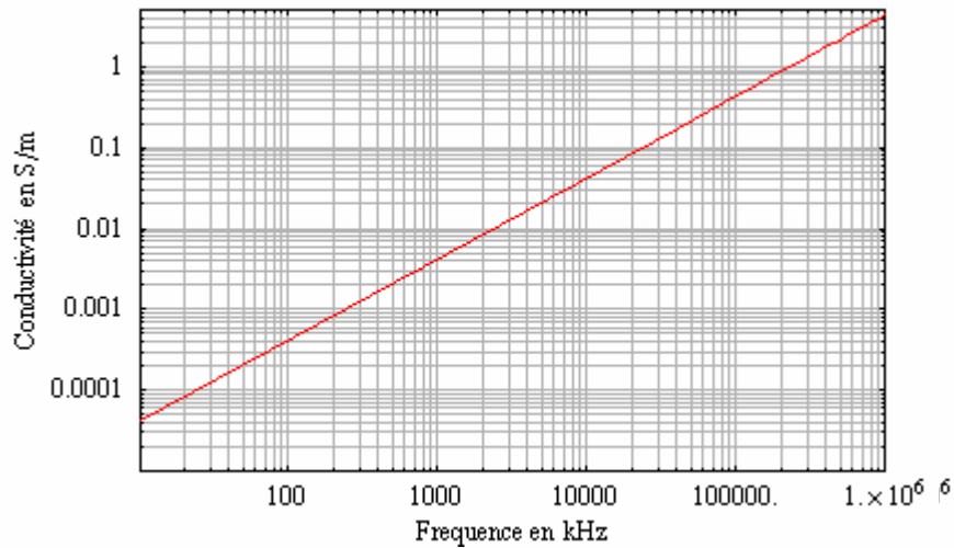
Figure III.27 : Variation de la partie imaginaire de la conductivité en fonction de la fréquence.
