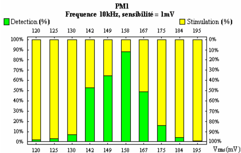
Figure V.4 : Graphe statistique du stimulateur PM1.
