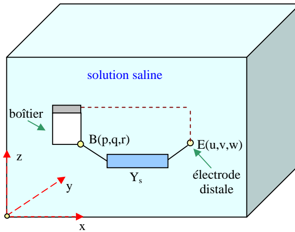
Figure V.12 : Prise en compte de l'admittance interne Y_s dans le modèle.
