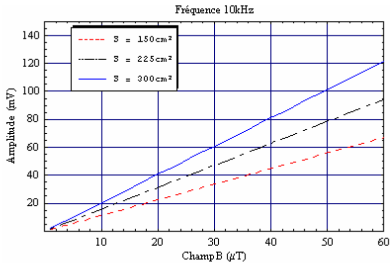
Figure V.35 : Variation de la tension V_{stim} en fonction du champ magnétique pour f = 10 kHz.
