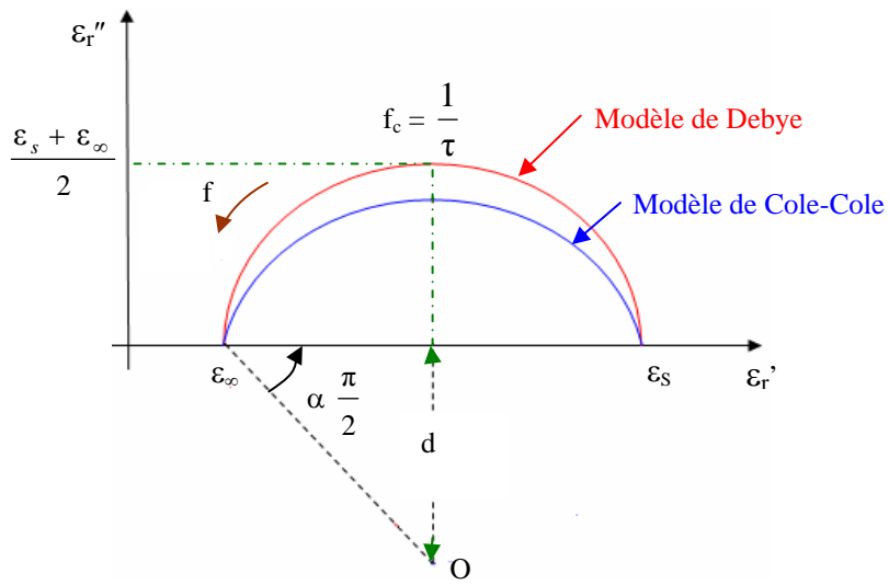
Figure I.19 : Diagramme d'Argand d'après les modèles de Debye et Cole-Cole.
