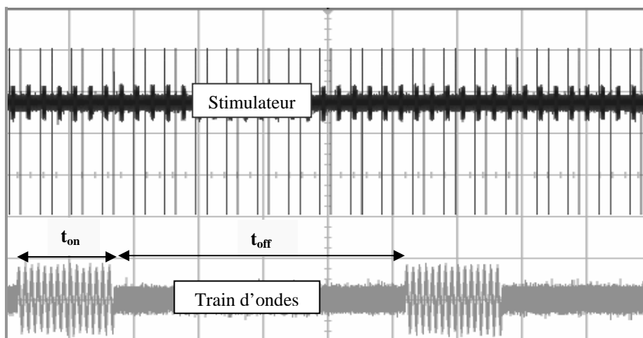
Figure V.21 : Signal de perturbation : train d'ondes sinusoïdales.
