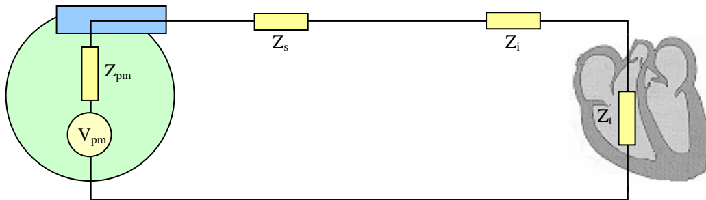
Figure II.11 : Circuit électrique équivalent en stimulation.
