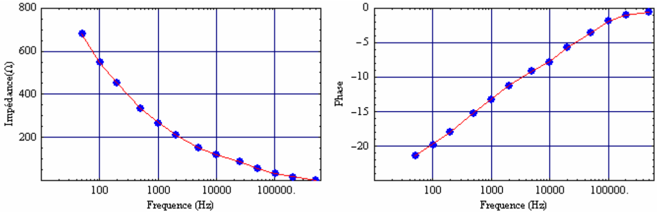
Figure III.33: Impédance de polarisation stimulateur + électrode distale.
