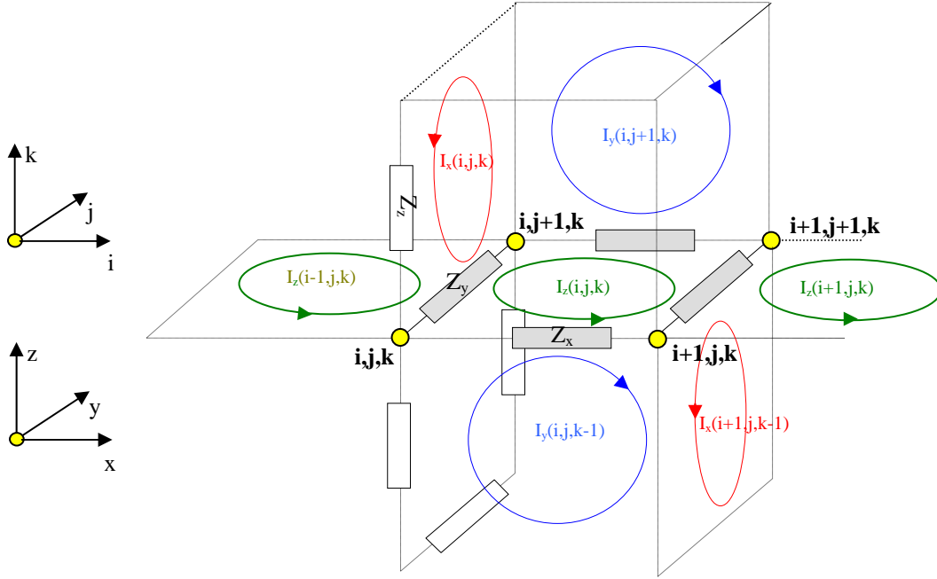
Figure IV.9 : Courants de boucle dans le plan (x,0,y).
