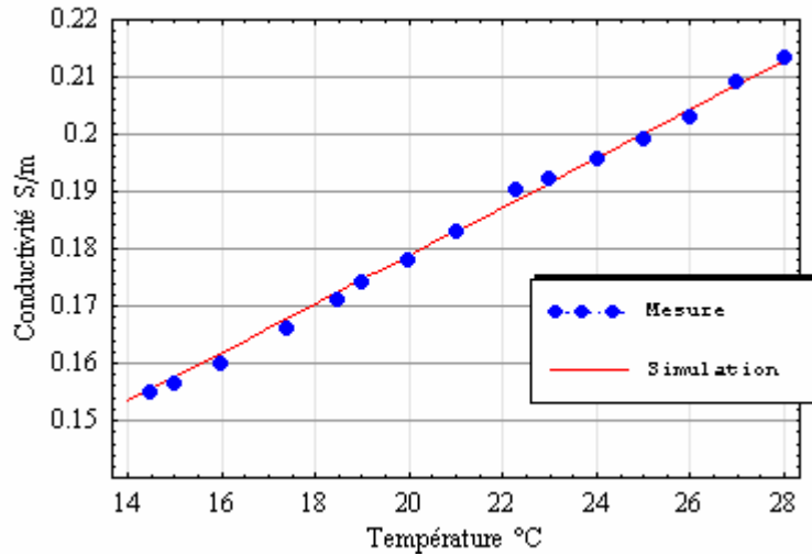
Figure III.23: Variation de la conductivité en fonction de la température (solution NaCl).
