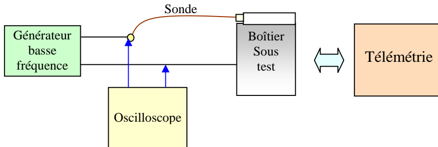
Figure V.1 : Essais dans l’air.
