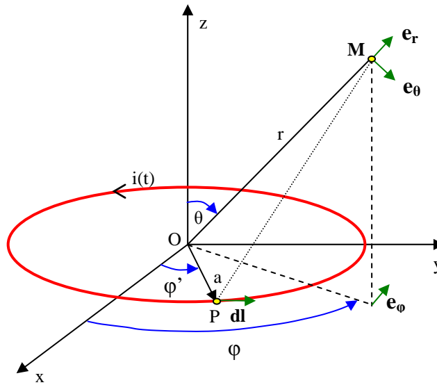
Figure II.14 : Dipôle magnétique.
