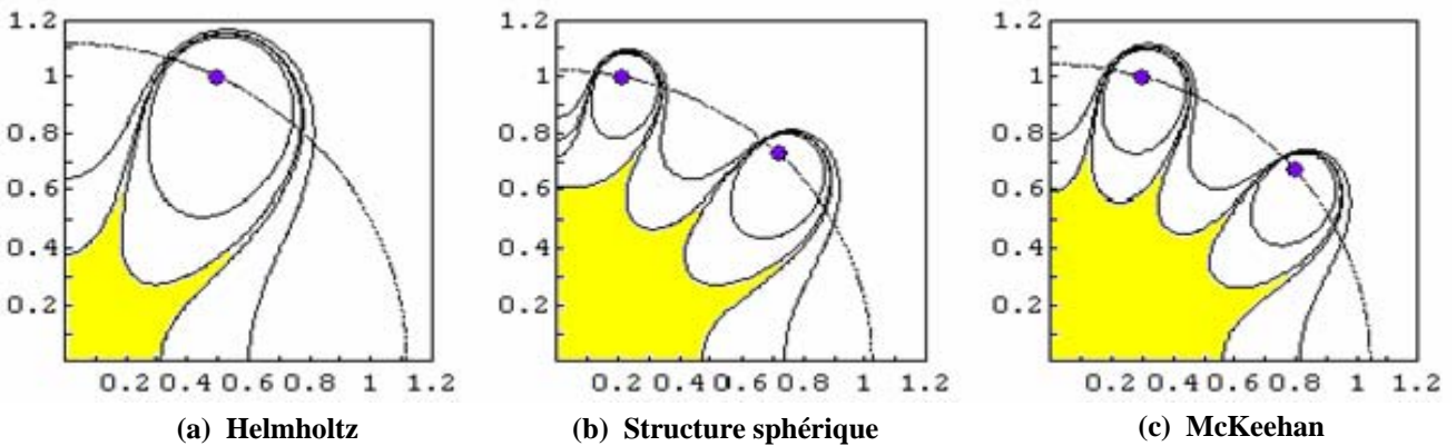
Figure III.11 : Courbes iso-champ des différentes structures.
