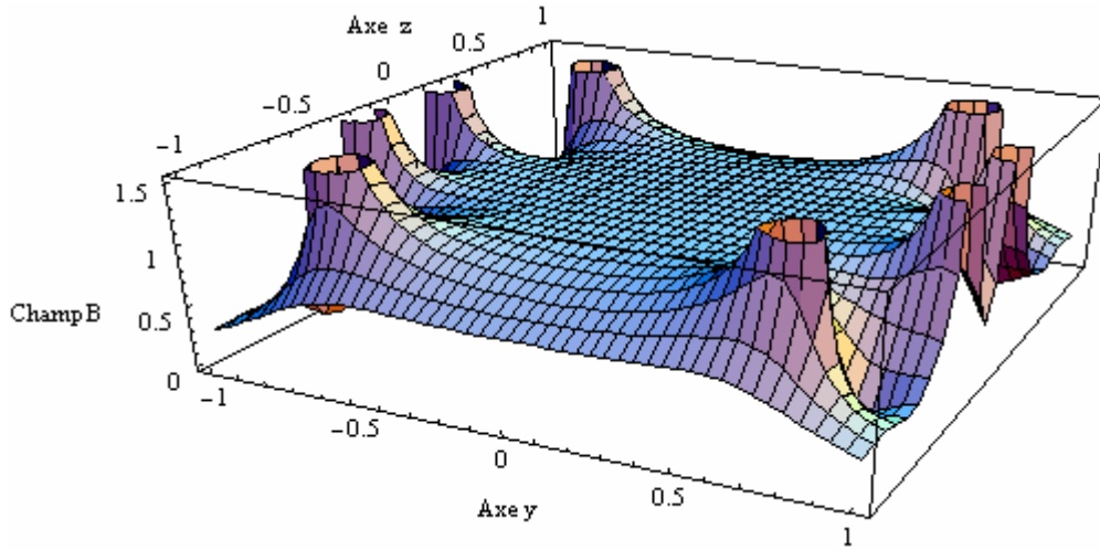
Figure III.8 : Représentation du champ magnétique dans le plan (y,0,z)
