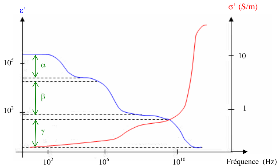
Figure I.16 : Principaux phénomènes de relaxation dans les tissus.
