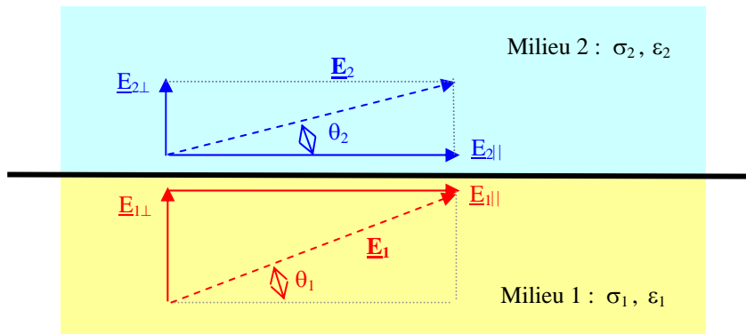
Figure I.3 : Conditions de passage du champ électrique.
