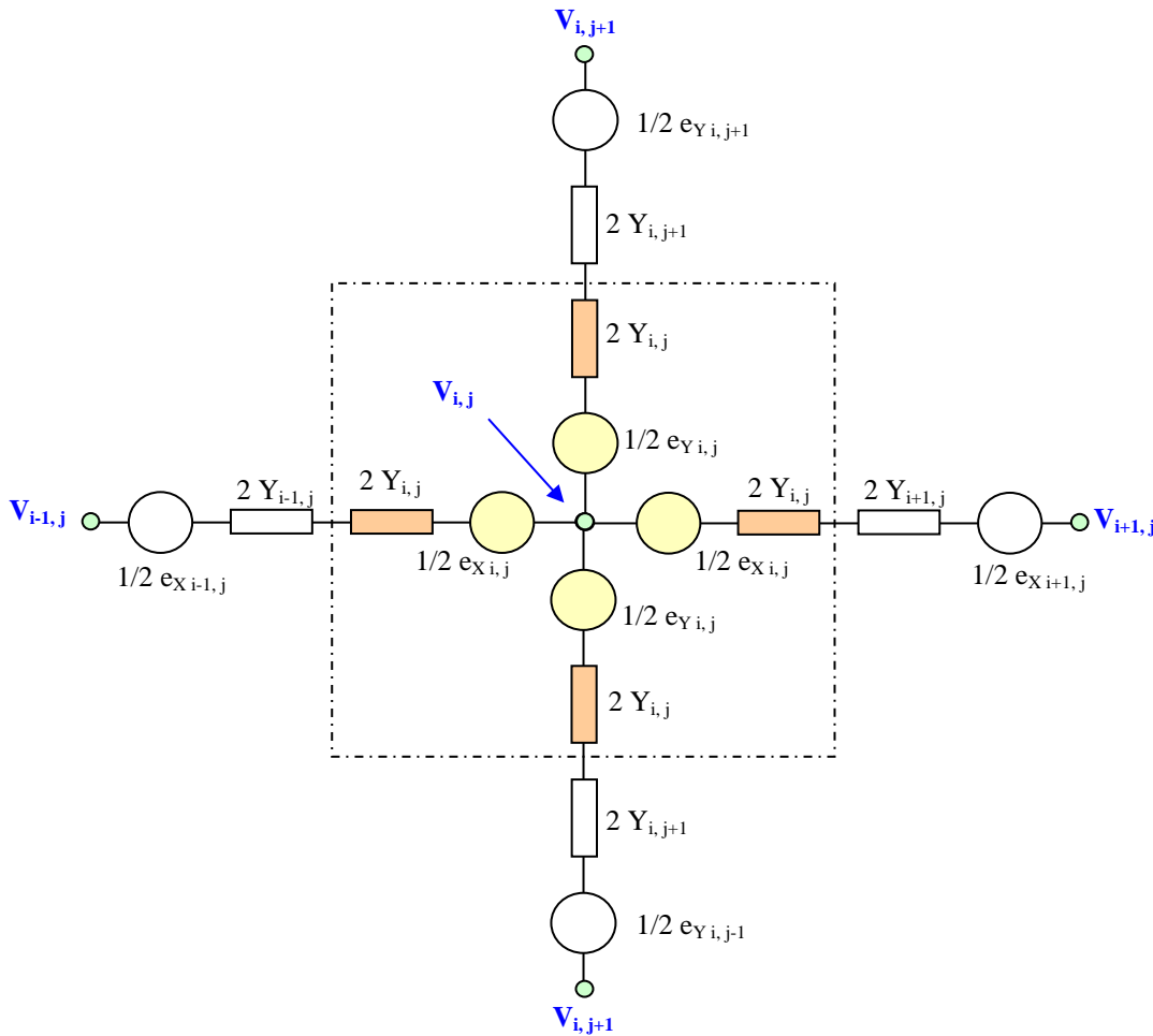
Figure IV.5 : Représentation bidimensionnelle de la cellule élémentaire.
