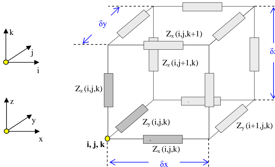
Figure IV.6 : Discrétisation d'un volume élémentaire.
