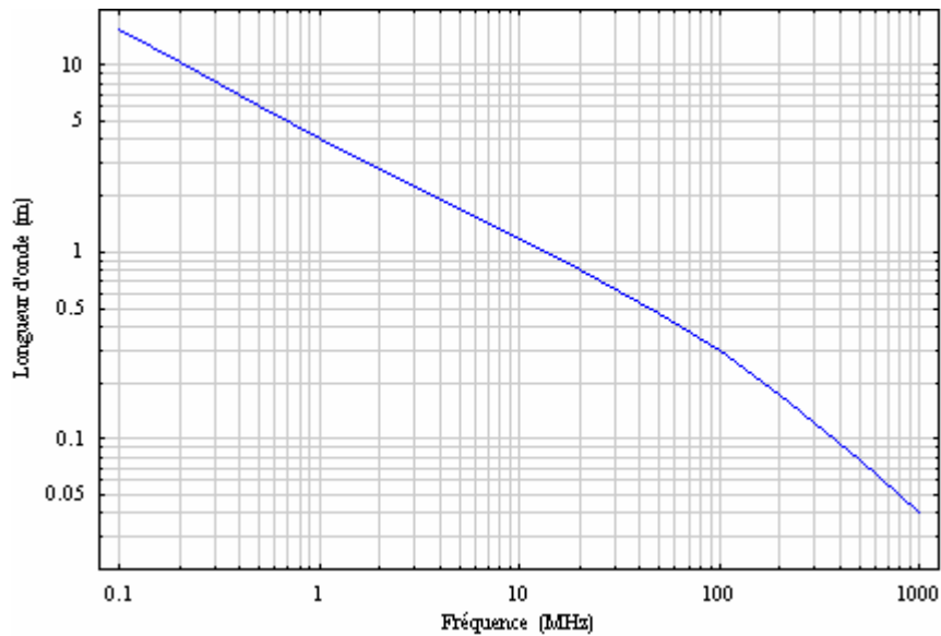
Figure I.1 : Variation de la longueur d'onde dans le muscle en fonction de la fréquence.
