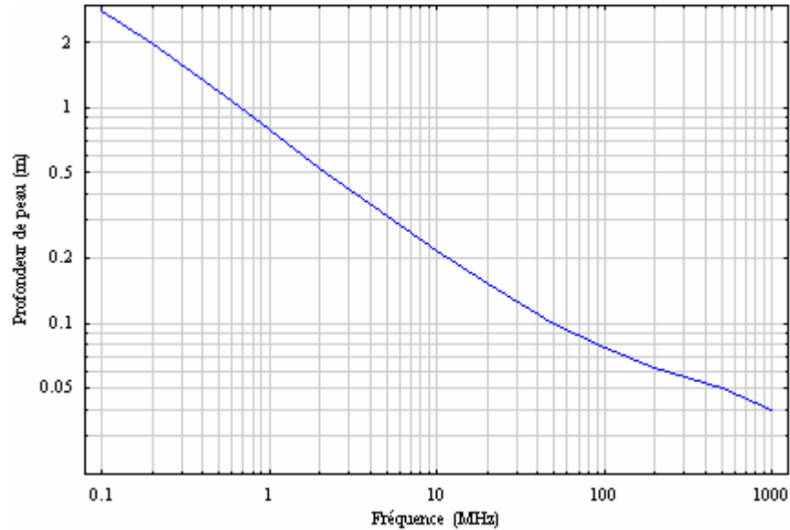
Figure : I.2 Variations de la profondeur de peau \delta en fonction de la fréquence pour le muscle.
