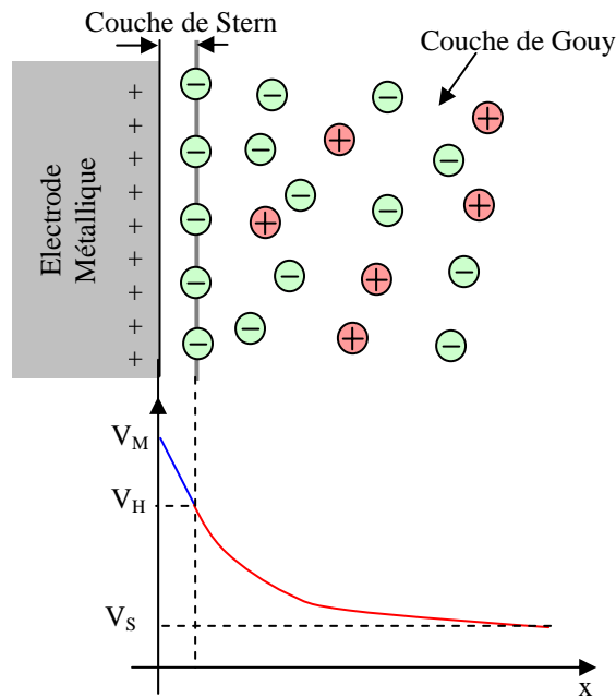
Figure III.31 : Structure du modèle double couche suivant le modèle de Stern.
