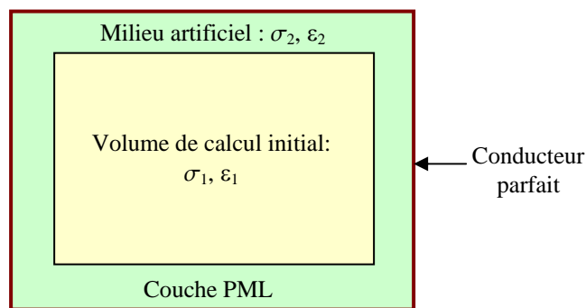
Figure IV.4 : Principe de la méthode PML.
