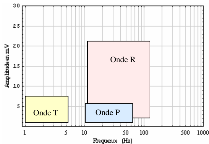
Figure II.5 : Spectre de fréquence des signaux cardiaques.
