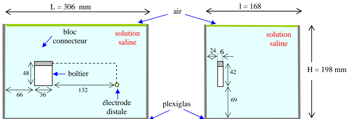
Figure V.11 : Modèle utilisé pour la simulation.
