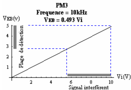
Figure V.20 : Variations de V_{EB} en fonction de V_i pour le pacemaker PM3.
