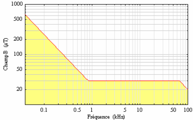
Figure III.14 Champ B maximum admissible par la directive 2004/40CE.
