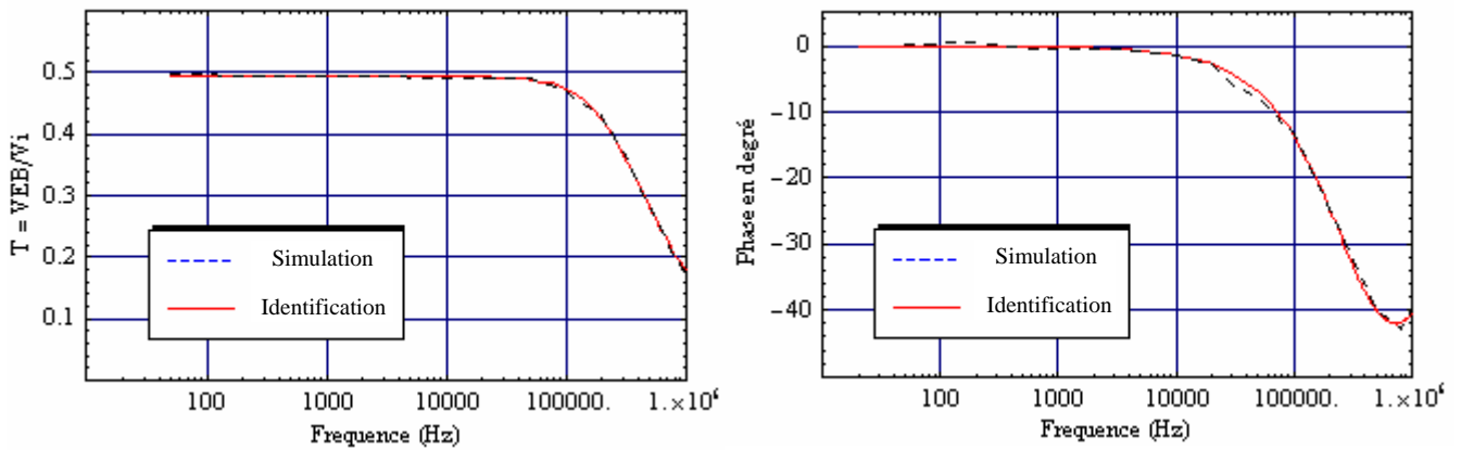
Figure V.19 : Modélisation de la fonction de transfert pour PM3.
