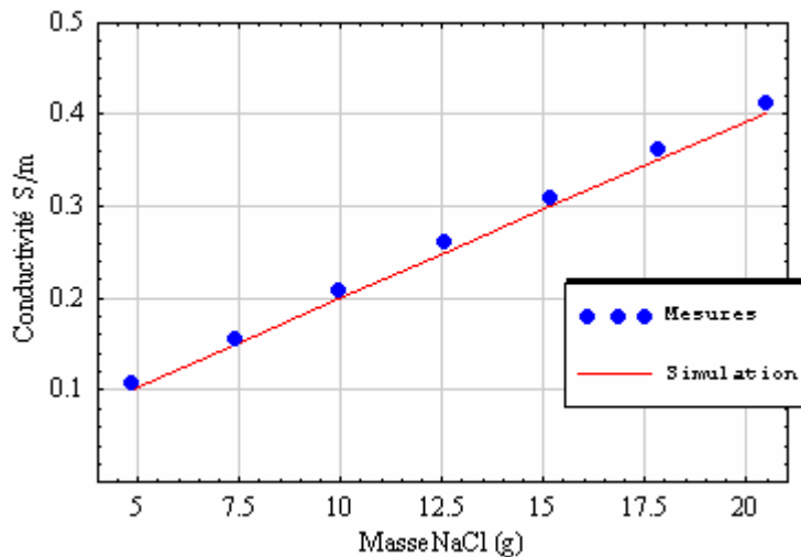
Figure III.24 : Mesure de la conductivité en fonction de la masse de NaCl.
