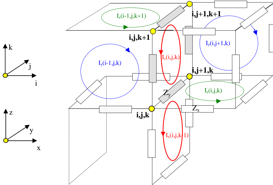
Figure IV.7 : Courants de boucle dans le plan (y,0,z).
