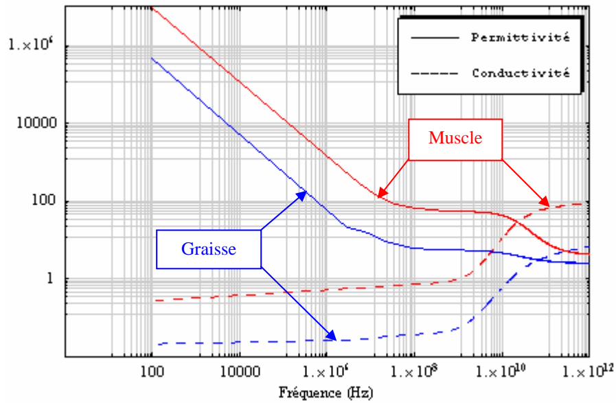
Figure I.20 : Permittivité et conductivité du muscle et de la graisse.
