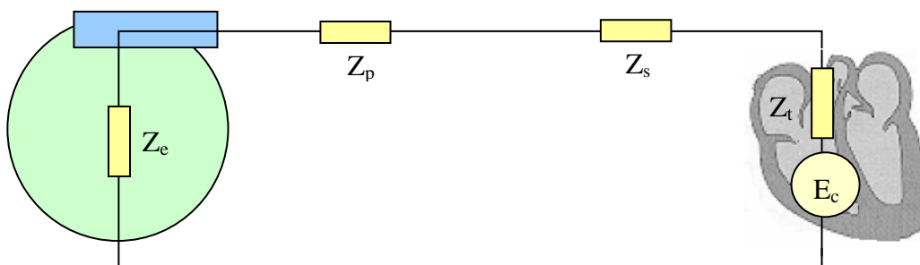
Figure II.12 : Circuit électrique équivalent en détection.
