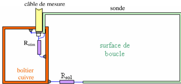
Figure V.25 : Boîtier d'essai muni de sa sonde.
