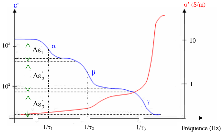
Figure I.18 : Variations de la permittivité relative et de la conductivité apparente dans l'équation de Debye modifiée.
