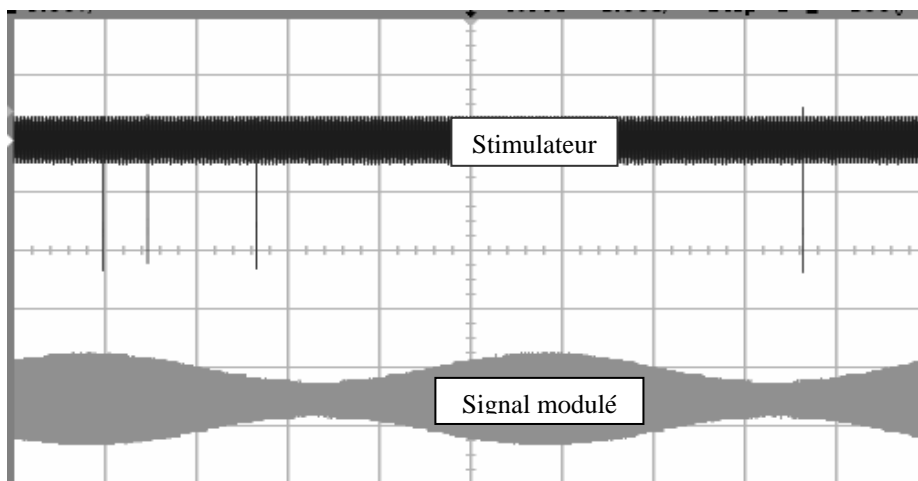
Figure V.22 : Signal de perturbation : signal modulé en amplitude.
