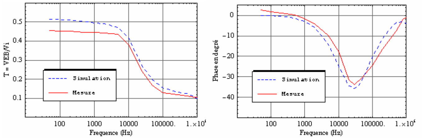
Figure V.14a : Fonction de transfert du stimulateur PM1.
