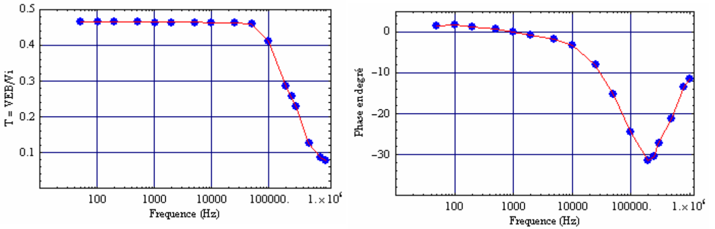
Figure V.10b : Fonction de transfert du stimulateur PM2.
