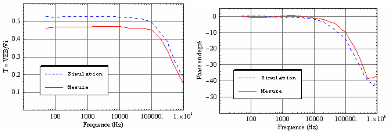
Figure V.14c : Fonction de transfert du stimulateur PM3.
