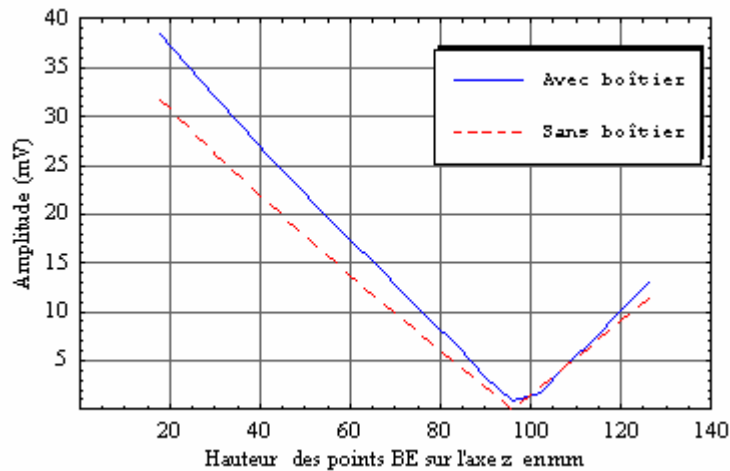
Figure V.33 : Variation de la tension induite sur l'axe z.
