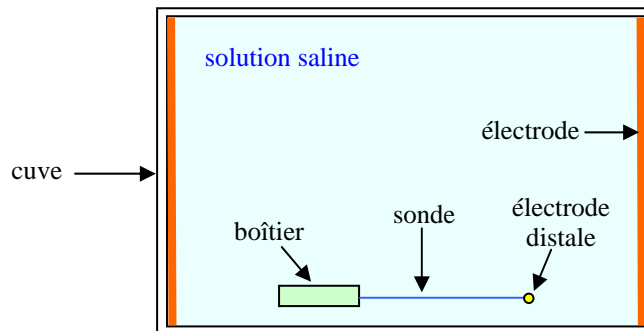
Figure V.8 : Dispositif sous test.
