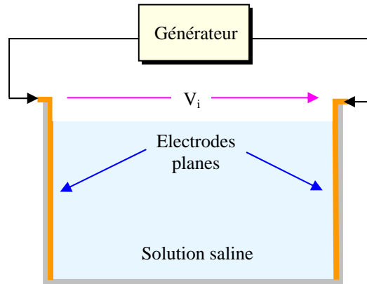
Figure III.30 : D.S.T. en configuration perturbations conduites.
