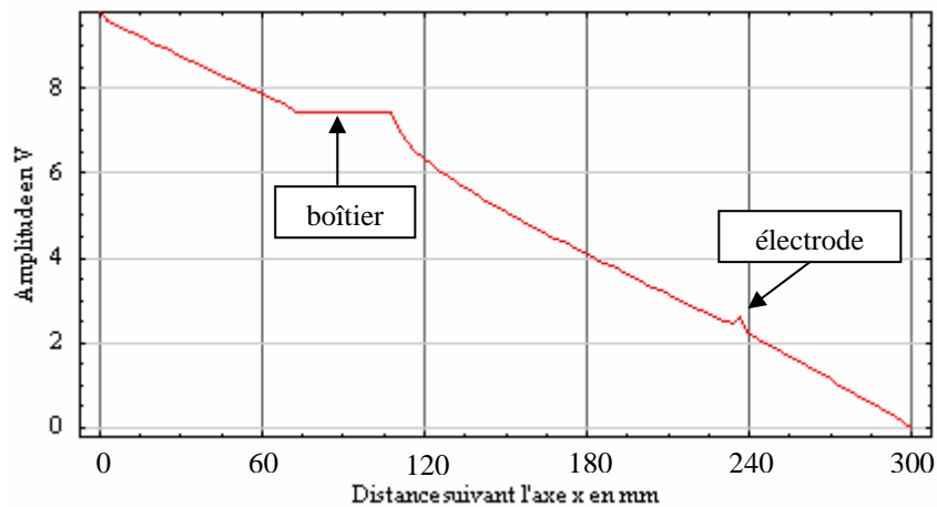
Figure V.17 : Profil de la distribution des potentiels dans le modèle équivalent tissu.
