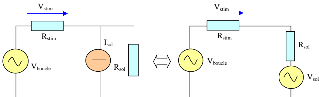
Figure V.30 : Schéma équivalent du D.S.T. in vitro en perturbations rayonnées.
