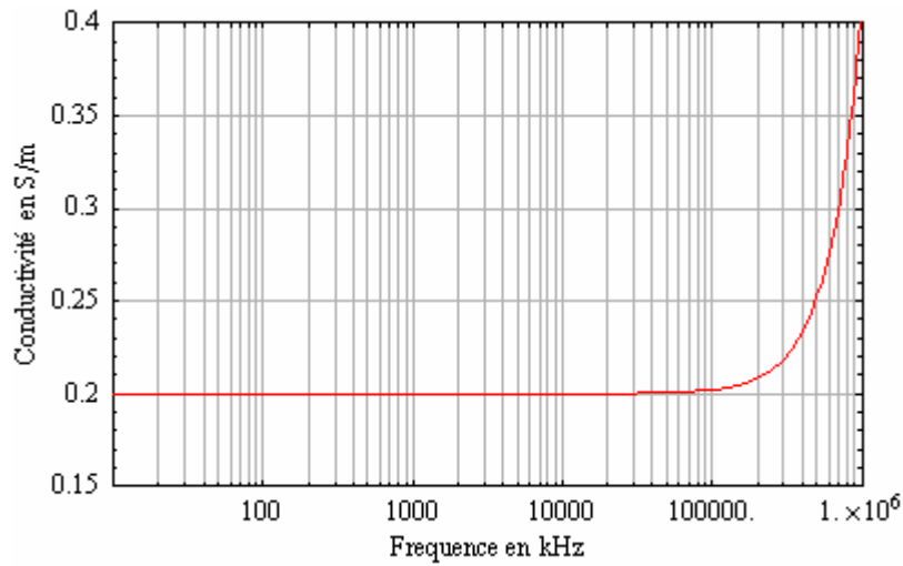
Figure III.26 : Variation de la partie réelle de la conductivité en fonction de la fréquence.
