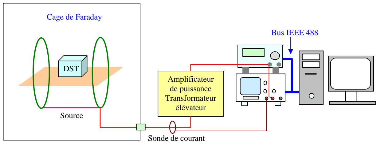
Figure III.2 : Banc expérimental en configuration perturbations par couplage magnétique.
