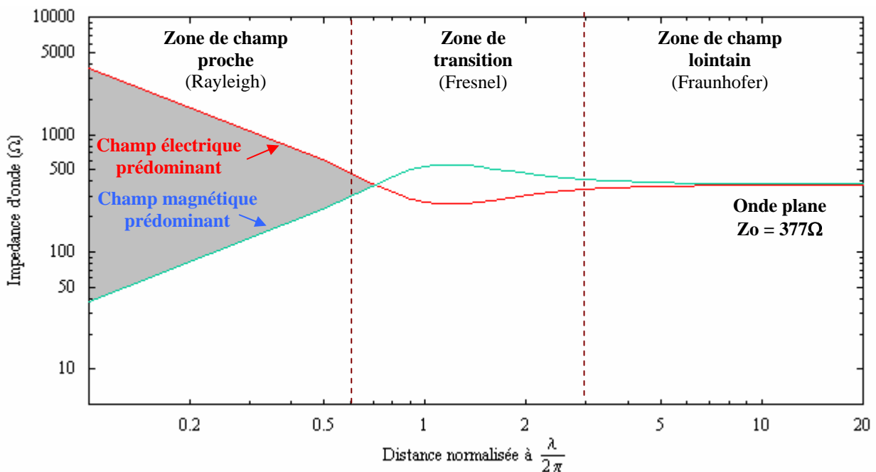
Figure II.17 : Variation de l'impédance d'onde en fonction de la distance normalisée par rapport à la source.
