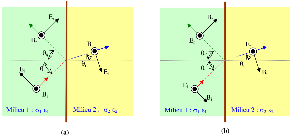
Figure I.6 : Polarisation parallèle (a) et polarisation perpendiculaire (b).
