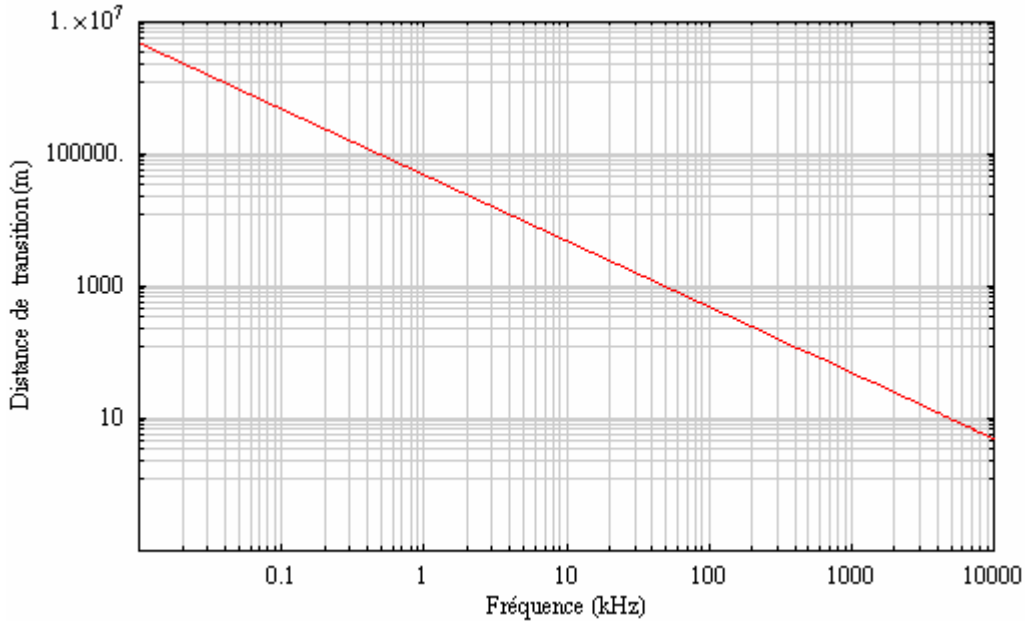
Figure II.18 : Distance de transition entre champ proche et champ lointain en fonction de la fréquence.
