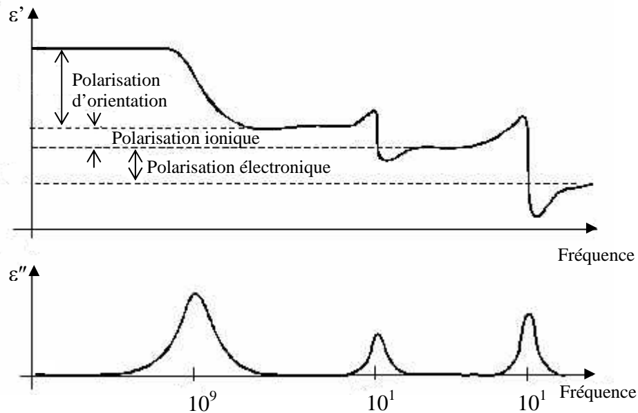
Figure I.13 : Phénomènes de relaxation et mécanismes de polarisation associés.
