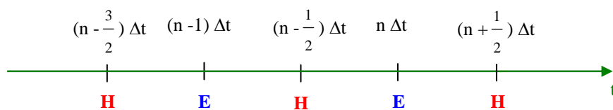
Figure IV.3 : Discrétisation temporelle.
