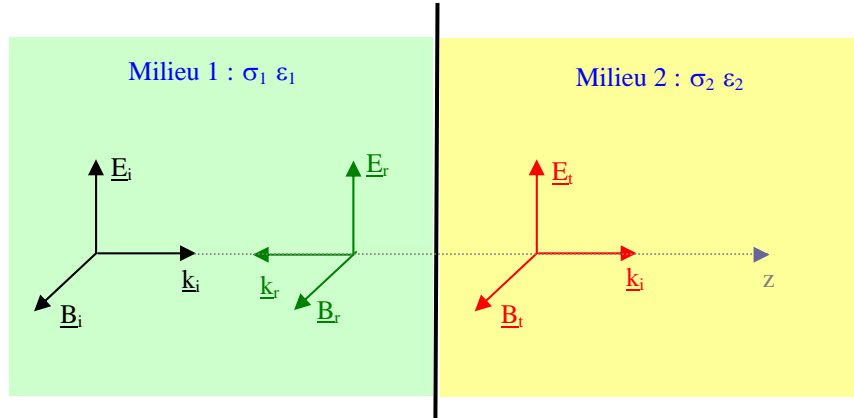
Figure I.7 : Ondes transmises et réfléchi en incidence normale.
