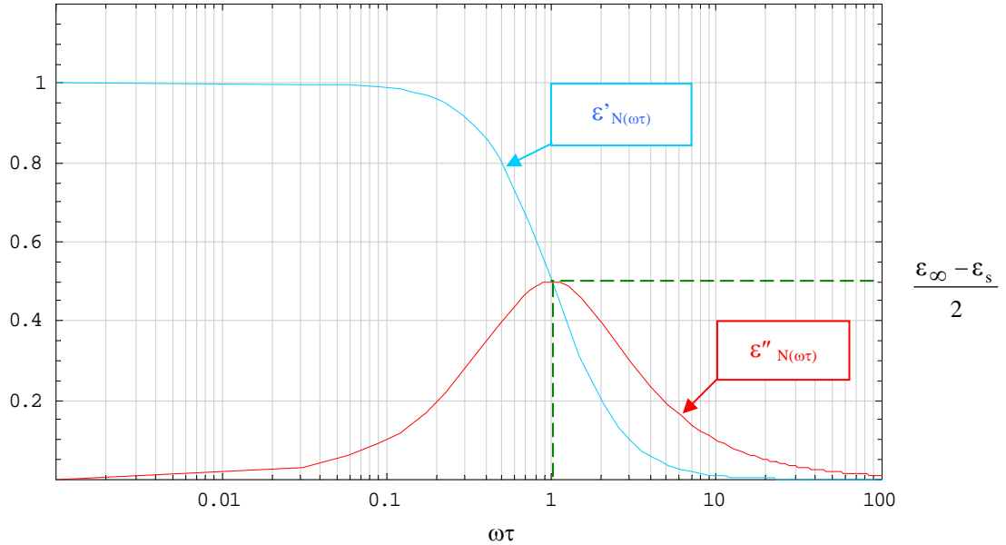
Figure I.17 : Evolution des parties réelle et imaginaire de la permittivité normalisée.
