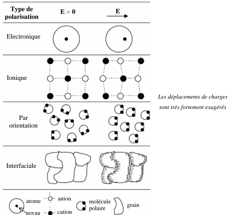
Figure I.12 : Différents types de polarisation.
