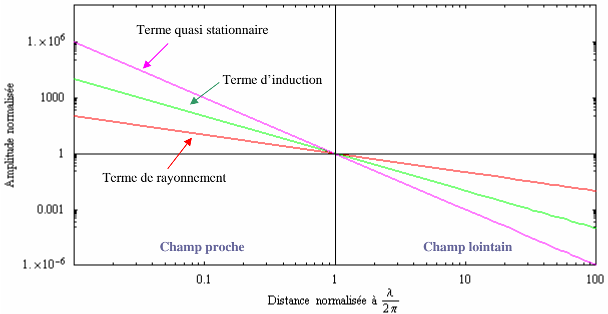
Figure II.16 : Variation relative des termes de rayonnement, d'induction et quasi-stationnaire.
