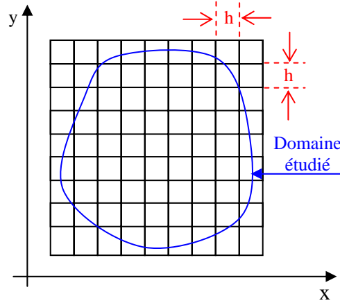
Figure IV.1 : Grille de calcul pour la méthode des différences finies.
