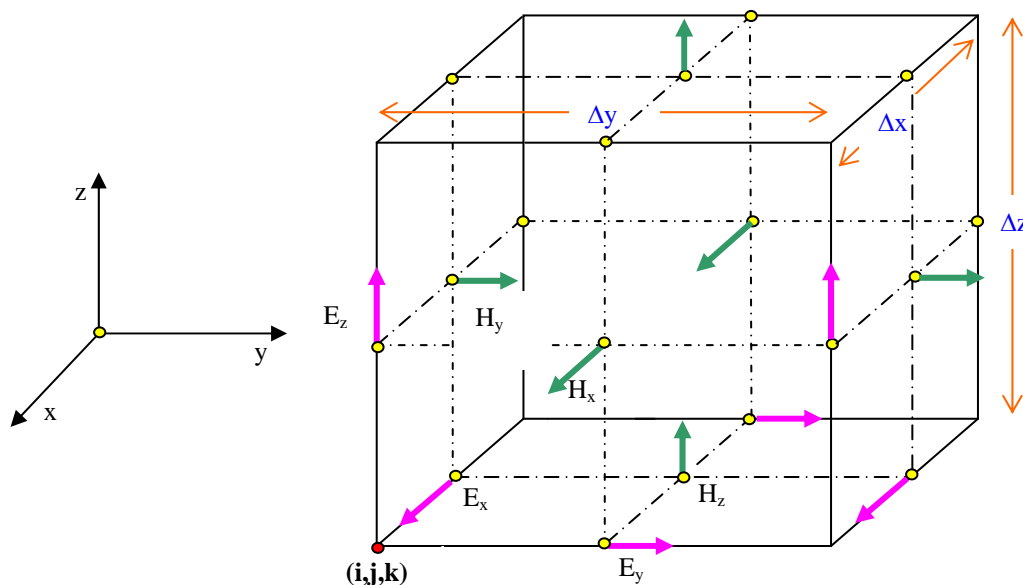
Figure IV.2 : Positions des composantes du champ dans la maille de Yee.
