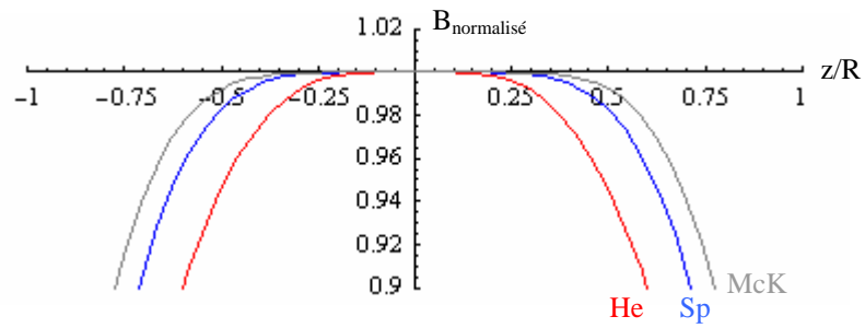
Figure III.9 : Profil axial du champ normalisé.
