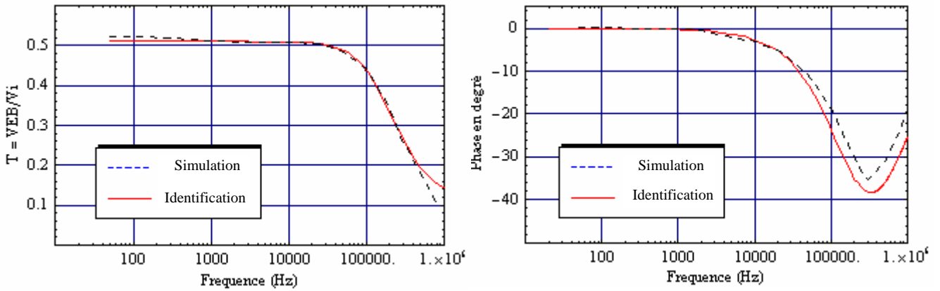
Figure V.18b : Modélisation de la fonction de transfert pour PM2.
