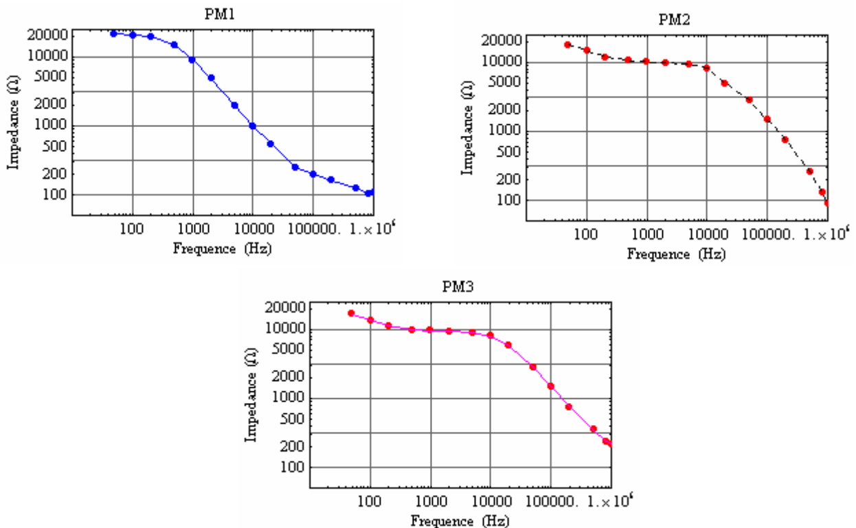
Figure V.6 : Variation de l'impédance en fonction de la fréquence.
