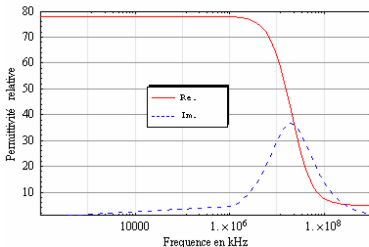
Figure III.28 : Variation des parties réelle et imaginaire de la permittivité.
