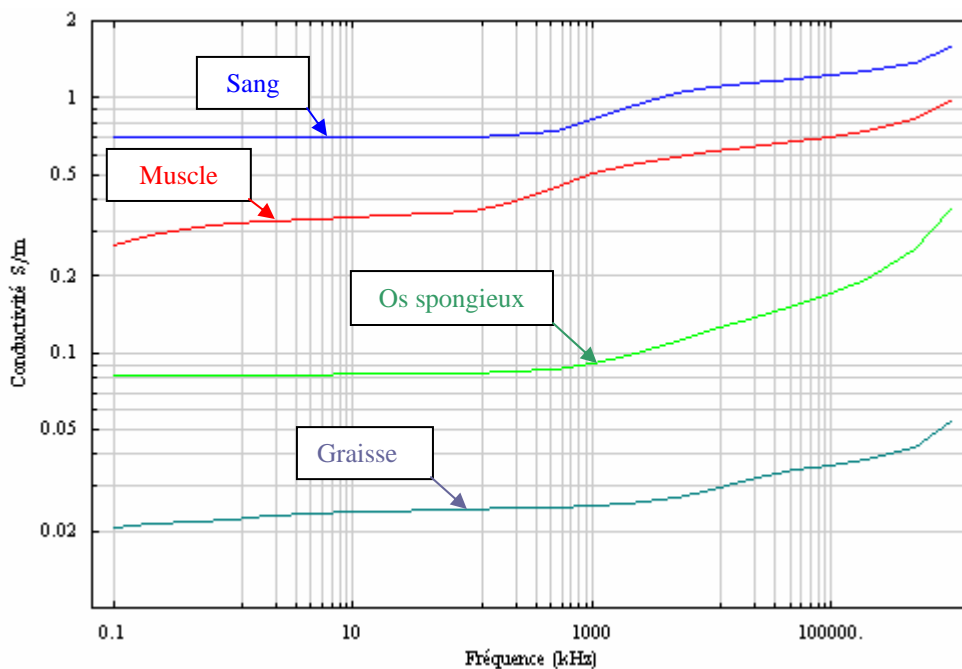
Figure I.11 : Evolution de la conductivité de certains tissus.
