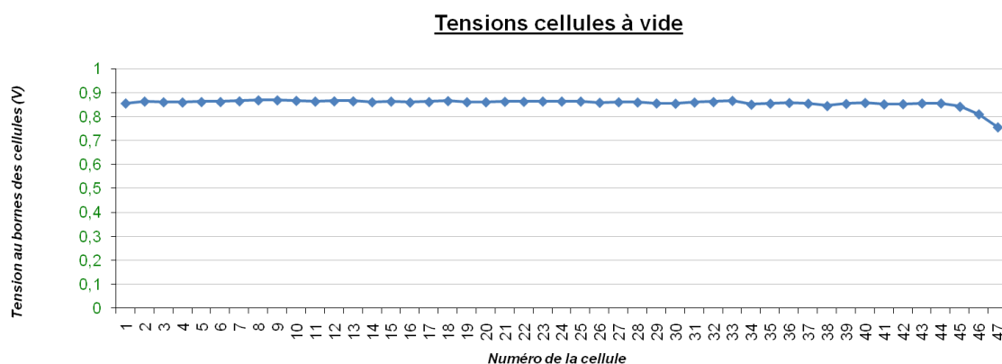
Figure 4.62 : Tension des cellules mesurée manuellement
