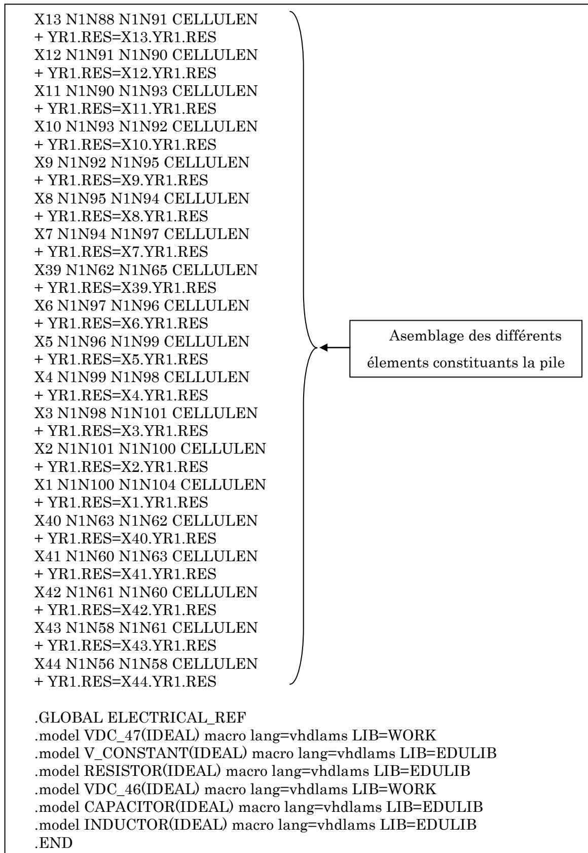
Figure 3.48 : Testbench de l'élément pile à combustible complète
