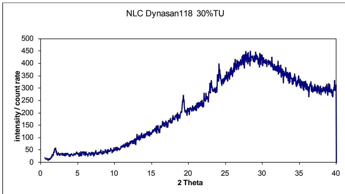
NLC 10 % lipid phase (30 % TU, 35 % Dynasan 118, 35 % oleic acid), 2 % Tween 80
