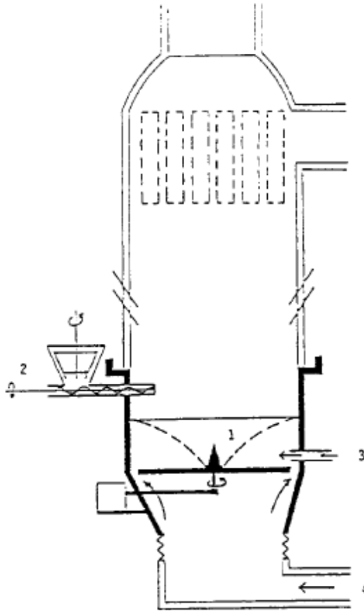
Figure 28 : Granulater rotatif à lit d'air fluidisé.
