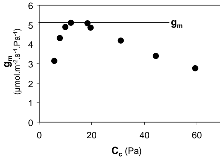
Figure 30 : Détermination de la conductance du mésophylle ( g_m ) appliquée à l'ajustement des courbes A/C_c à partir du plateau des courbes g_m/C_c .
