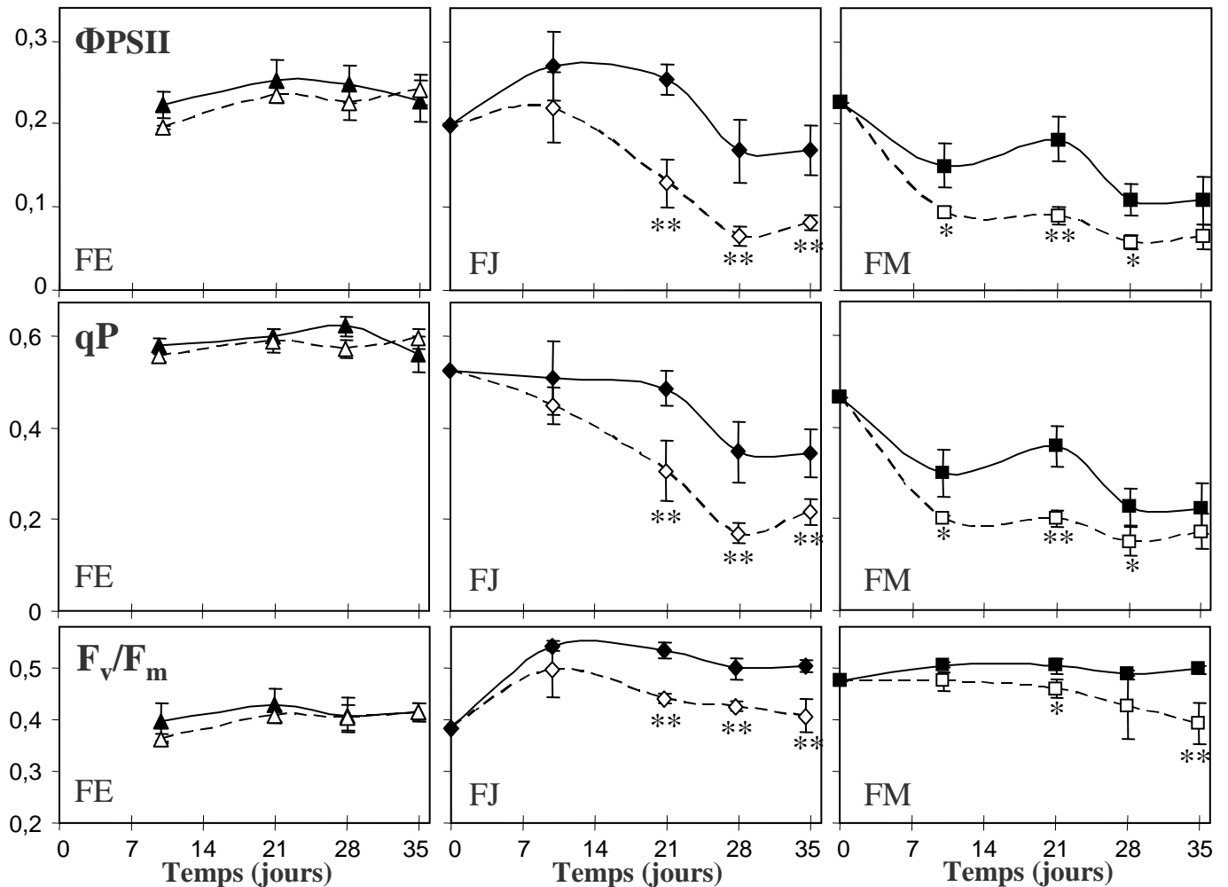
Figure 44 : Évolution des paramètres dérivés des mesures de fluorescence chlorophyllienne (rendement quantique du PSII \Phi_{PSII} , quenching photochimique qP et rapport F_v/F_m ) de feuilles à trois stades de développement (feuilles en expansion FE, feuilles jeunes FJ et feuilles matures FM) à 0, 10, 21, 28 et 35 jours de traitement (air filtré : symboles pleins et lignes continues ; ozone : symboles ouverts et lignes pointillées). Les valeurs représentent la moyenne \pm écart-type des paramètres considérés ( n = 4 ). Les étoiles indiquent une différence significative entre arbres traités et arbres témoins (test t de Student ; p < 0,05 ).
