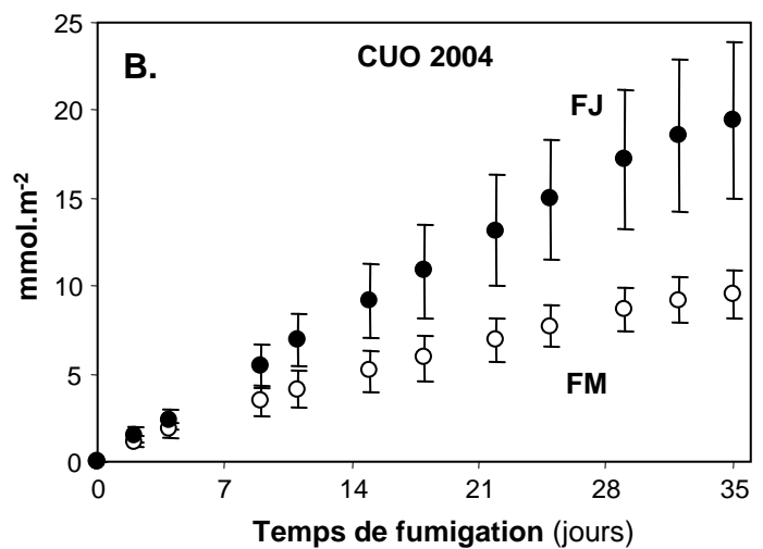
Figure 34 : Évolution des indices cumulatifs d'exposition à l'ozone au cours des trois périodes de fumigation (2004, 2006 et 2007) : A. SUM00 et d'AOT40 et B. dose cumulée d'ozone (CUO) pour l'expérience de 2004. Les valeurs de SUM00 et d'AOT40 représentent les moyennes en ppm-h des mesures dans les quatre chambres de fumigation enrichie en ozone. Le CUO a été déterminé à partir du flux stomatique pour les feuilles matures (FM) et jeunes (FJ) des peupliers traités. Pour chaque étage foliaire, moyenne et écart-type sont indiqués ( n = 8 ).
