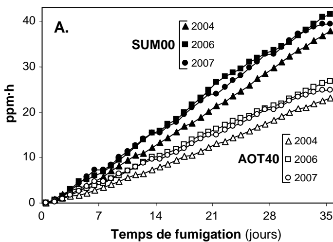
Figure 34 : Évolution des indices cumulatifs d'exposition à l'ozone au cours des trois périodes de fumigation (2004, 2006 et 2007) : A. SUM00 et d'AOT40 et B. dose cumulée d'ozone (CUO) pour l'expérience de 2004. Les valeurs de SUM00 et d'AOT40 représentent les moyennes en ppm-h des mesures dans les quatre chambres de fumigation enrichie en ozone. Le CUO a été déterminé à partir du flux stomatique pour les feuilles matures (FM) et jeunes (FJ) des peupliers traités. Pour chaque étage foliaire, moyenne et écart-type sont indiqués ( n = 8 ).
