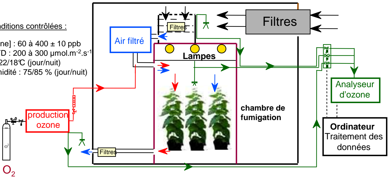
Figure 28 : A. Vue extérieure des chambres de fumigation, B. vue intérieure d'une chambre, C. schéma du dispositif expérimental de fumigation à l'ozone.
