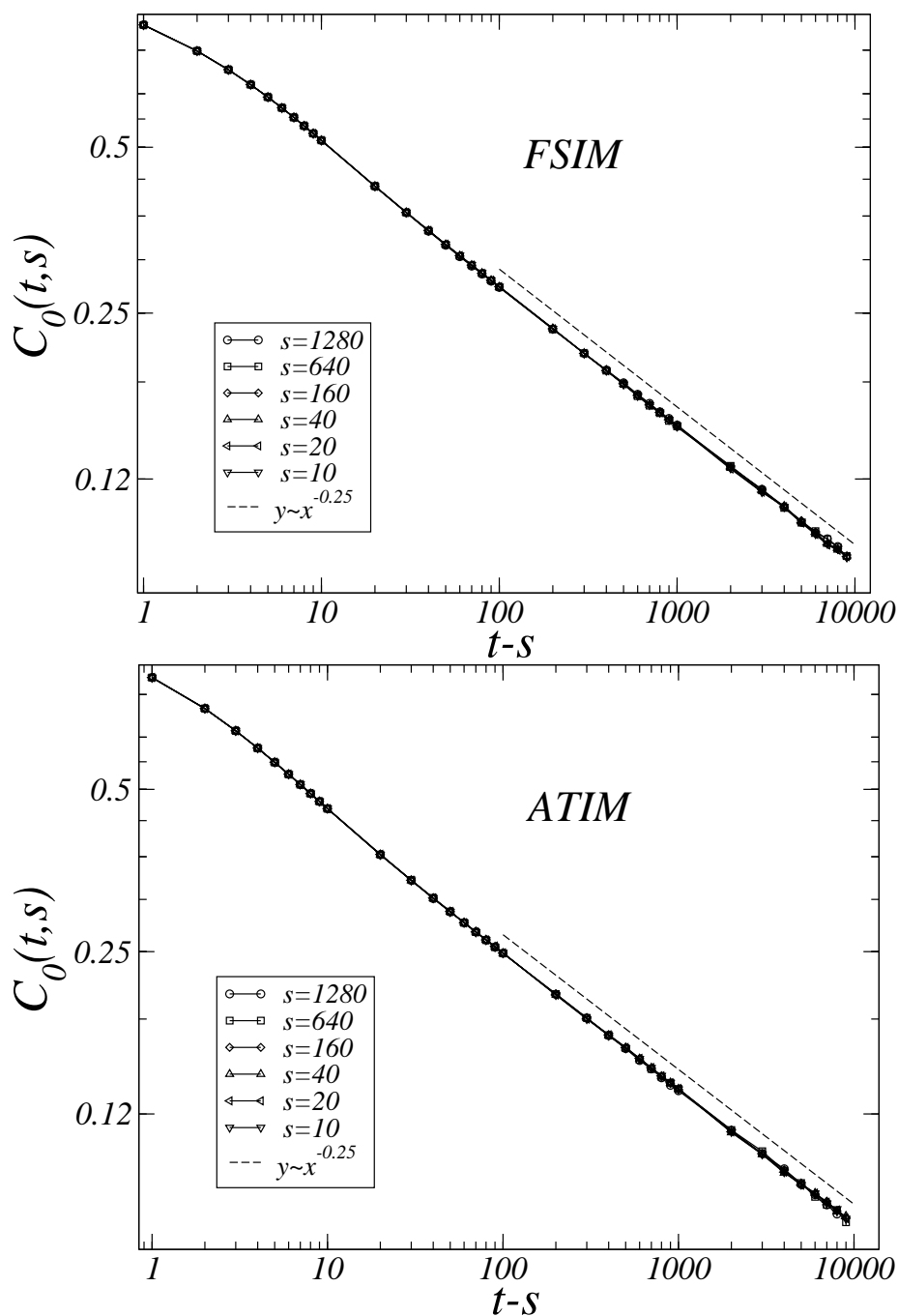
FIG. 5.12 – Fonction d'autocorrélation spin-spin à T = 0 dans le régime d'équilibre pour le FSIM (en haut) et le ATIM (en bas) tracée en fonction de t - s pour différents temps d'attente s écoulés depuis la fin de la thermalisation. On constate l'invariance par translation temporelle car toutes les courbes se superposent, comme on s'y attend à l'équilibre. La décroissance s'effectue selon (5.20) avec un exposant compatible avec a_c = 0.25 , ce qui mène à un exposant dynamique z_c en bon accord avec la valeur z = 2 du modèle XY.
