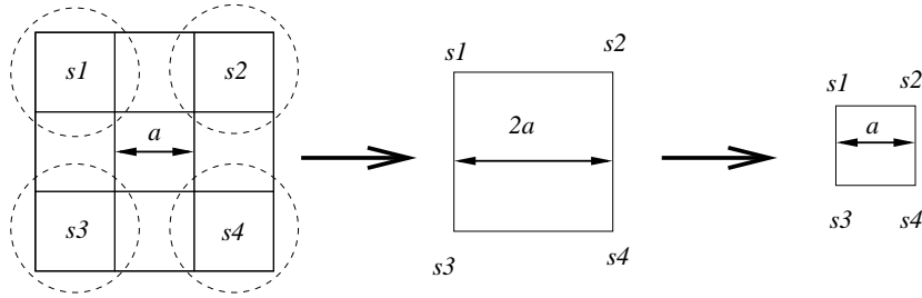
FIG. 1.10 – Transformation des blocs de spin dans l'espace réel. Les spins sont regroupés par blocs de volume 2^2 et chaque bloc est remplacé par un spin effectif s_i . Puis on norme les longueurs du système de façon à retrouver le pas de réseau initial a .
