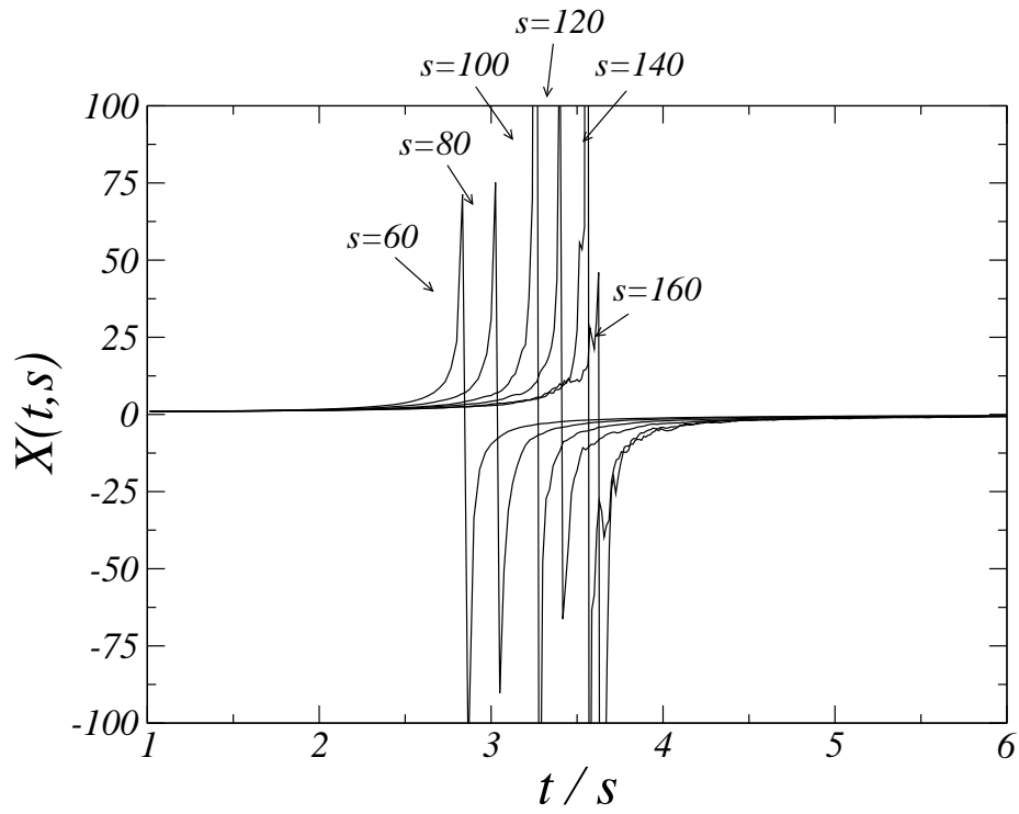
FIG. 6.9 – Le RFD pour une trempe depuis l'état fondamental jusqu'à 0.2T_{BKT}^{FF} est tracé en fonction de la variable d'échelle t/s . On observe une discontinuité qui évolue avec le temps d'attente.
