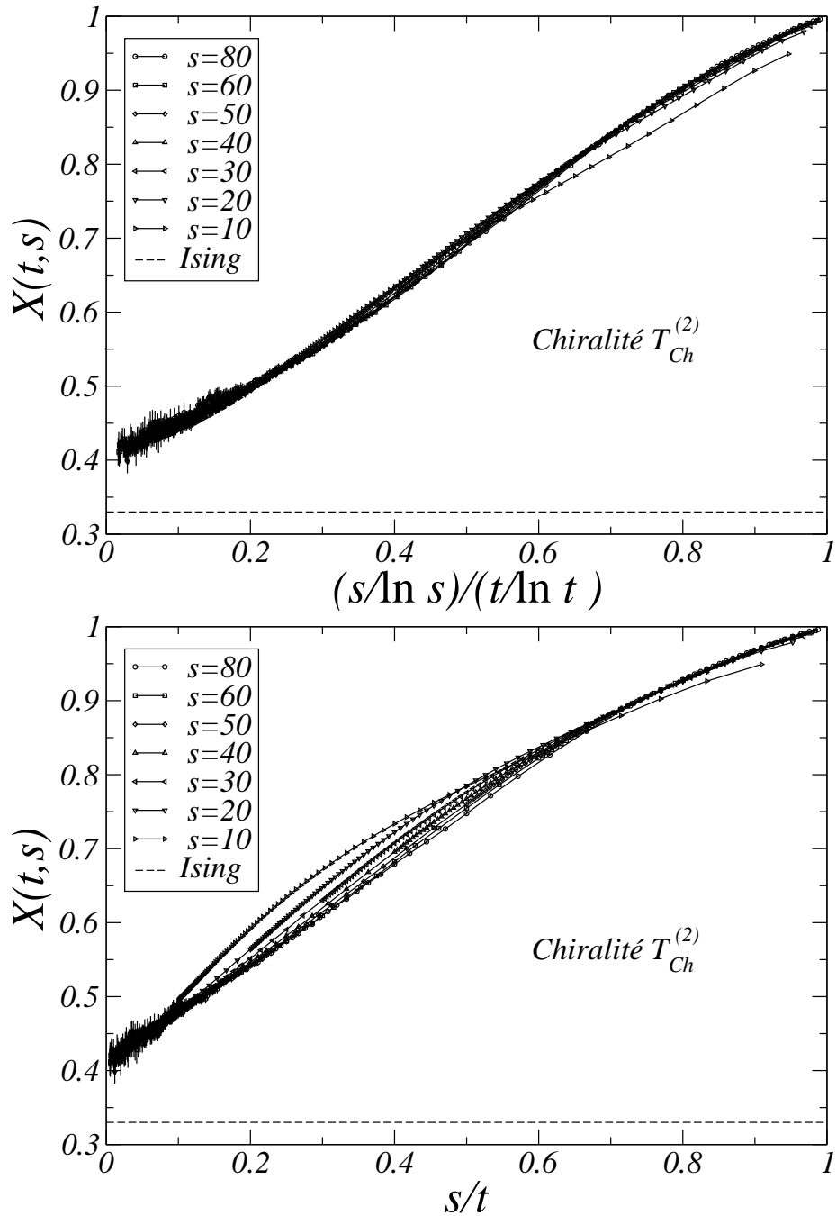
FIG. 6.15 – Le RFD de la chiralité pour une trempe depuis un état désordonné jusqu'à T_{Ch}^{(2)} est tracé en fonction de l'inverse des variables d'échelle de sorte que la valeur asymptotique se lit par extrapolation sur l'axe des ordonnées. L'ajout de corrections logarithmiques dans la variable d'échelle sous la forme \frac{s \ln t}{t \ln s} (en haut) permet d'améliorer la superposition par rapport à la variable \frac{s}{t} (en bas). On estime X_\infty = 0.405(5) en considérant les corrections logarithmiques. Une valeur compatible est obtenue sans logarithmes. Cette estimation est compatible avec la valeur estimée à la température T_{Ch}^{(1)} : le RFD est peu sensible à la température autour du point critique.
