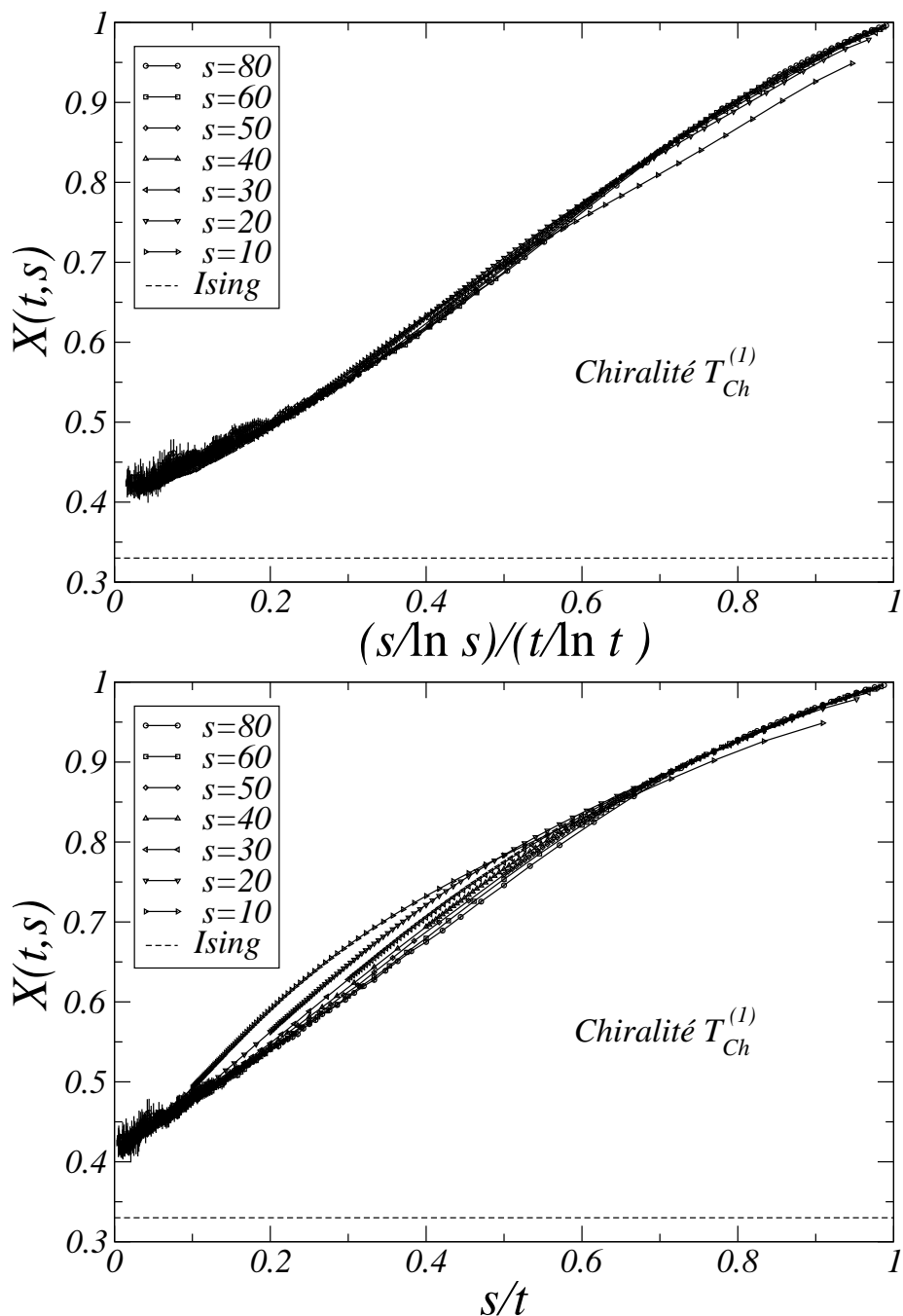
FIG. 6.14 – Le RFD de la chiralité pour une trempe depuis un état désordonné jusqu'à T_{Ch}^{(1)} est tracé en fonction de l'inverse des variables d'échelle de sorte que la valeur asymptotique se lit par extrapolation sur l'axe des ordonnées. L'ajout de corrections logarithmiques dans la variable d'échelle sous la forme \frac{s \ln t}{t \ln s} (en haut) permet d'améliorer la superposition par rapport à la variable \frac{s}{t} (en bas). On estime X_\infty = 0.410(10) avec les corrections logarithmiques. Une valeur compatible est obtenue sans logarithmes. Nos estimations sont incompatibles avec la valeur du modèle d'Ising X_\infty = 0.330(5) [Chat04].
