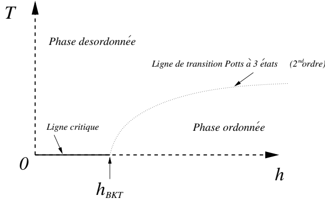
FIG. 5.4 – Diagramme de phase du ATIM dans le plan h - T [Blöt93]. Sur la ligne critique (pour T = 0 et h < h_{BKT} ) le système donne lieu à une transition de type Berezinskiï-Kosterlitz-Thouless [Bere71, Kost73, Kost74]. Puis, pour h > h_{BKT} , le système présente une phase désordonnée et une phase ordonnée avec une transition du second ordre dans la classe d'universalité du modèle de Potts à trois états.
