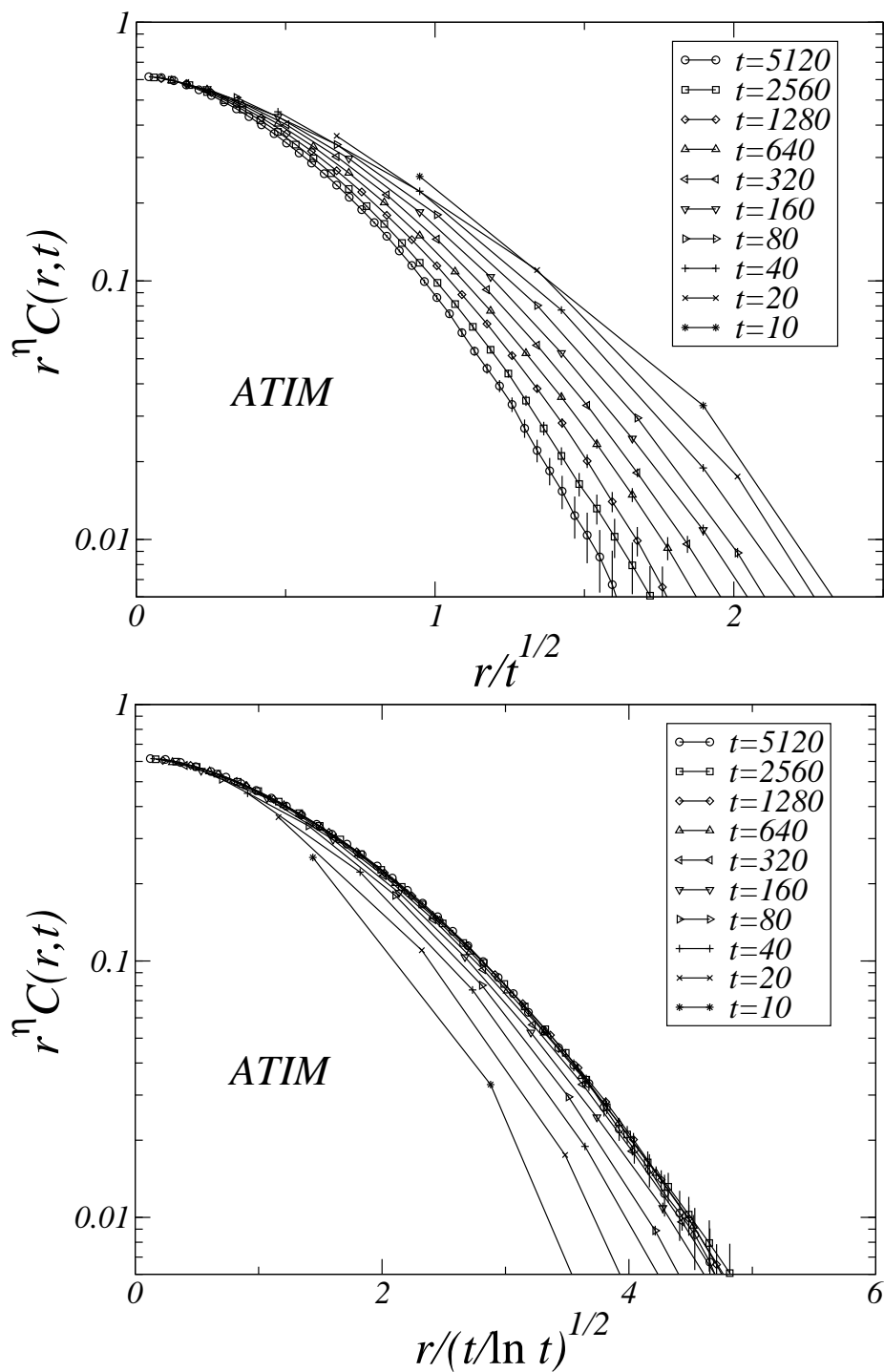
FIG. 5.14 – La fonction d'échelle C_c^{sp}(r/\xi(t)) = r^\eta C(r,t) de la corrélation spatiale spin-spin à temps égaux du ATIM trempé depuis un état désordonné jusqu'à la température critique est tracée en fonction de r/\xi(t) où \xi(t) \sim t^{1/2} (en haut) et \xi(t) \sim (t/\ln t)^{1/2} (en bas). Le temps t représente le temps écoulé depuis la trempe. Les corrections logarithmiques de la variable d'échelle permettent d'obtenir une superposition des courbes à partir de t = 320 aux barres d'erreur près. On ne constate aucune superposition lorsqu'on utilise la variable d'échelle sans correction logarithmique.
