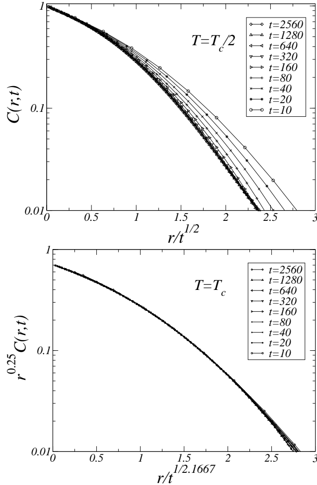
FIG. 4.9 – La fonction de corrélation spatiale spin-spin à temps égaux du modèle d’Ising pour une trempe par dynamique de Glauber depuis un état désordonné est tracée pour deux températures de trempe finale : jusque dans la phase basse température ( T_c/2 ) en haut et jusqu’au point critique en bas. Les données sont les mêmes que pour la figure 4.4 mais tracées en normant r par les longueurs caractéristiques L(t) = t^{1/2} (en haut) et L(t) = t^{1/2.1667} (en bas). Les courbes se superposent pour des temps suffisamment grands. Cette superposition illustre l’hypothèse d’échelle dynamique : il existe une seule longueur caractéristique dans le système.
