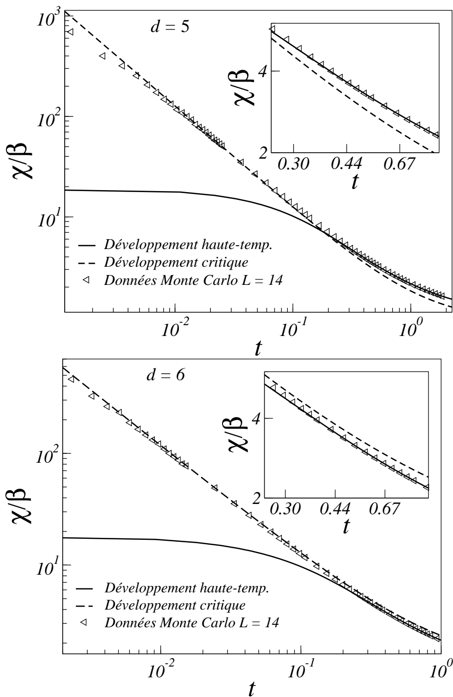
FIG. 2.2 – Afin d’illustrer la description de la susceptibilité par la méthode habituelle, des données numériques obtenues par simulations Monte Carlo en dimensions d = 5 (en haut) et d = 6 (en bas) sont comparées au développement critique de Guttman [Gutt81] obtenu par analyse de séries et le développement haute température de Gofman et al [Gofm93]. On constate que les données numériques basculent entre les deux développements. Dans l’insert se trouve un agrandissement de la région où le développement critique sort de son régime de validité. Notons que lorsque t \rightarrow 0 , les données numériques ressentent les effets de taille finie du réseau qui ne sont pas décrits par le développement critique.
