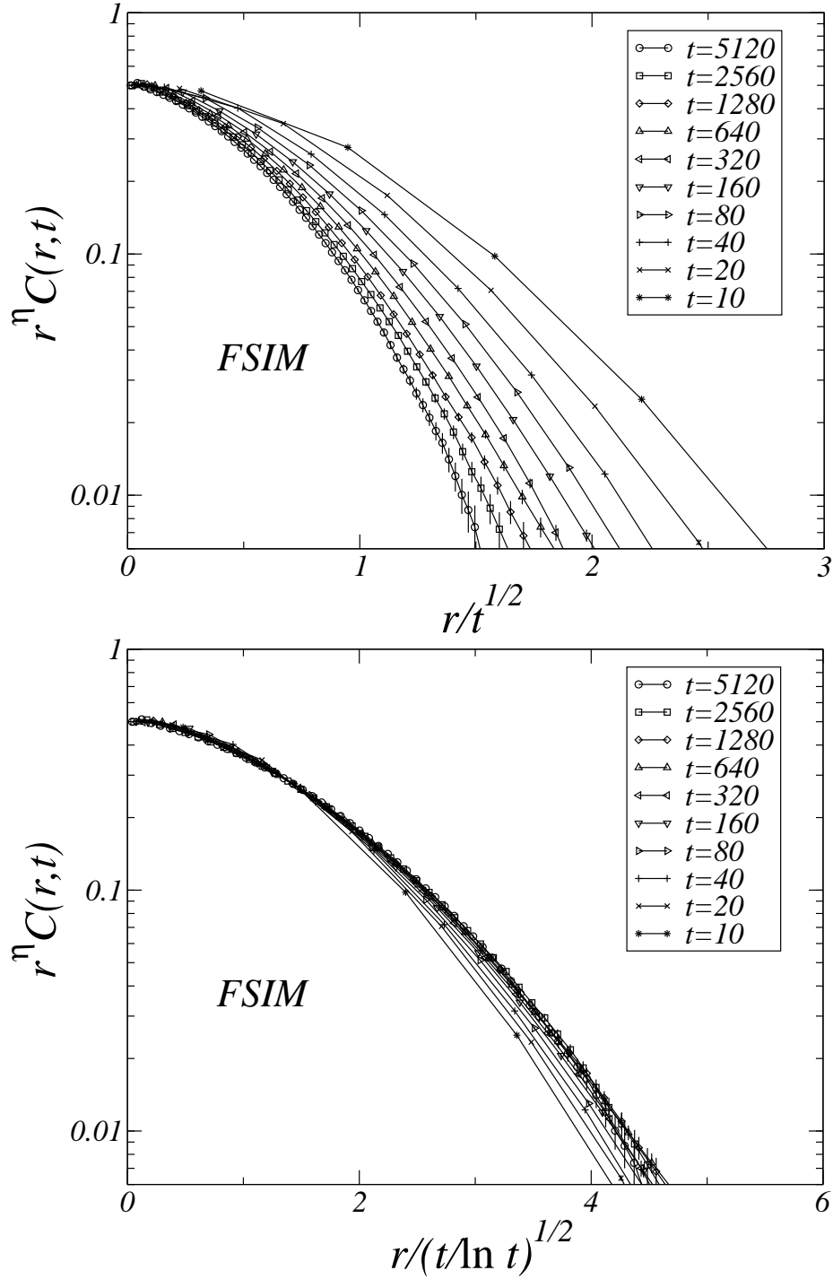
FIG. 5.13 – La fonction d'échelle C_c^{sp}(r/\xi(t)) = r^\eta C(r,t) de la corrélation spatiale spin-spin à temps égaux du FSIM trempé depuis un état désordonné jusqu'à la température critique est tracée en fonction de r/\xi(t) où \xi(t) \sim t^{1/2} (en haut) et \xi(t) \sim (t/\ln t)^{1/2} (en bas). Le temps t représente le temps écoulé depuis la trempe. Les corrections logarithmiques de la variable d'échelle permettent d'obtenir une superposition des courbes à partir de t = 160 aux barres d'erreur près. On ne constate aucune superposition lorsqu'on utilise la variable d'échelle sans correction logarithmique.
