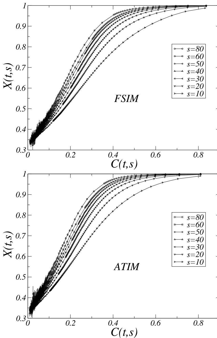
FIG. 5.24 – Le RFD X(t, s) est tracé en fonction de l'autocorrélation C(t, s) . L'absence de superposition signifie que le RFD n'est pas une fonction de C(t, s) pour les paramètres qu'on considère, comme cela fut suggéré dans le contexte du vieillissement des modèles de champ moyen de verres de spins [Cug194].
