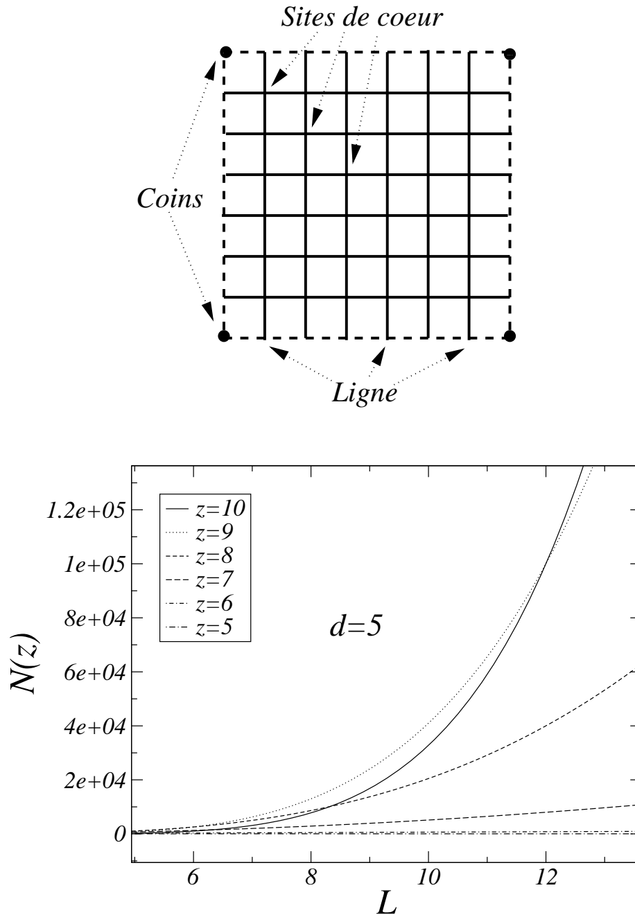
FIG. 3.8 – En haut, illustration de la coordinece en fonction de la position sur le réseau carré bidimensionnel. Le système présente des sites de cœurs de coordinece z = 4 , sur les bords la coordinece est z = 3 et sur les coins la coordinece est z = 2 . En bas, le nombre de spins de coordinece z est tracé en fonction de la taille du système pour le modèle d'Ising 5d avec des conditions de bords libres. À partir de la taille L = 12 (qui représente déjà un réseau de 12^5 = 248832 sites) le système commence seulement à avoir des spins majoritaires de volume avec une coordinece z = 10 .
