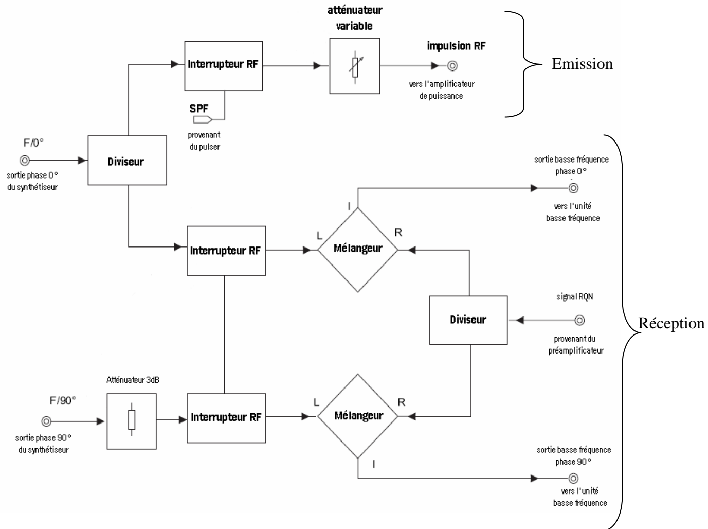
Figure II.12 : Diagramme des constituants de l'unité radiofréquence
