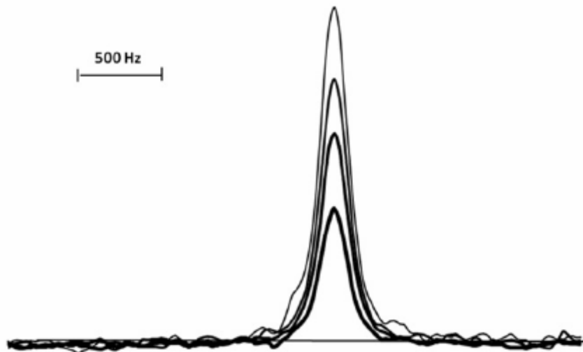
Figure II.8 : Spectres d'un échantillon de nitrite de sodium à une fréquence de 4.64 MHz, obtenus pour différentes valeurs du rapport \frac{T}{T_1} (de haut en bas : 1.3, 2, 3 et 5) et pour un temps total d'expérience constant.
