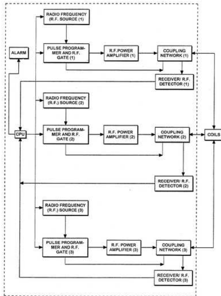
Figure I.7 : Diagramme de blocs représentant les circuits nécessaires à la réalisation d'expériences de triple résonance.
