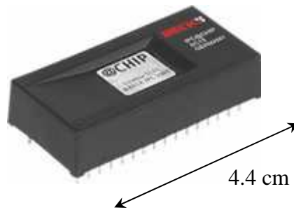
Figure III.3 : Photographie d'un composant SC- 13, Beck IPC GmbH
