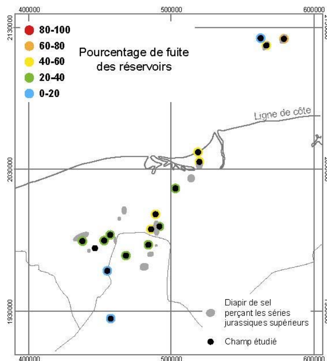
Figure 6.12. Carte des fuites des champs pétroliers mésozoïques localisés sur le horst de Reforma-Akal.
