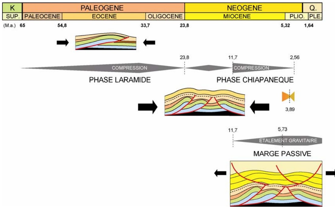
Figure 2.8. Schéma général d'évolution du bassin du Sud-Est au cours du Tertiaire.
