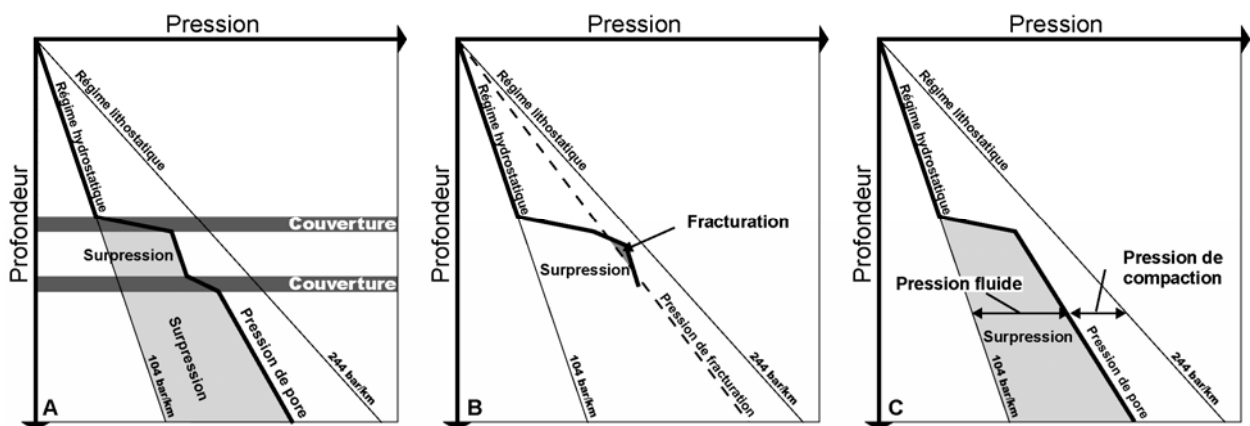
Figure 1.2. Diagrammes schématiques pression-profondeur illustrant les notions de régime de pression des bassins sédimentaires ainsi que de surpression (A), de fracturation (B), de pression de pore et de compaction (C).
