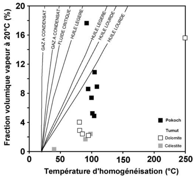
Figure 5.20. Diagramme des fractions volumiques vapeur à 20°C en fonction des températures d'homogénéisation des inclusions hydrocarbonées mesurées dans les échantillons Tumut-1 et Pokoch-1.
