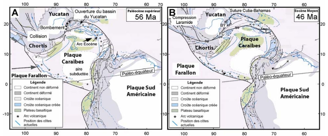
Figure 2.6. Reconstitution des positions des plaques montrant la progression vers l'Est de la plaque Caraïbes au cours du Paléogène (d'après Pindell & Kennan, 2001). (A) Positionnement au Paléocène supérieur (56 m.a.) ; (B) positionnement à l'Eocène moyen (46 m.a.).
