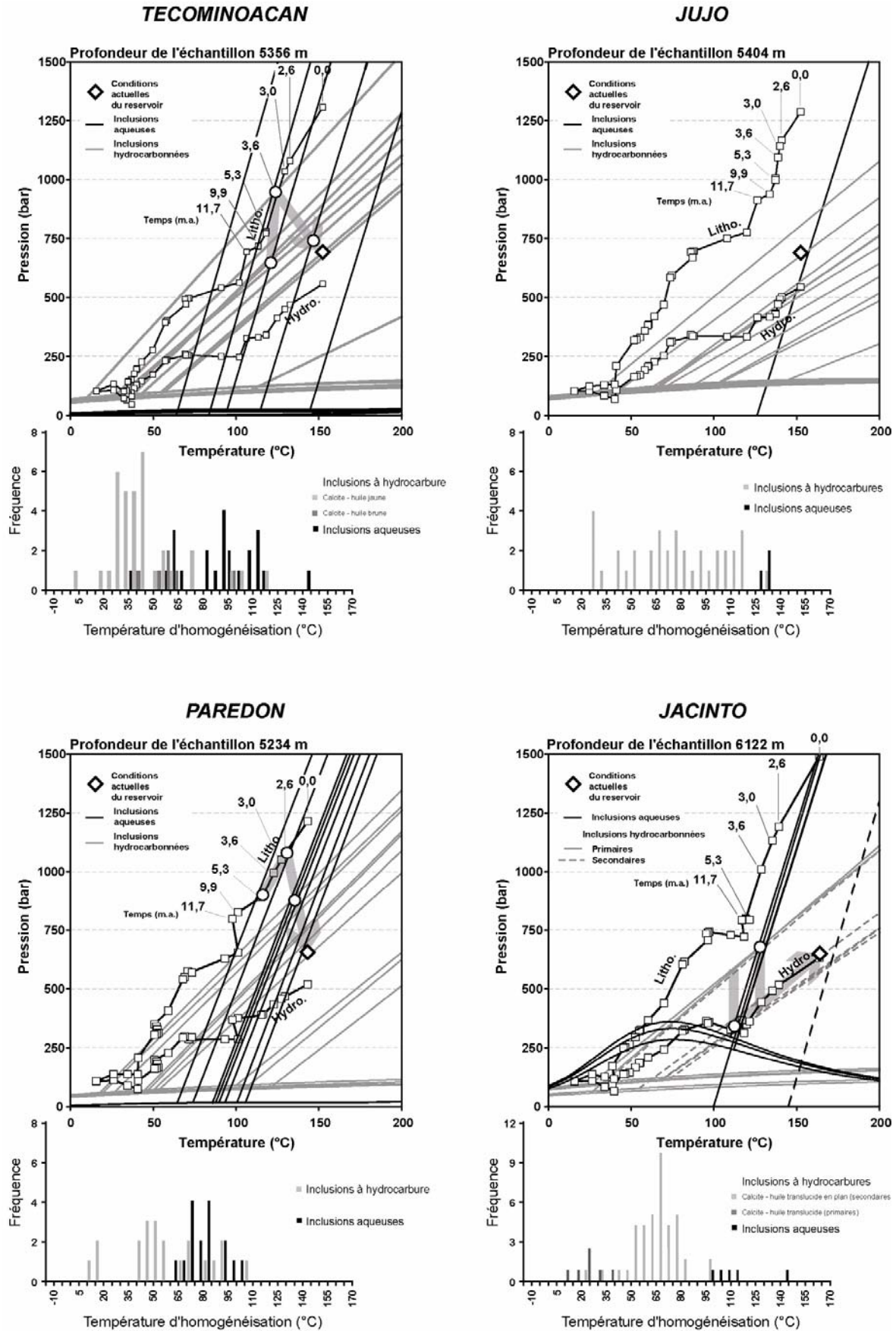
Figure 5.41. Diagramme PT rassemblant les isoplèthes et isochores obtenues des modélisations des fluides aqueux et pétroliers contenus dans les inclusions fluides des échantillons des puits Tecminoacan-447, Jujo-2A, Paredon-1 et Jacinto-24. Les courbes d'évolution des conditions hydrostatiques et lithostatiques en fonction de la température des niveaux Tithonien, calculées par PetroMod sont également reportées pour chaque puits.
