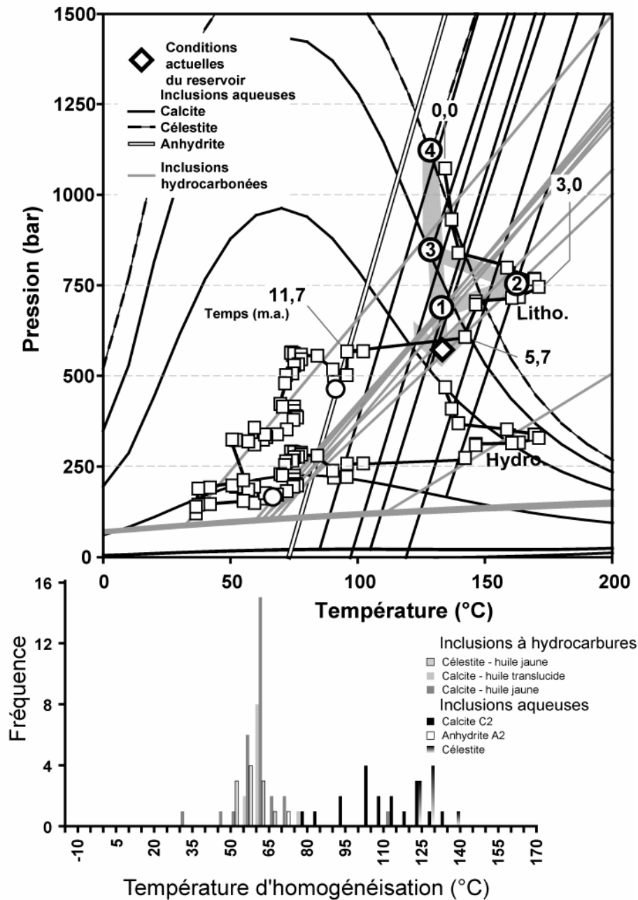
Figure 5.46. Combinaison des reconstructions PVTX , acquises par l'étude des inclusions fluides, et des modélisations des conditions PT d'enfouissement au cours du temps du puits Iride-140.
