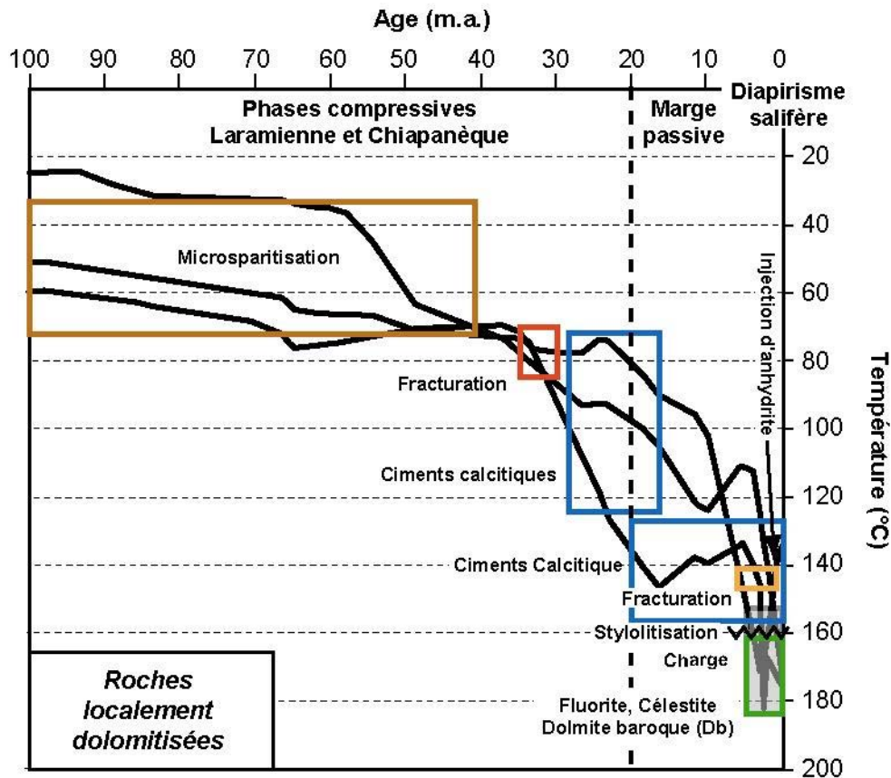
Figure 6.6. Courbes d'évolutions des températures des ensembles de puits à dolomitisation accompagnées de leurs évolutions diagenétiques.
