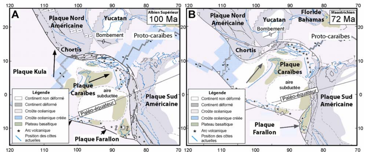
Figure 2.5. Reconstitution des positions des plaques montrant la progression NE de la plaque Caraïbes au cours du Crétacé supérieur (d'après Pindell & Kennan, 2001). (A) Positionnement à l'Albien supérieur (100 m.a.) ; (B) positionnement au Maastrichien (72 m.a.).
