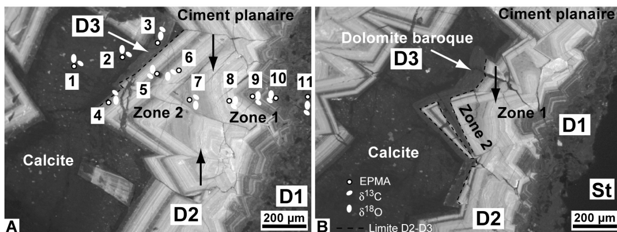
Figure 5.38. Photographies en cathodoluminescences de l'échantillon Paredon-1 montrant les positions des points de mesures réalisées par les sondes électronique et ionique.
