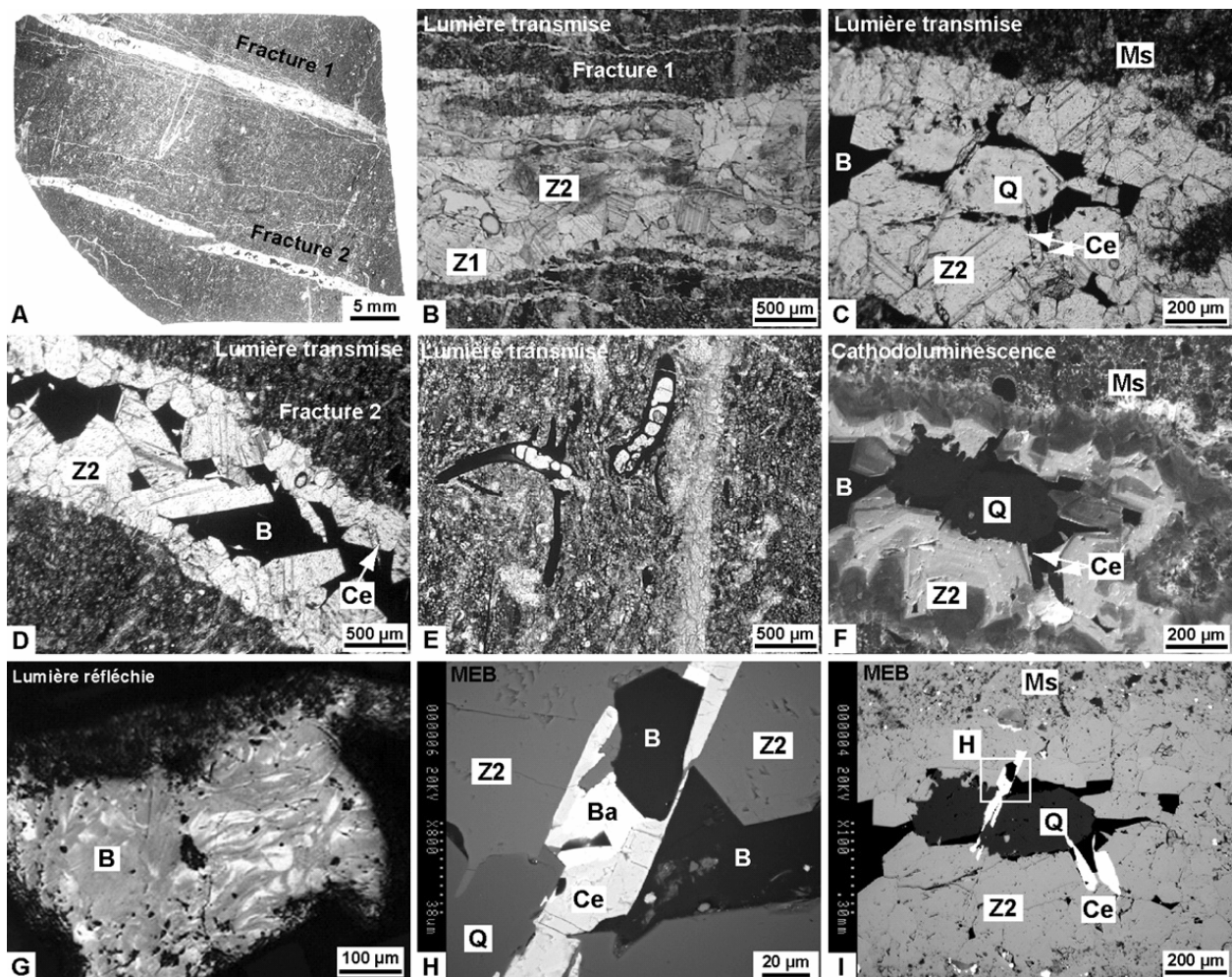
Figure 5.24. Photographies de l'échantillon du puit Caparoso 1, en macroscopie (A) en microscopie optique à transmission (B-E), à réflexion (G), en CL (F) et en MEB, mode électron rétrodiffusé (H et I). L'encarre blanc visible sur l'image I correspond au cadre de l'image H.
