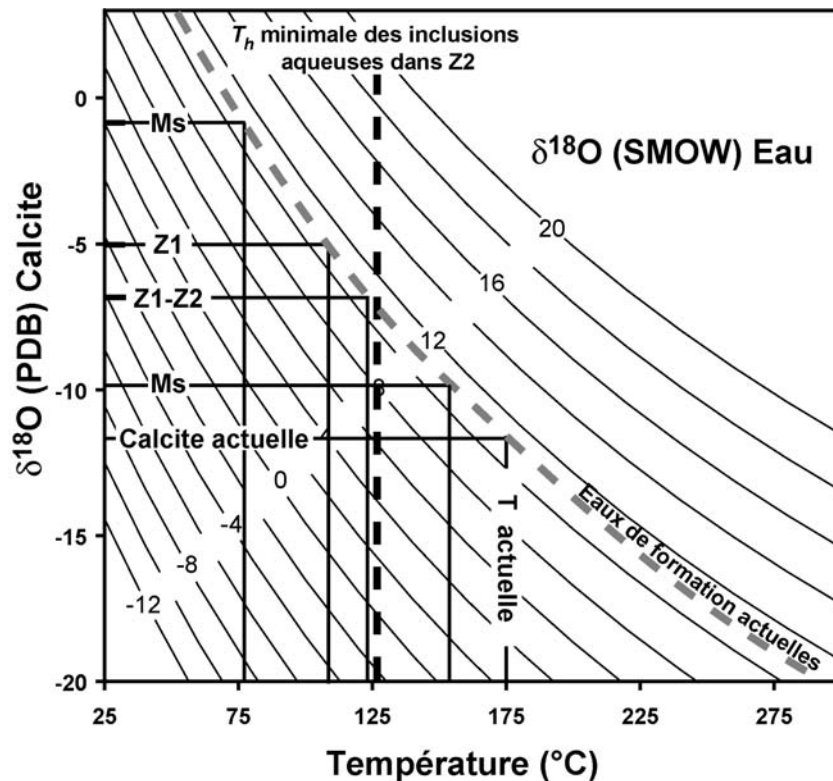
Figure 6.4. Diagramme des \delta^{18}\text{O}_{\text{PDB}} de la calcite en fonction de la température de précipitation rassemblant plusieurs courbes de valeur de \delta^{18}\text{O} de l'eau parente (SMOW) calculées d'après l'équation de fractionnement de Kim & O'Neil (1997). Cette équation est valable sur la gamme de température 25-350°C. Ms : microsparite ; Z1 : zone 1 ; Z2 : zone 2.
