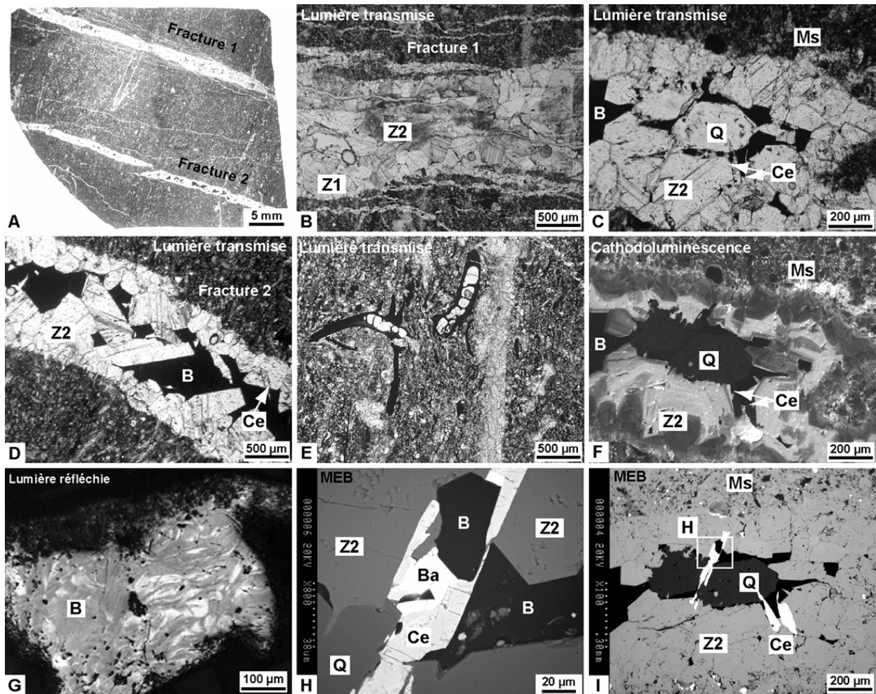
Figure 5.24. Photographies de l'échantillon du puit Caparroso 1, en macroscopie (A) en microscopie optique à transmission (B-E), à réflexion (G), en CL (F) et en MEB, mode électrons rétrodiffusés (H et I). L'encadre blanc visible sur l'image I correspond au cadre de l'image H.
