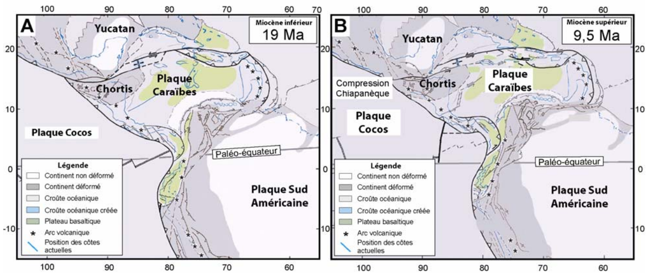
Figure 2.7. Reconstitution des positions des plaques montrant la progression vers l'Est de la plaque Caraïbes au cours du Néogène (d'après Pindell & Kennan, 2001). (A) Positionnement au Miocène inférieur (19 m.a.) ; (B) positionnement au Miocène supérieur (9,5 m.a.).
