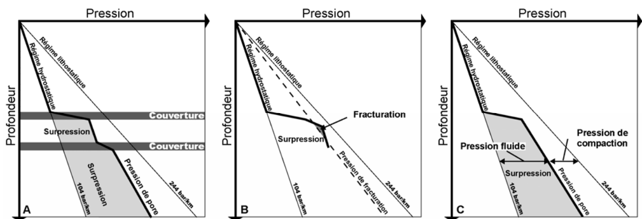
Figure 1.2. Diagrammes schématiques pression-profondeur illustrant les notions de régime de pression des bassins sédimentaires ainsi que de surpression (A), de fracturation (B), de pression de pore et de compaction (C).
