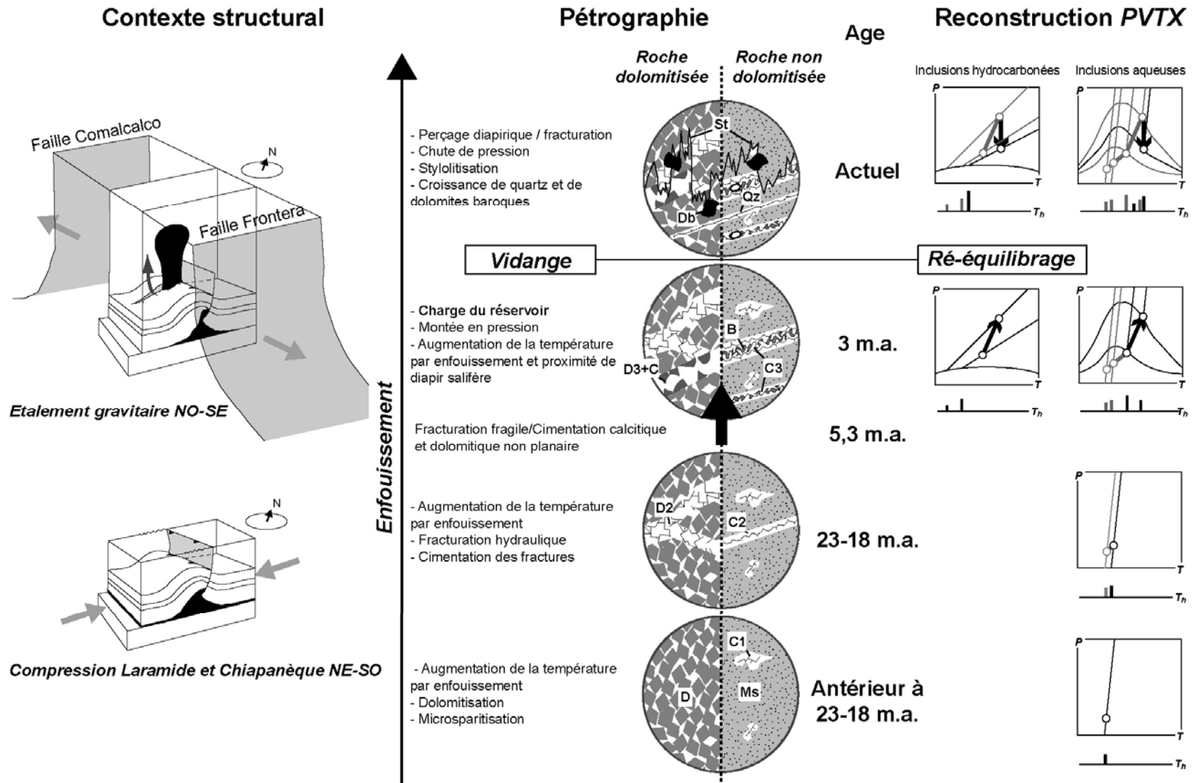
Figure 6.13. Mécanisme de remplissage et vidange des réservoirs profonds offshore et onshore du Horst de Reforma-Akal, Bassin du Sud-Est Mexicain (Golfe du Mexique).
