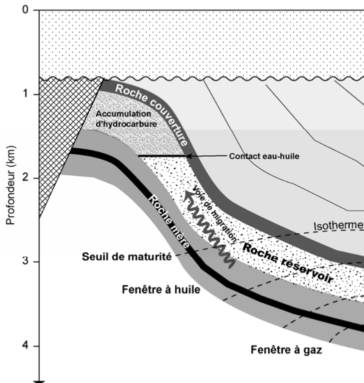
Figure 1.1. Génération, migration et piégeage des hydrocarbures (Jahn et al. , 2003 modifié).
