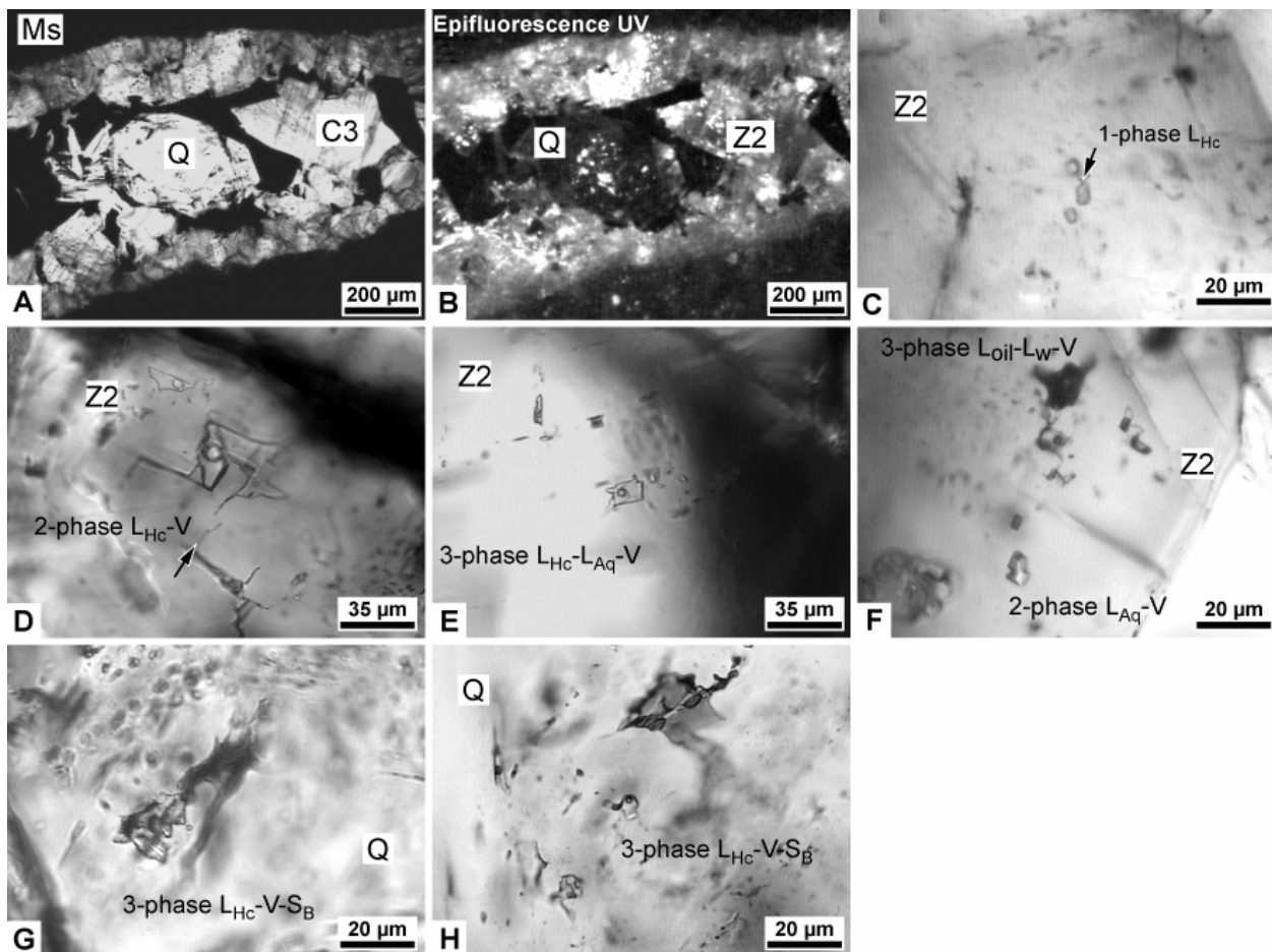
Figure 5.27. Photographies en microscopie optique à épi-fluorescence-UV et en lumière transmise montrant la distribution des inclusions hydrocarbonées dans les minéraux de la diagenèse de l'échantillon Caparoso 1, ainsi que plusieurs exemples d'inclusions fluides.
