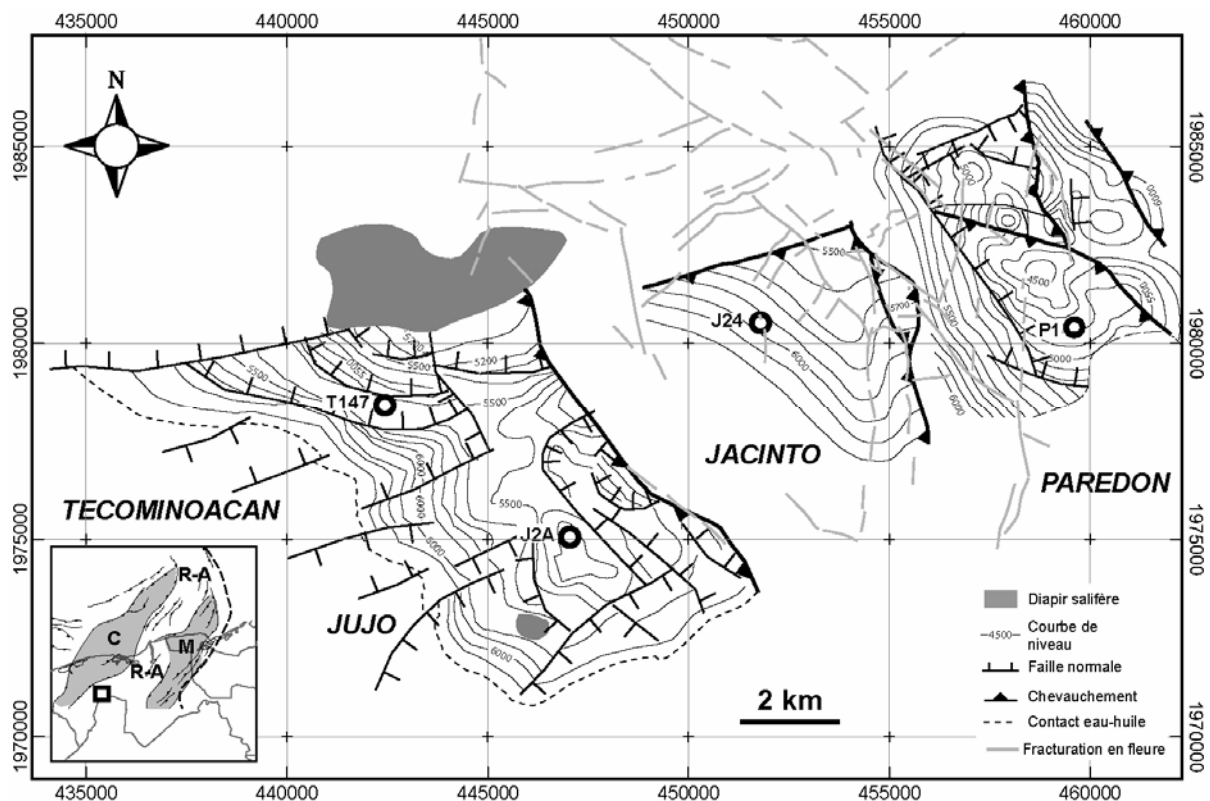
Figure 5.36. Carte du secteur de Tecminoacán rassemblant les champs pétroliers mésozoïques de Tecminoacán, Jujo, Jacinto et Paredon. Les courbes de niveaux indiquent les profondeurs du toit du Tithonien.
