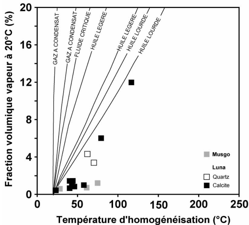
Figure 5.33. Diagramme des fractions volumiques vapeur ( \varphi_{\text{vap}} ) à 20°C en fonction des températures d'homogénéisation des inclusions hydrocarbonées mesurées dans les échantillons Luna-15 et Musgo-101.
