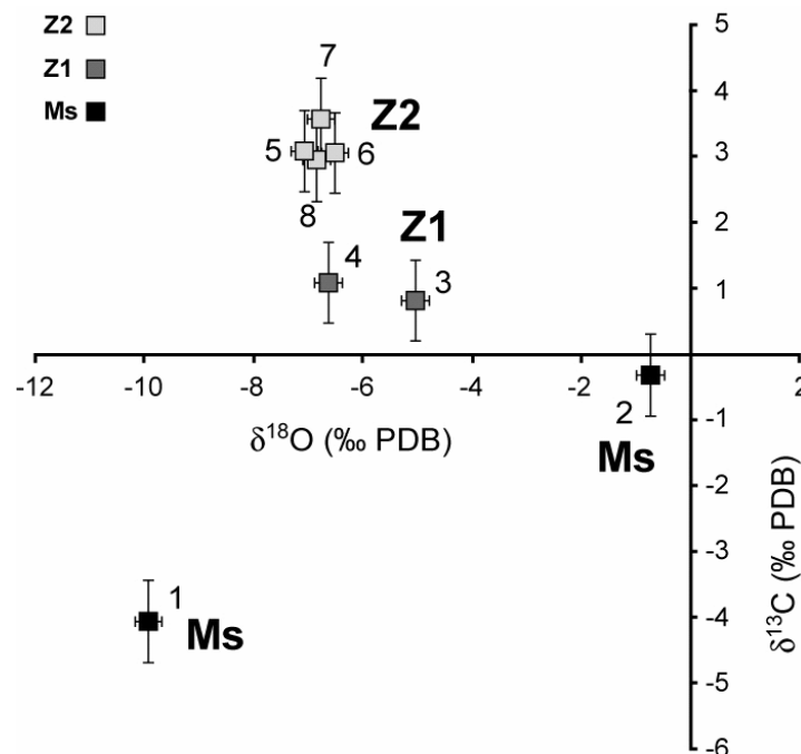
Figure 5.26. Diagramme \delta^{18}\text{O} en fonction de \delta^{13}\text{C} rassemblant l'ensemble des points de mesures réalisés à la sonde ionique sur la microsparite et les ciments calcitiques de l'échantillon du puits Caparoso 1. Les positions des points sont localisées sur la figure 5.25 (A et B).
