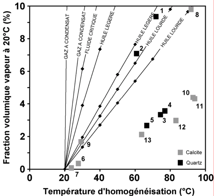
Figure 5.29. Diagramme des fractions volumiques vapeur ( \varphi_{vap} ) à 20°C en fonction des températures d'homogénéisation des inclusions hydrocarbonées mesurées dans les échantillons Caparoso 1.
