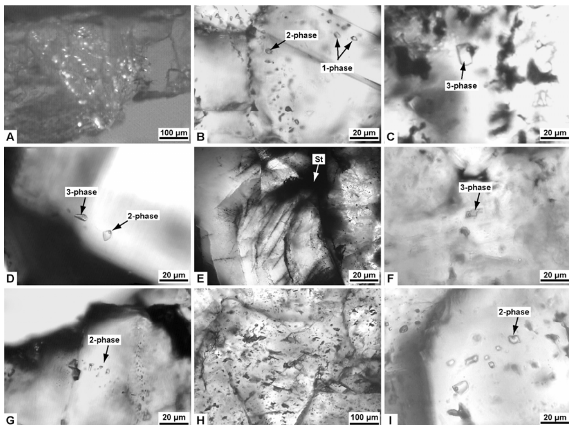
Figure 5.32. Photographies en microscopie optique à épi-fluorescence-UV et en lumière transmise montrant la distribution des inclusions hydrocarbonées dans les minéraux de la diagenèse de l'échantillon Luna 15 et Musgo 101, ainsi que plusieurs exemples d'inclusions fluides.
