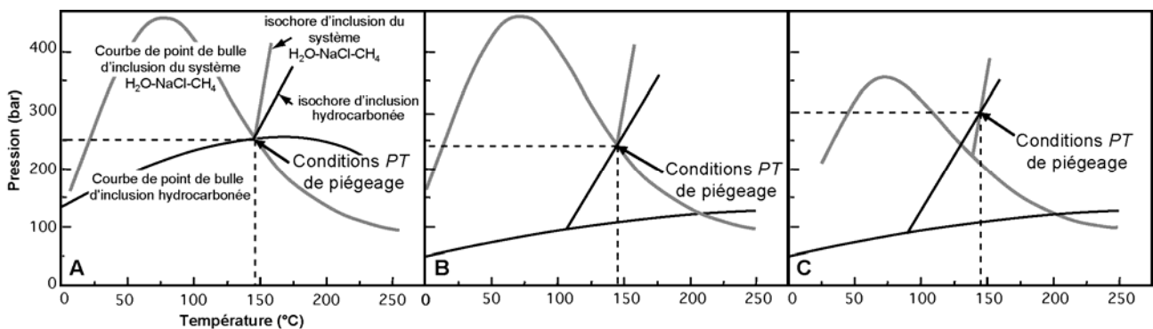
Figure 3.2. Trois différents cas possibles d'association d'inclusions hydrocarbonées et aqueuses suivant le point d'intersections des isochores. A. Inclusions hydrocarbonées et aqueuses saturées en gaz ; B. Inclusions hydrocarbonées sous-saturées en gaz et inclusions aqueuses saturées en gaz ; C. Inclusions hydrocarbonées et aqueuses sous-saturées en gaz (Pironon, 2004, modifié).
