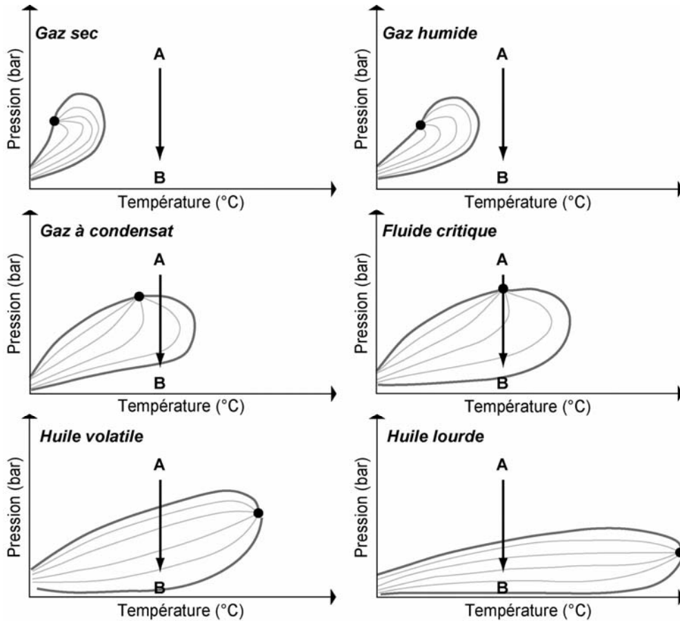
Figure 1.6. Diagrammes de phases des six compositions type de mélanges d'hydrocarbures de réservoir.
