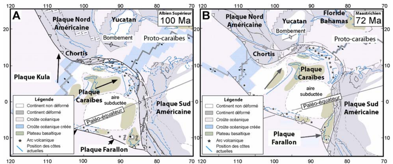
Figure 2.5. Reconstitution des positions des plaques montrant la progression NE de la plaque Caraïbes au cours du Crétacé supérieur (d'après Pindell & Kennan, 2001). (A) Positionnement à l'Albien supérieur (100 m.a.) ; (B) positionnement au Maastrichien (72 m.a.).
