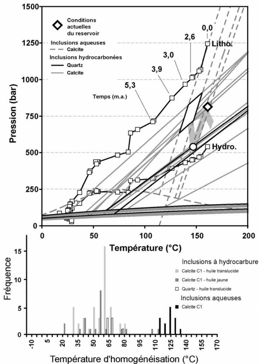
Figure 5.34. Reconstruction PVTX du puits Luna-15.
