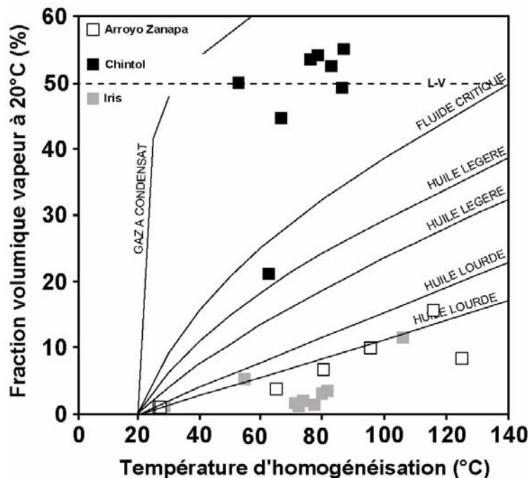
Figure 5.61. Diagramme des fractions volumiques vapeur ( \phi_{\text{vap}} ) à 20°C en fonction des températures d'homogénéisation des inclusions hydrocarbonées mesurées dans les échantillons du secteur Chintol, Iris et Arroyo Zanapa. L-V : ligne séparant les homogénéisation en phase liquide (sous la ligne) des homogénéisation en phase vapeur (au dessus de la ligne).
