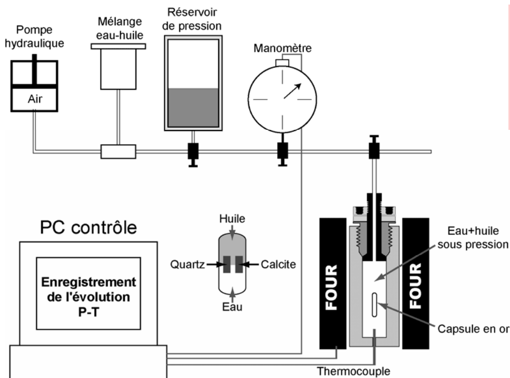
Figure 3.6. Dispositif expérimental utilisant un autoclave à pression fluide visant à créer des inclusions de synthèse.
