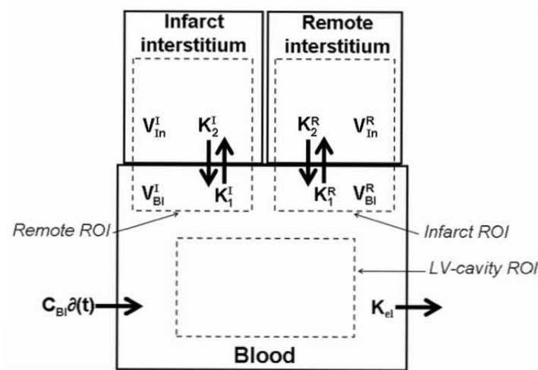
Figure 52. Représentation schématique du modèle utilisé pour l'analyse à 3 compartiments : sang (blood, BI), myocarde sain (remote, R) et infarctus (infarct, I). K_1 représente l'influx et k_2 l'efflux, k_{el} la constante d'élimination du compartiment sanguin, V_{In} le volume de distribution interstitiel du Gd-DTPA, V_{BI} le volume de distribution sanguine et C_{BI} \ddot{a}(t) la concentration initiale de Gd-DTPA.
