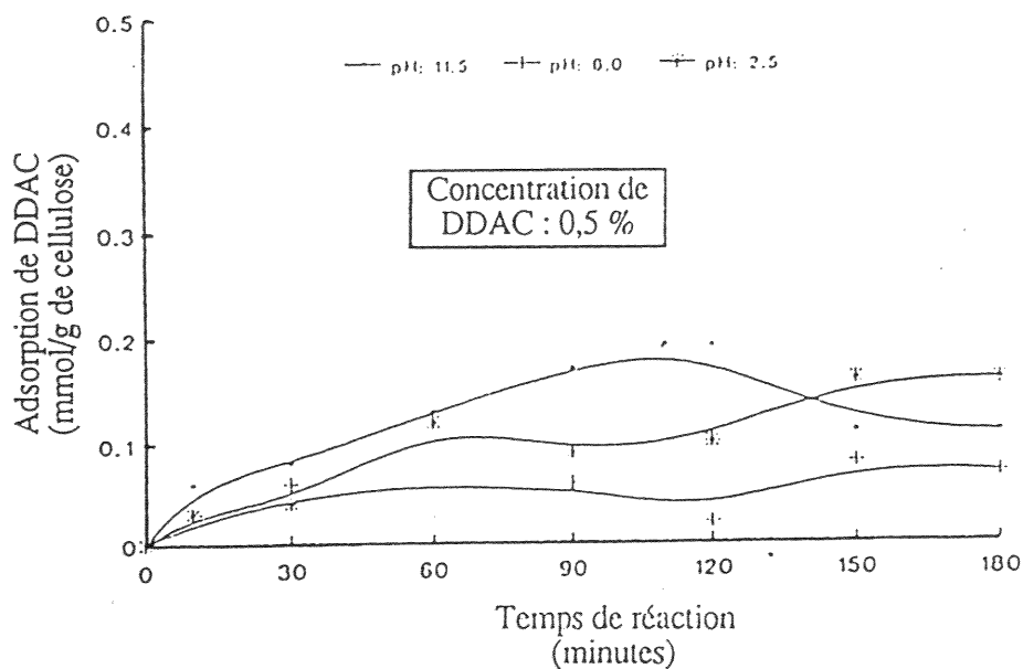
Figure 10 : L'adsorption de chlorure de didécyl diméthyl ammonium (DDAC) sur la cellulose à différents pH. (Preston et al.1991)
