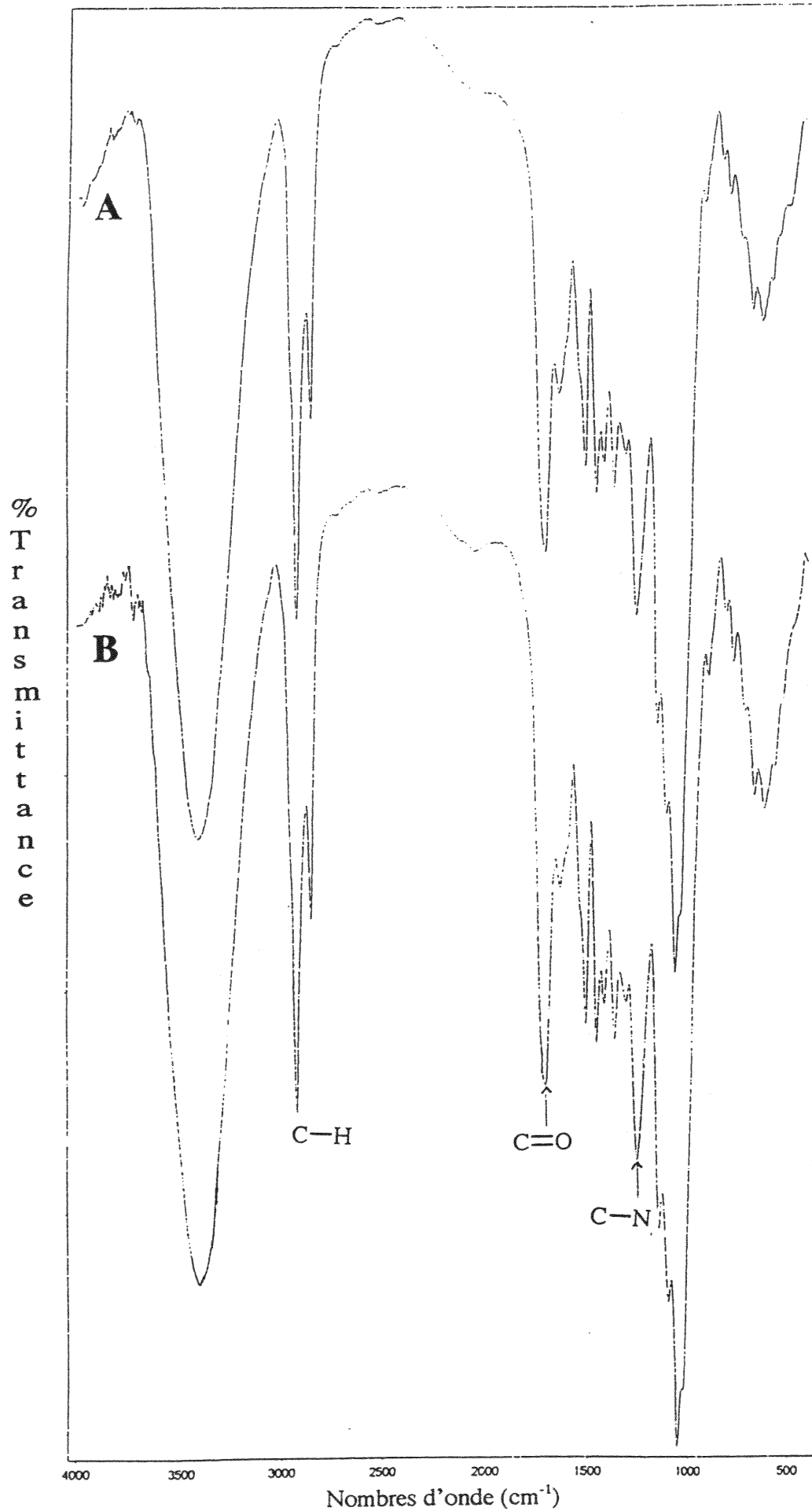
Figure 46 : Spectres infrarouge de la sciure d'Épicéa modifiée par le mélange d'azidures d'acyle gras et mise dans le milieu de culture sans champignon pendant 21 jours. A : en absence de glucose et B : en présence de glucose
