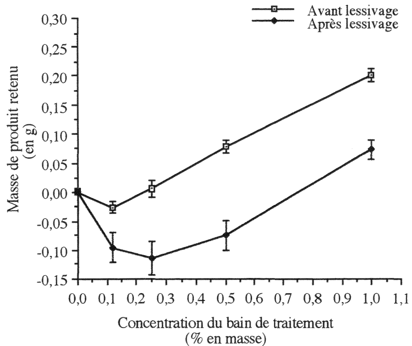
Figure 32 : Quantité d'hexafluorophosphate d'ammonium B_{80}, PF_6 retenu en gramme sur des éprouvettes de Hêtre en fonction des différentes concentrations (% en masse)
